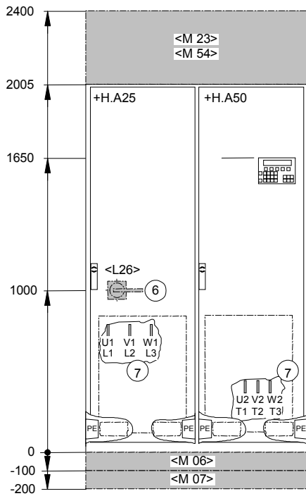
Габаритный чертёж 4: 380 В до 480 В
