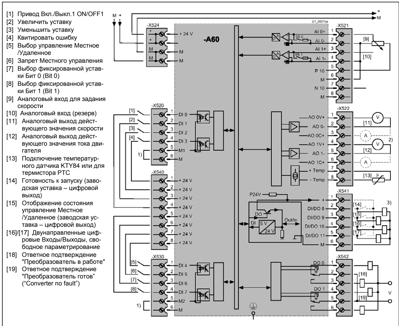
Интерфейсный модуль для внешних подключений
