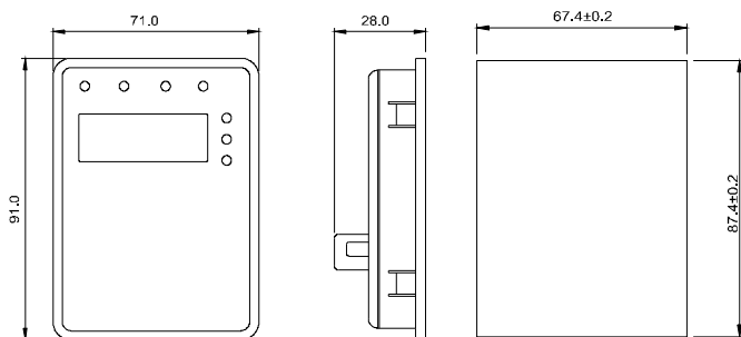
Рисунок 3.4. Размеры малой клавиатуры.
