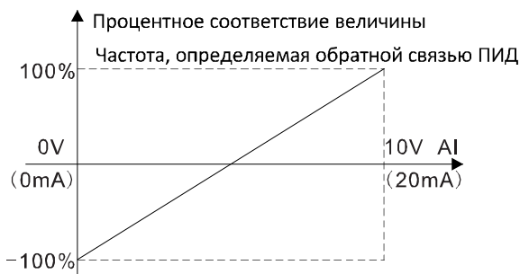
Рисунок 6.14. Отношение между сигналом аналогового входа AI и соответствующей величиной.
