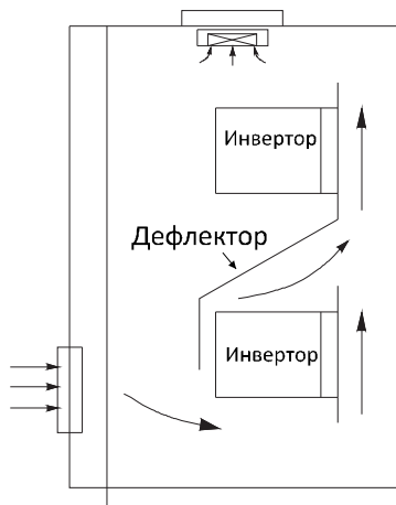
Рисунок 3.3. Установка нескольких преобразователей
