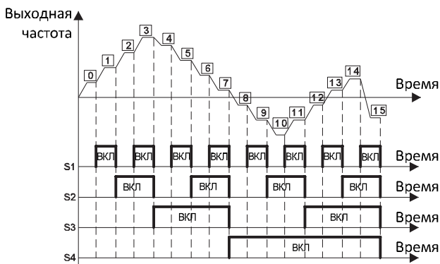
Рисунок 6.26. Схема многоступенчатого регулирования скорости.
