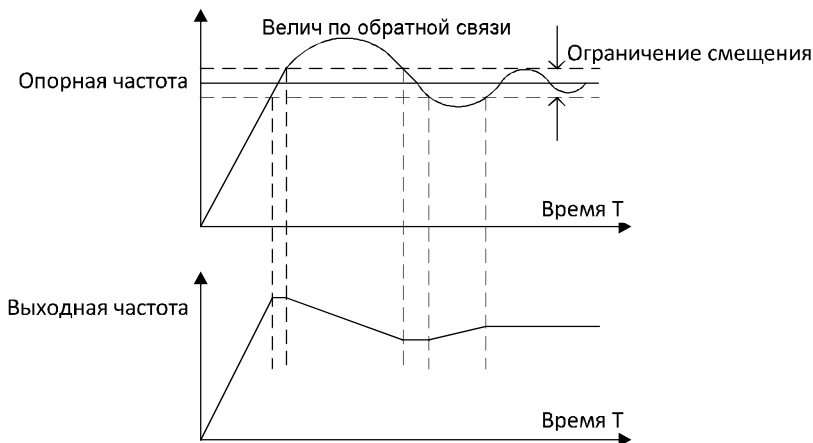
Рисунок 6.25. Отношения ограничения смещения и выходной частоты.
