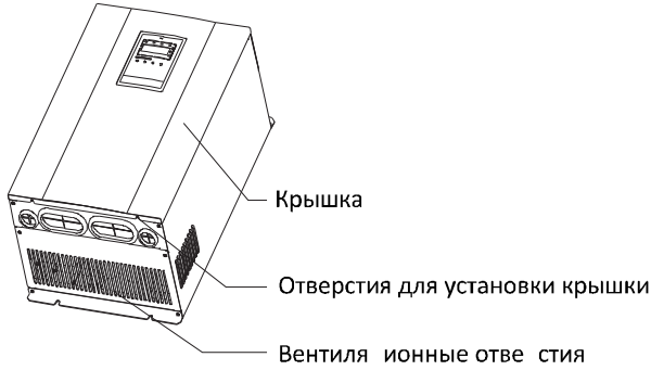
Рисунок 1.3. Компоненты инверторов (18.5 кВт и больше)
