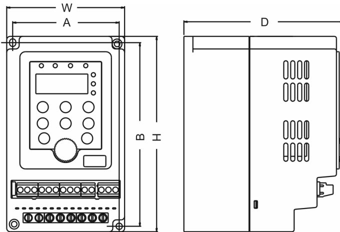
Рисунок 1.4. Габаритные размеры (0.4–0.75 кВт однофазный 220 В пер. тока)
