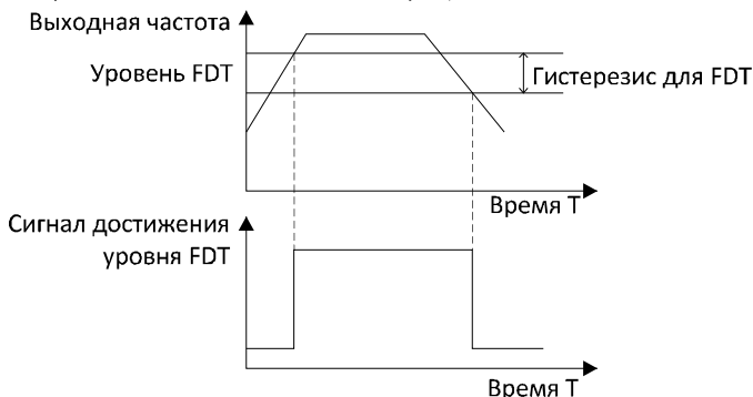
Рисунок 6.18. Уровень FDT и гистерезис FDT.
