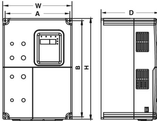
Рисунок 1.5. Габаритные размеры (0,75–15 кВт)
