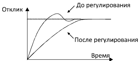
Рисунок 6.21. Подавление переуправл.Время
