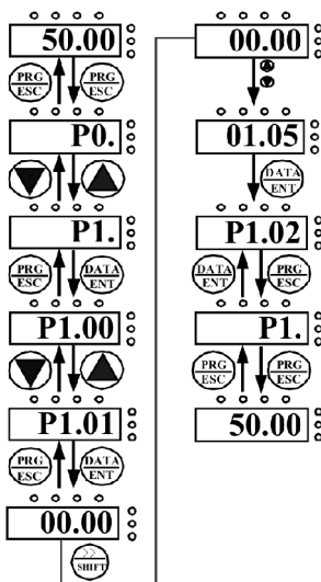
Рисунок 5.2. Блок-схема установки параметров
