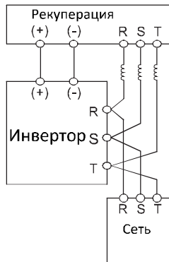
Рисунок 4.15. Электромонтаж цепи рекуперации
