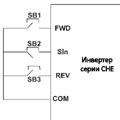
Рисунок 6.13. Трехпроводное управление режим 2.
