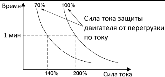
Рисунок 6.27. Кривые защиты двигателя от перегрузки по току.
