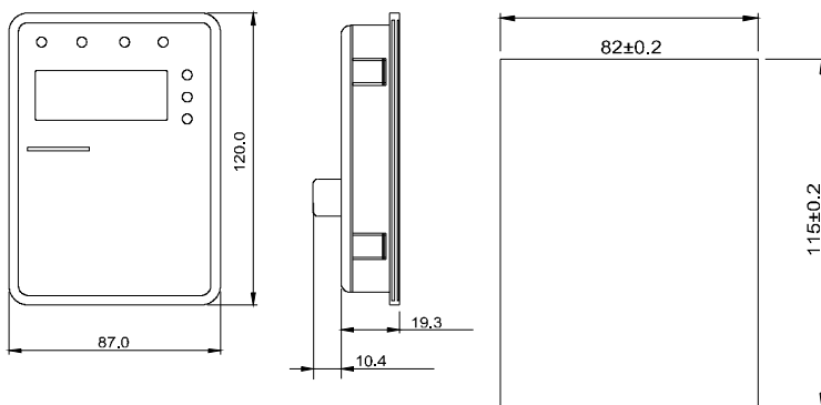
Рисунок 3.5. Размеры большой клавиатуры
