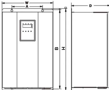
Рисунок 1.6. Габаритные размеры (18,5–110 кВт)
