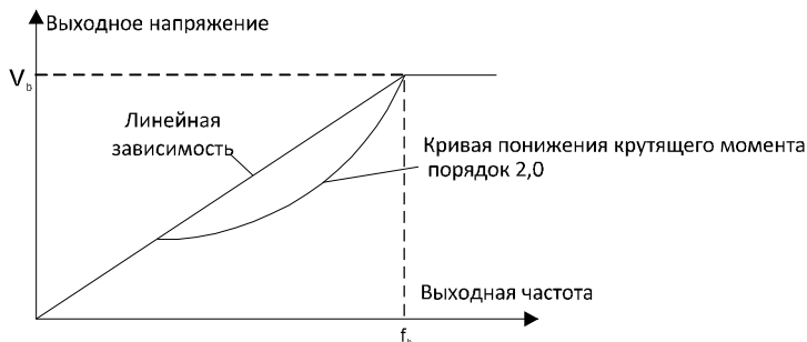
Рисунок 6.8. Вольт-частотная характеристика
