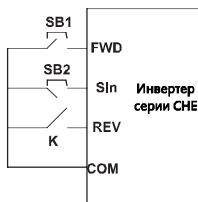
Рисунок 6.12. Трехпроводное управление режим 1.
