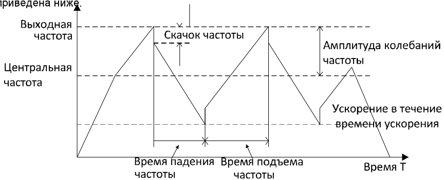
Рисунок 6.17. График управления двигателем с колебаниями частоты.
