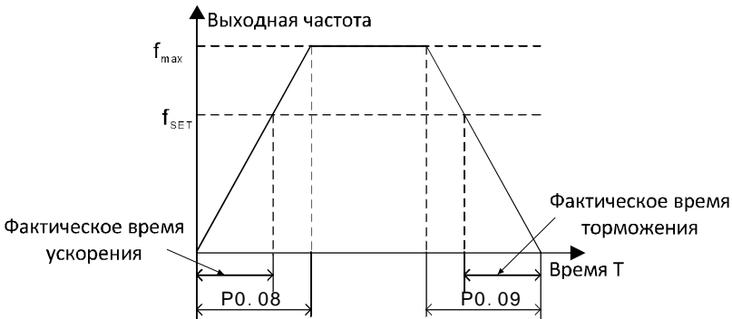
Рисунок 6.1. Времена ускорения/торможения
