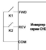
Рисунок 6.11. Двухпроводное управление режим 2.
