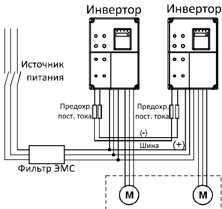
Рисунок 4.16. Электромонтаж общей шины постоянного тока
