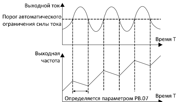
Рисунок 6.29. Функция защиты от сверхтоков.
