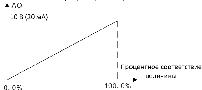
Рисунок 6.15. Отношение между сигналом аналогового выхода АО и соответствующей величиной.
