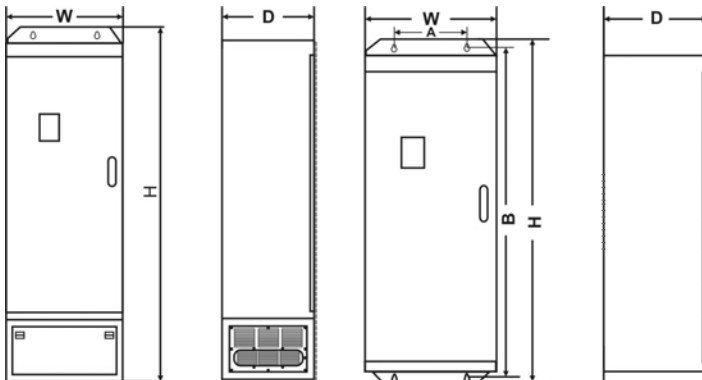
Рисунок 1.7. Габаритные размеры (132–500 кВт)
