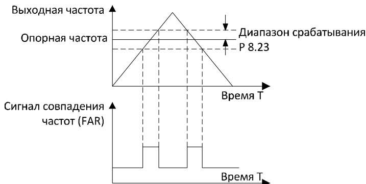
Рисунок 6.19. График сигнала совпадения частот (FAR).
