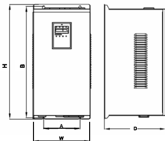
Рисунок А. 6. Габаритные размеры (22–55 кВт)
