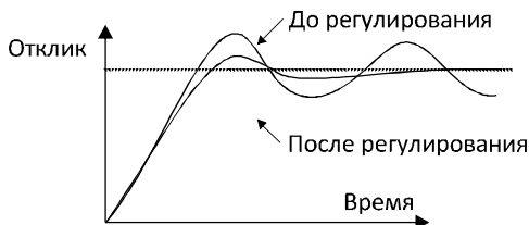
Рисунок 6.23. Подавление низкочастотных осцилляций.
