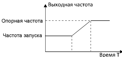
Рисунок 6.3. График пуска
