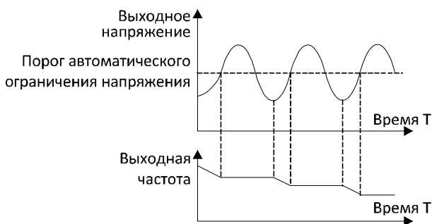
Рисунок 6.28. Функция защиты от перенапряжения.
