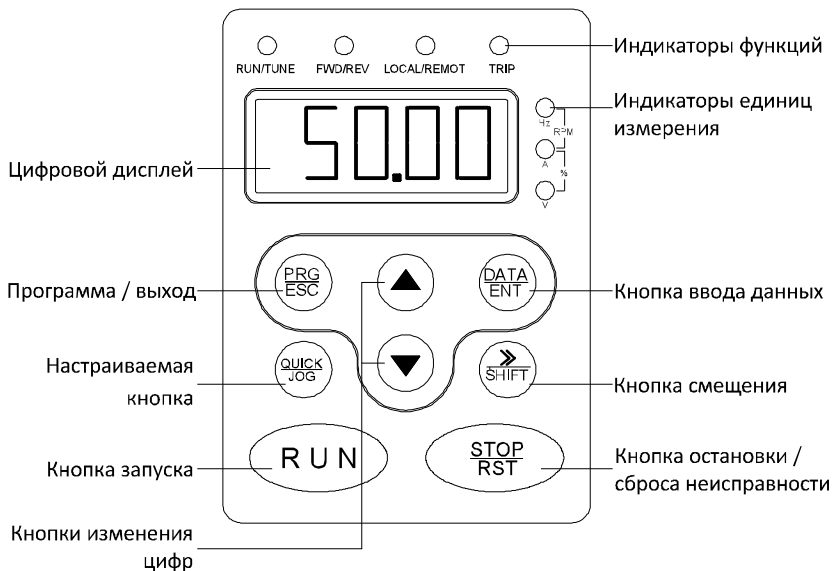
Рисунок 5.1. Схема панели оператора
