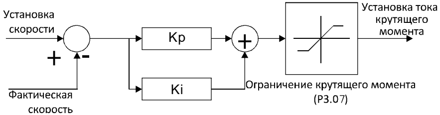
Рисунок 6.6. Схема регулятора скорости ASR
