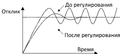
Рисунок 6.24. Подавление высокочастотных осцилляций.
