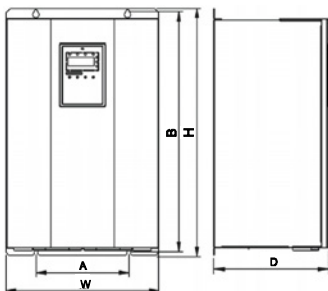
Рисунок А. 5. Габаритные размеры (11–18.5 кВт)
