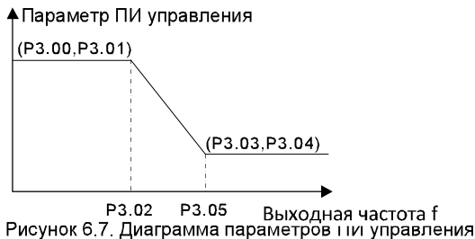
Рисунок 6.7. Диаграмма параметров пи управления
