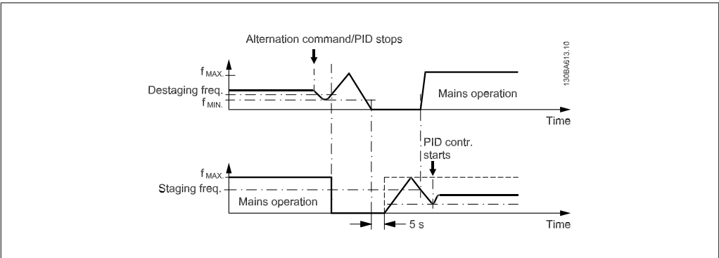
Рисунок 2.2: Конфигурация с медленным режимом
