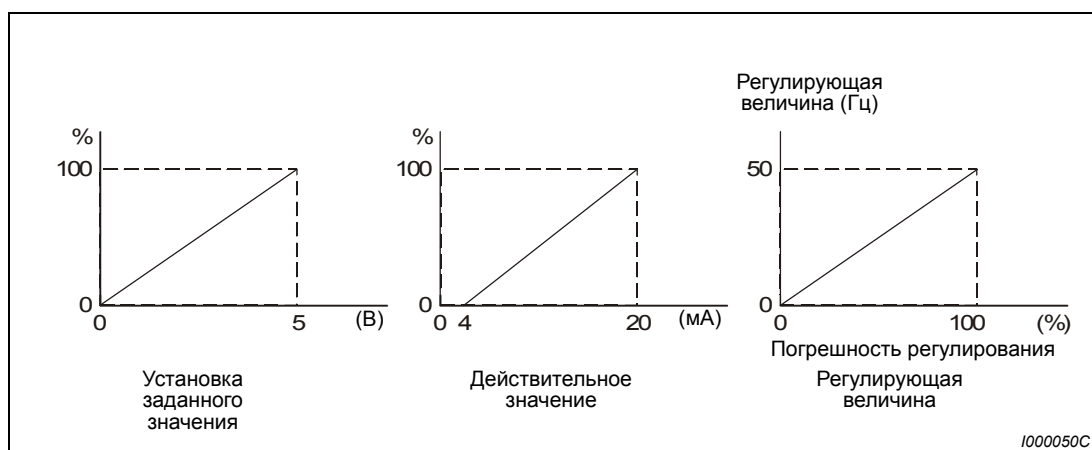
Рис. 6-149: Калибровка входов
