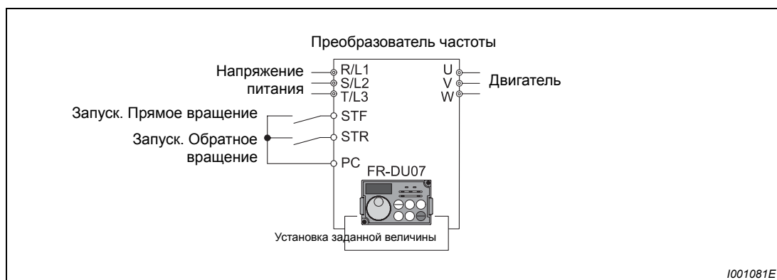
Рис. 4-18: Внешнее управление
