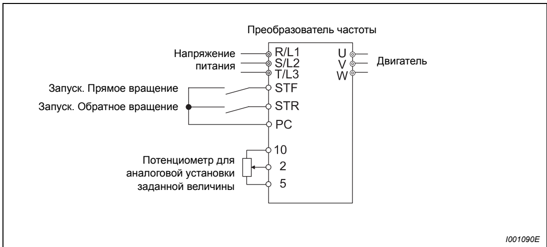
Рис. 4-23: Аналоговая установка заданного значения напряжения через потенциометр
