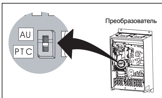
Рис. 6-41: Переключатель AU/PTC
