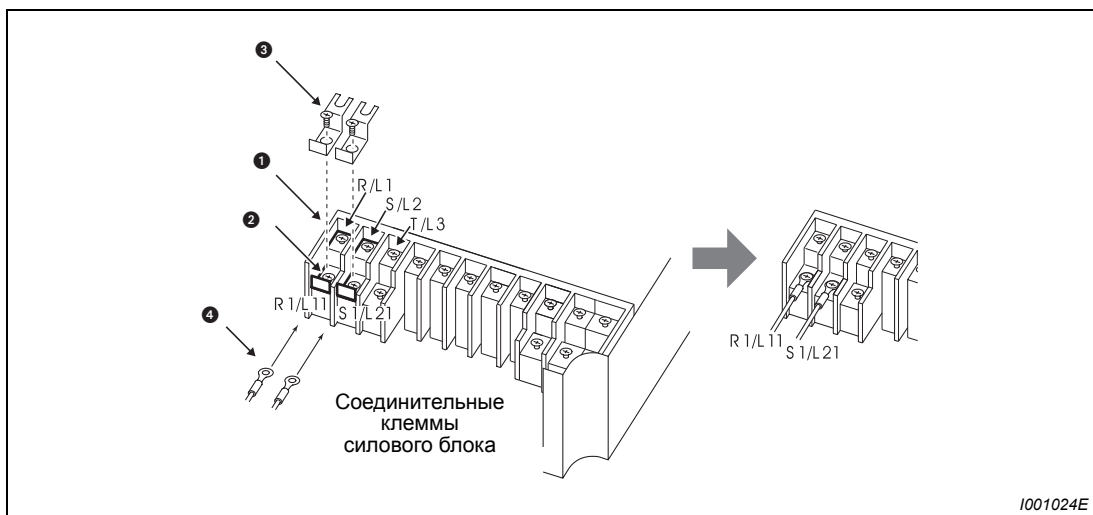
Рис. 3-12: Соединительные клеммы
