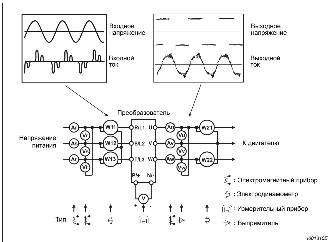
Рис. 8-12: Измерения на силовых элементах
