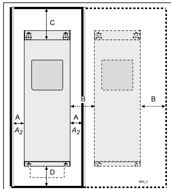
Рисунок 5-11. Вентиляционные промежутки
