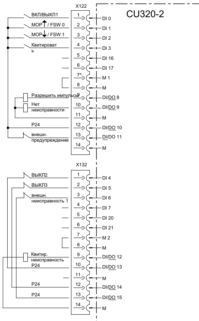
Изображение 6-14 Назначение клемм управляющего модуля при предварительной установке «Клеммы CU»
