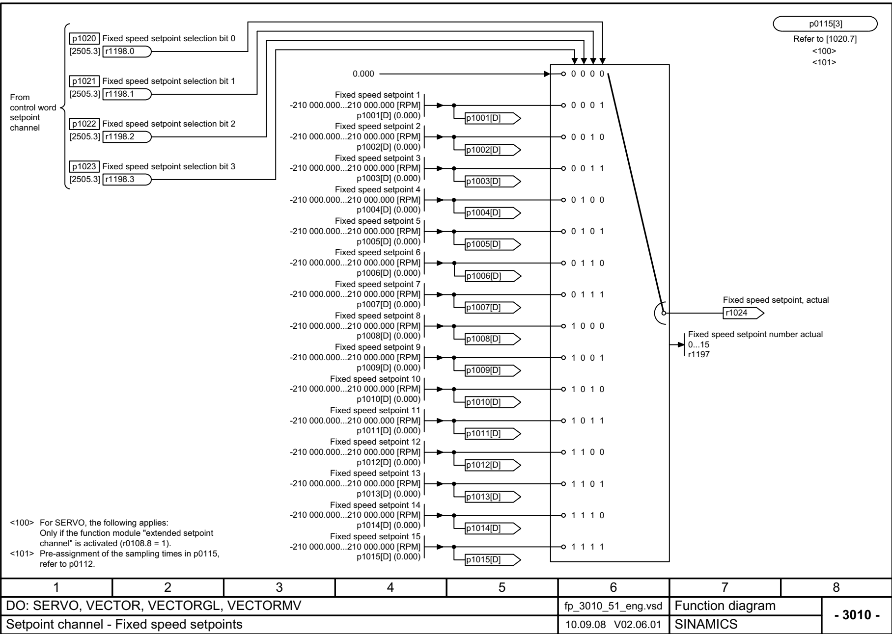
Рис. 2-74 3010 – Постоянные заданные значения частоты вращения
