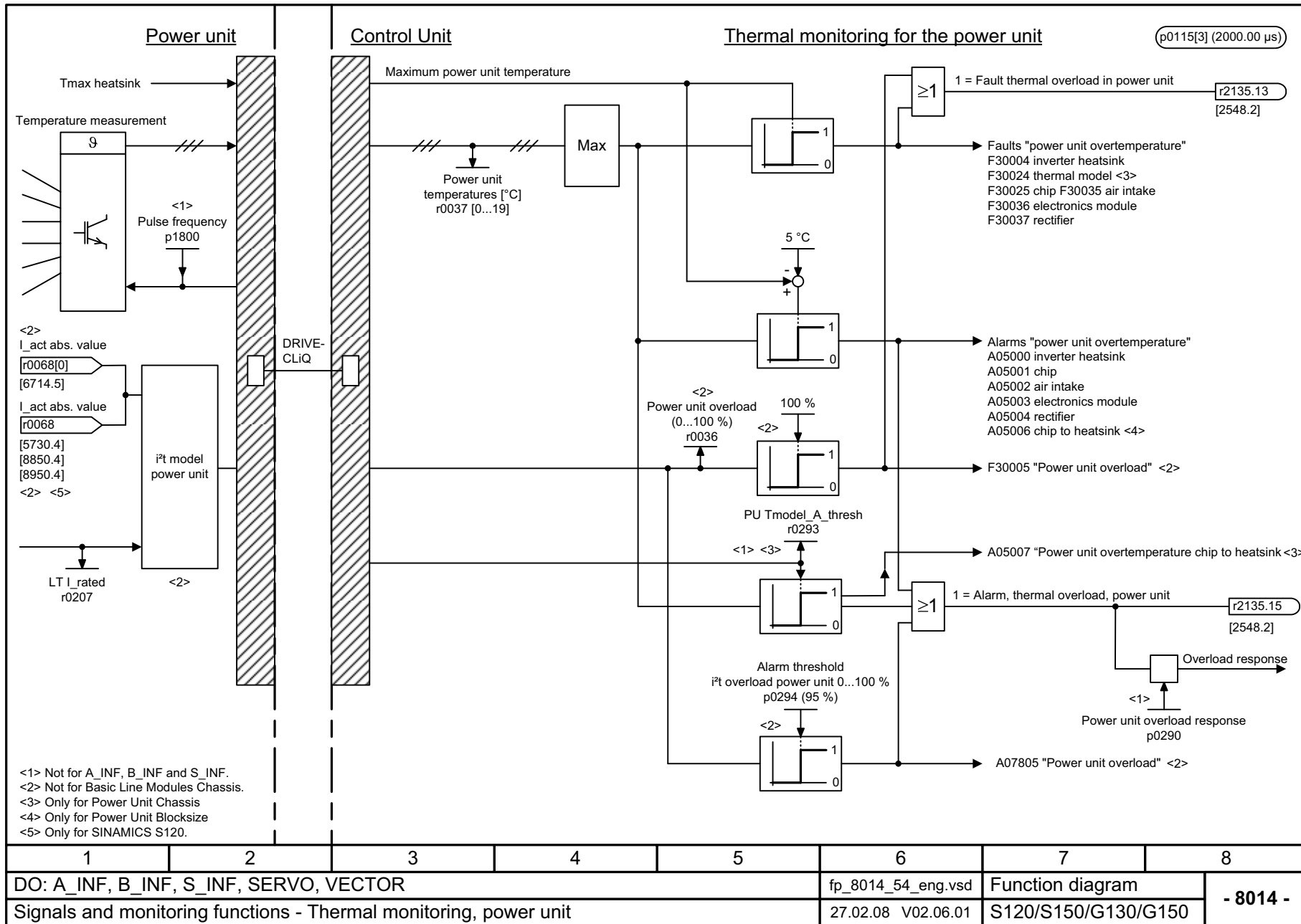
Рис. 2-117 8014 – Тепловой контроль силового блока
