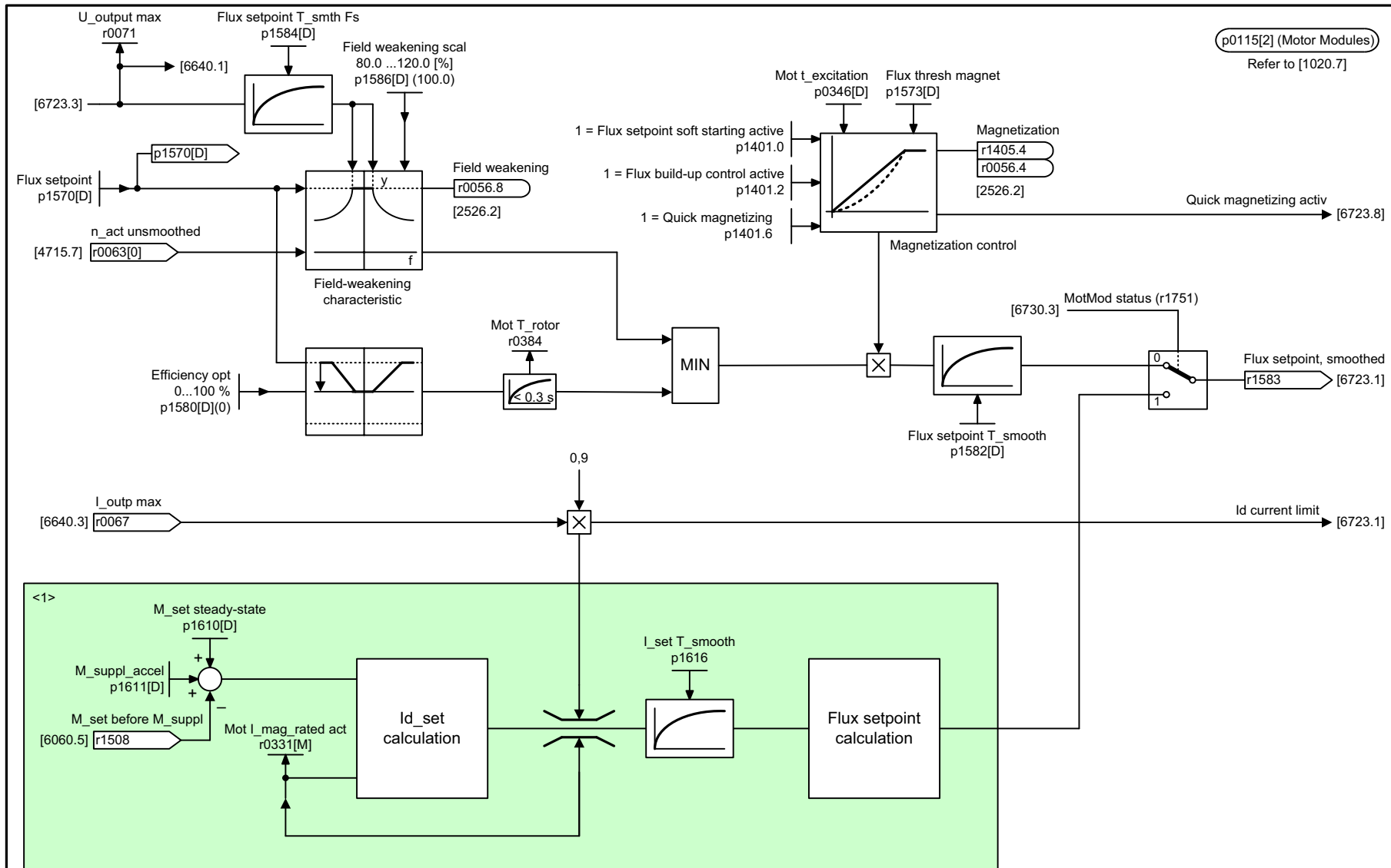
Рис. 2-100 6722 – Характеристика гашения поля, заданное значение Id (ASM, p0300 = 1)
