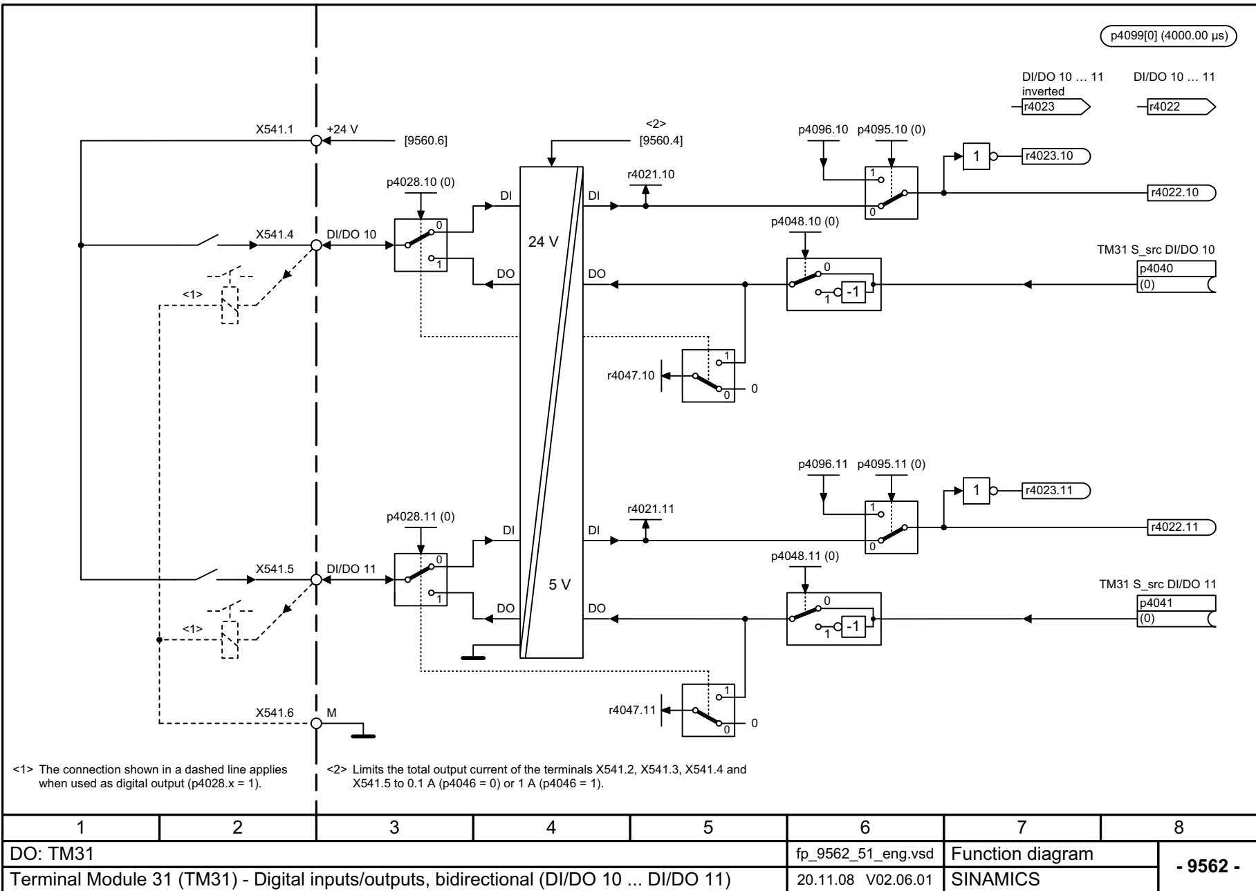
Рис. 2-144 9562 – Цифровые входы/выходы двусторонние (DI/DO 10 ... DI/DO 11)
