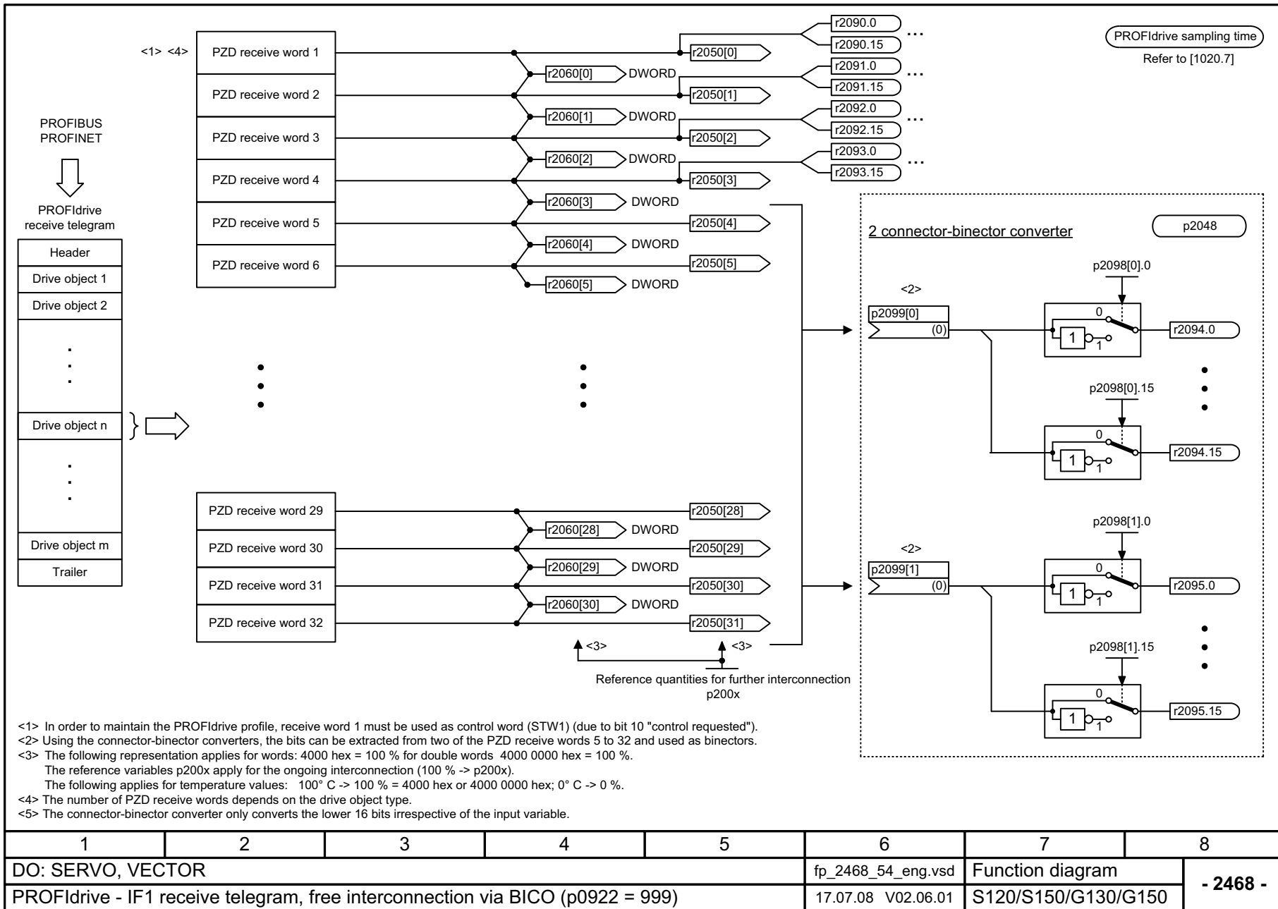
Рис. 2-40 2468 – IF1 Приемная телеграмма - свободное подключение через BICO (p0922 = 999) . . . .
