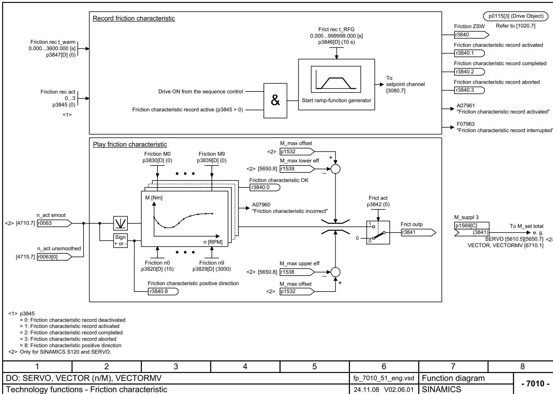
Рис. 2-106 7010 – Характеристика трения
