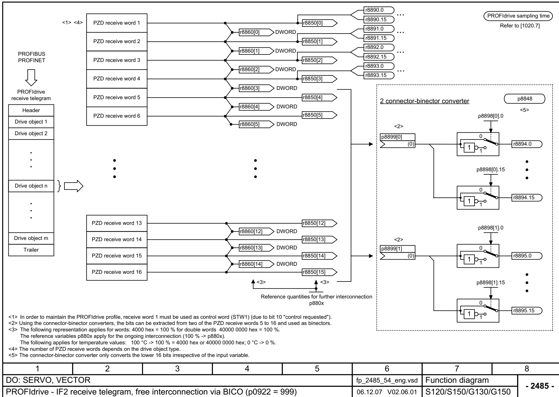
Рис. 2-45 2485 – IF2 Приемная телеграмма - свободное переключенение через BICO (p0922 = 999).
