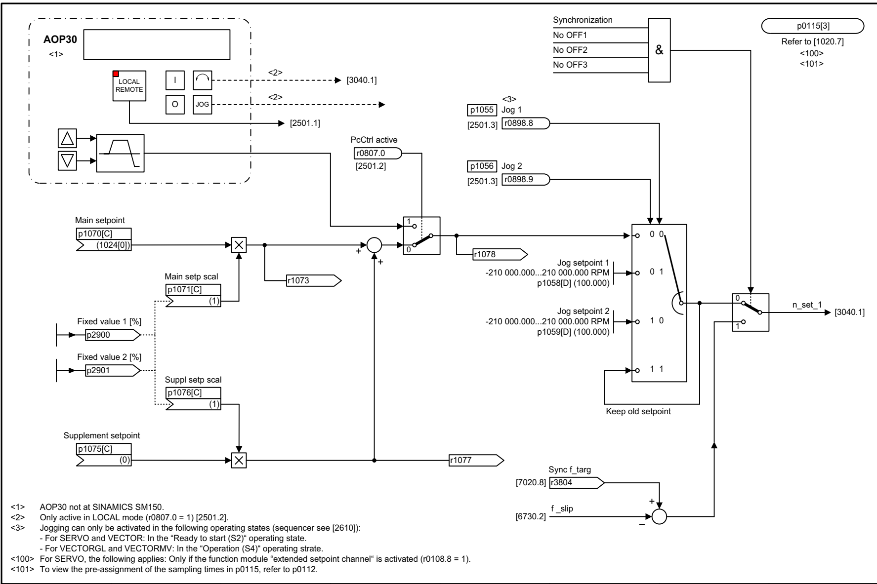
Рис. 2-76 3030 – Основное/дополнительное заданное значение, масштабирование заданного значения, толчковый режим .....
