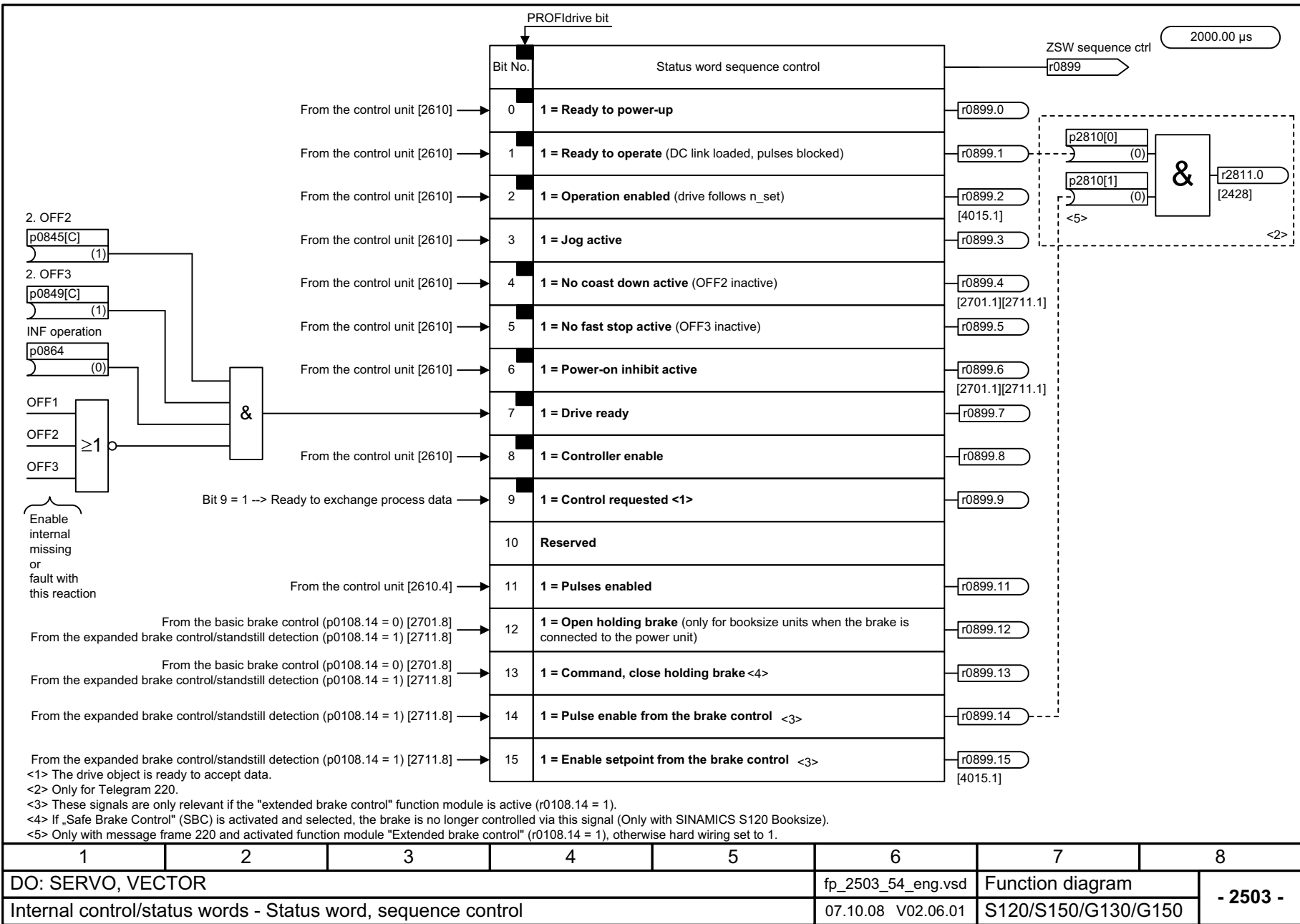
Рис. 2-53 2503 – Слово состояния - программное управление
