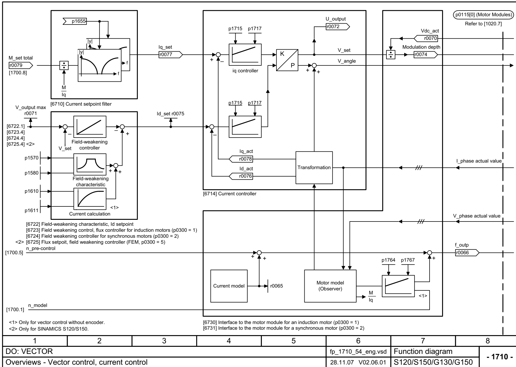
Рис. 2-12 1710 – Векторная регулировка, регулировка тока
