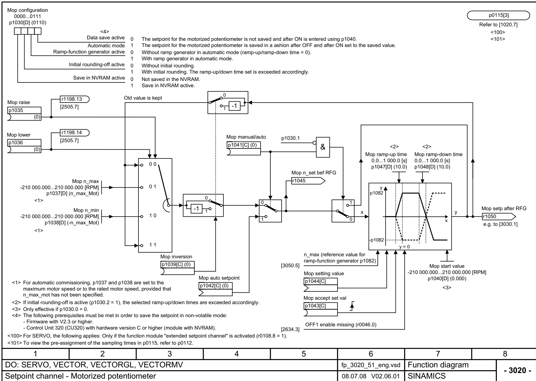
Рис. 2-75 3020 – Потенциометр двигателя
