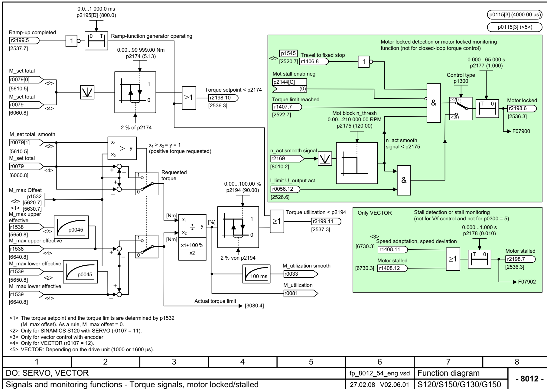
Рис. 2-115 8012 – Сообщения о моменте вращения, двигатель заблокирован/опрокинулся
