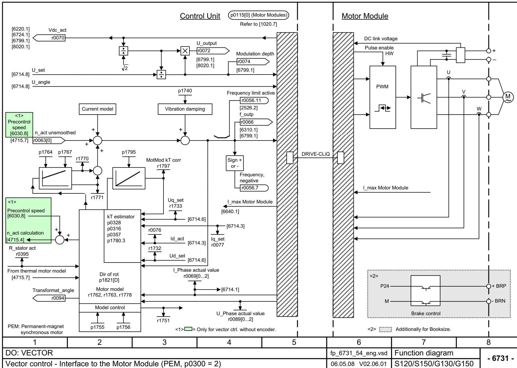
Рис. 2-104 6731 – Интерфейс для модулей двигателя (PEM, p0300 = 2)
