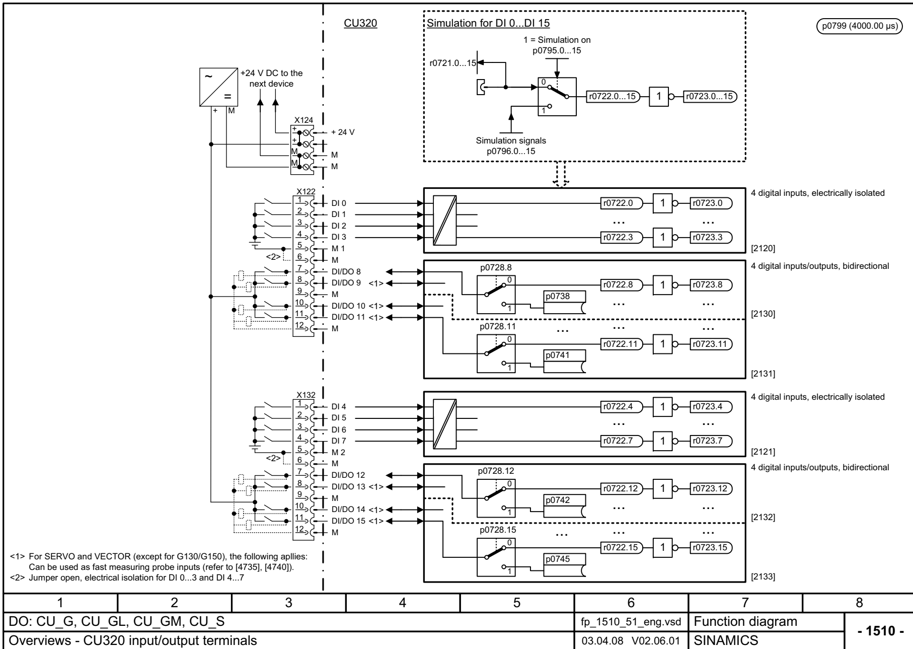
Рис. 2-5 1510 – CU320 входные/выходные клеммы
