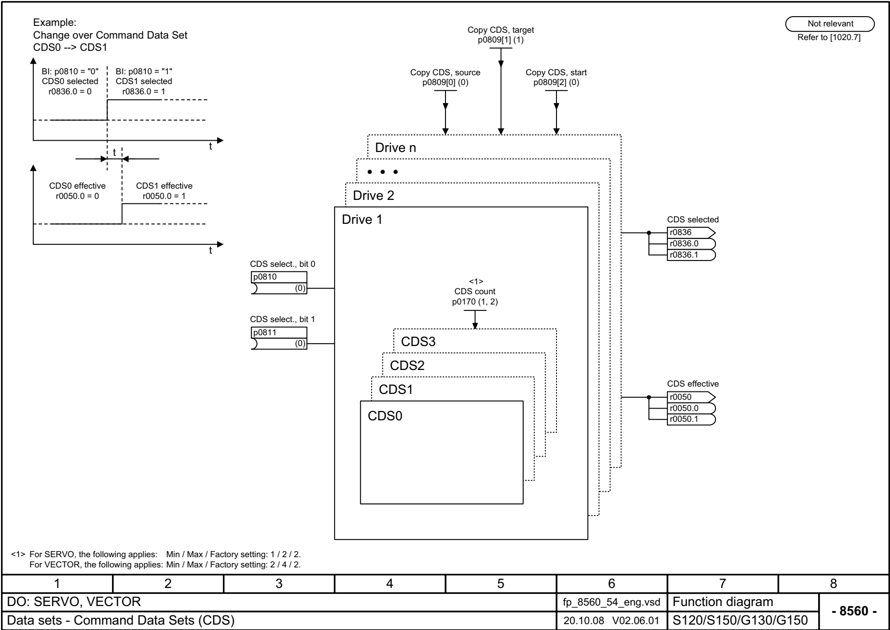
Рис. 2-125 8560 – Наборы команд (Command Data Set, CDS)
