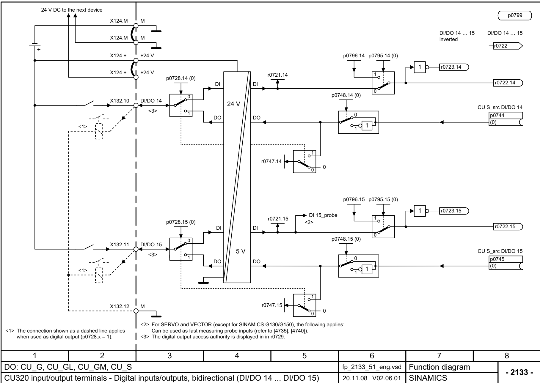
Рис. 2-21 2133 – Цифровые входы/выходы двусторонние (DI/DO 14 ... DI/DO 15)
