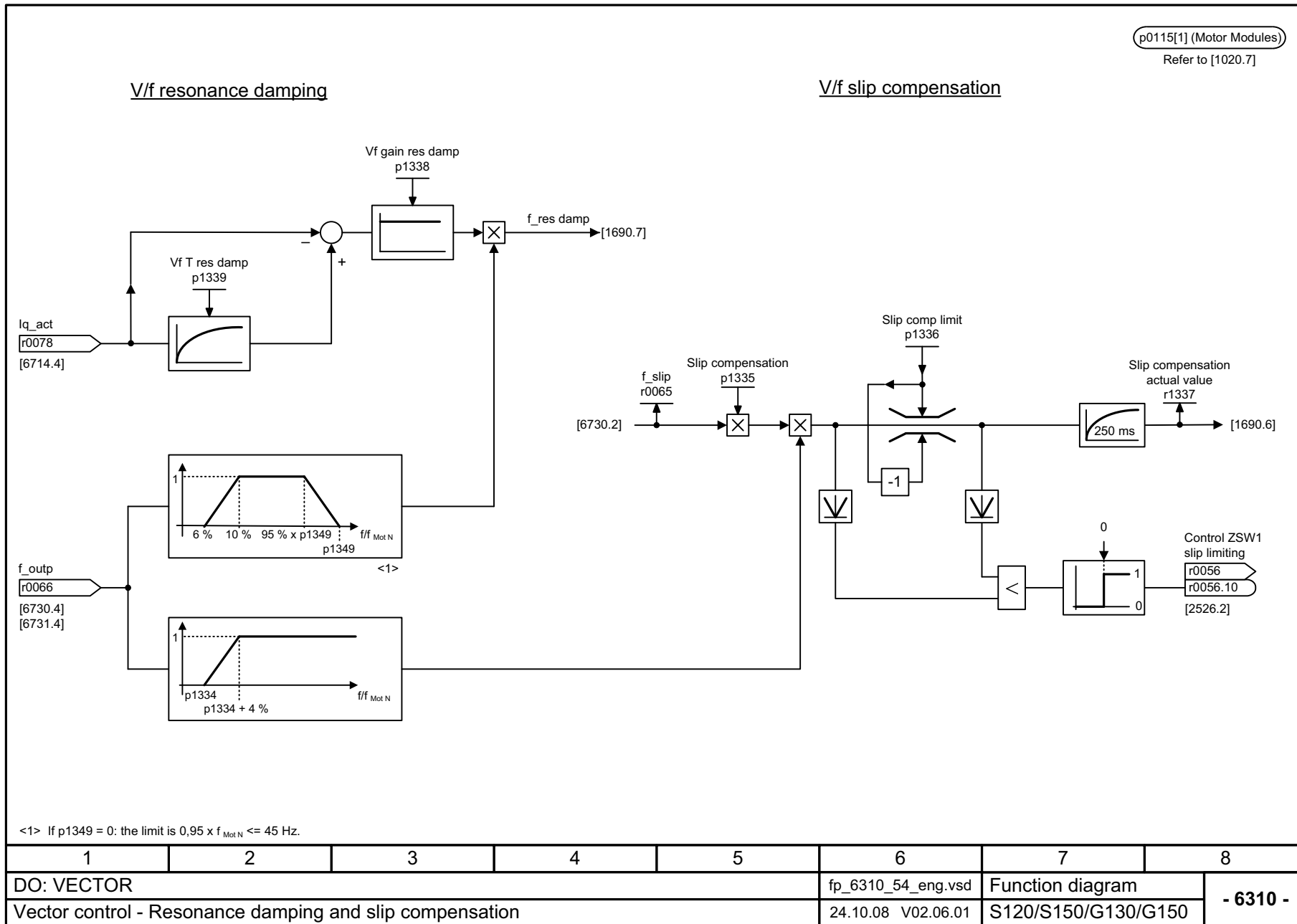
Рис. 2-91 6310 – Поглощение резонанса и компенсация скольжения
