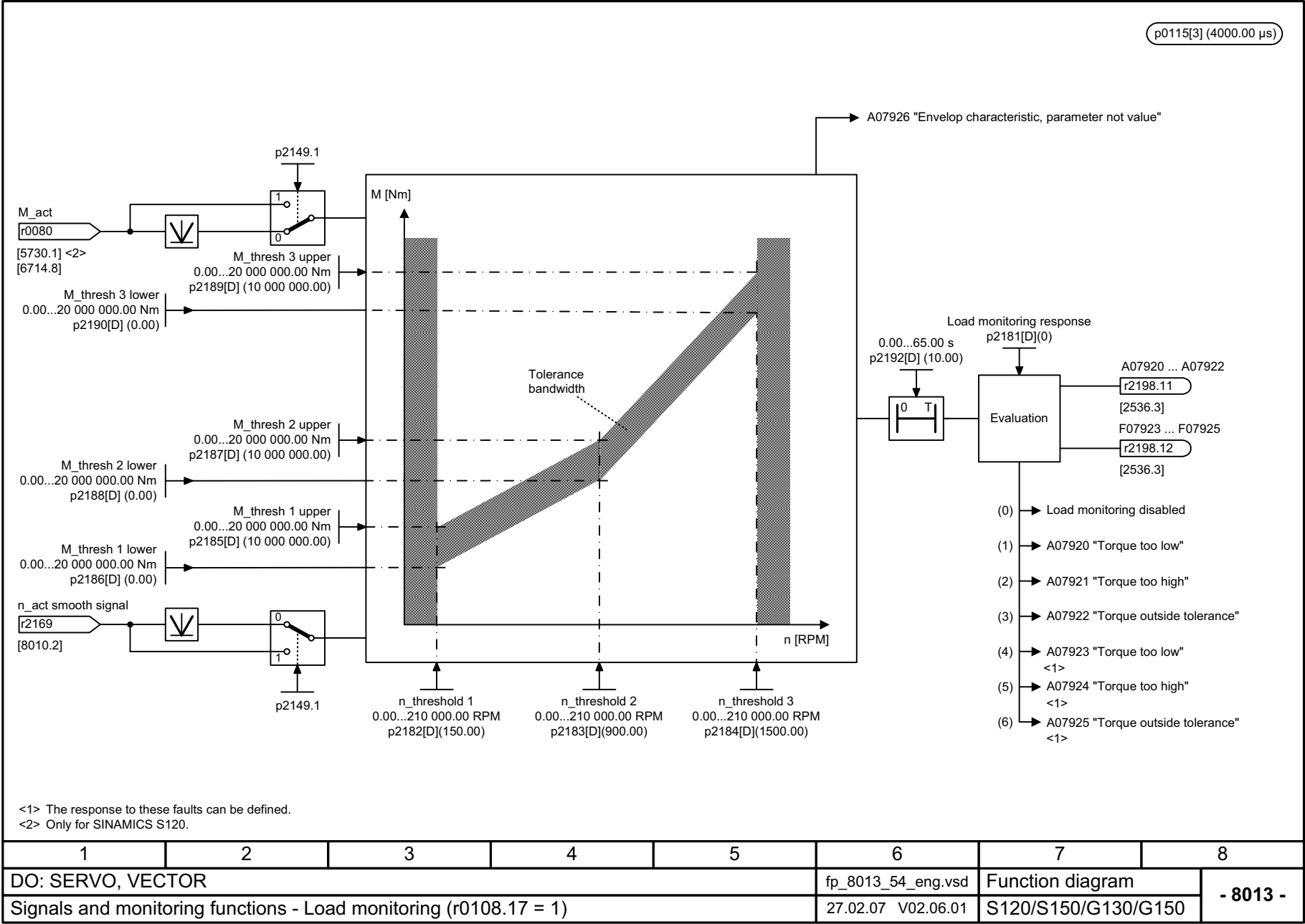
Рис. 2-116 8013 – Контроль нагрузки (r0108.17 = 1)
