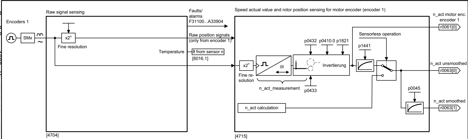
Рис. 2-9 1680 – Векторная регулировка, обработка сигналов датчиков (положение, скорость, температура)
