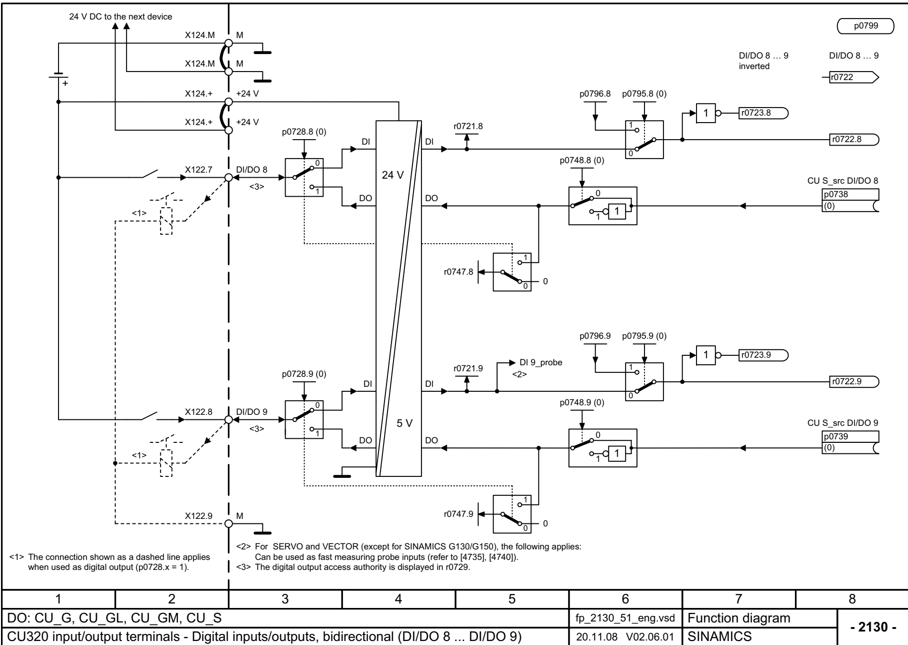
Рис. 2-18 2130 – Цифровые входы/выходы двусторонние (DI/DO 8 ... DI/DO 9)
