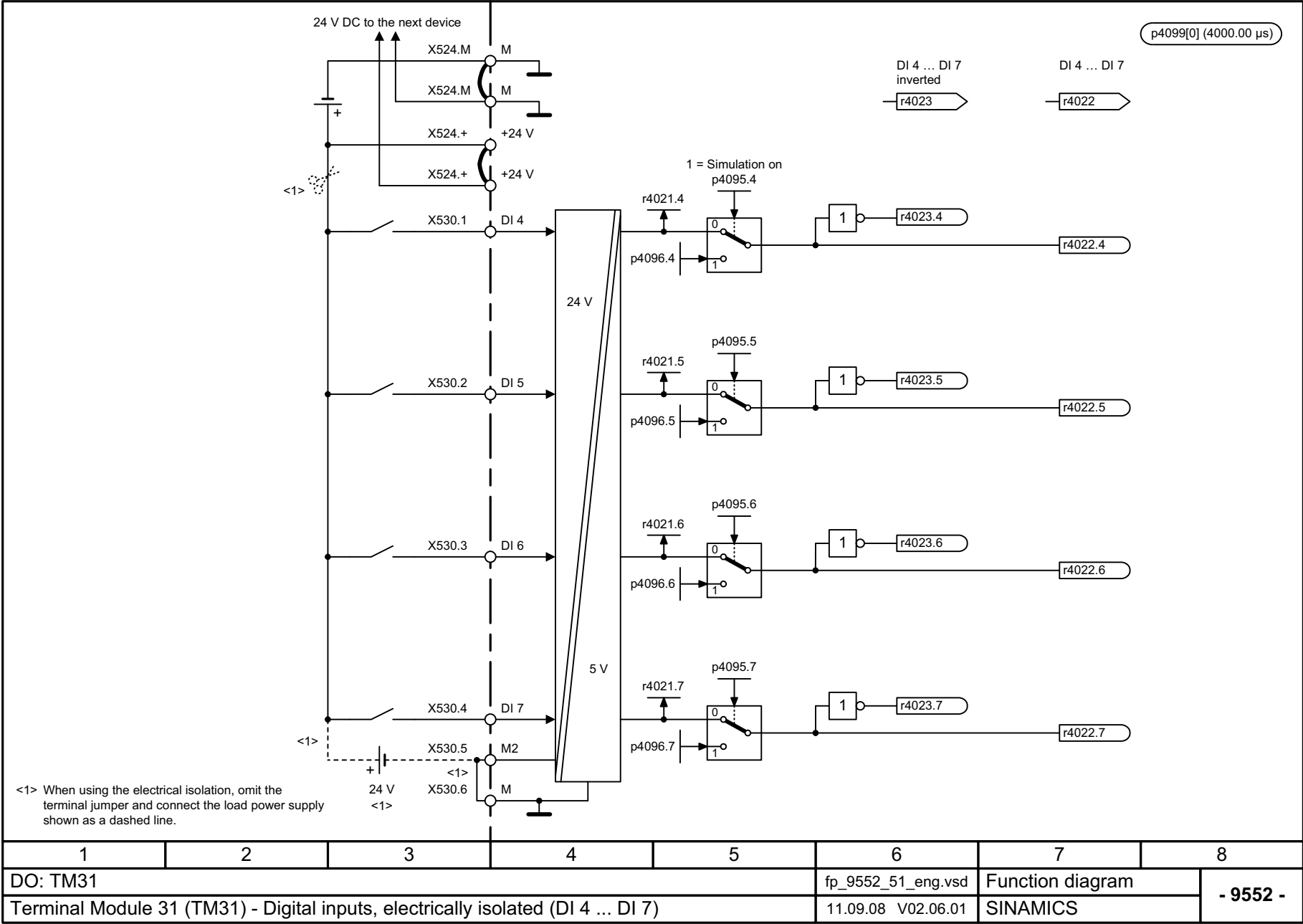
Рис. 2-141 9552 – Цифровые входы с разделением потенциалов (DI 4 ... DI 7)
