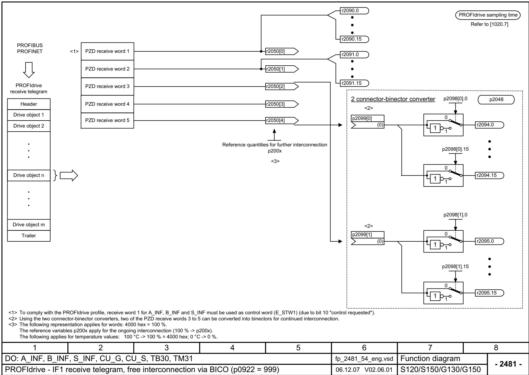
Рис. 2-43 2481 – IF1 Приемная телеграмма - свободное подключение через BICO ( p0922 = 999 ) ...
