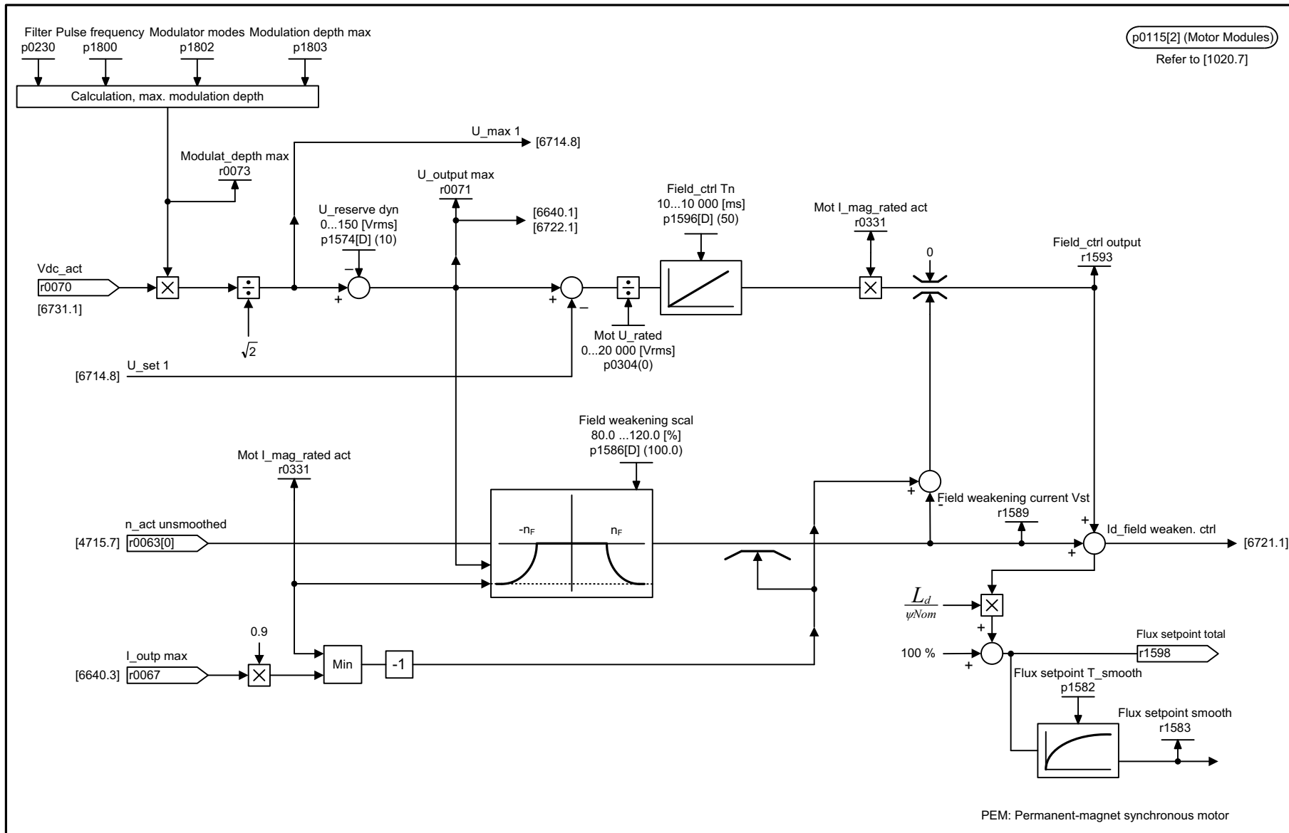
Рис. 2-102 6724 – Регулятор ослабления поля (РЕМ, p0300 = 2)
