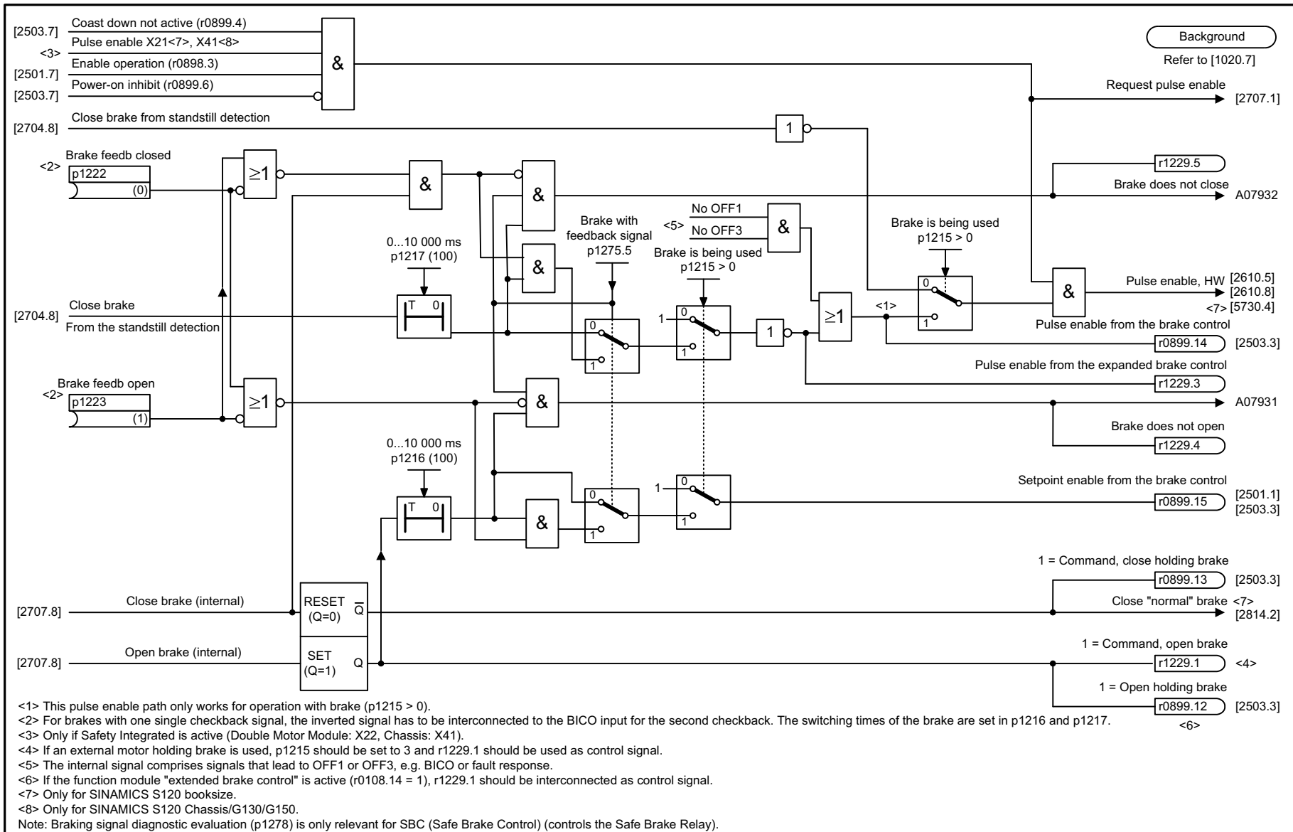
Рис. 2-69 2711 – Расширенная регулировка торможения, сигнальные выходы (r0108.14 = 1)
