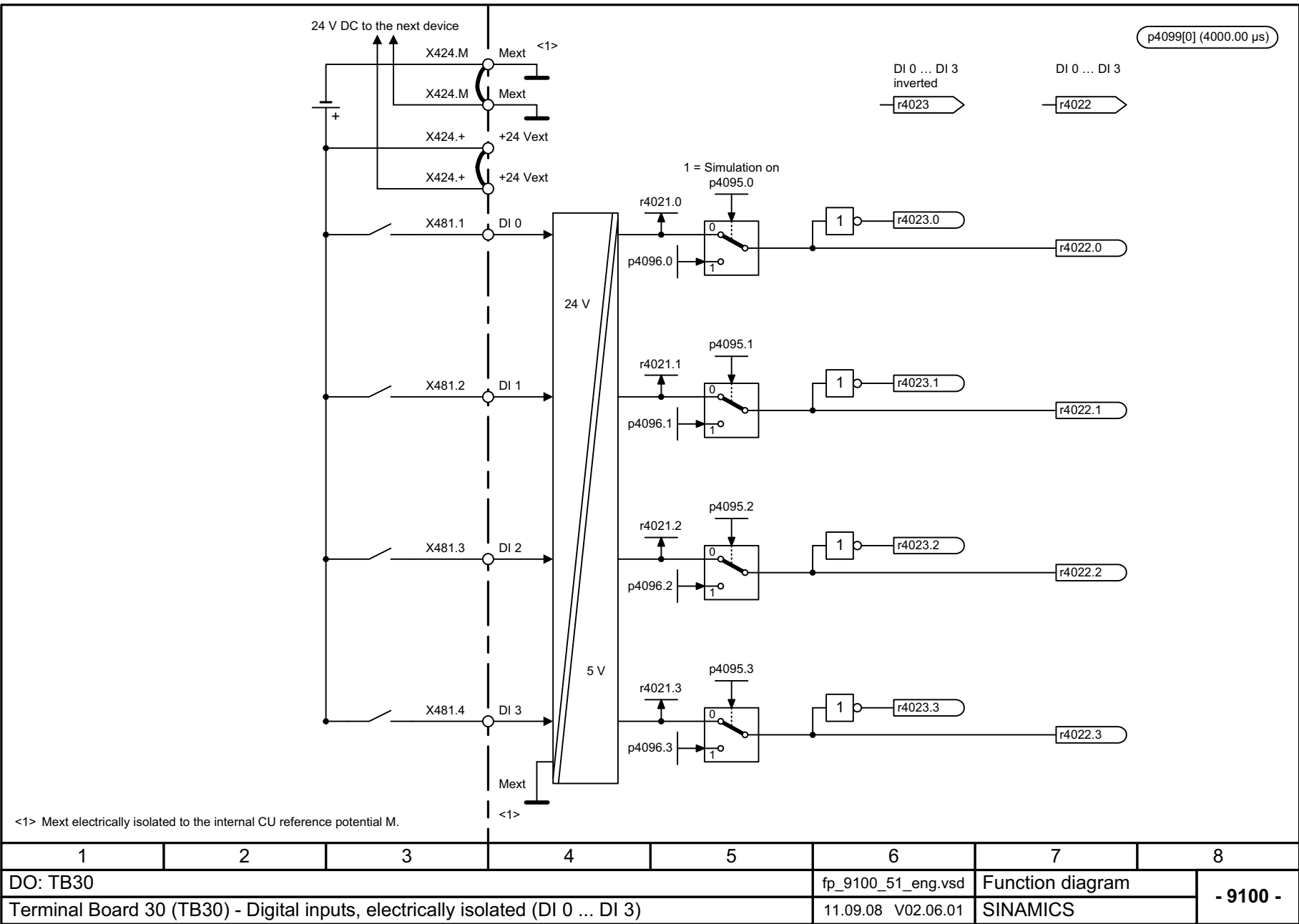
Рис. 2-130 9100 – Цифровые входы с разделением потенциалов (DI 0 ... DI 3)
