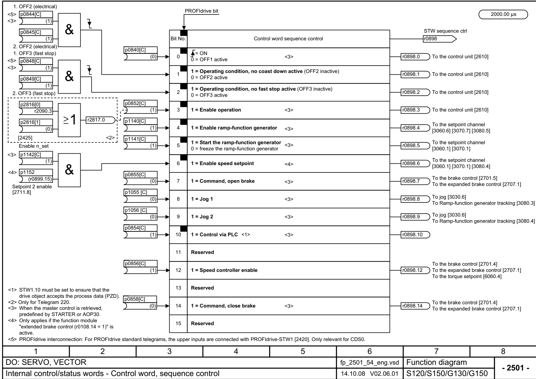
Рис. 2-52 2501 – Управляющее слово - программное управление
