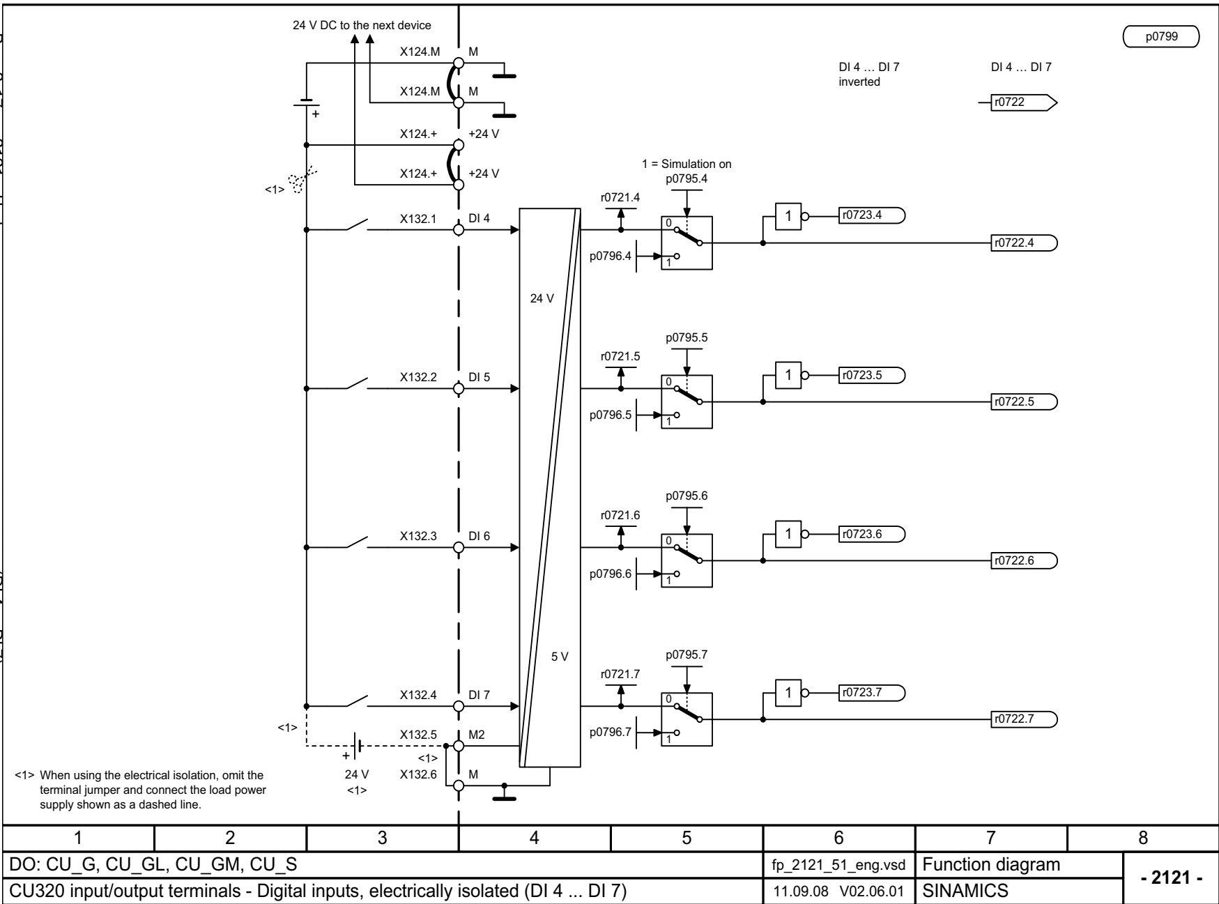
Рис. 2-17 2121 – Цифровые входы с разделением потенциалов (DI 4 ... DI 7)
