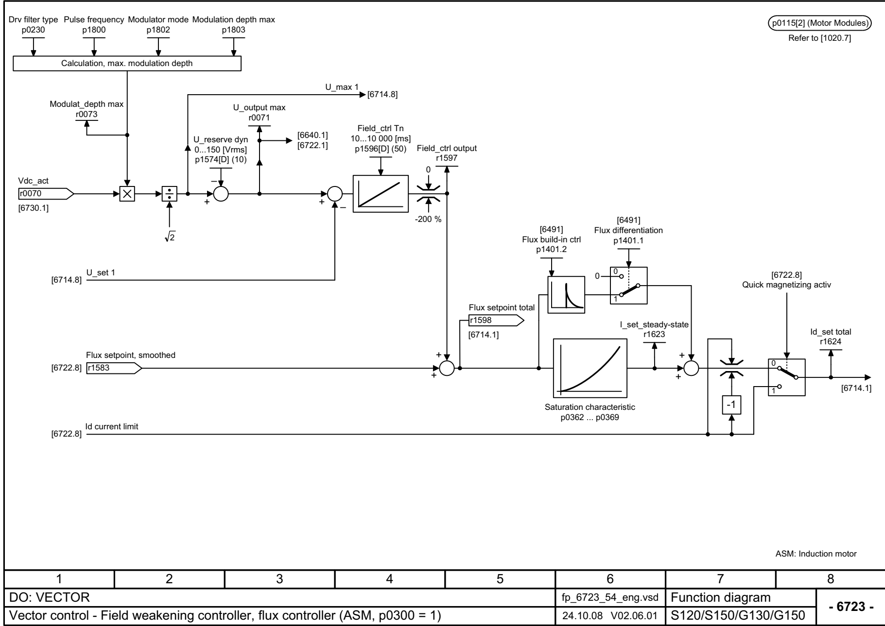
Рис. 2-101 6723 – Регулятор ослабления поля, регулятор тока (ASM, p0300 = 1)
