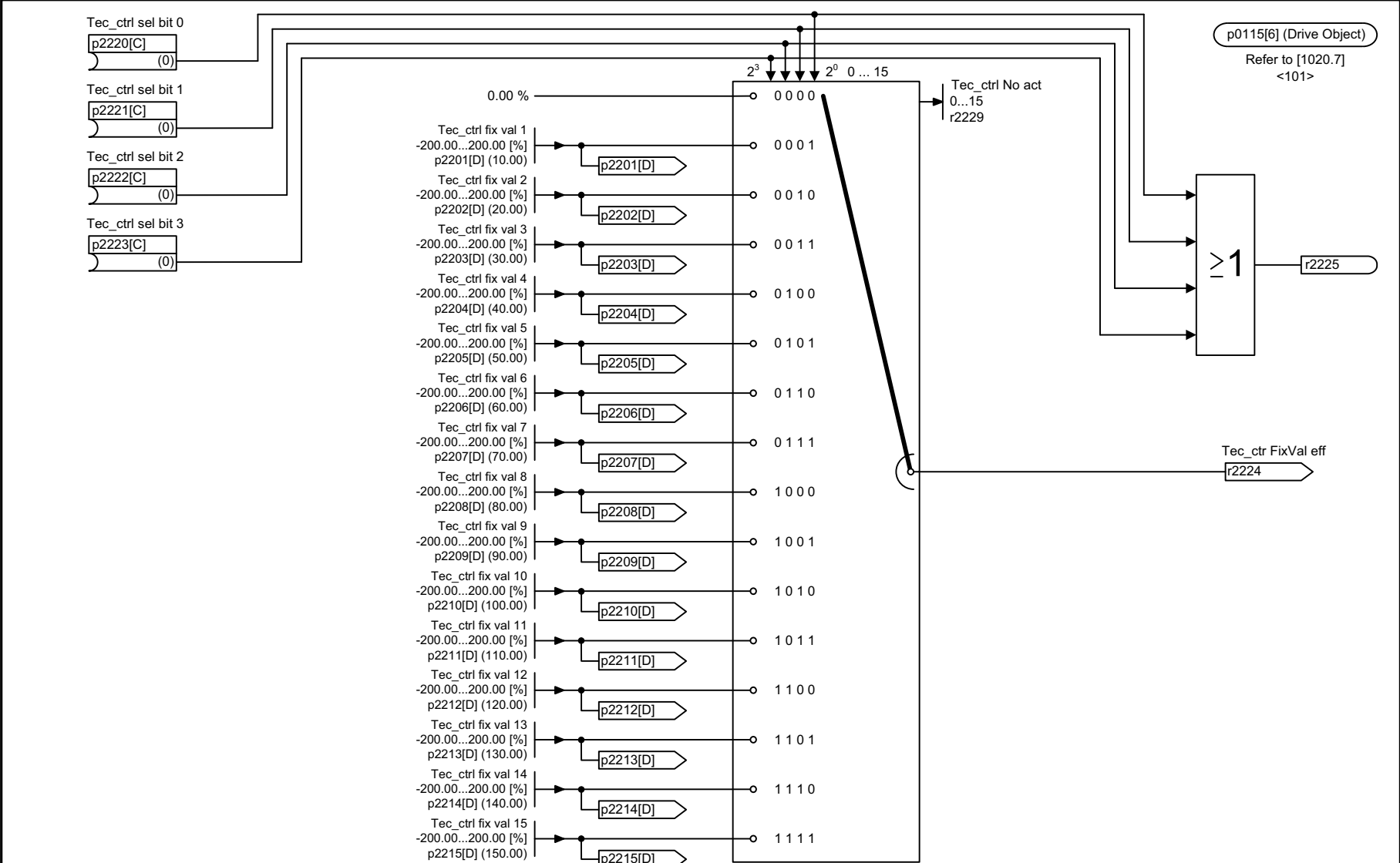
Рис. 2-111 7950 – Фиксированные значения (r0108.16 = 1)
