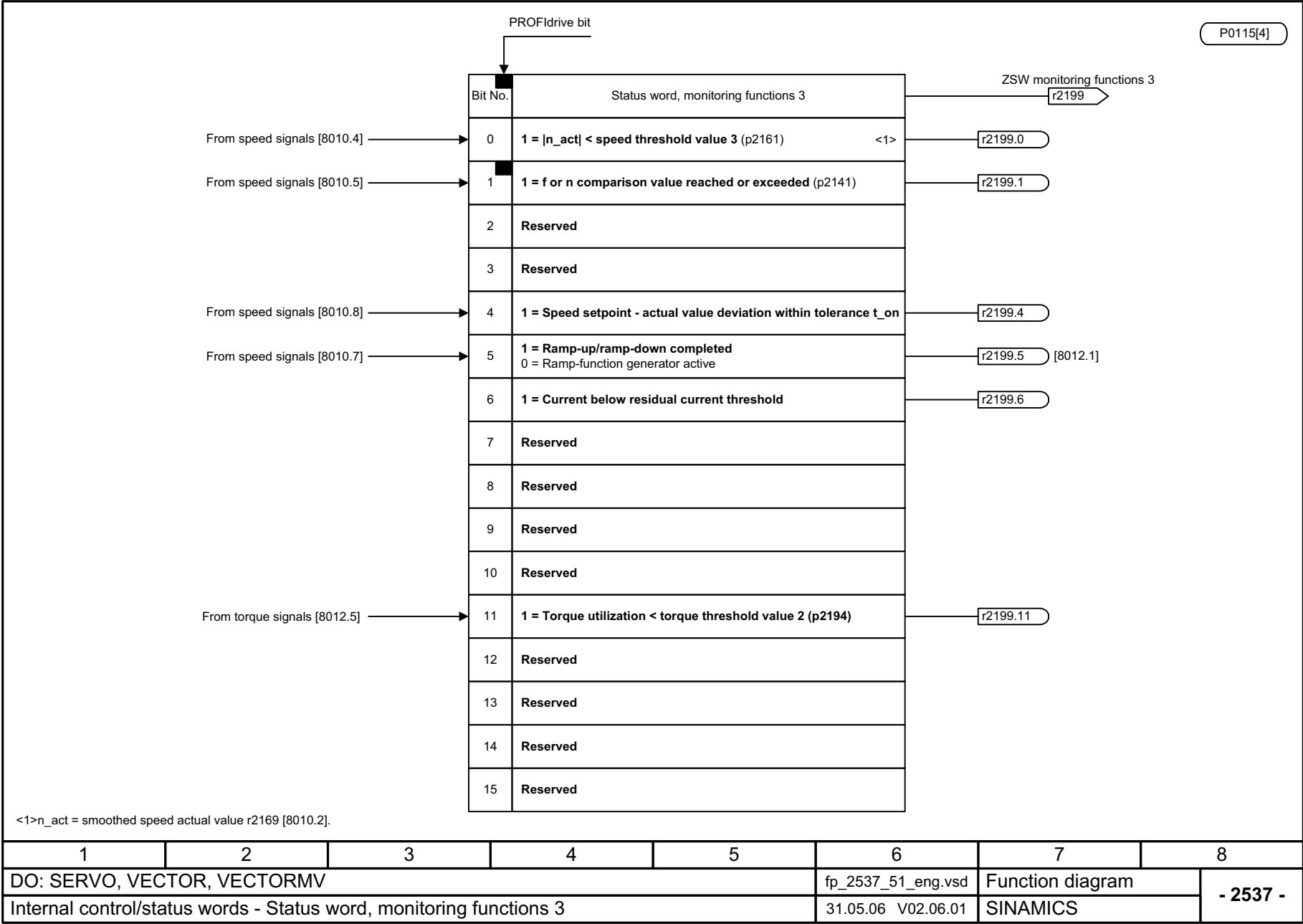
Рис. 2-61 2537 – Слово состояния - Контроль 3
