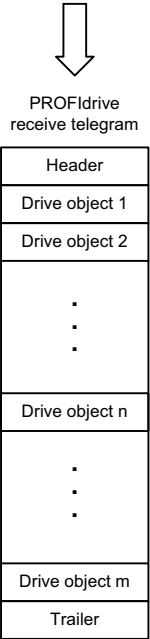
Рис. 2-31 2440 – Подключение приемных сигналов PZD по производителю
