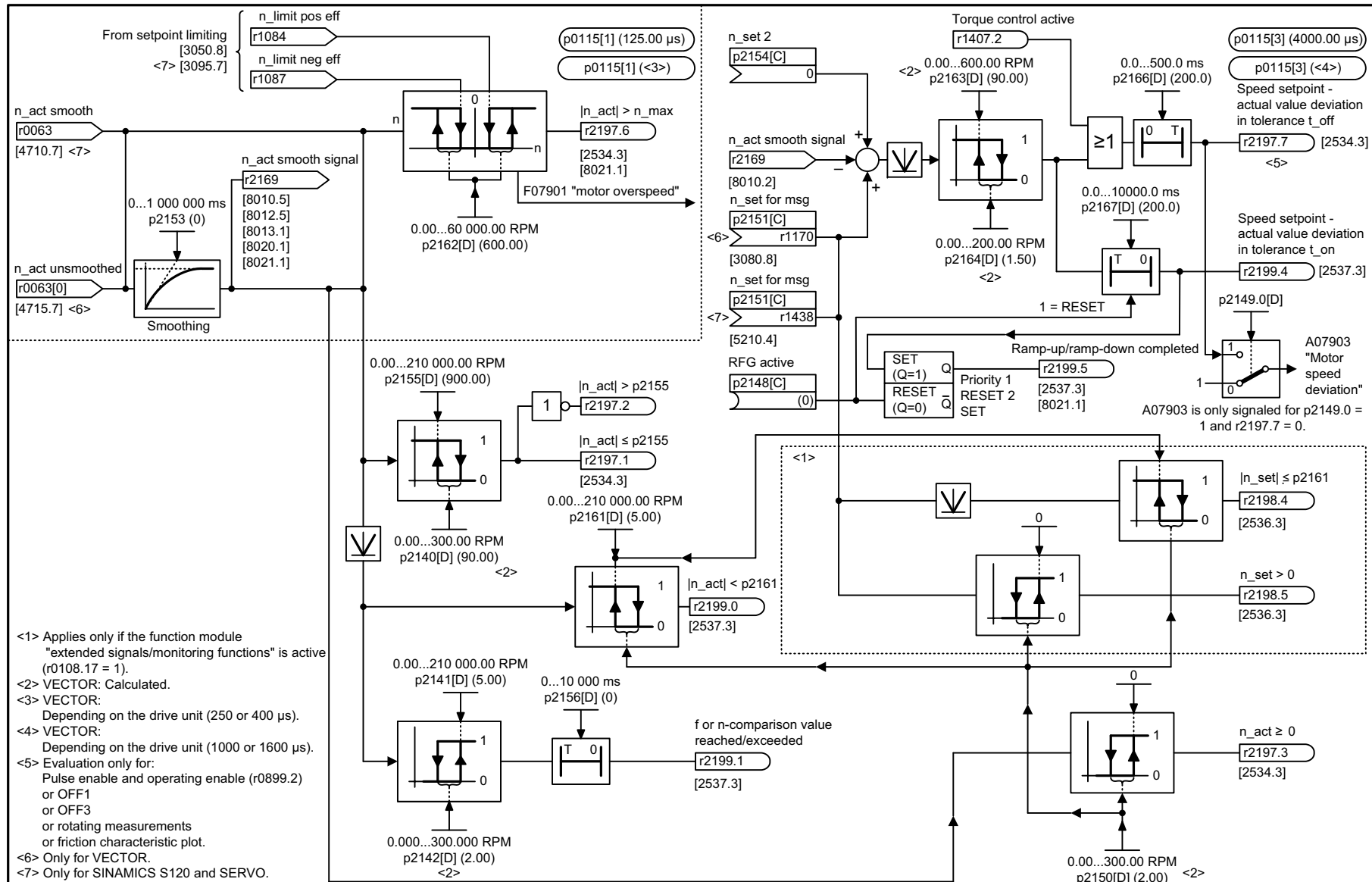
Рис. 2-114 8010 – Сообщения о частоте вращения
