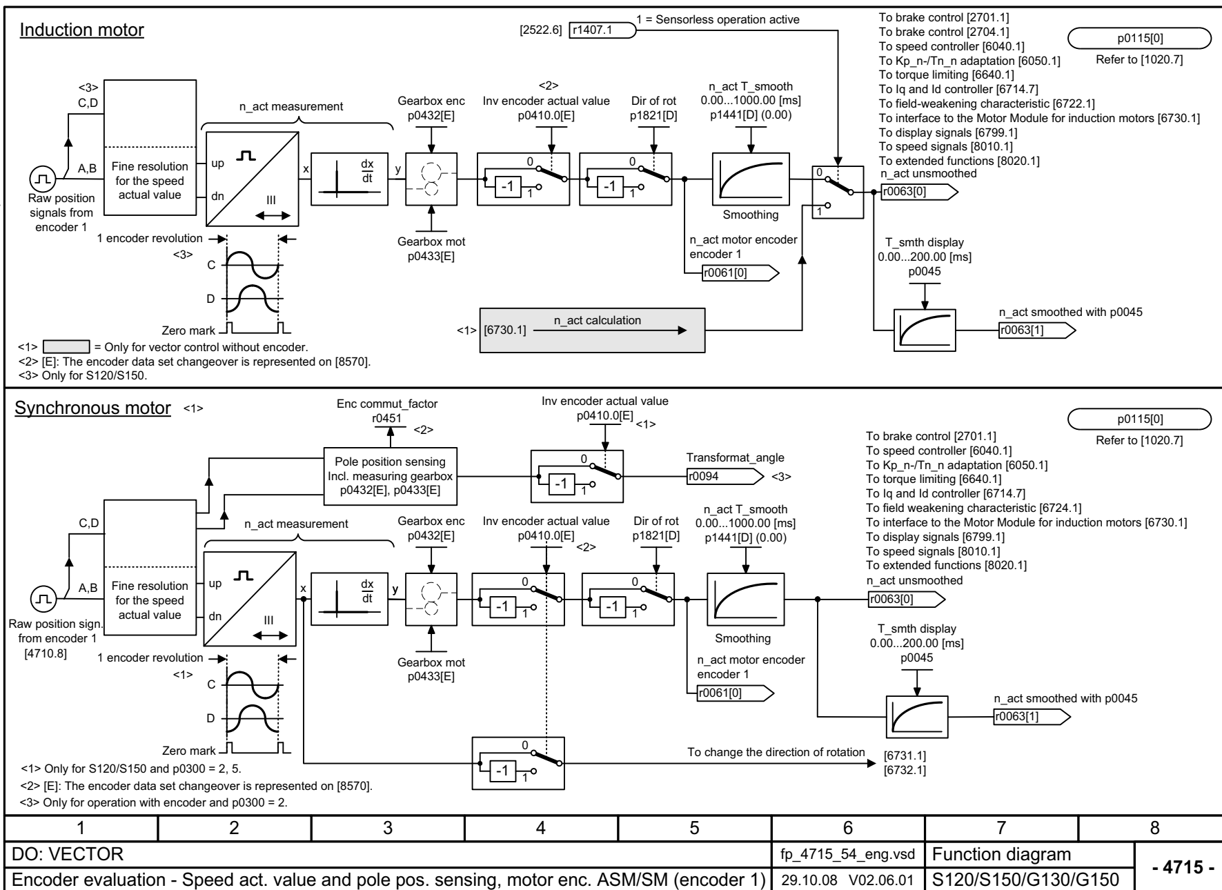
Рис. 2-83 4715 – Сбор данных о фактической частоте вращения и расположении полюсов датчика двигателя ASM/SM (датчик1)
