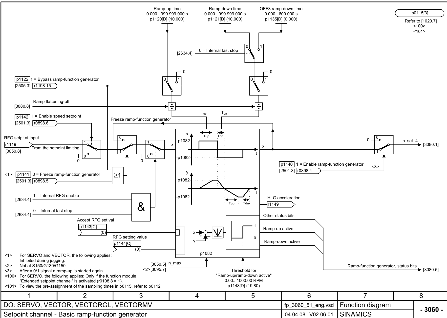
Рис. 2-79 3060 – Простой датчик разгона
