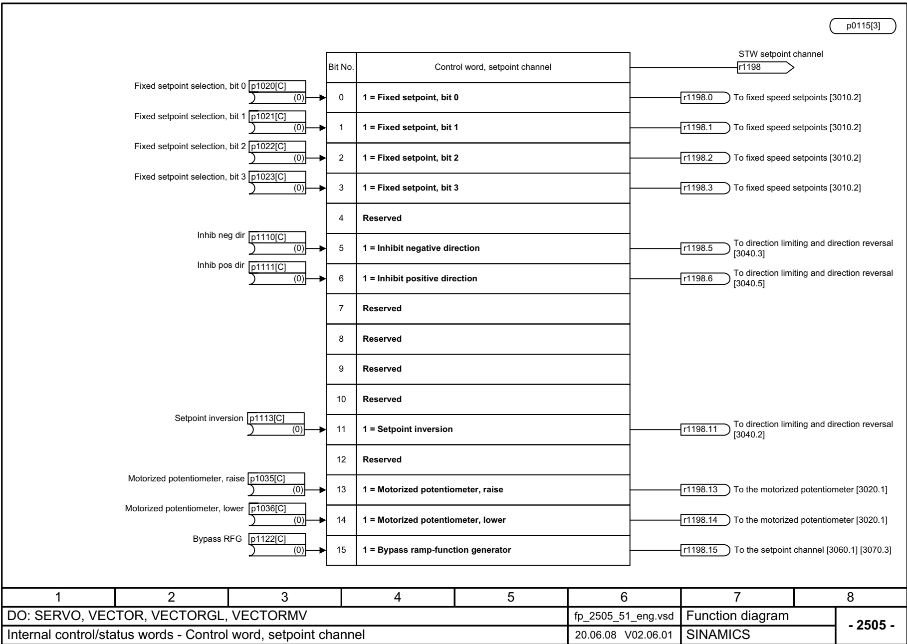
Рис. 2-54 2505 – Управляющее слово - Канал уставок
