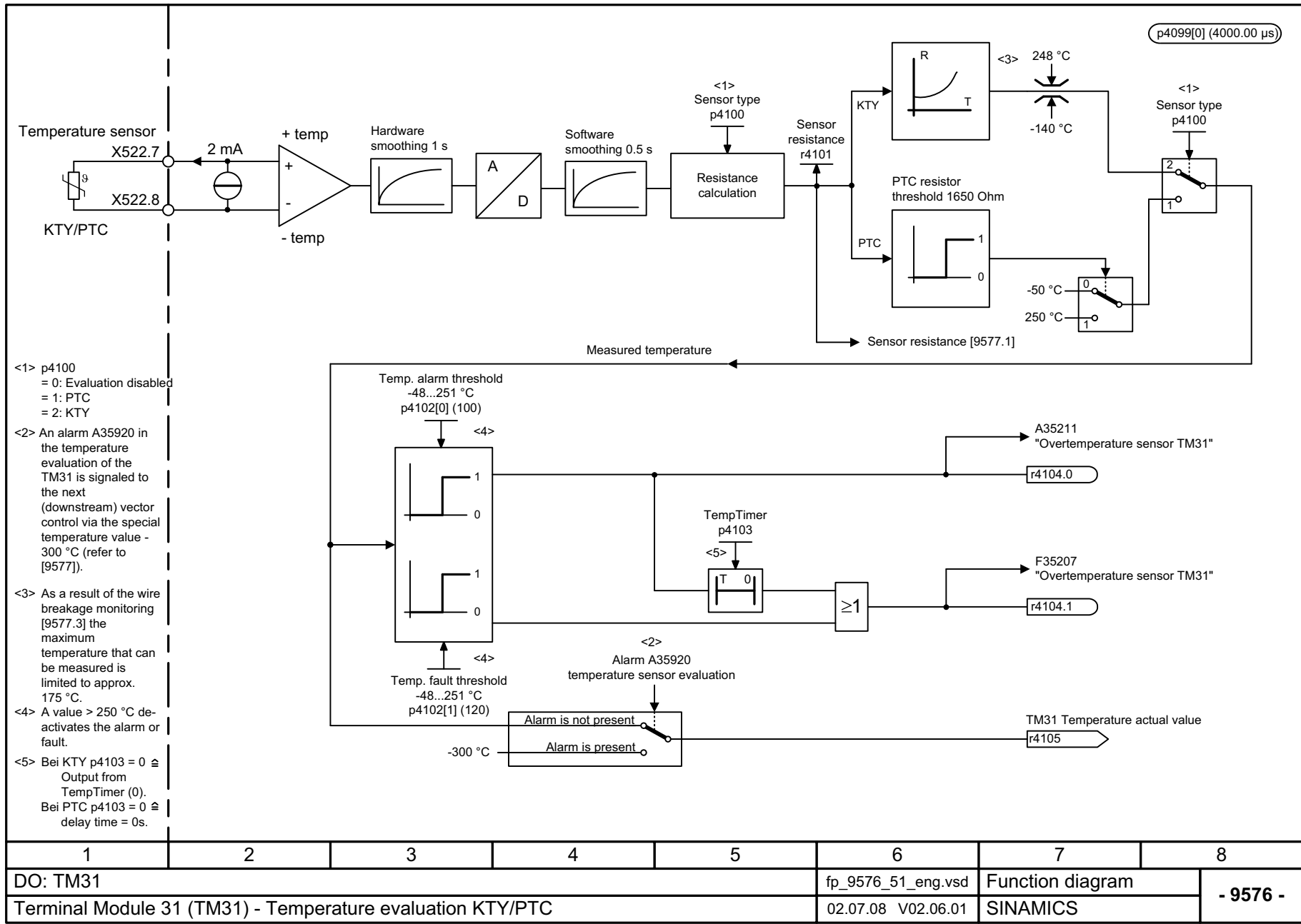
Рис. 2-148 9576 – Обработка температуры KTY/PTC
