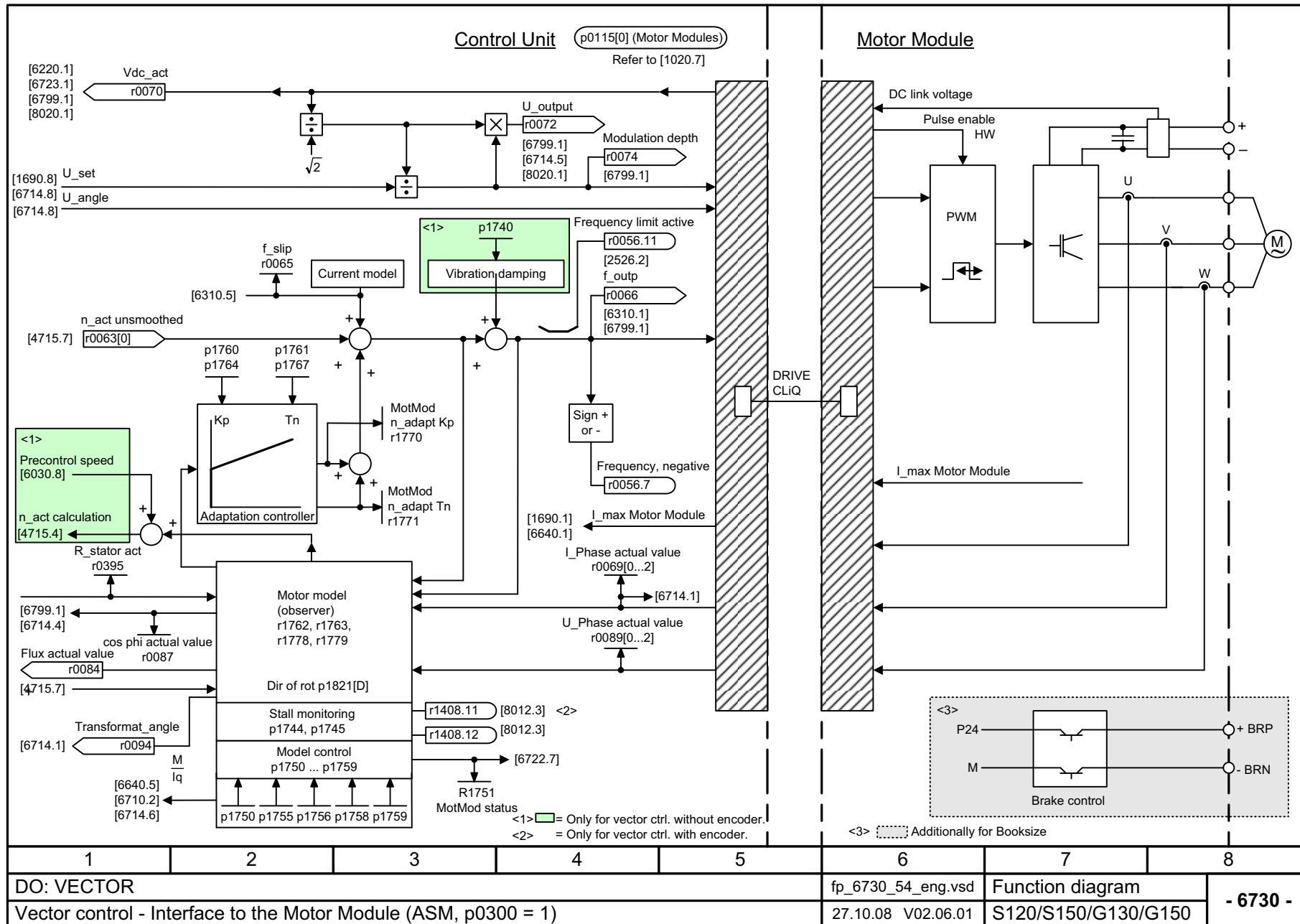
Рис. 2-103 6730 – Интерфейс для модулей двигателя (ASM, p0300 = 1)
