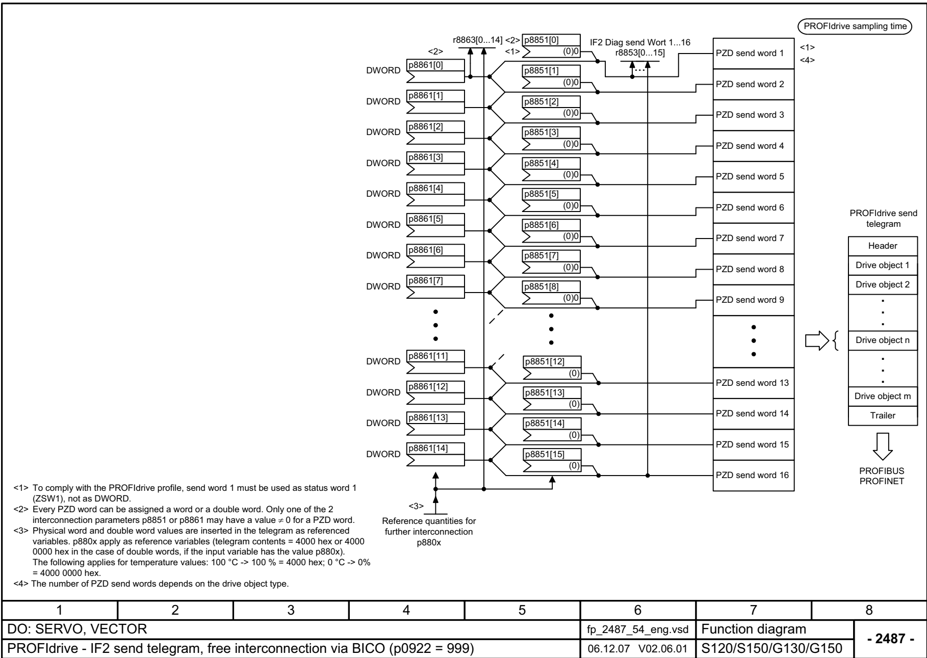
Рис. 2-46 2487 – IF2 Телеграмма передачи - свободное подключение через BICO (p0922 = 999) ...
