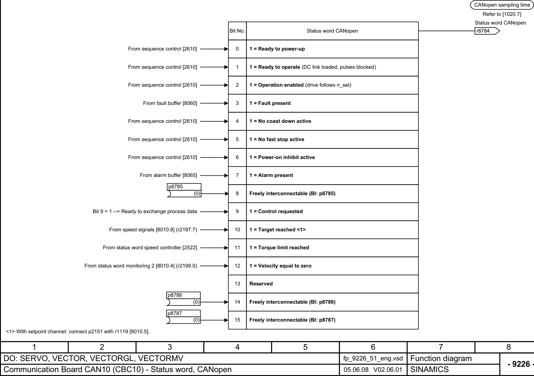
Рис. 2-139 9226 – Словно состояния CANopen
