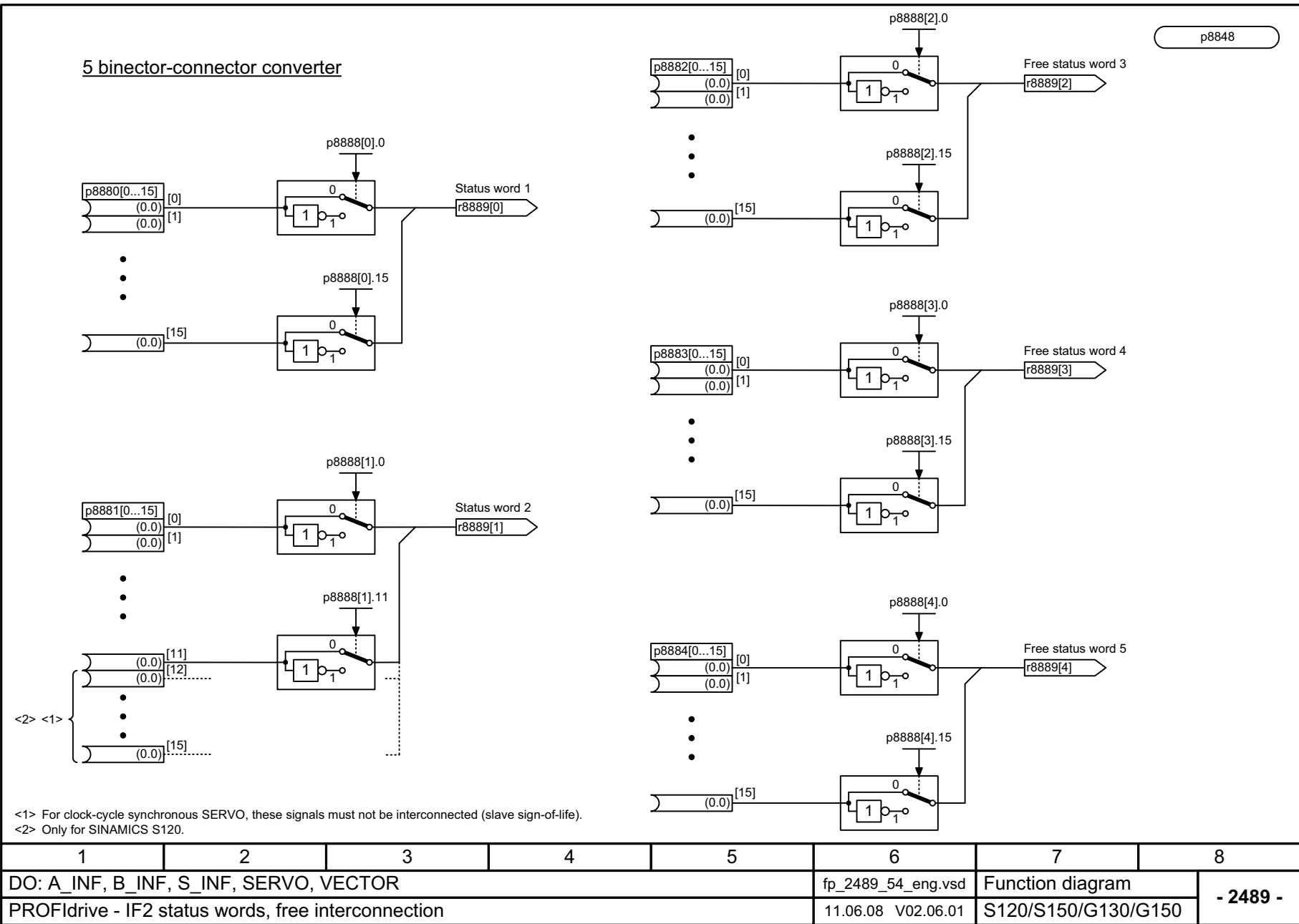
Рис. 2-47 2489 – IF2 Слова состояния - свободное переключение
