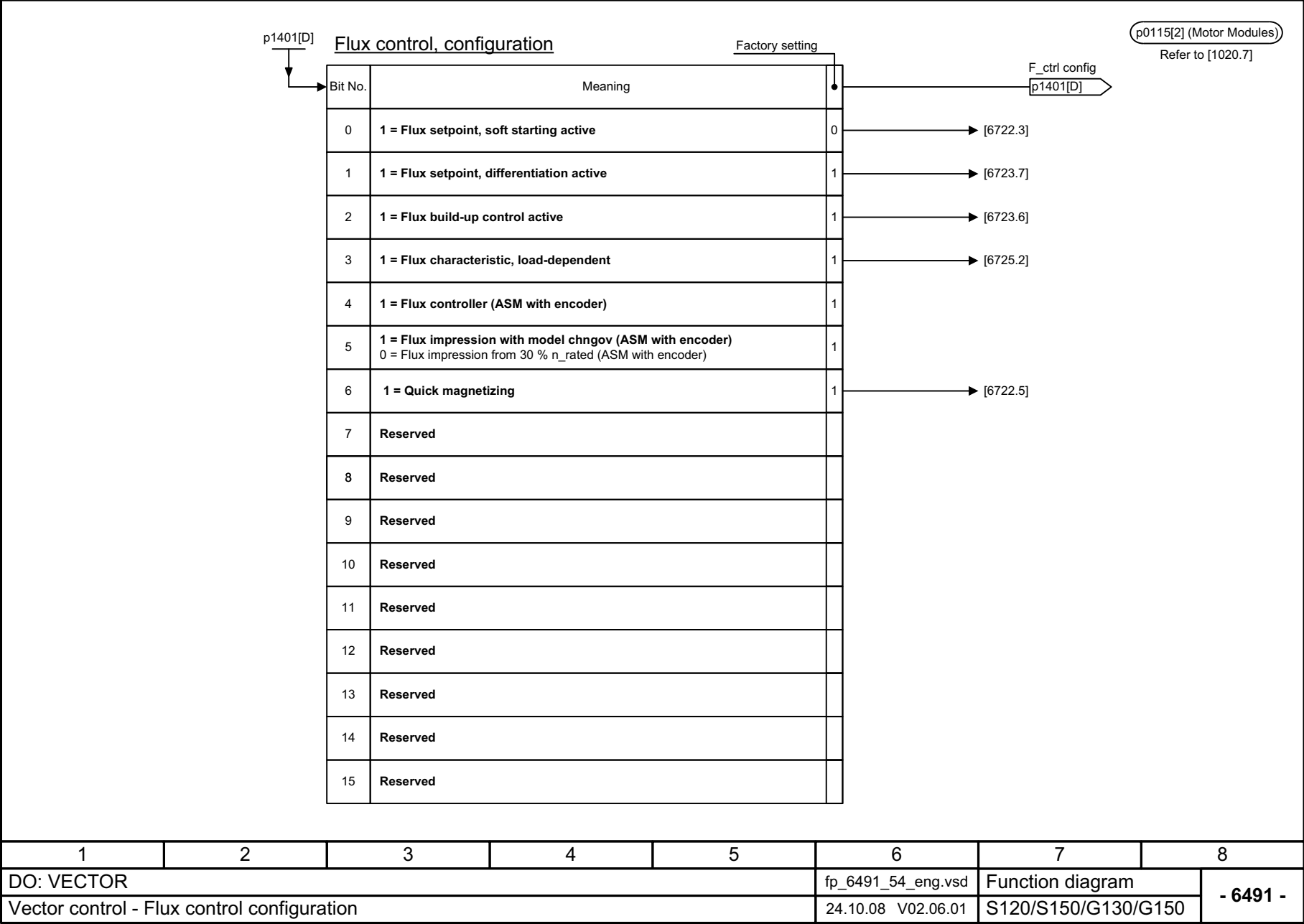
Рис. 2-94 6491 – Регулирование тока - Конфигурация
