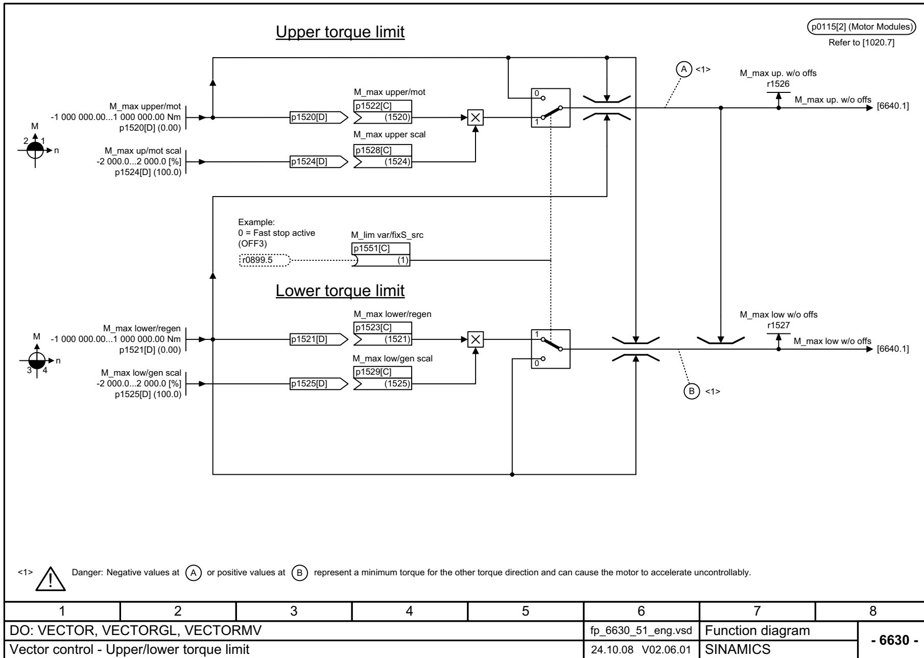
Рис. 2-95 6630 – Верхний/нижний предел момента
