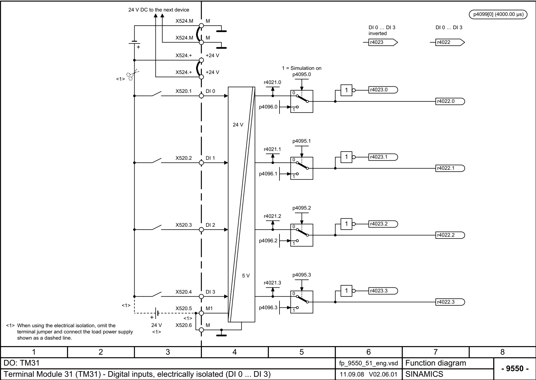
Рис. 2-140 9550 – Цифровые входы с разделением потенциалов (DI 0 ... DI 3)
