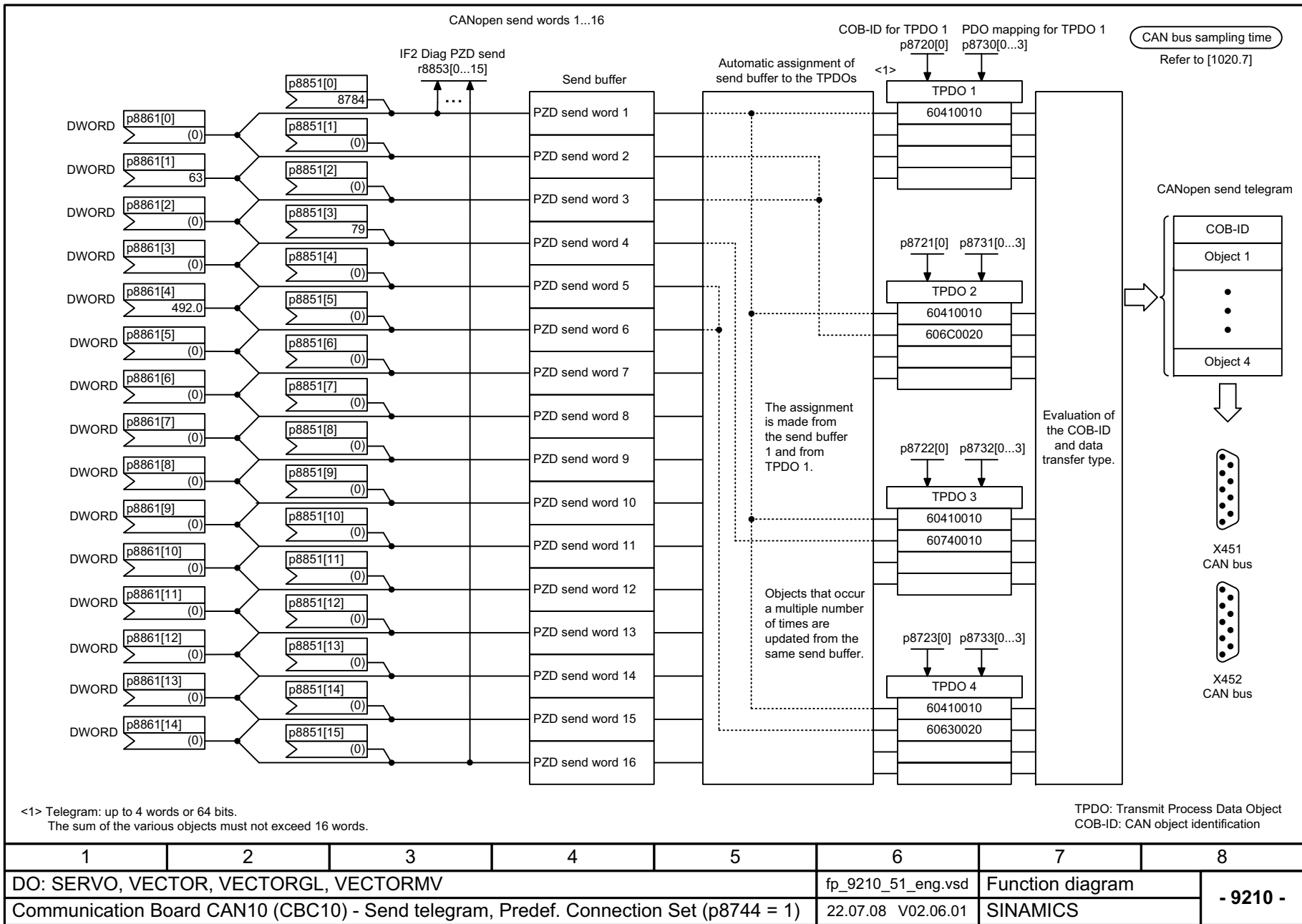
Рис. 2-137 9210 – Телеграмма отправки - Predefined Connection Set (p8744 = 1)
