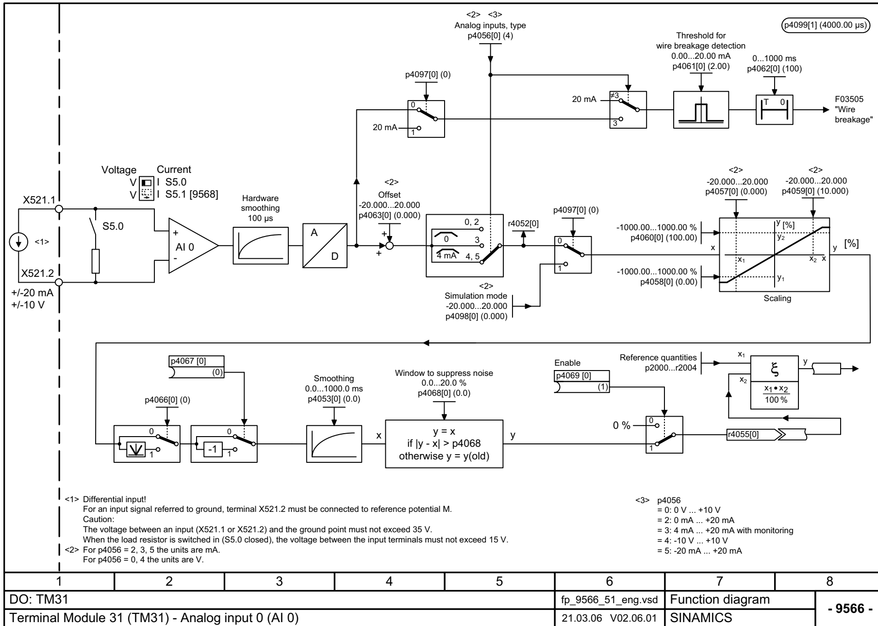
Рис. 2-145 9566 – Аналоговый вход 0 (AI 0)
