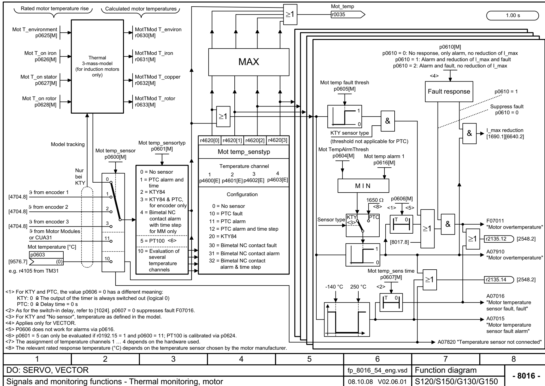
Рис. 2-118 8016 – Тепловой контроль двигателя
