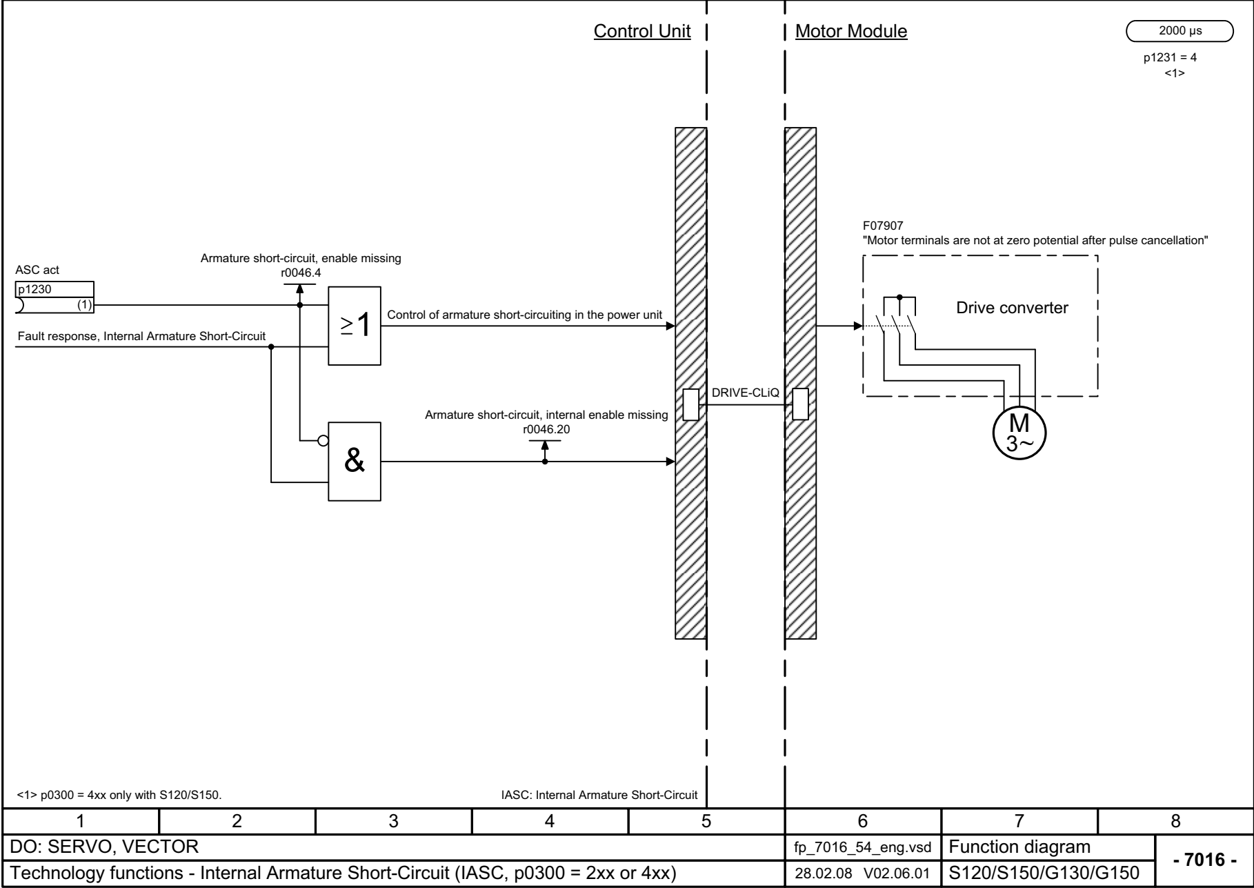
Рис. 2-108 7016 – Внутреннее короткое замыкание якоря (IASC, p0300 = 2xx)
