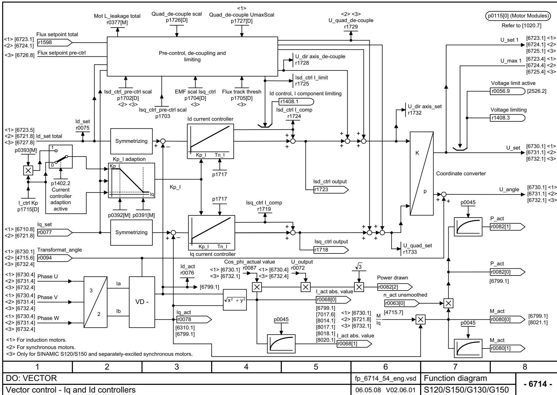
Рис. 2-98 6714 – Iq-регулятор и Id-регулятор
