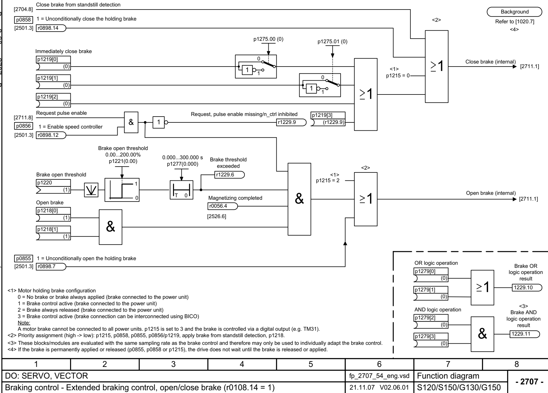
Рис. 2-68 2707 – Расширенная регулировка торможения, включение / выключение тормоза (r0108.14 = 1)
