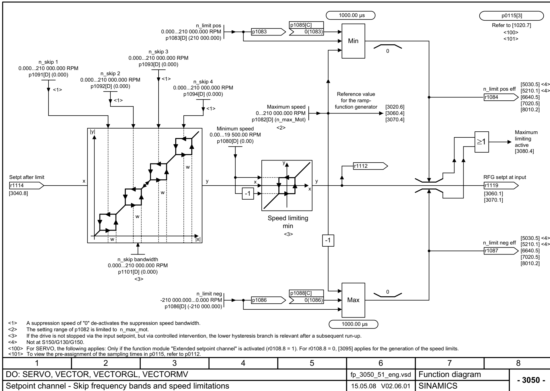
Рис. 2-78 3050 – Выделенные диапазоны и ограничения частоты вращения
