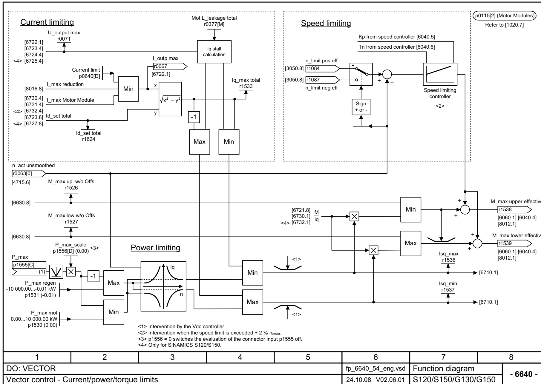
Рис. 2-96 6640 – Пределы тока/мощности/момента
