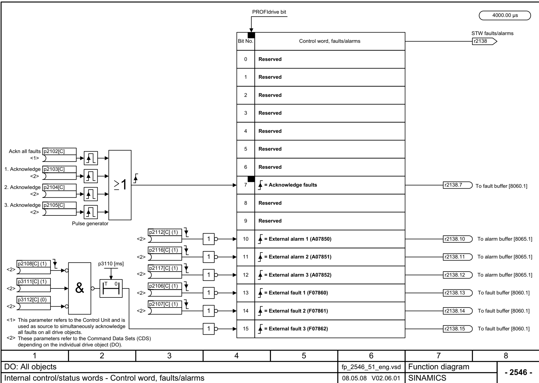
Рис. 2-62 2546 – Управляющее слово - Сообщения о неисправностях/предупреждения
