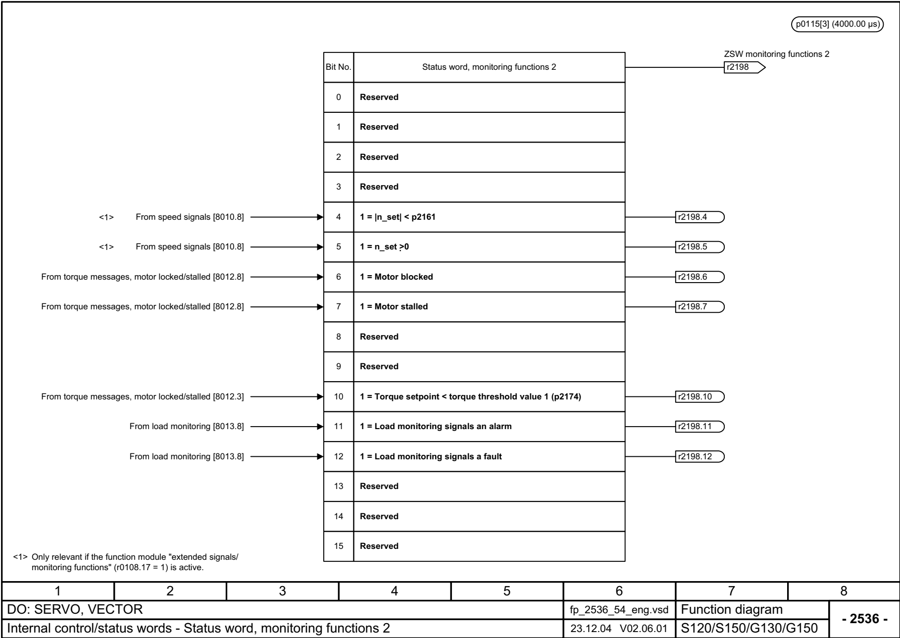
Рис. 2-60 2536 – Слово состояния - Контроль 2
