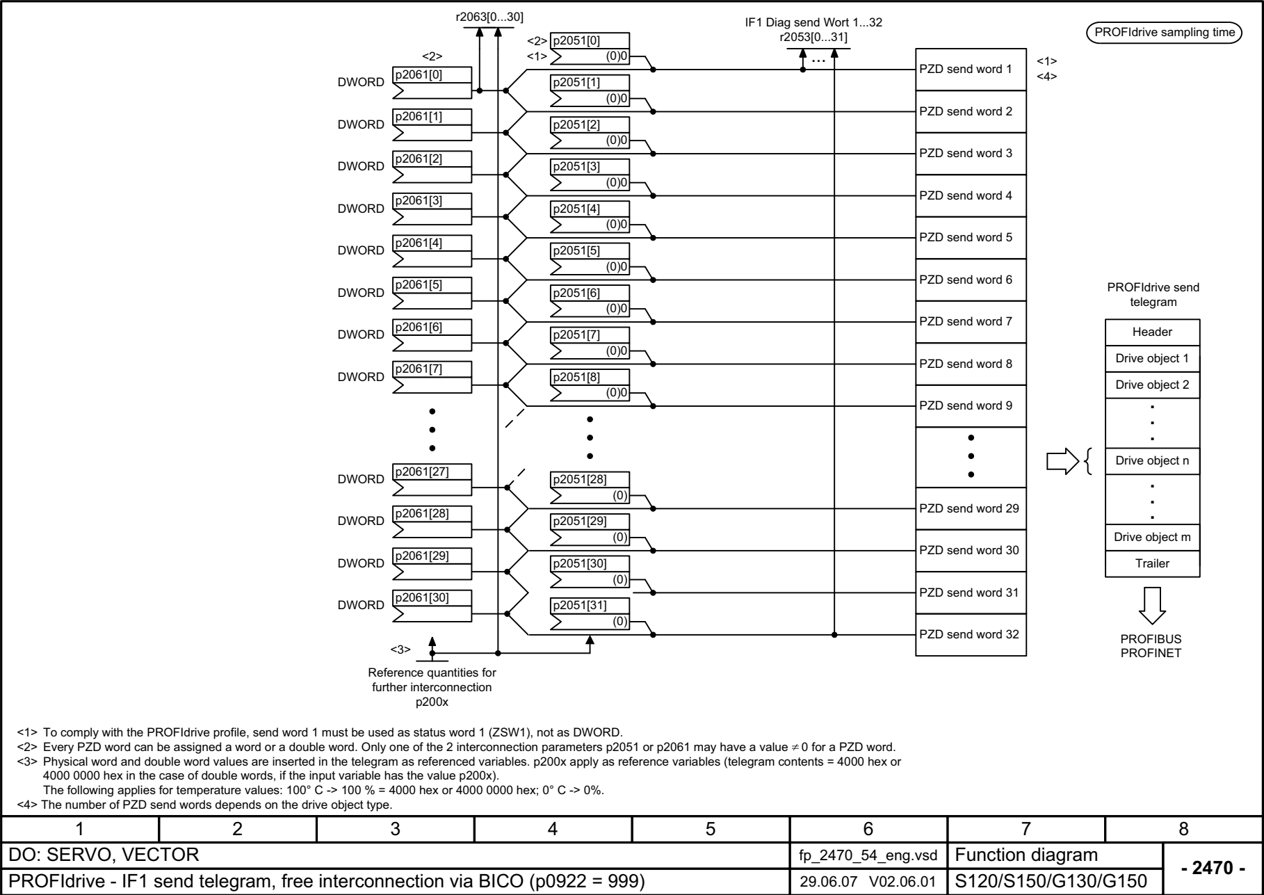
Рис. 2-41 2470 – IF1 Телеграмма передачи - свободное переопределение через BICO (p0922 = 999) ..
