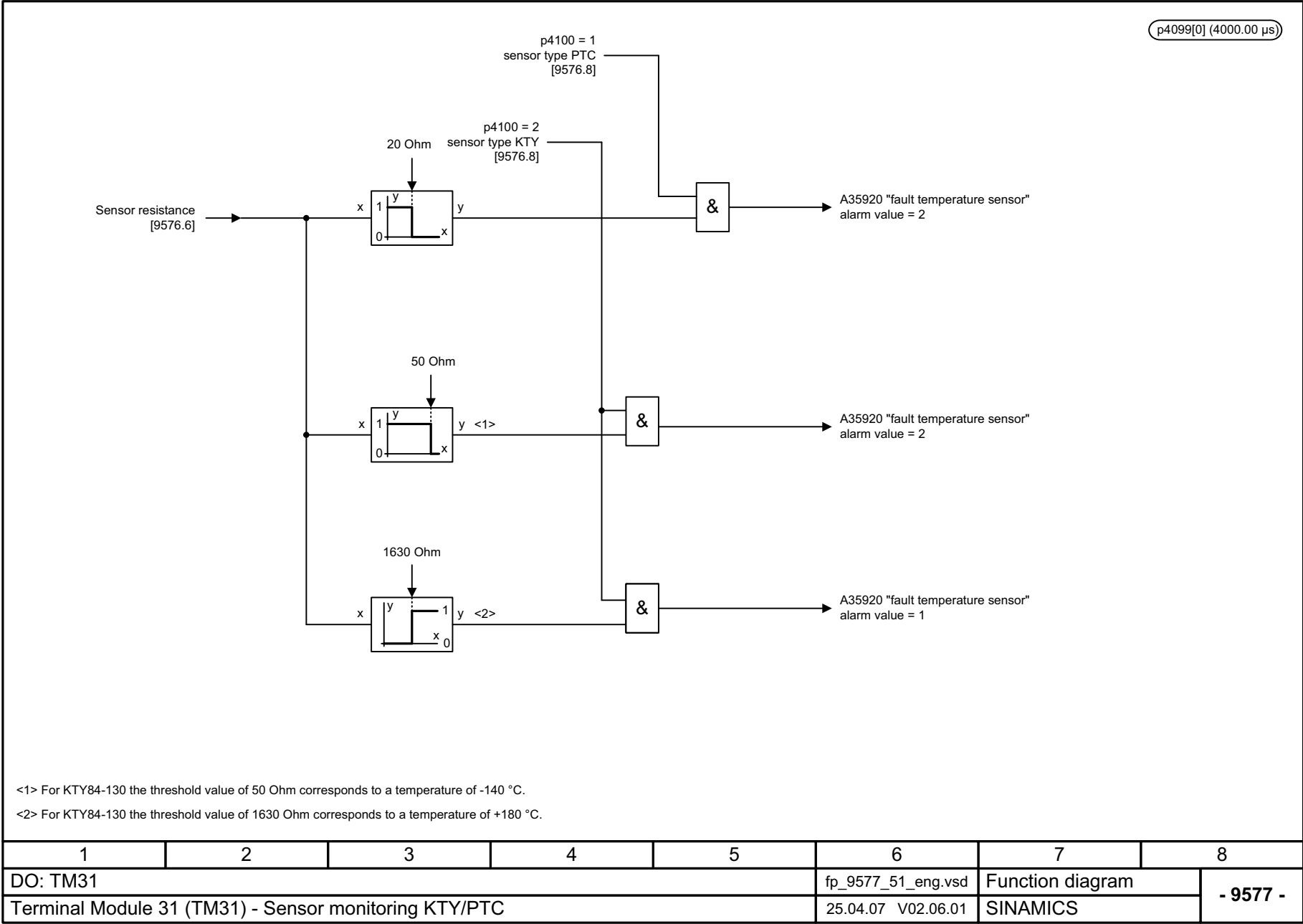
Рис. 2-149 9577 – Контроль датчика КТУ/РТС
