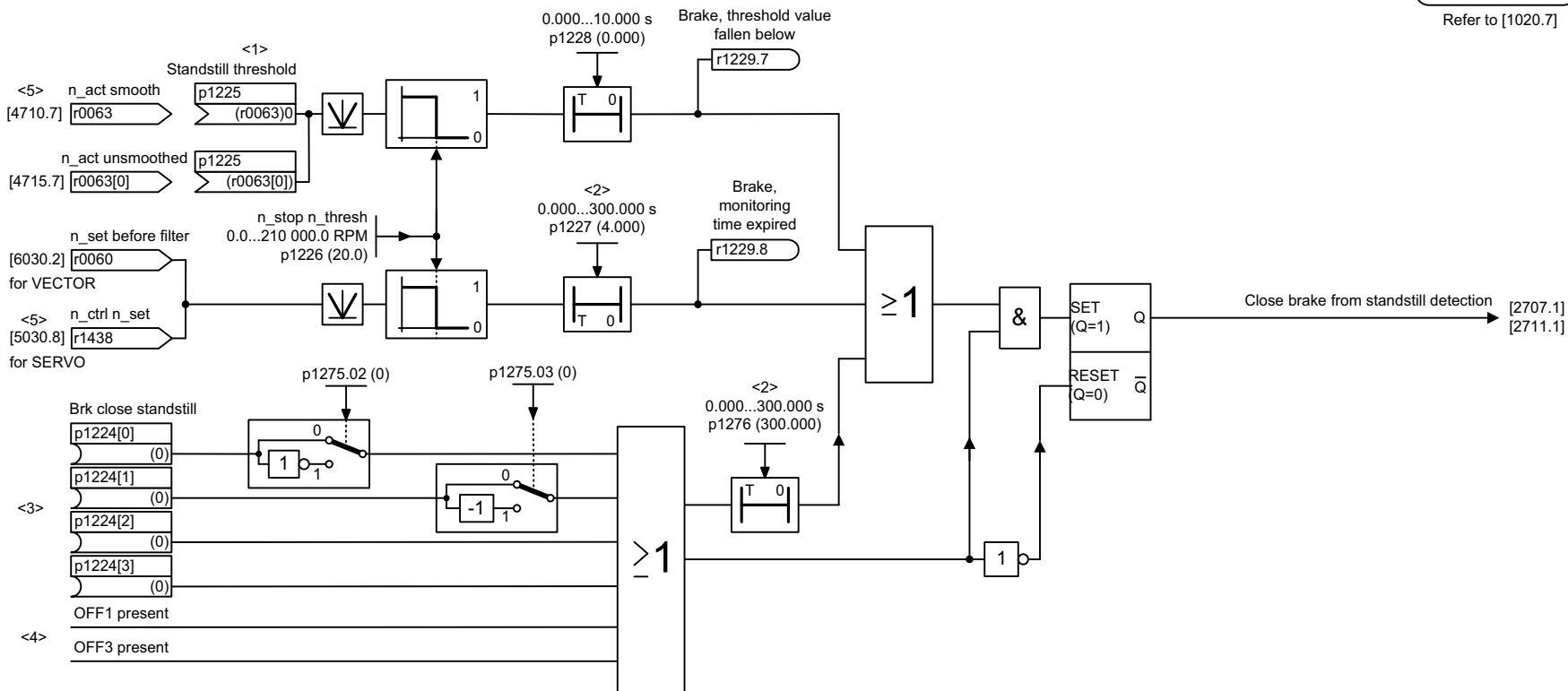
Рис. 2-67 2704 – Расширенная регулировка торможения, распознавание состояния покоя (r0108.14 = 1)
