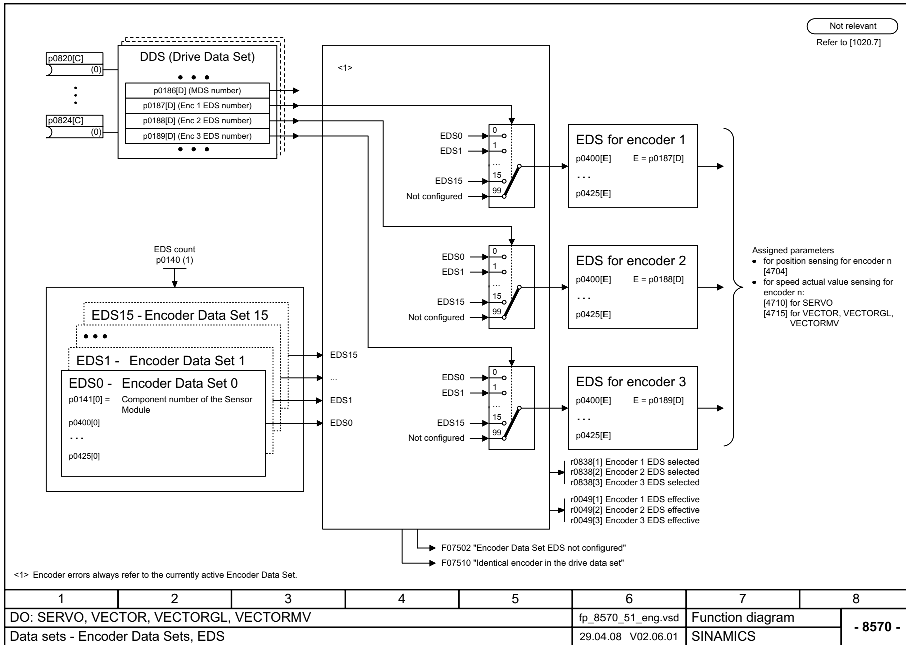
Рис. 2-127 8570 – Наборы данных датчика (Encoder Data Set, EDS)
