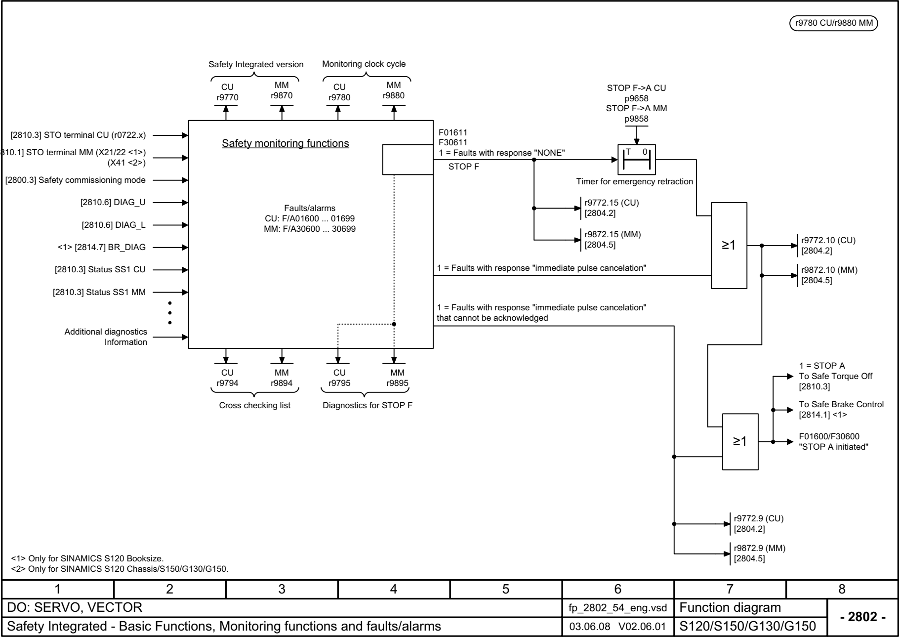
Рис. 2-71 2802 – Основные функции, контроль и неисправности/предупреждения
