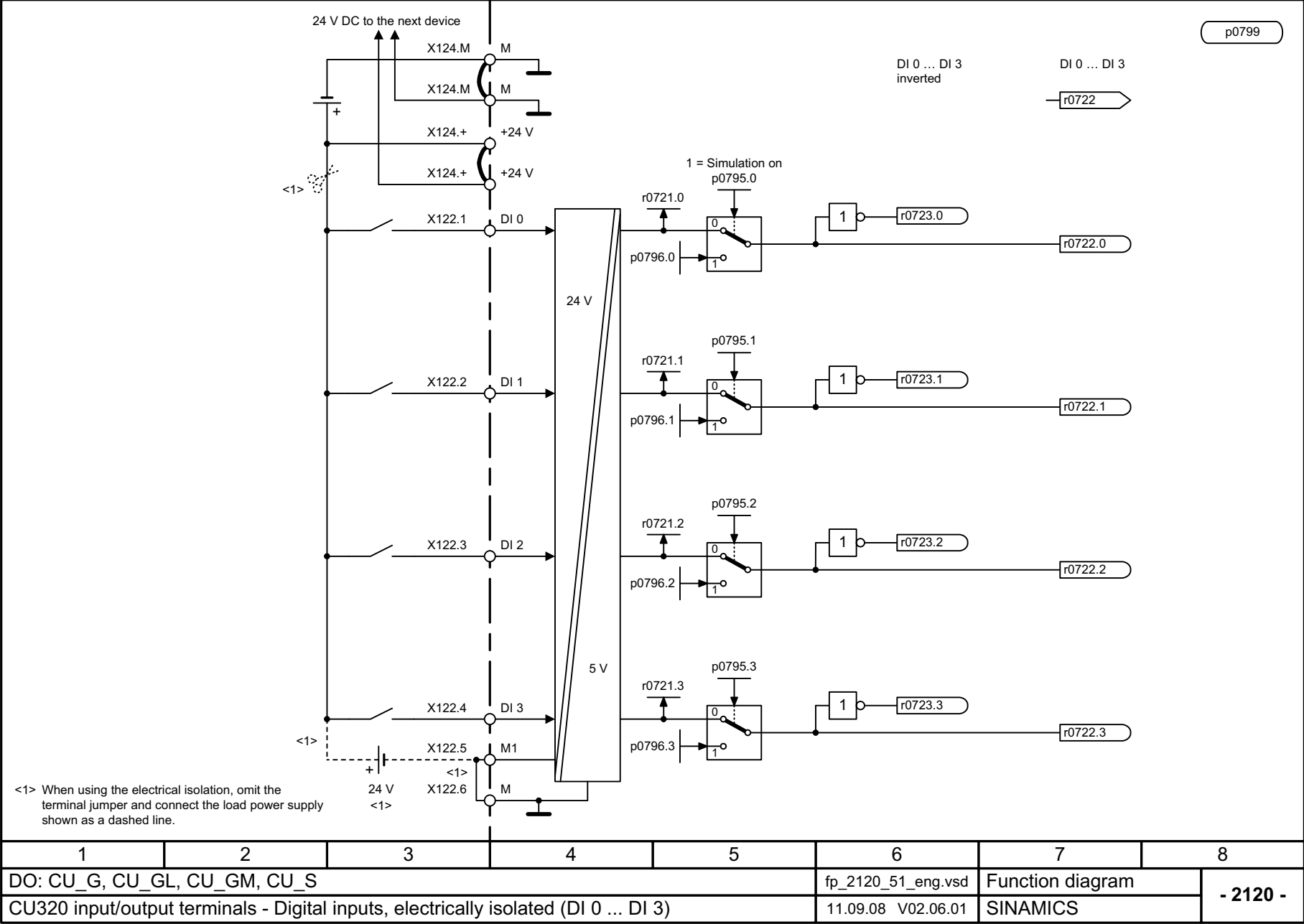
Рис. 2-16 2120 – Цифровые входы с разделением потенциалов (DI 0 ... DI 3)
