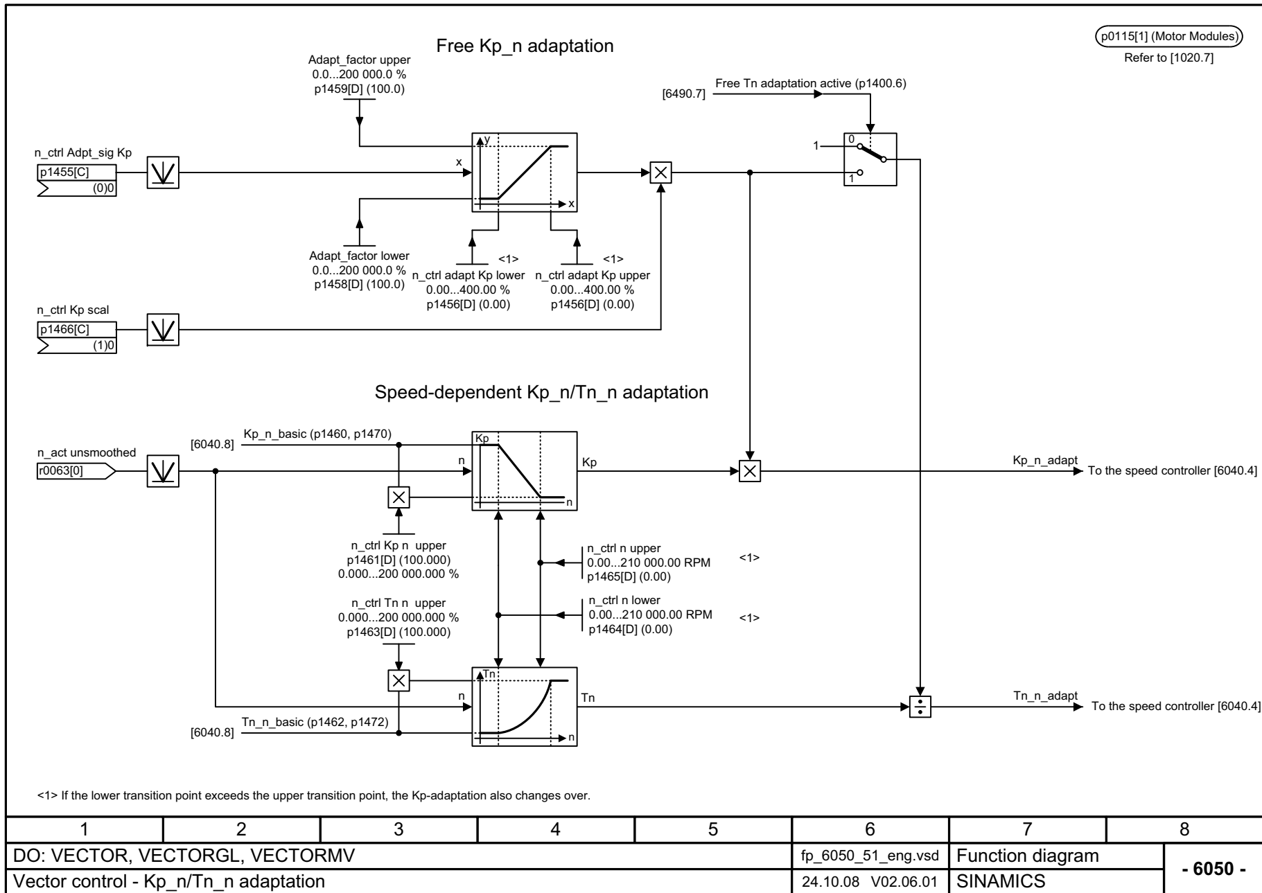
Рис. 2-87 6050 – Согласование Kp_n-/Tn_n
