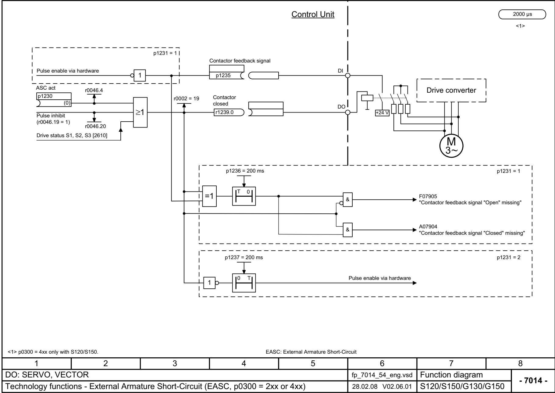
Рис. 2-107 7014 – Внешнее короткое замыкание якоря (EASC, p0300 = 2xx)
