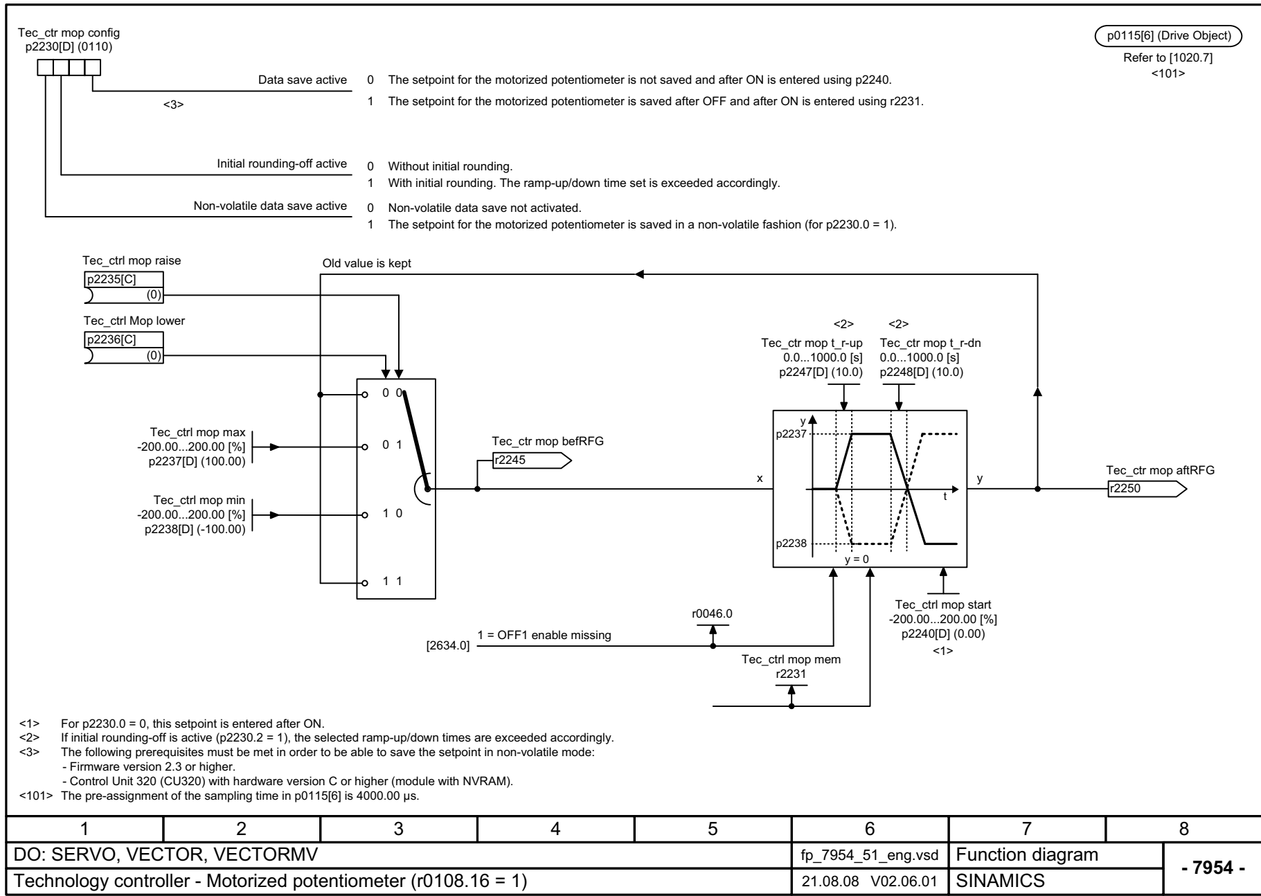
Рис. 2-112 7954 – Потенциометр двигателя (r0108.16 = 1)
