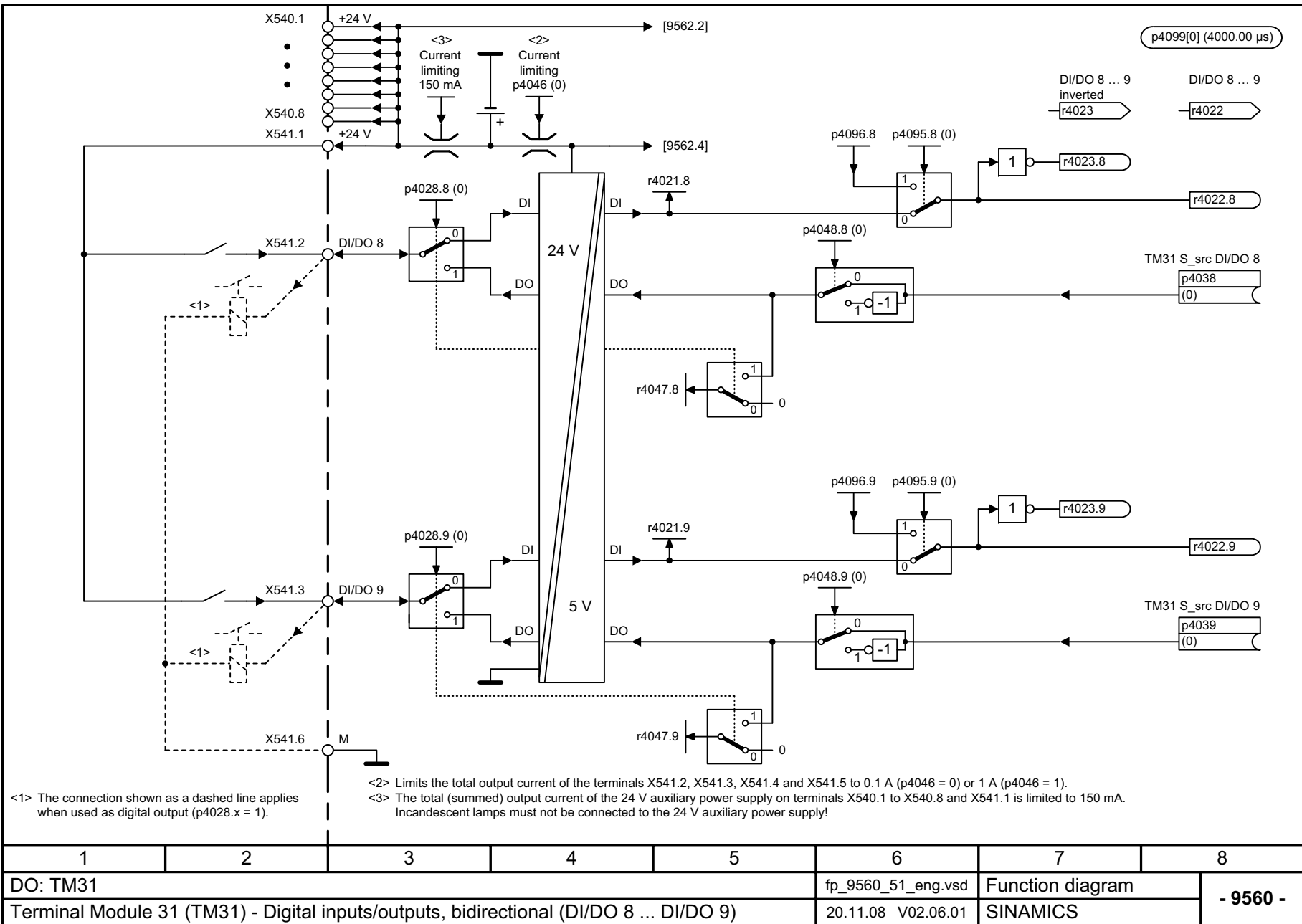
Рис. 2-143 9560 – Цифровые входы/выходы двусторонние (DI/DO 8 ... DI/DO 9)
