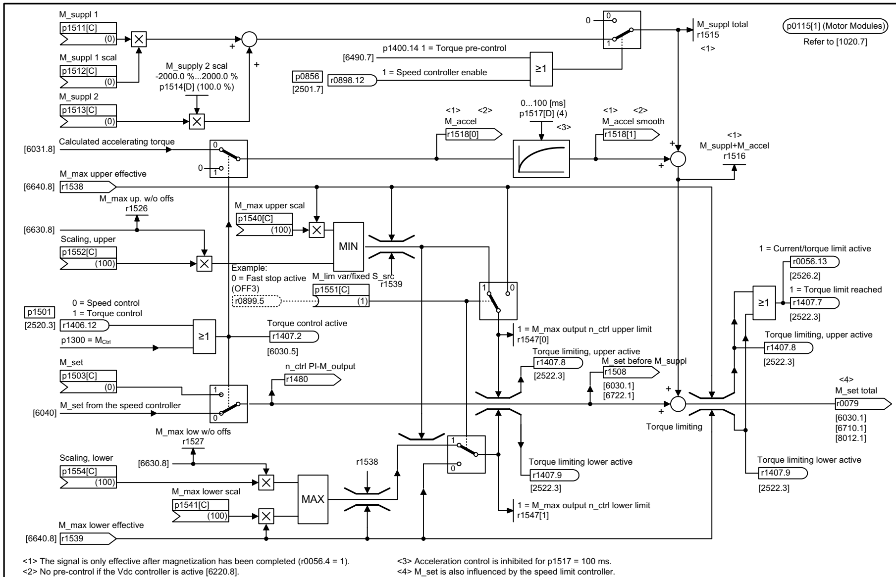
Рис. 2-88 6060 – Заданное значение крутящего момента
