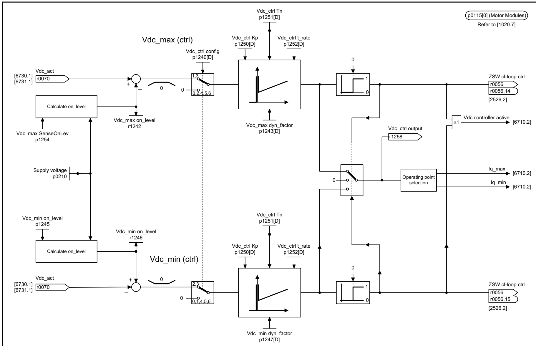
Рис. 2-89 6220 – Перулятор Vdc_max и перулятор Vdc_min
