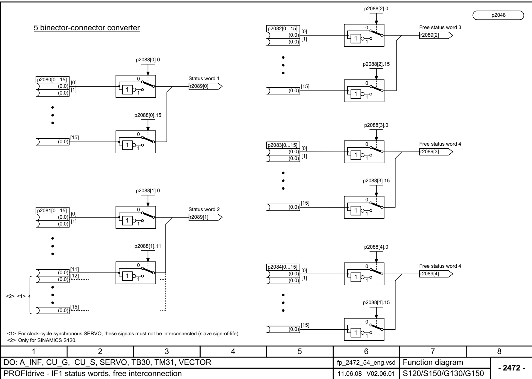
Рис. 2-42 2472 – IF1 Слова состояния - свободное переключение
