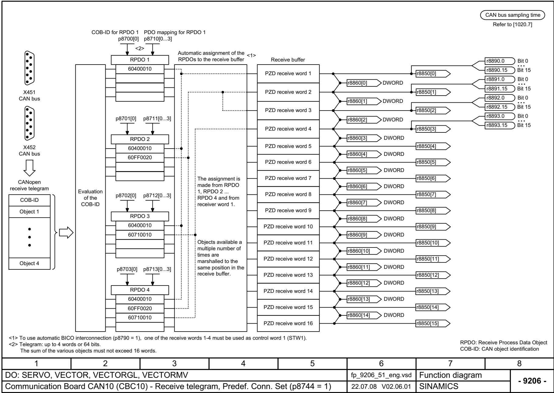
Рис. 2-135 9206 – Приемная телеграмма - Predefined Connection Set (p8744 = 1)
