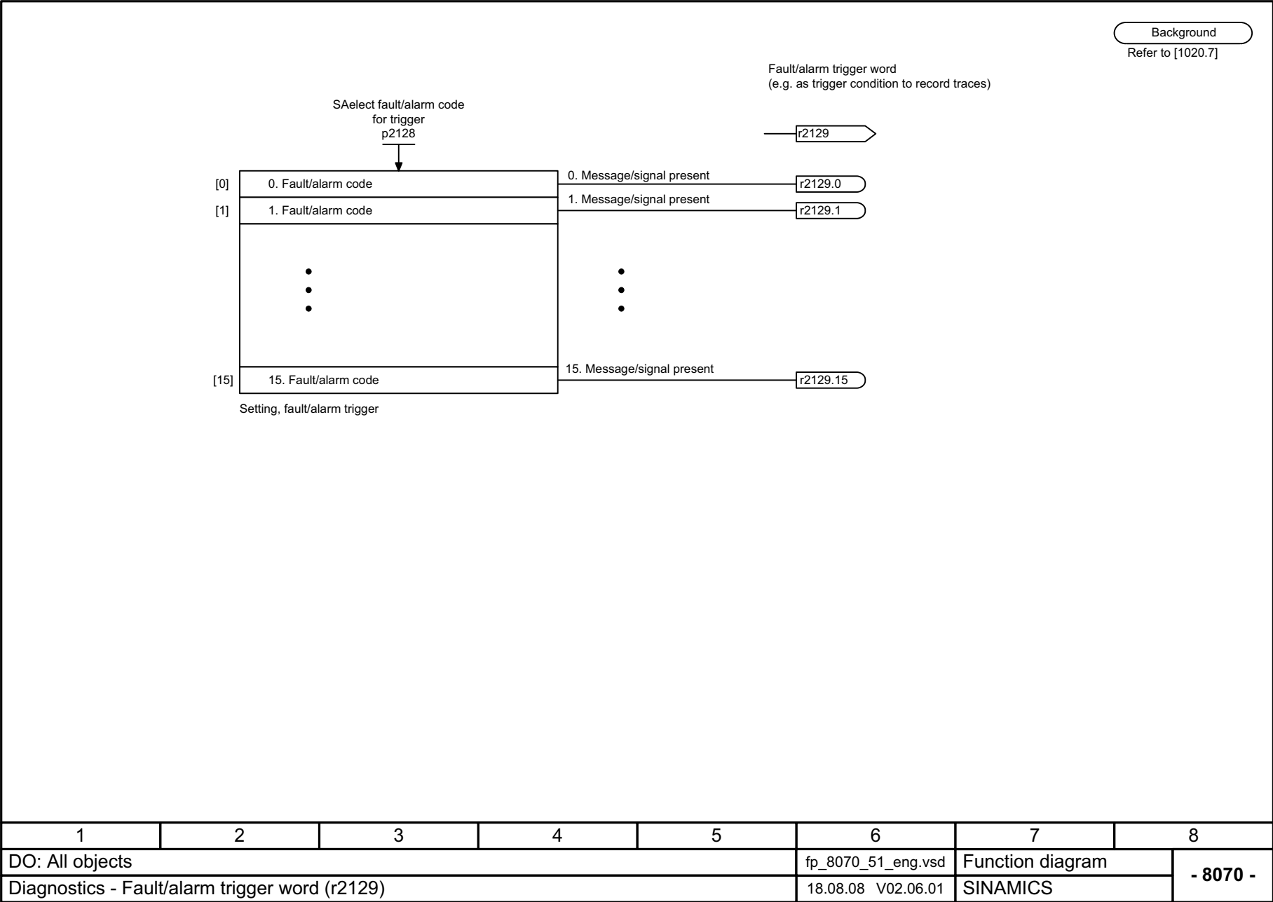
Рис. 2-122 8070 – Триггерное слово сообщений о неисправностях/предупреждений (r2129)
