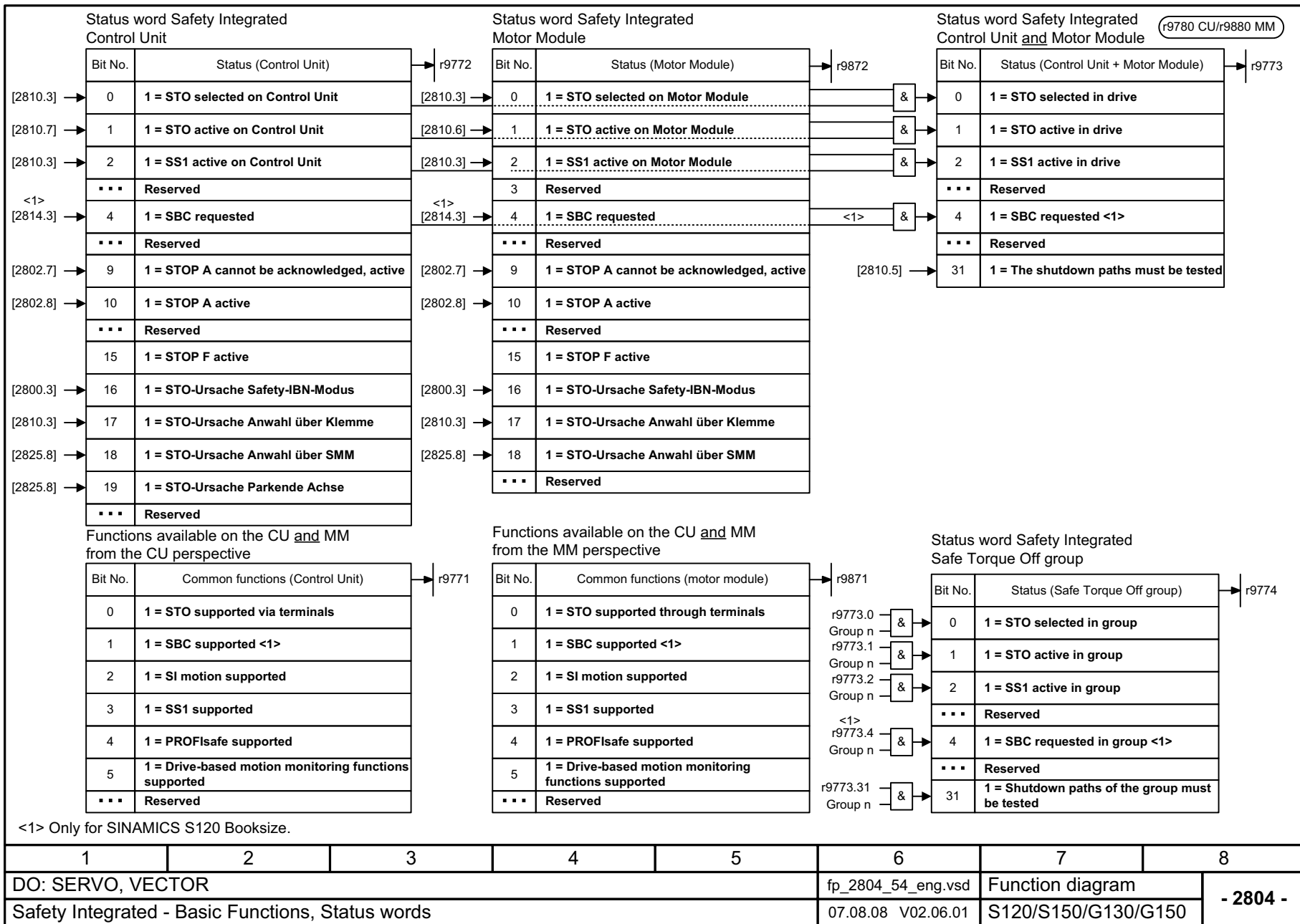
Рис. 2-72 2804 – Основные функции, слово состояния
