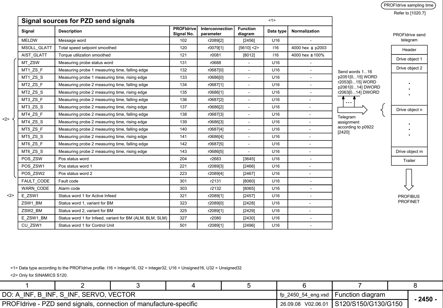
Рис. 2-36 2450 – Подключение сигналов передачи PZD по производителю
