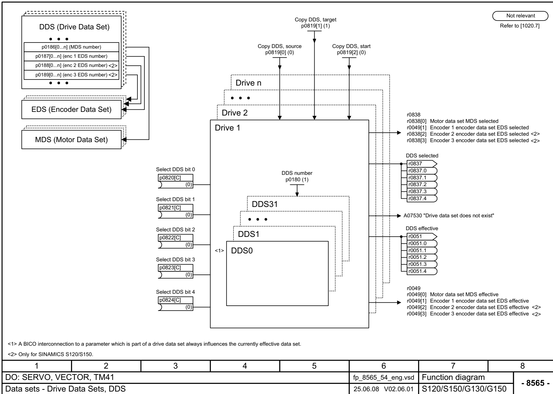
Рис. 2-126 8565 – Наборы приводных данных (Drive Data Set, DDS)
