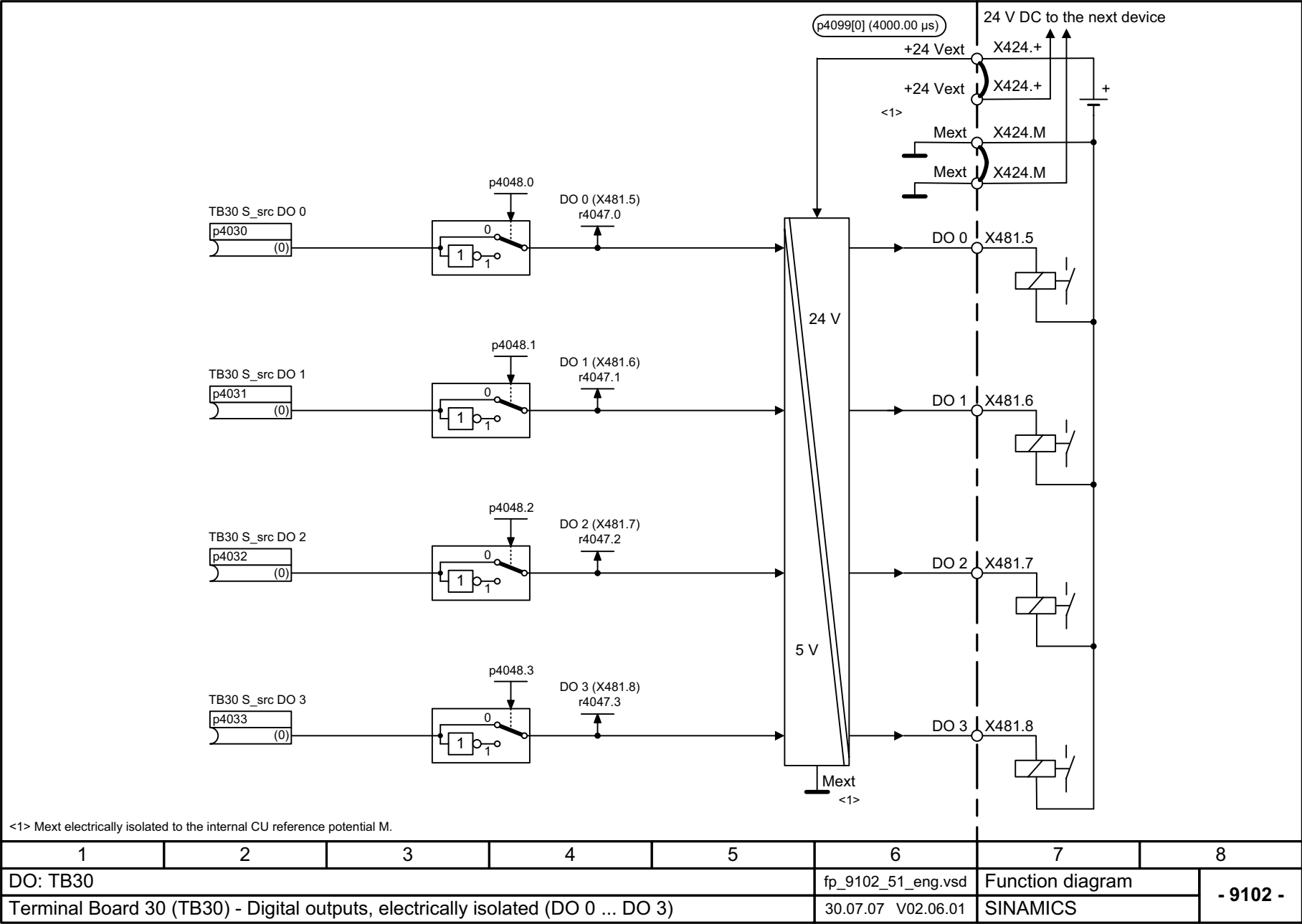
Рис. 2-131 9102 – Цифровые выходы с разделением потенциалов (DO0 ... DO3)
