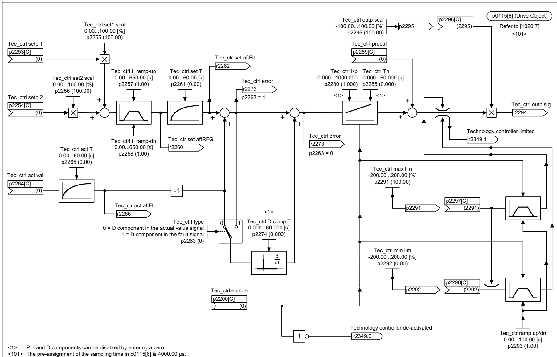
Рис. 2-113 7958 – Перуировка (r0108.16 = 1)
