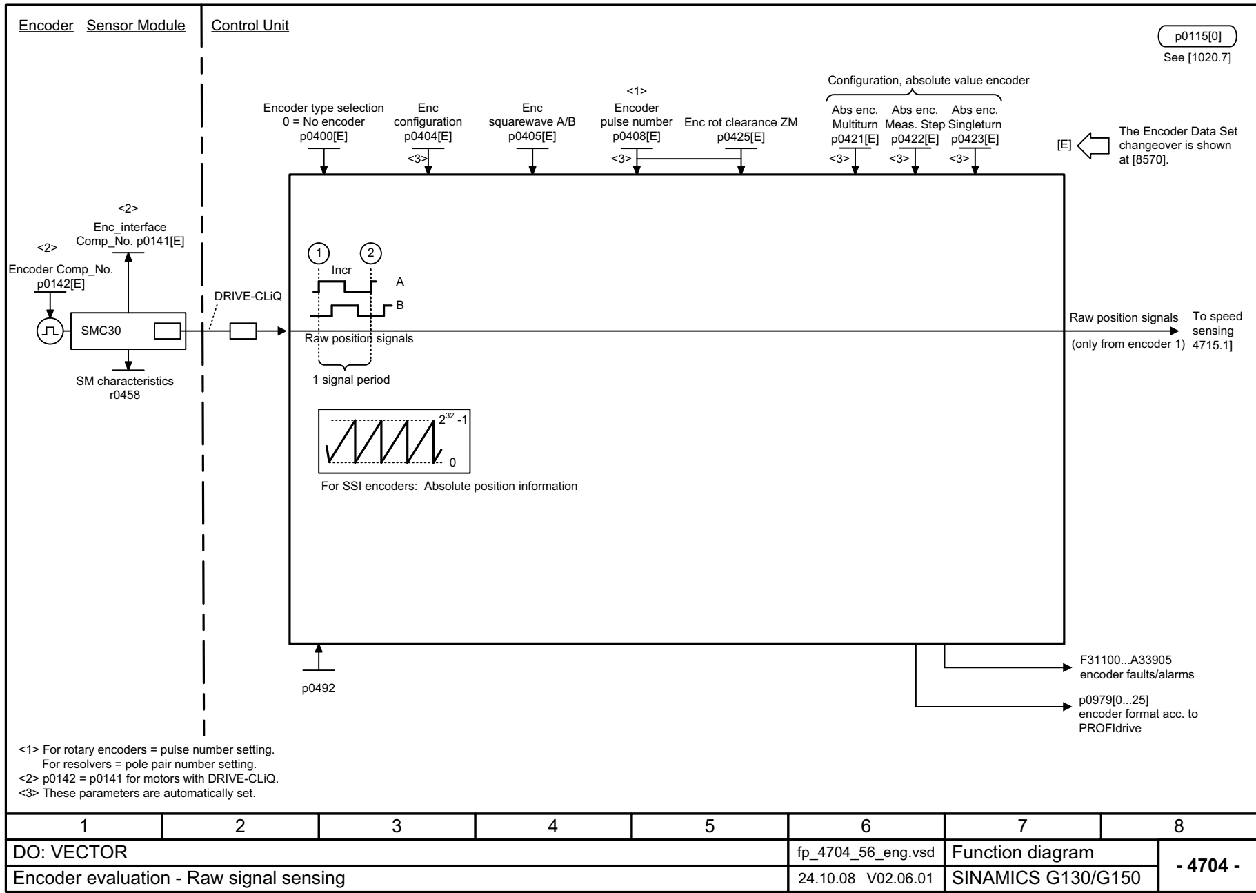
Рис. 2-82 4704 – Регистрация необработанного сигнала
