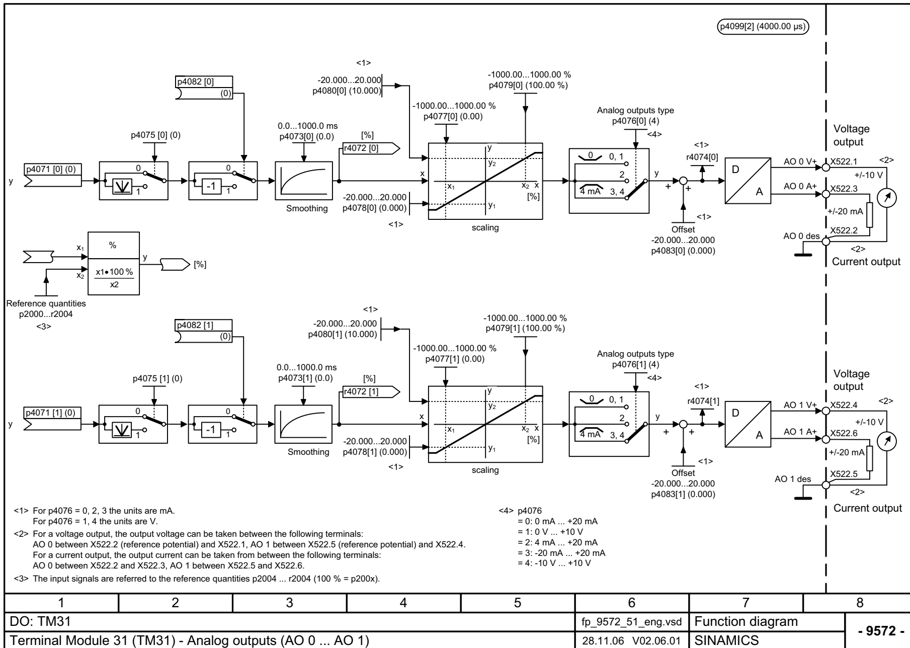
Рис. 2-147 9572 – Аналоговые выходы (AO 0 ... AO 1)
