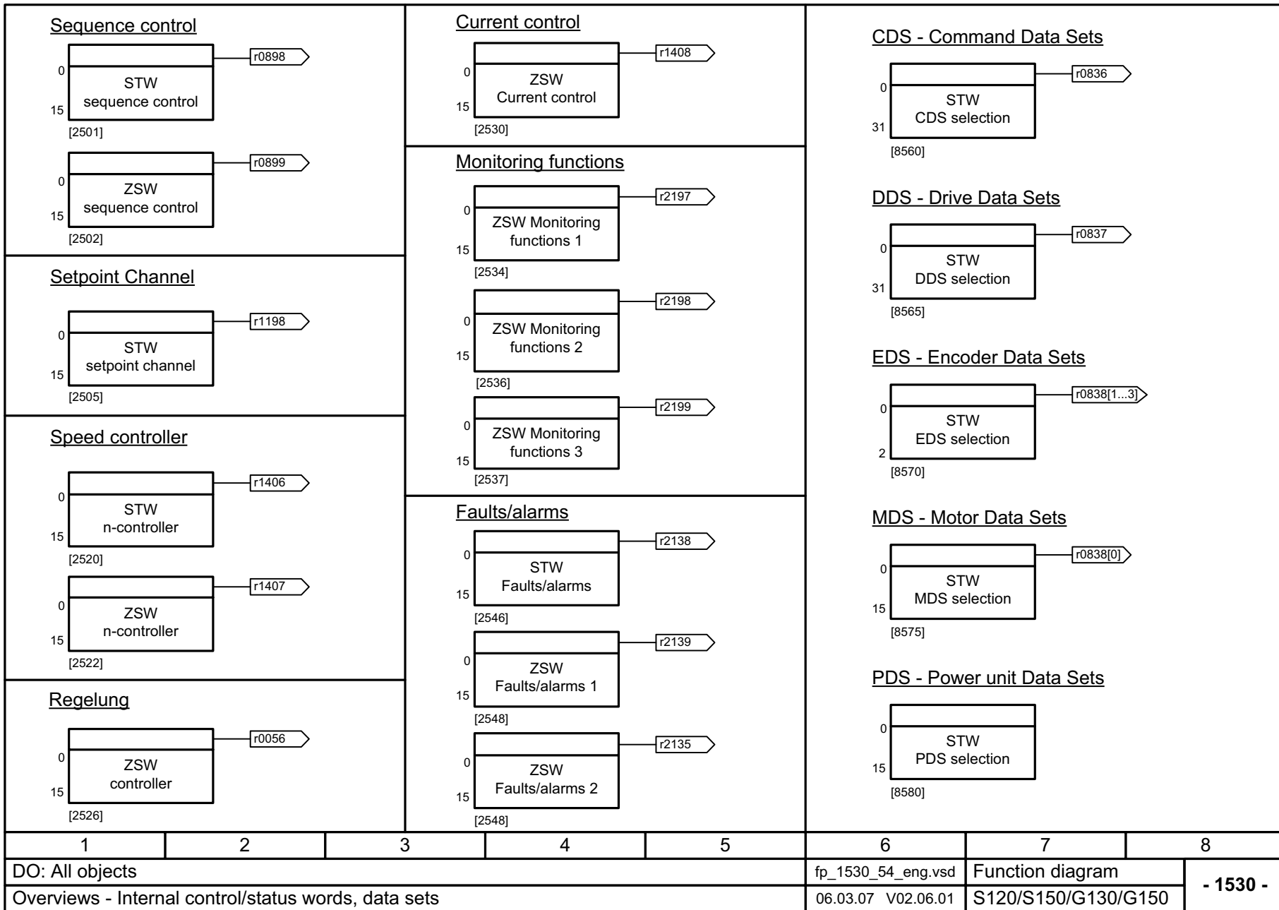
Рис. 2-7 1530 – Внутренние управляющие слова / слова состояний, наборы данных
