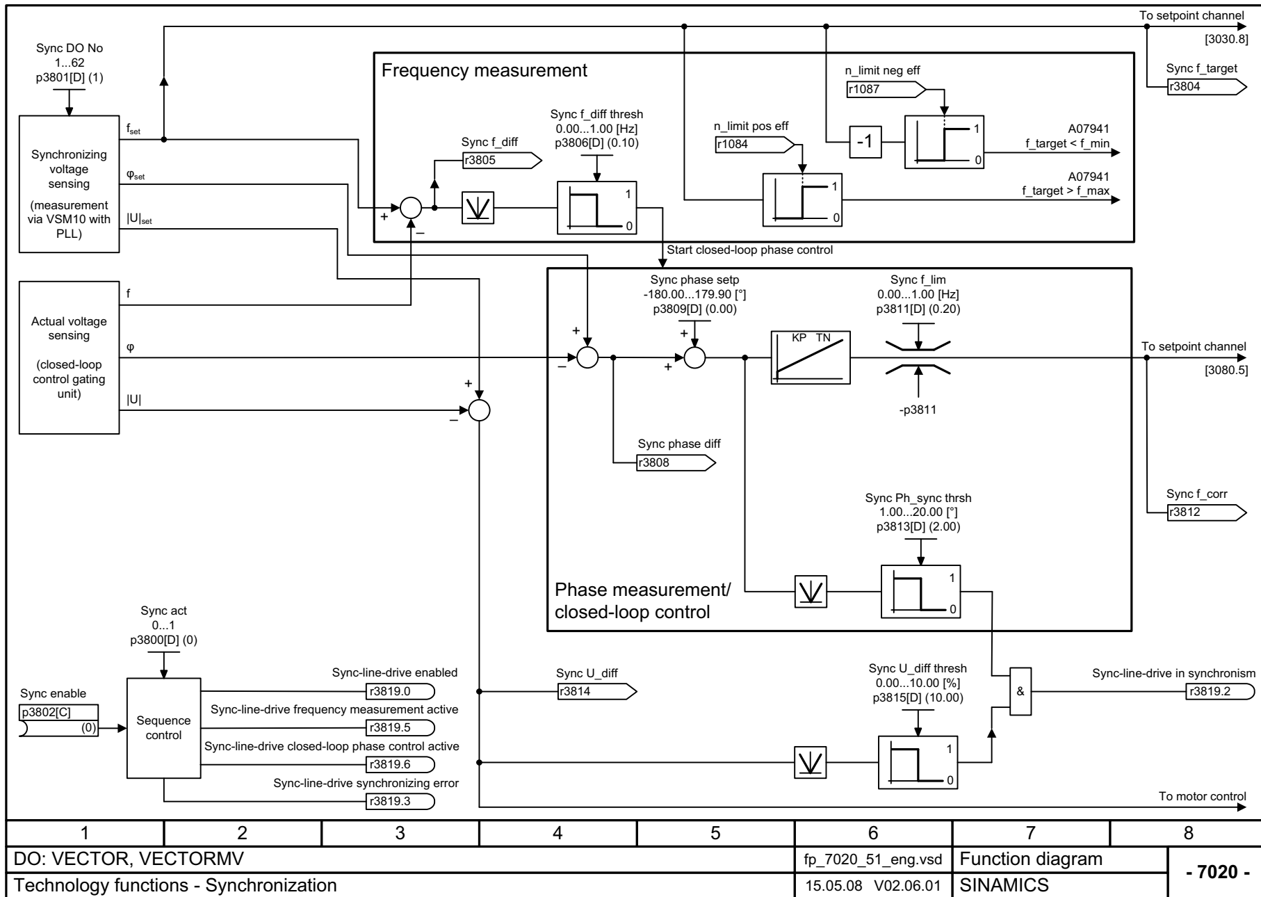
Рис. 2-110 7020 – Синхронизация
