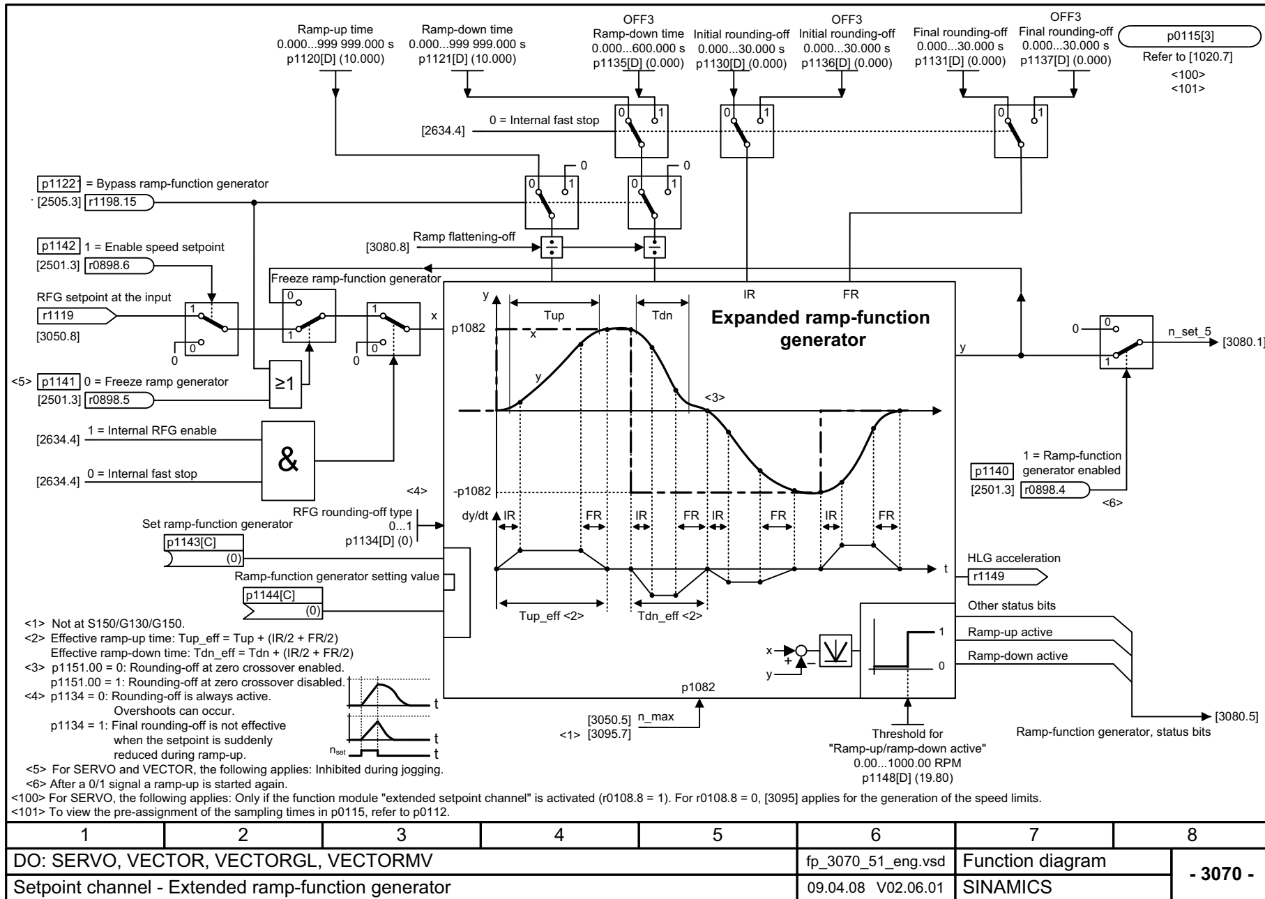
Рис. 2-80 3070 – Расширенный датчик разгона
