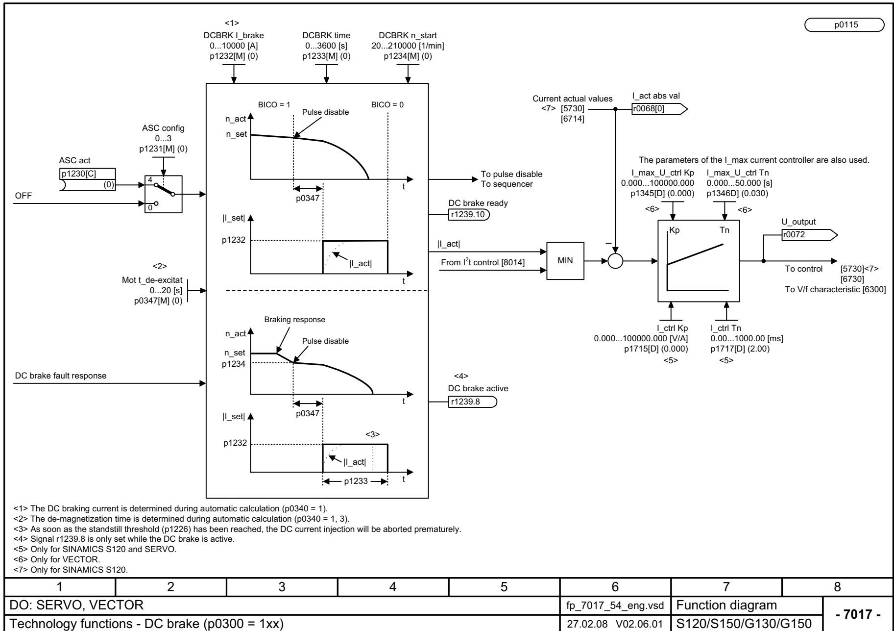
Рис. 2-109 7017 – Тормоз постоянного тока (p0300 = 1xx)
