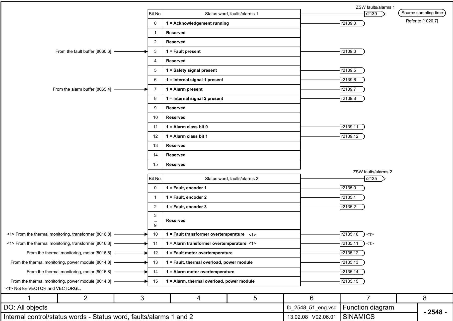
Рис. 2-63 2548 – Слово состояния - Сообщения о неисправностях/предупреждения 1 и 2
