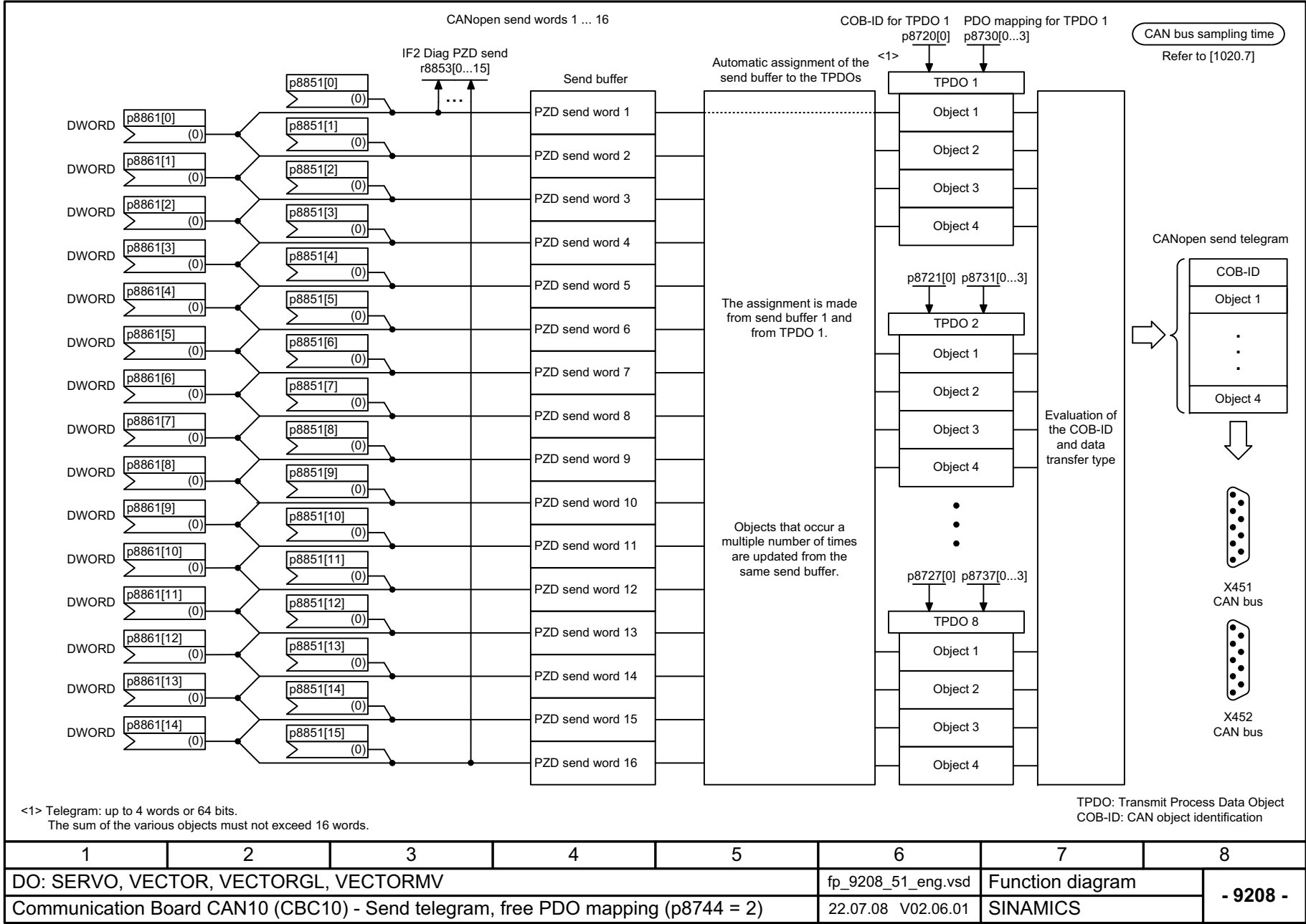
Рис. 2-136 9208 – Телеграмма отправки - Свободное назначение РДО (p8744 = 2)
