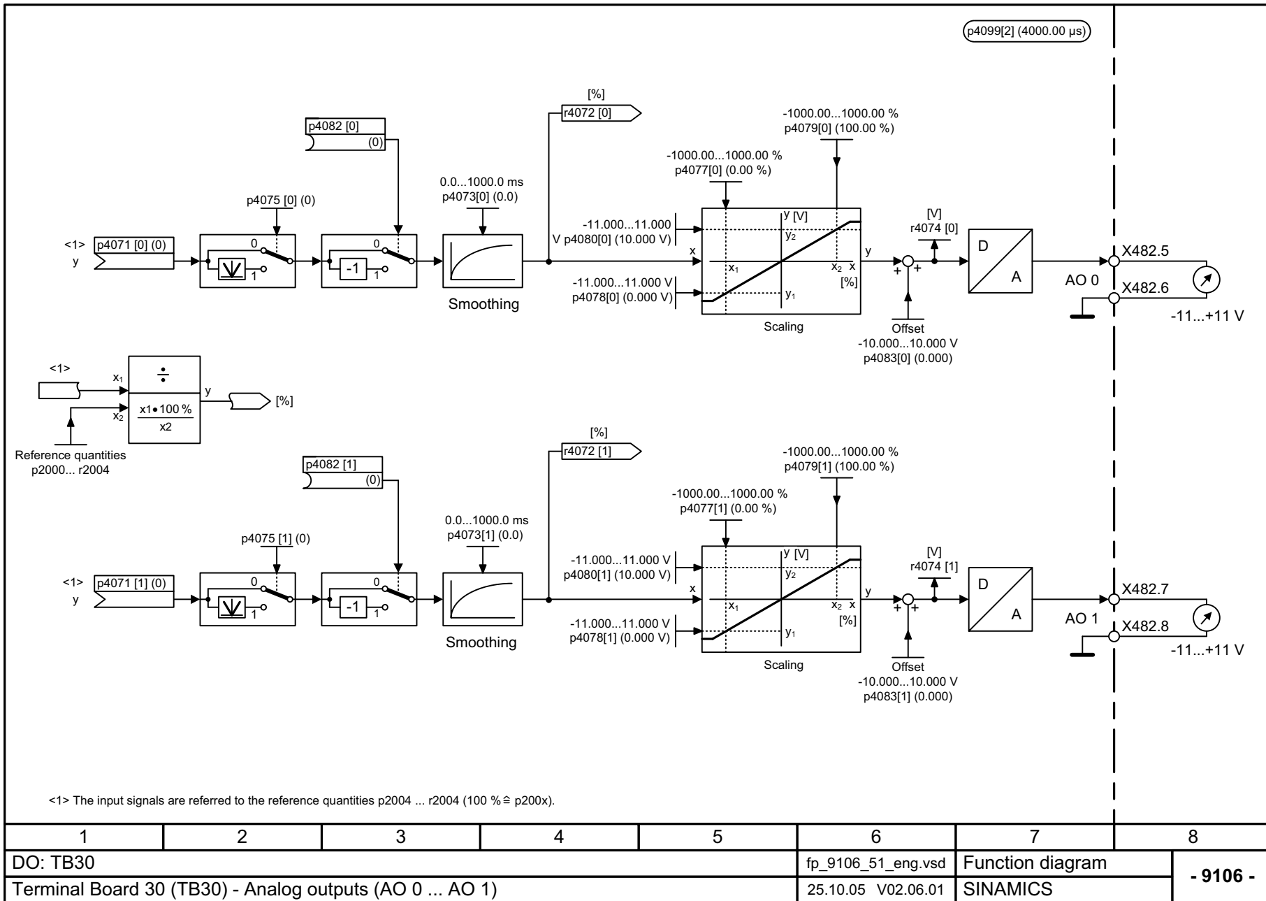
Рис. 2-133 9106 – Аналоговые выходы (АО 0 ... АО 1)
