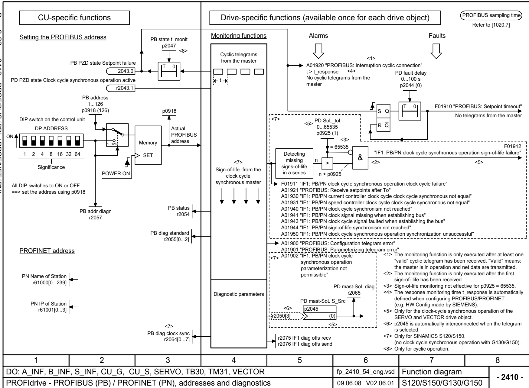
Рис. 2-22 2410 – PROFIBUS (PB) / PROFINET (PN), адреса и диагностика
