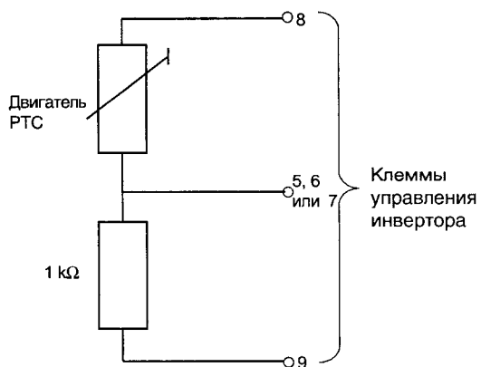
Рис. 3-6 Подключение PTC датчика перегрузки двигателя
