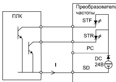
Вход с отрицательной логикой: многофункциональная клемма управления соединена с разомкнутым коллектором ПЛК
