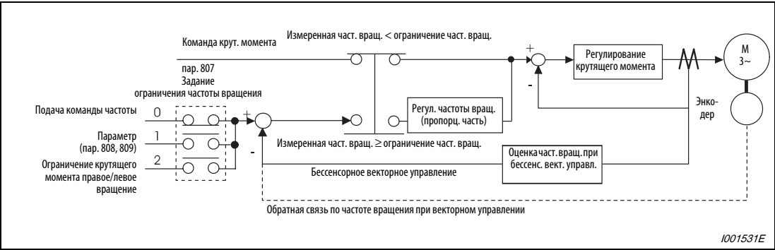
Рис. 6-30: Блок-схема
