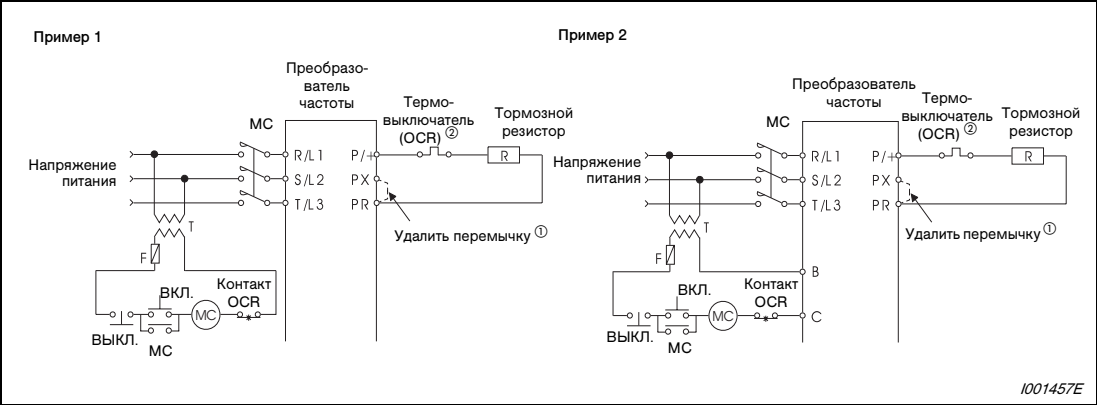
Рис. 3-33: Защитная схема
