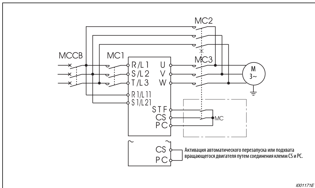
Рис. 6-156: Пример подключения
