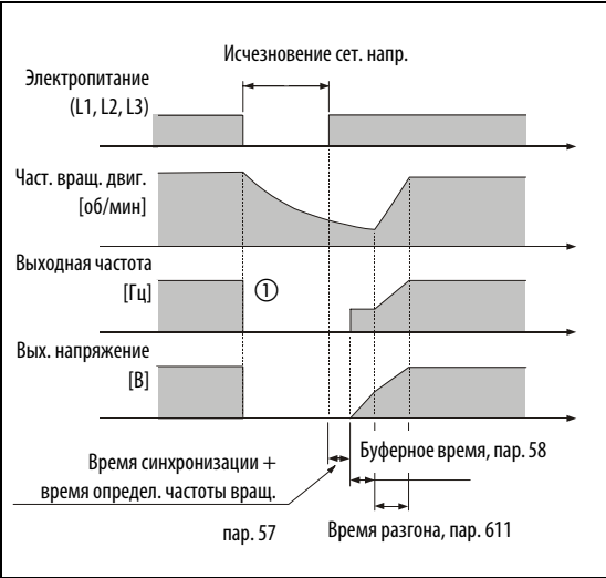
Рис. 6-157: Управление по характеристике U/f и расширенное управление вектором потока
