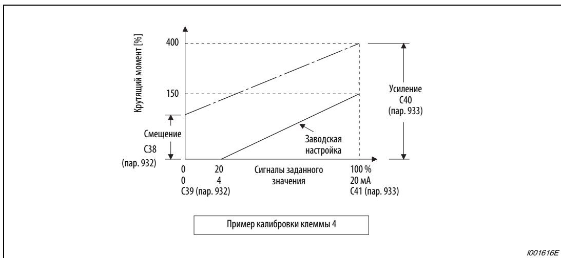
Рис. 6-192: Настройка сигнала на клемме 4
