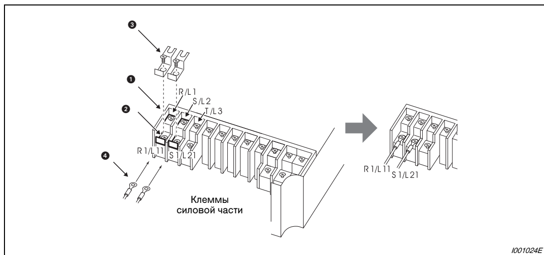
Рис. 3-9: Детализированный вид клемм
