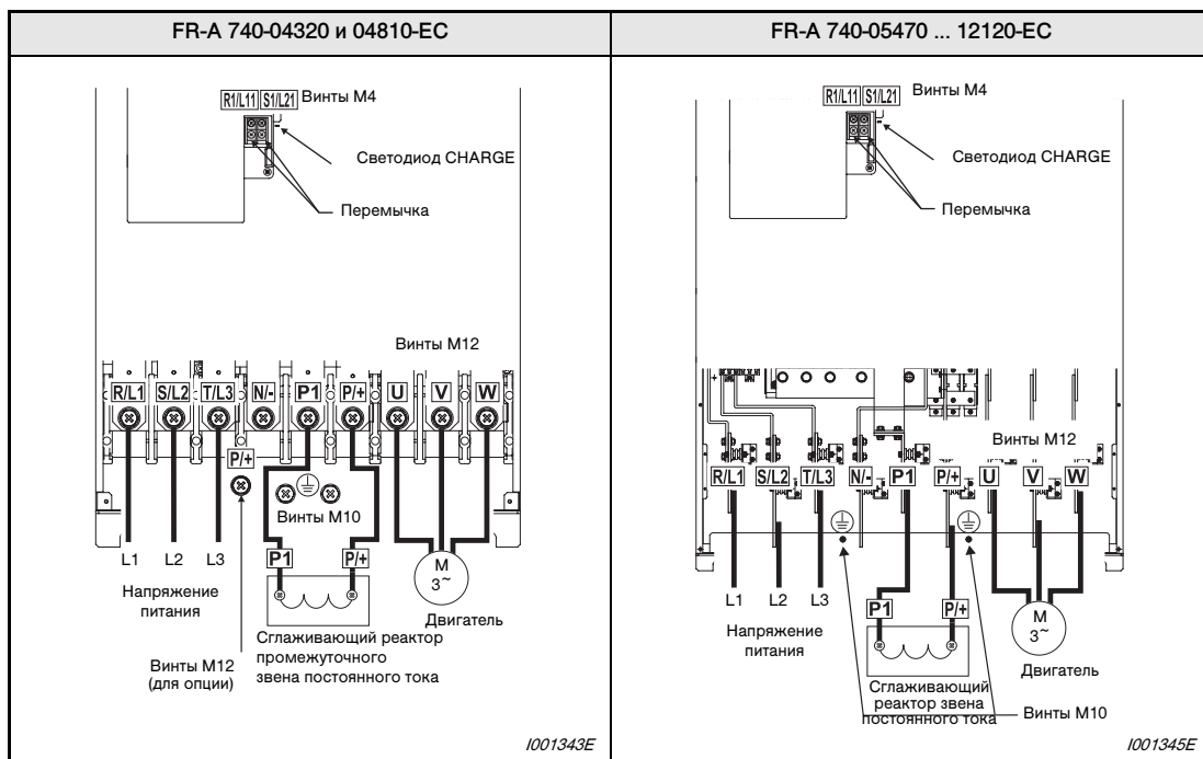
Таб. 3-3: Разводка клемм и электропроводка (3)
