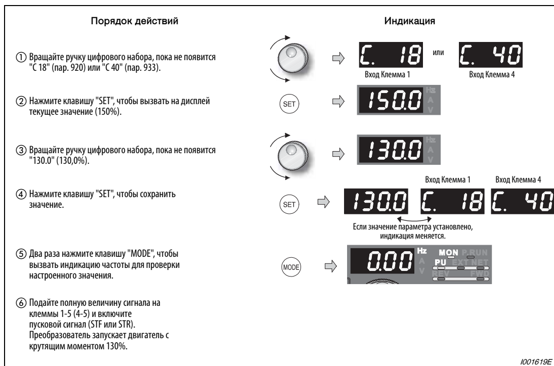
Рис. 6-195: Установка крутящего момента без изменения настроек входного сигнала напряжения (тока)
