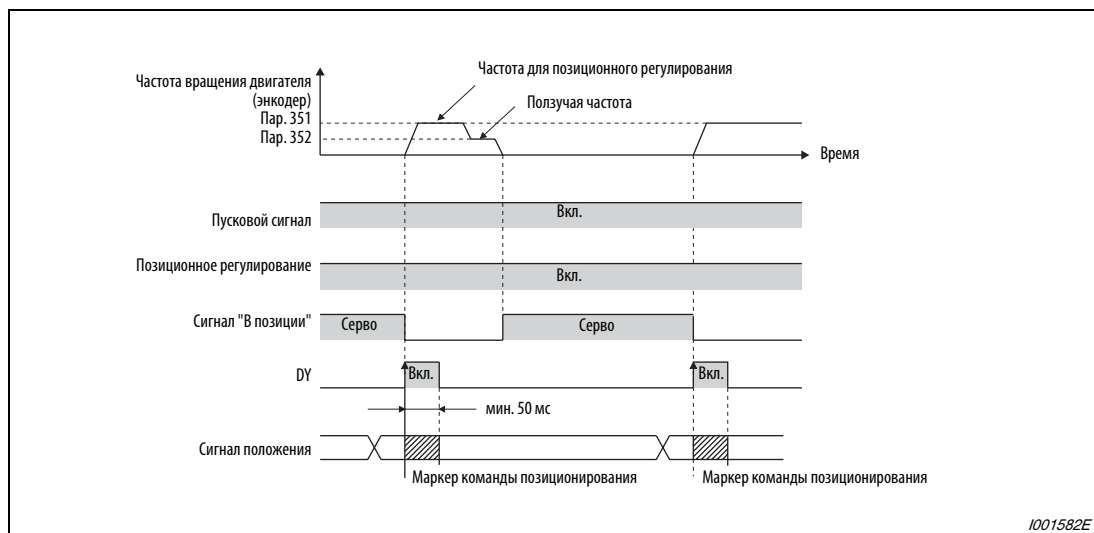
Рис. 6-118: Многопозиционная ориентация
