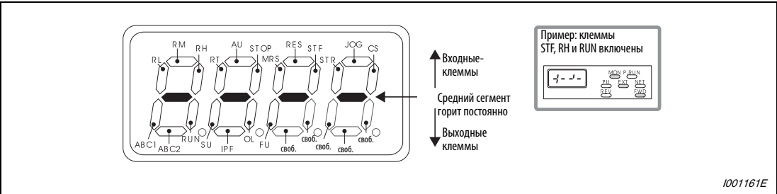
Рис. 6-145: Индикация состояний клемм ввода-вывода
