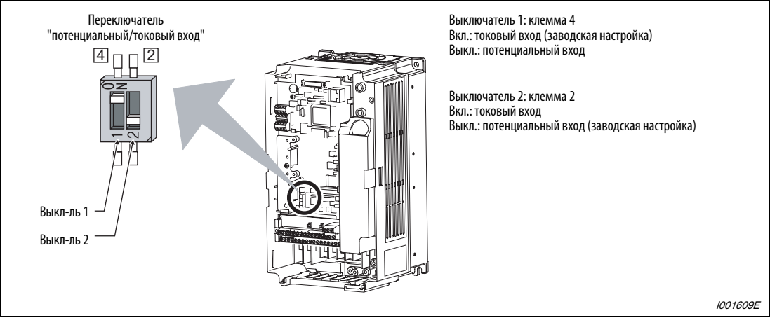
Рис. 6-175: Переключатель "потенциальный/токовый вход"
