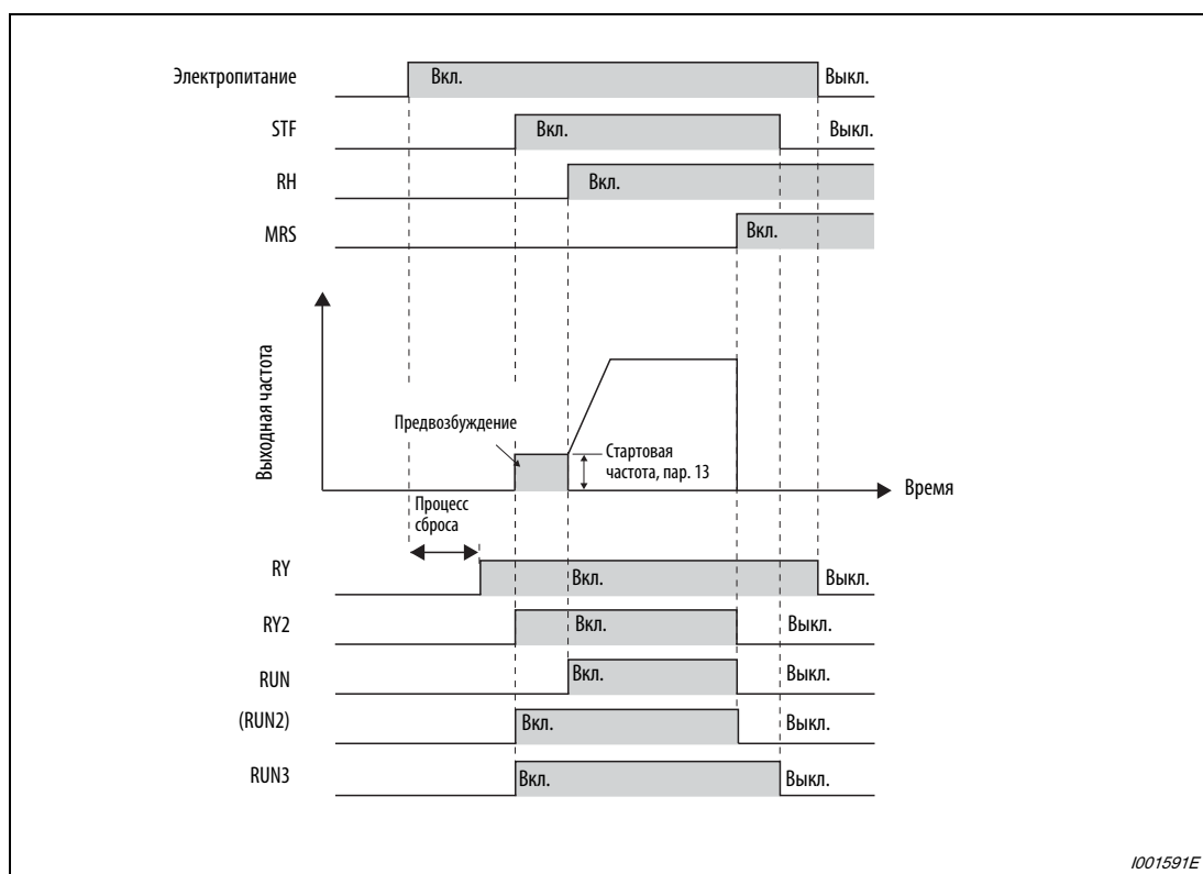
Рис. 6-132: Готовность к работе и вращение двигателя
