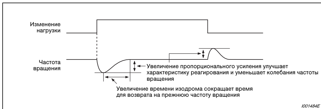
Рис. 5-15: Характеристика частоты вращения при изменении нагрузки
