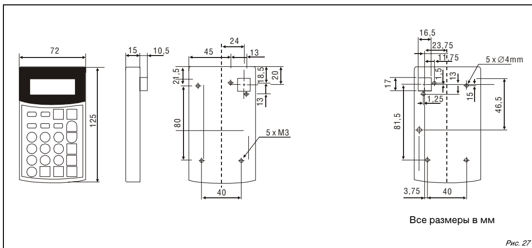
Рис. А-20: Пульт управления FR-PU04
