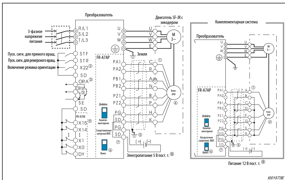
Рис. 6-113: Пример схемы
