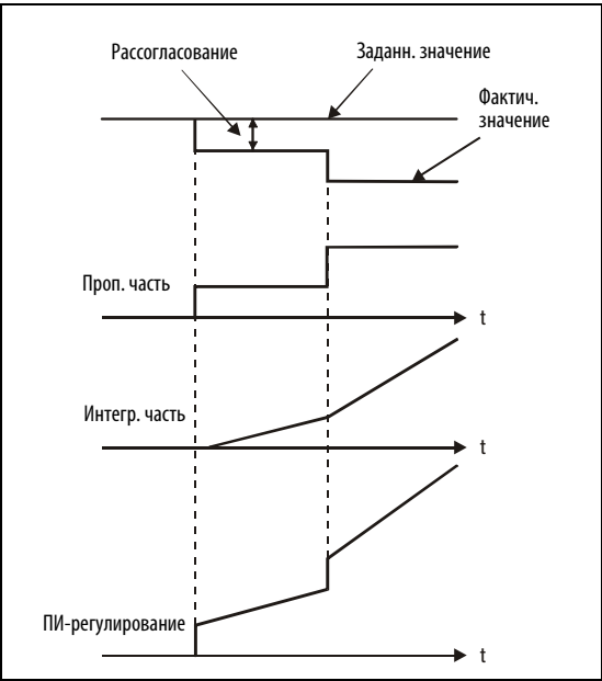
Рис. 6-237: Принцип действия ПИ-регулятора
