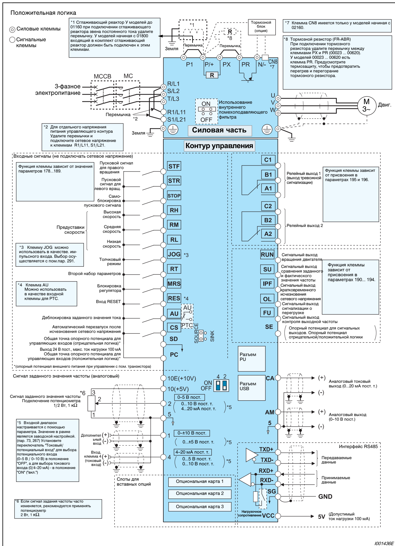
Рис. 3-3: Схема подключения преобразователя частоты
