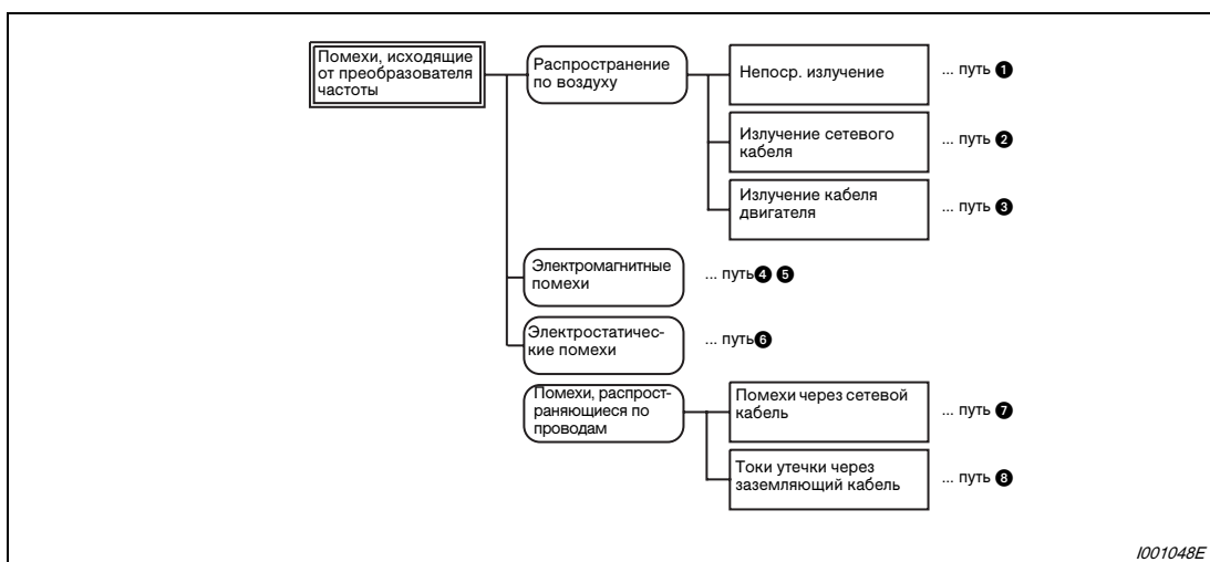
Рис. 3-47: Распространение помех
