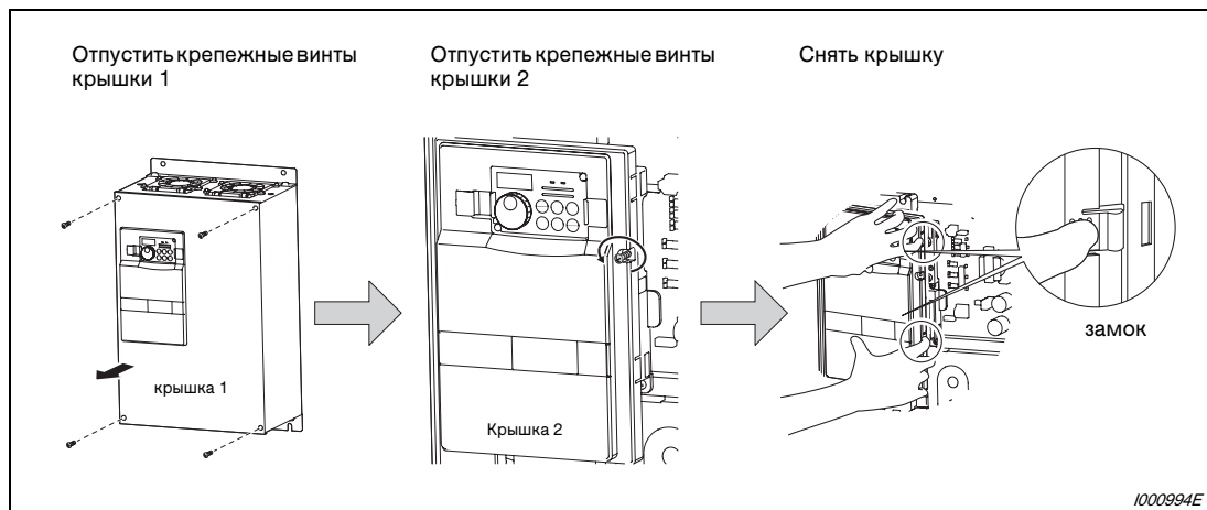
Рис. 2-4: Снятие передней крышки
