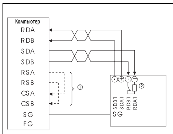
Рис. 6-218: Соединение с одним преобразователем частоты
