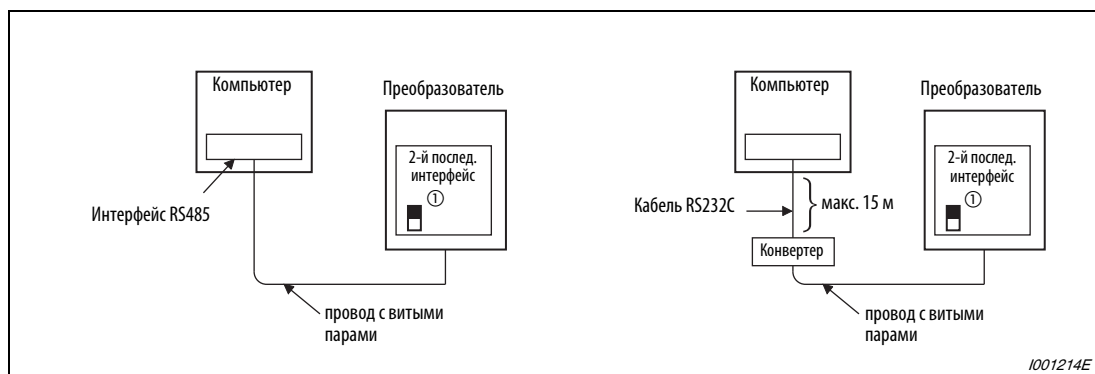
Рис. 6-216: Соединение с одним преобразователем частоты
