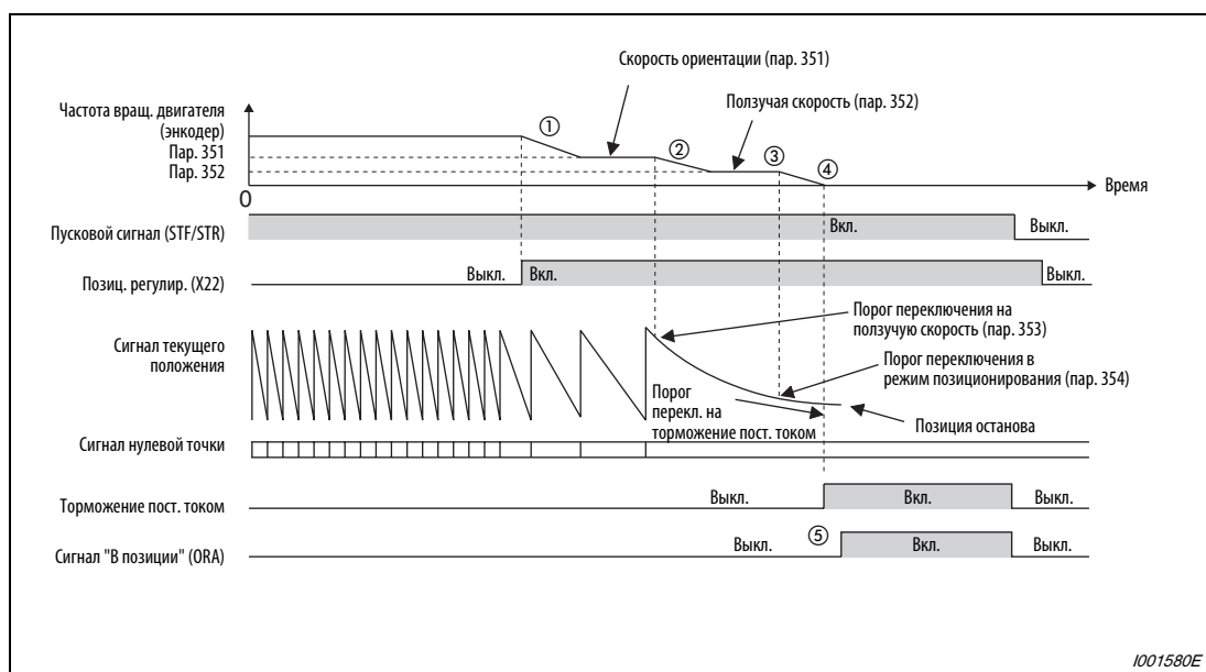
Рис. 6-116: Диаграмма переключения сигналов при запуске ориентации во время работы
