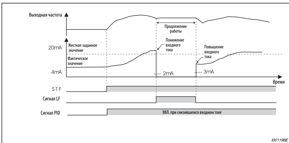
Рис. 6-198: Потеря токового заданного значения при ПИД-регулировании (реверсное вращение, пар. 573 = 1)
