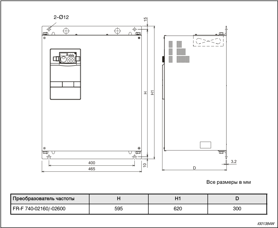
Рис. А-6: Размеры FR-A 740-02160 и FR-A 740-02600
