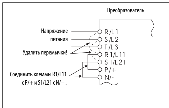
Рис. 6-163: Подключение
