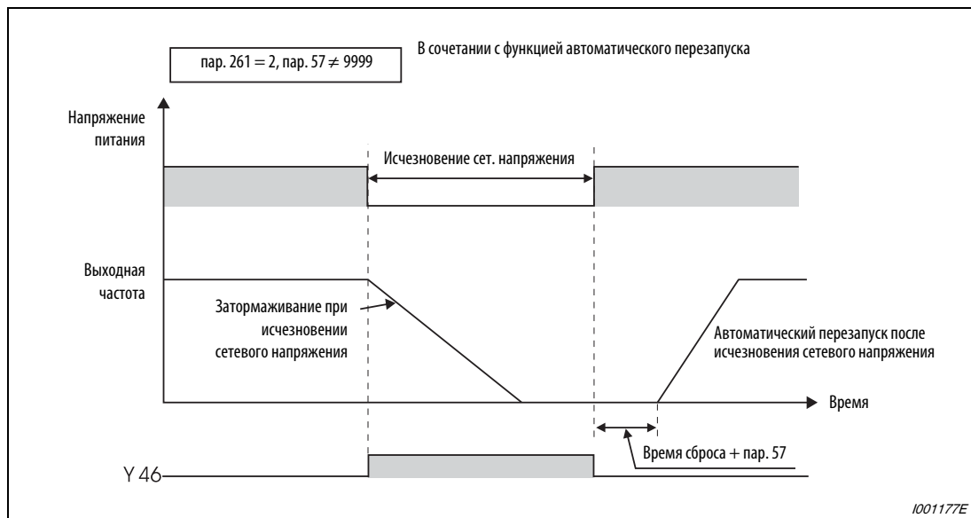
Рис. 6-168: Продолжение работы после исчезновения сетевого напряжения
