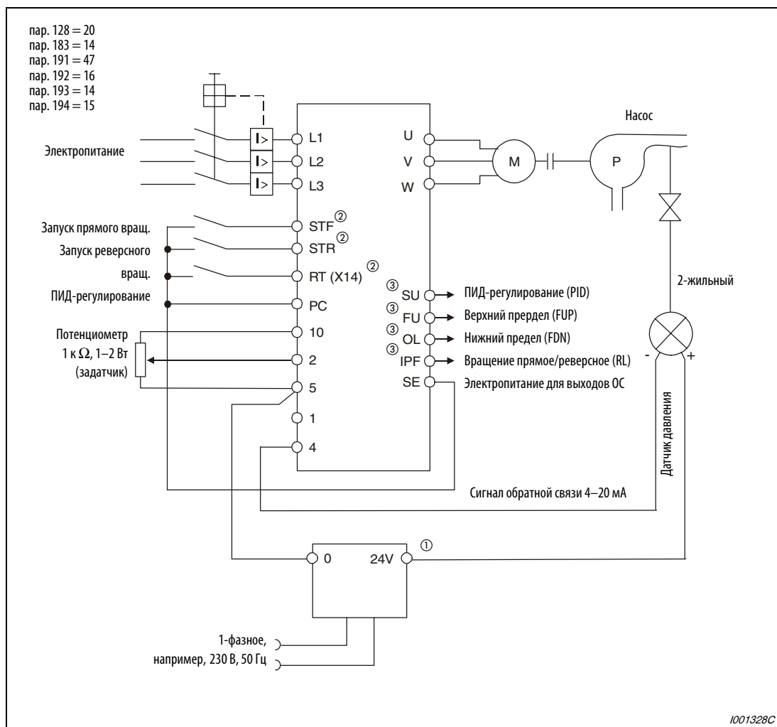
Рис. 6-242: Пример подключения при положительной логике
