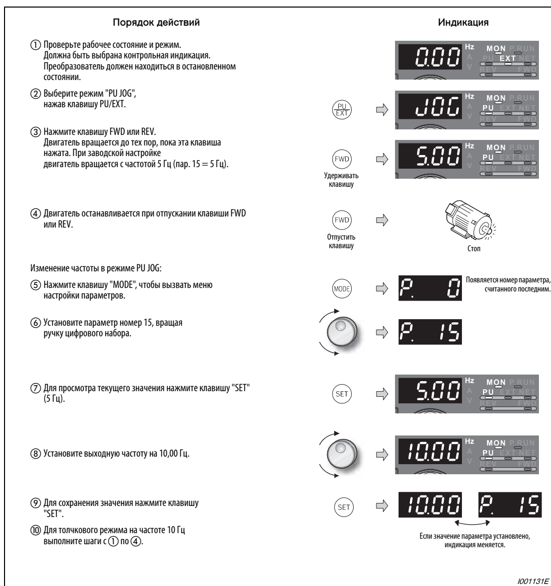
Рис. 6-72: Толчковое включение с помощью панели управления
