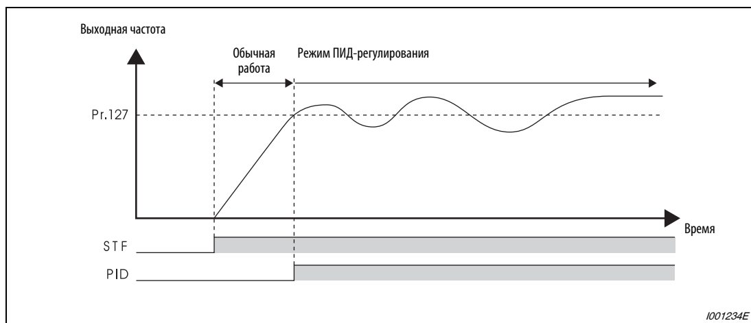
Рис. 6-243: Автоматическое переключение в режим ПИД-регулирования
