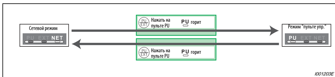
Рис. 6-204: Переключение режима при пар. 340 = 10 или 12
