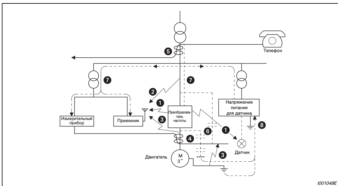
Рис. 3-48: Пути распространения помех
