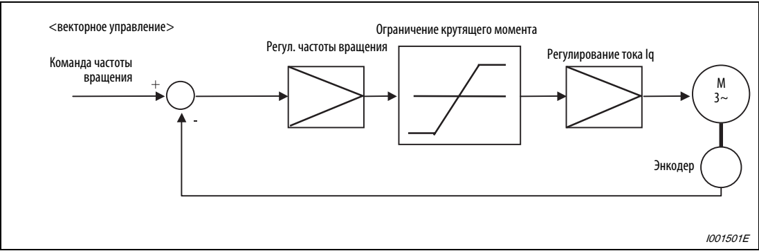
Рис. 6-7: Блок-схема ограничения крутящего момента
