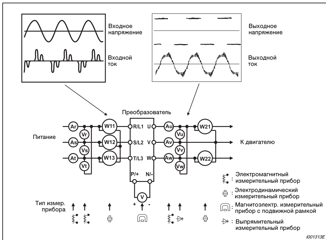
Рис. 8-15: Измерения на силовой части
