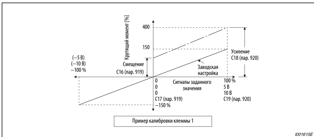
Рис. 6-191: Настройка сигнала на клемме 1
