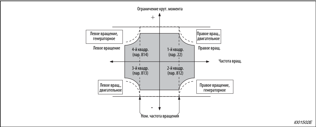
Рис. 6-8: Задание ограничения крутящего момента с помощью параметра
