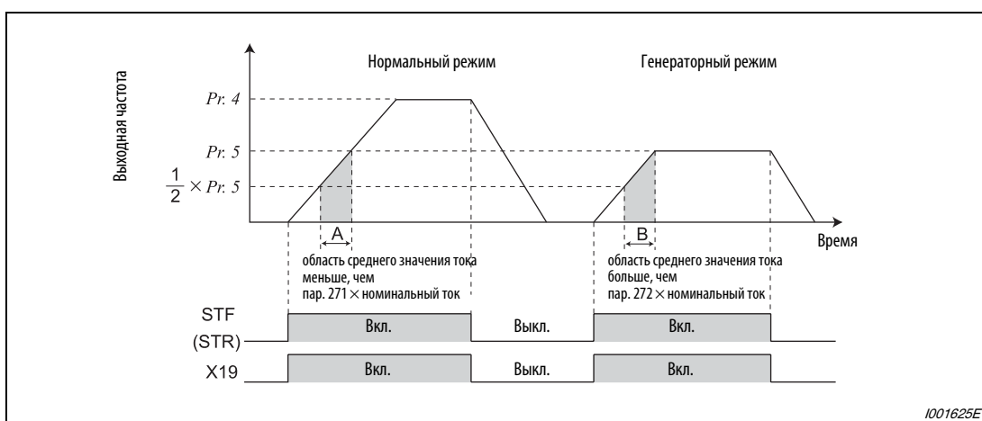
Рис. 6-255: Частота вращения в зависимости от среднего значения тока
