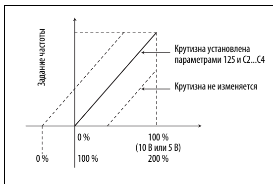
Рис. 6-185: Настройка смещения
