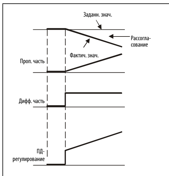
Рис. 6-238: Принцип действия ПД-регулятора
