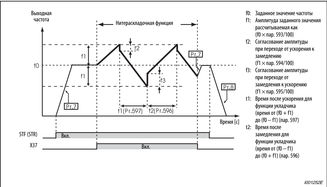
Рис. 6-261: Функция укладчика
