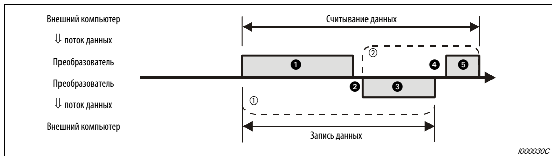
Рис. 6-221: Схематическое изображение обмена данными
