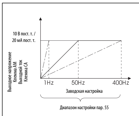
Рис. 6-148: Опорная величина для внешней индикации частоты
