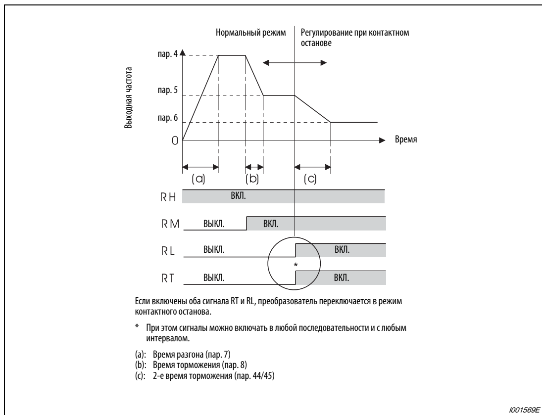
Рис. 6-109: Переключение на контактный останов
