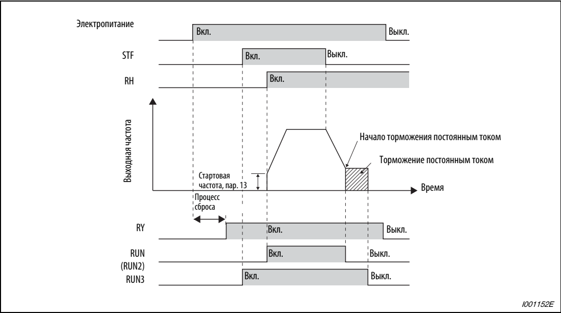
Рис. 6-131: Готовность к работе и вращение двигателя
