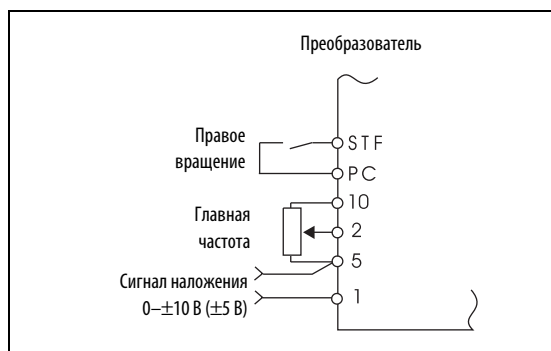
Рис. 6-180: Пример схемы для арифметического наложения
