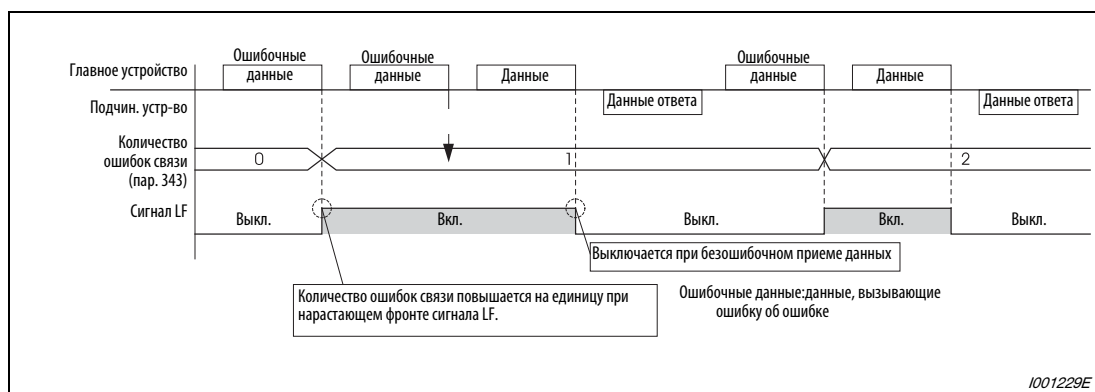
Рис. 6-232: Вывод сигнала LF
