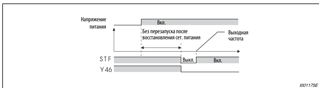
Рис. 6-166: Повторный запуск при восстановлении электропитания
