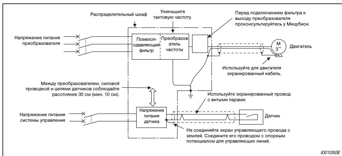
Рис. 3-49: Примеры подавления помех
