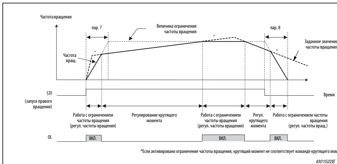
Рис. 6-36: Переходная характеристика
