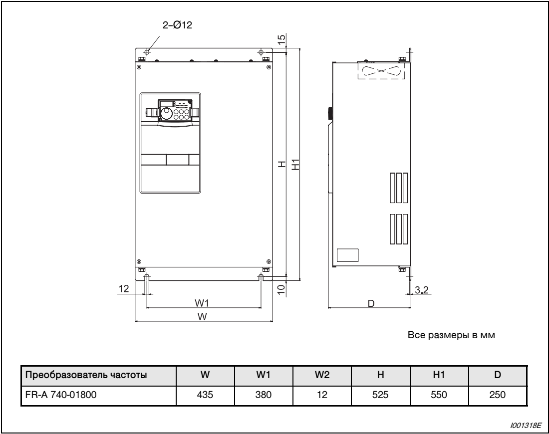
Рис. А-5: Размеры FR-A 740-01800
