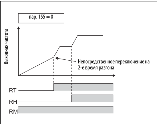
Рис. 6-126: Пример переключения времени разгона/торможения
