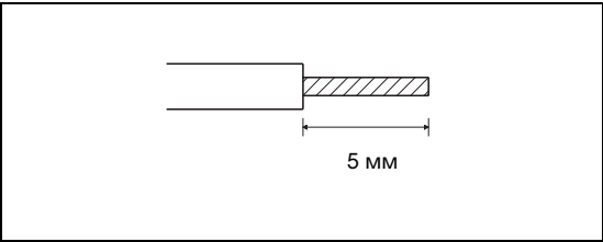
Рис. 3-18: Подготовка кабеля
