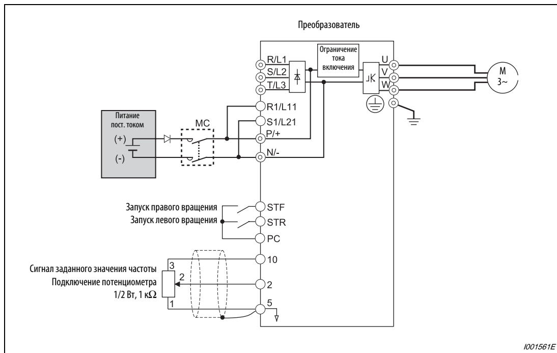
Рис. 6-99: Пример подключения для варианта 1 питания контура постоянного тока
