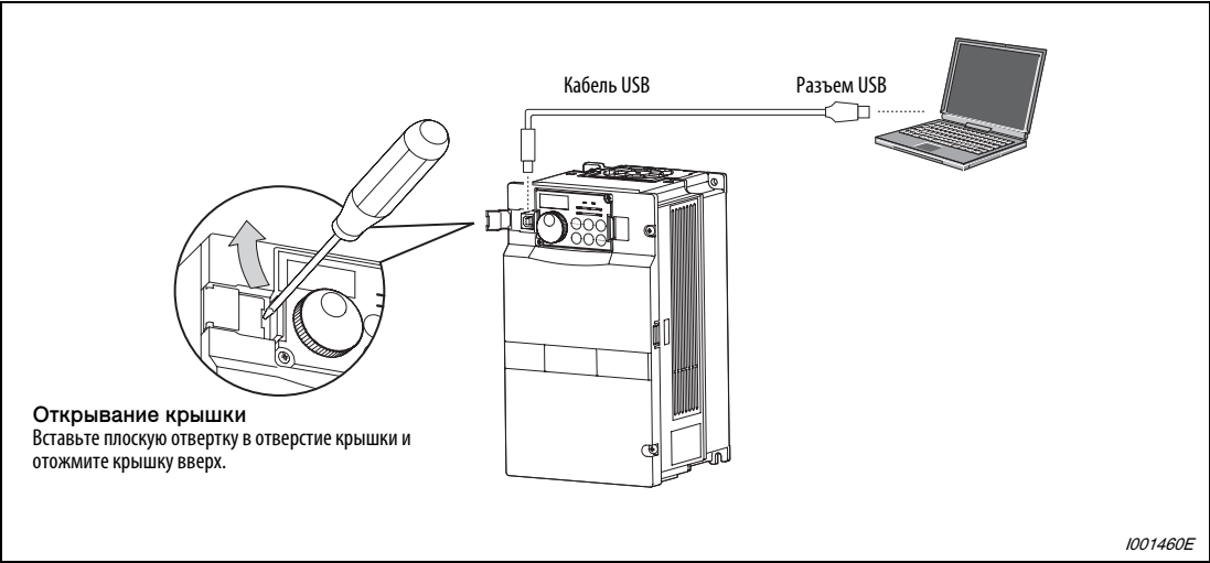
Рис. 6-234: Подключение к интерфейсу USB
