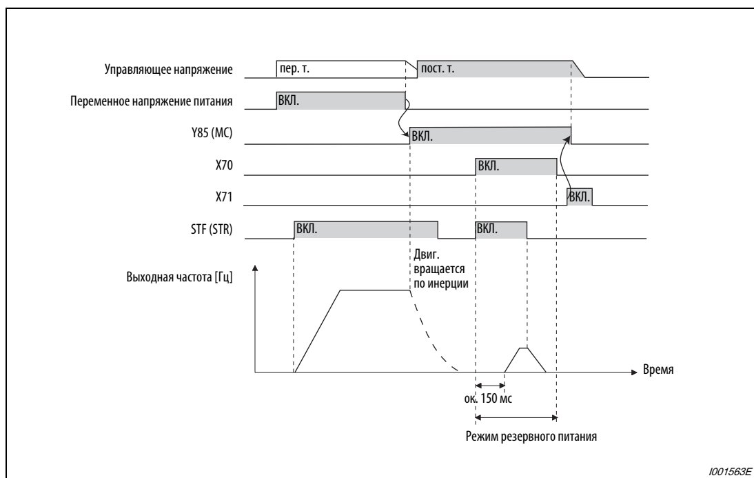
Рис. 6-101: Пример 1 работы при исчезновении сетевого напряжения
