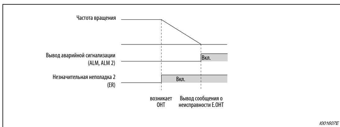
Рис. 6-172: Вывод аварийной сигнализации (пар. 875 = 1)
