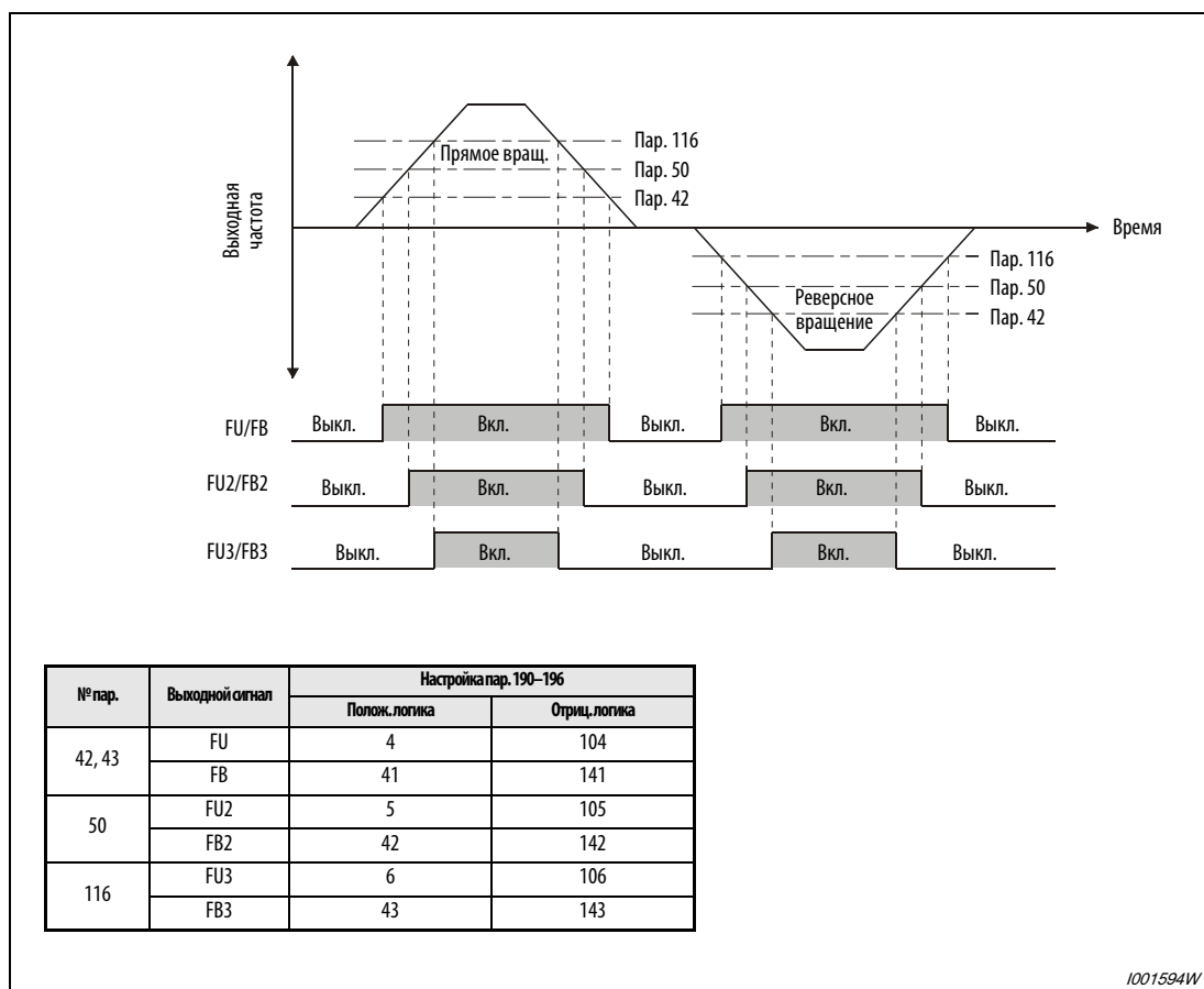
Рис. 6-137: Контроль частоты при прямом и реверсном вращении
