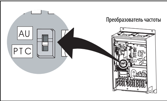
Рис. 6-93: Переключатель AU/PTC
