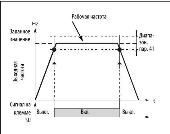
Рис. 6-136: Диаграмма срабатывания выходного сигнала на клемме SU
