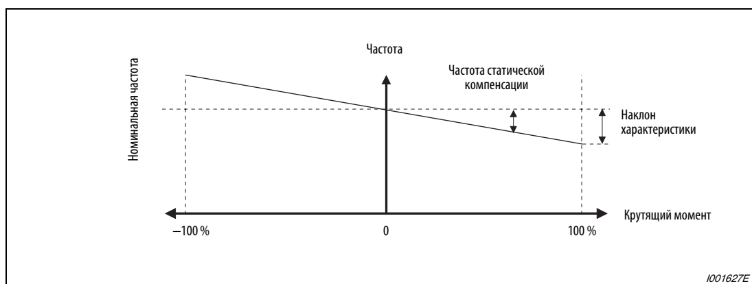
Рис. 6-257: Функция управления жесткостью механической характеристики
