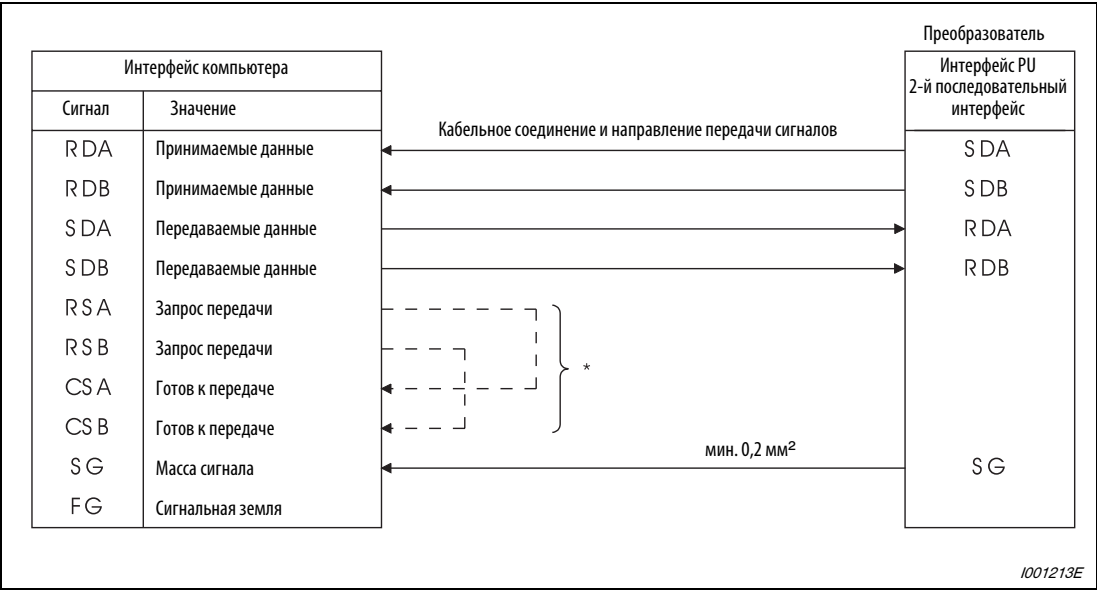
Рис. 6-213: Соединение с преобразователем частоты
