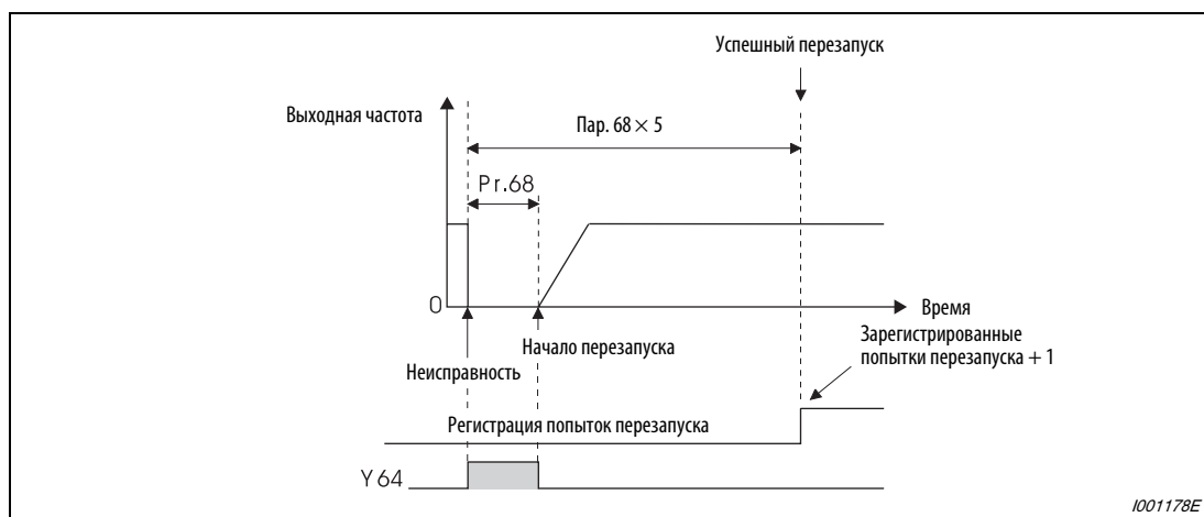
Рис. 6-169: Пример успешно выполненного перезапуска
