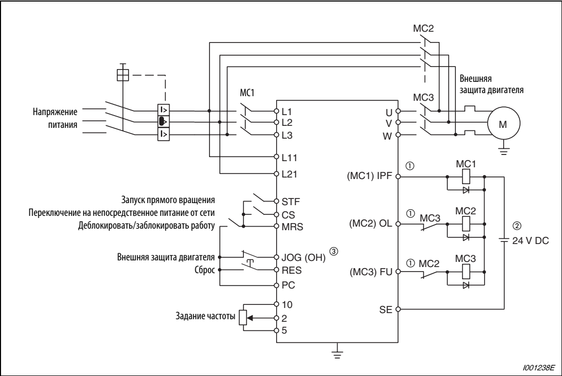
Рис. 6-248: Подключение силовых контакторов
