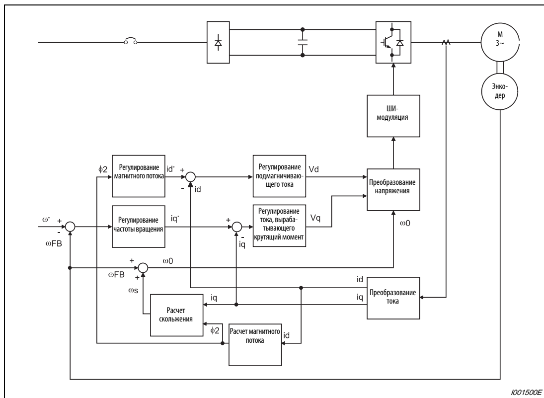
Рис. 6-4: Блок-схема векторного управления
