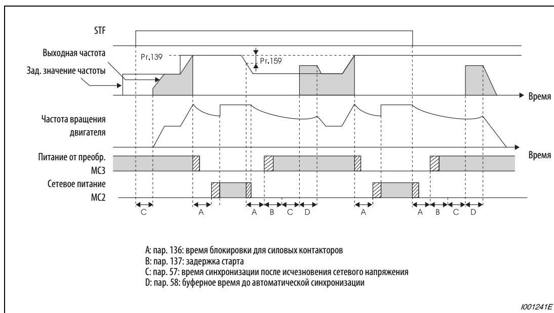
Рис. 6-251: Временная диаграмма сигналов с автоматическим переключением на сетевое питание
