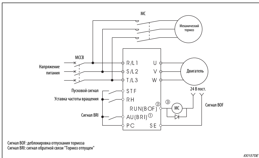
Рис. 6-110: Пример схемы с механическим тормозом (пар. 184 = 15, пар. 190 = 20)
