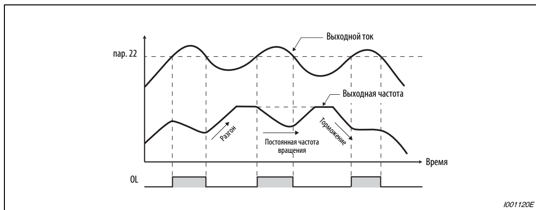
Рис. 6-48: Принцип работы ограничения тока
