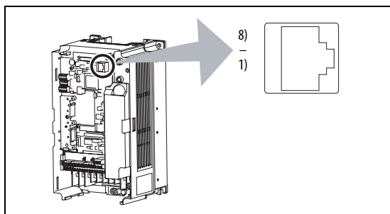
Рис. 6-209: Разводка клемм разъема пульта управления (интерфейса PU)
