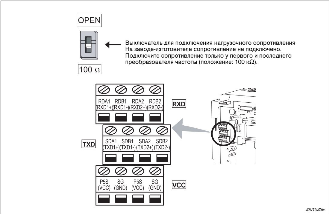
Рис. 3-23: 2-й последовательный интерфейс преобразователя частоты
