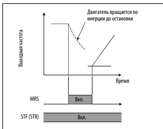
Рис. 6-123: Блокировка регулятора
