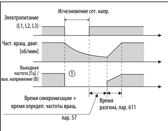
Рис. 6-158: Бессенсорное векторное управление
