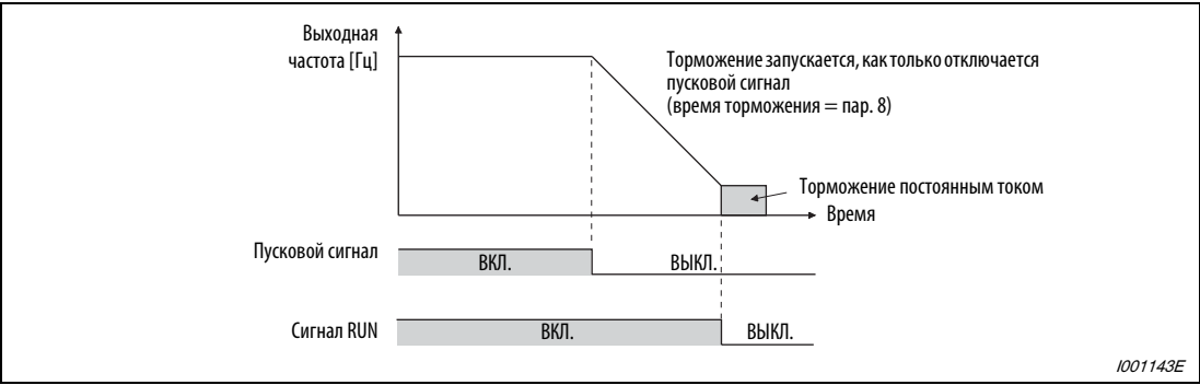
Рис. 6-105: Метод останова, если параметр 250 = 8888 или 9999
