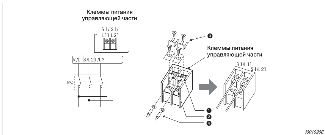
Рис. 3-11: Детализированный вид клемм
