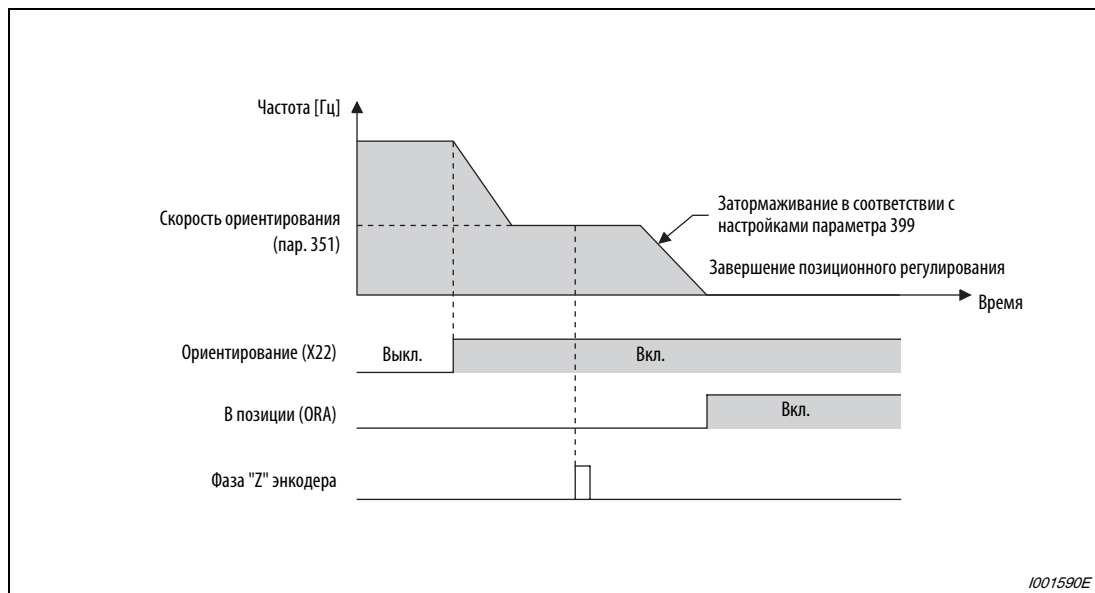
Рис. 6-122: Скорость в режиме ориентирования
