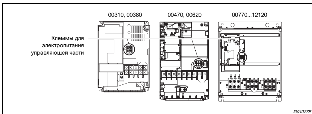
Рис. 3-12: Расположение клемм
