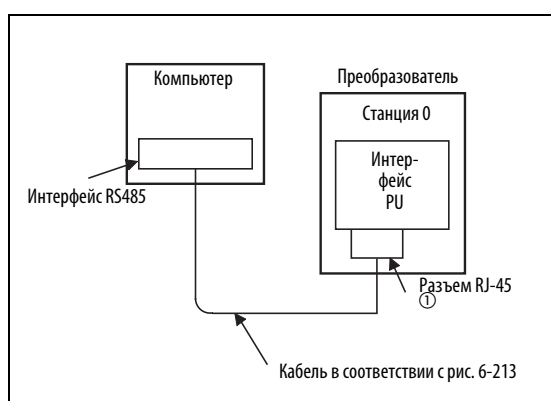
Рис. 6-211: Подключение персонального компьютера с интерфейсом RS485 к интерфейсу PU
