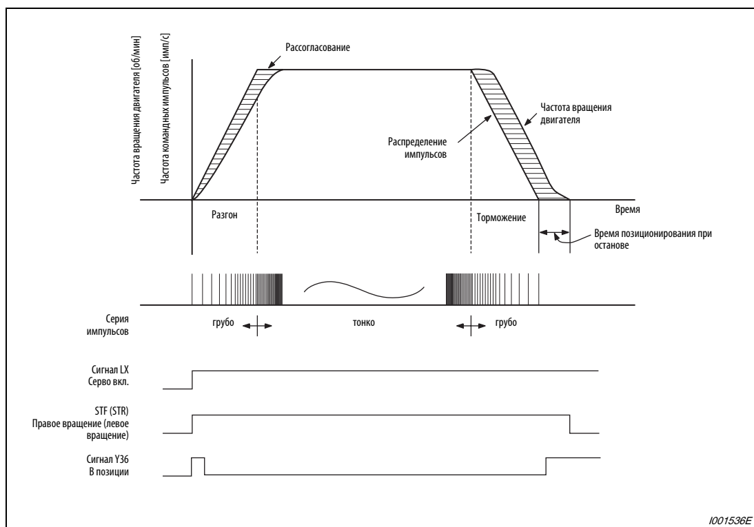
Рис. 6-39: Позиционирование
