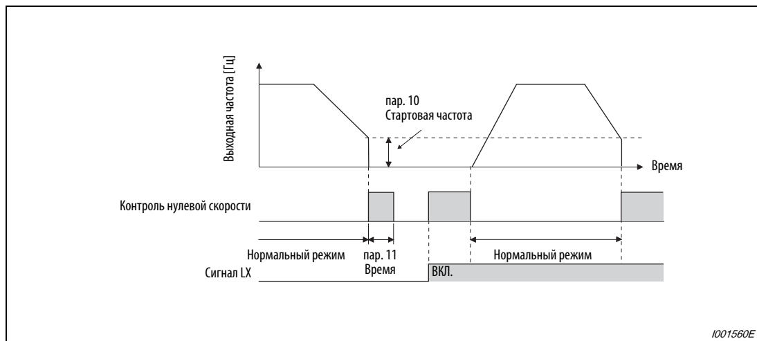
Рис. 6-98: Выбор предварительного возбуждения с помощью внешнего сигнала
