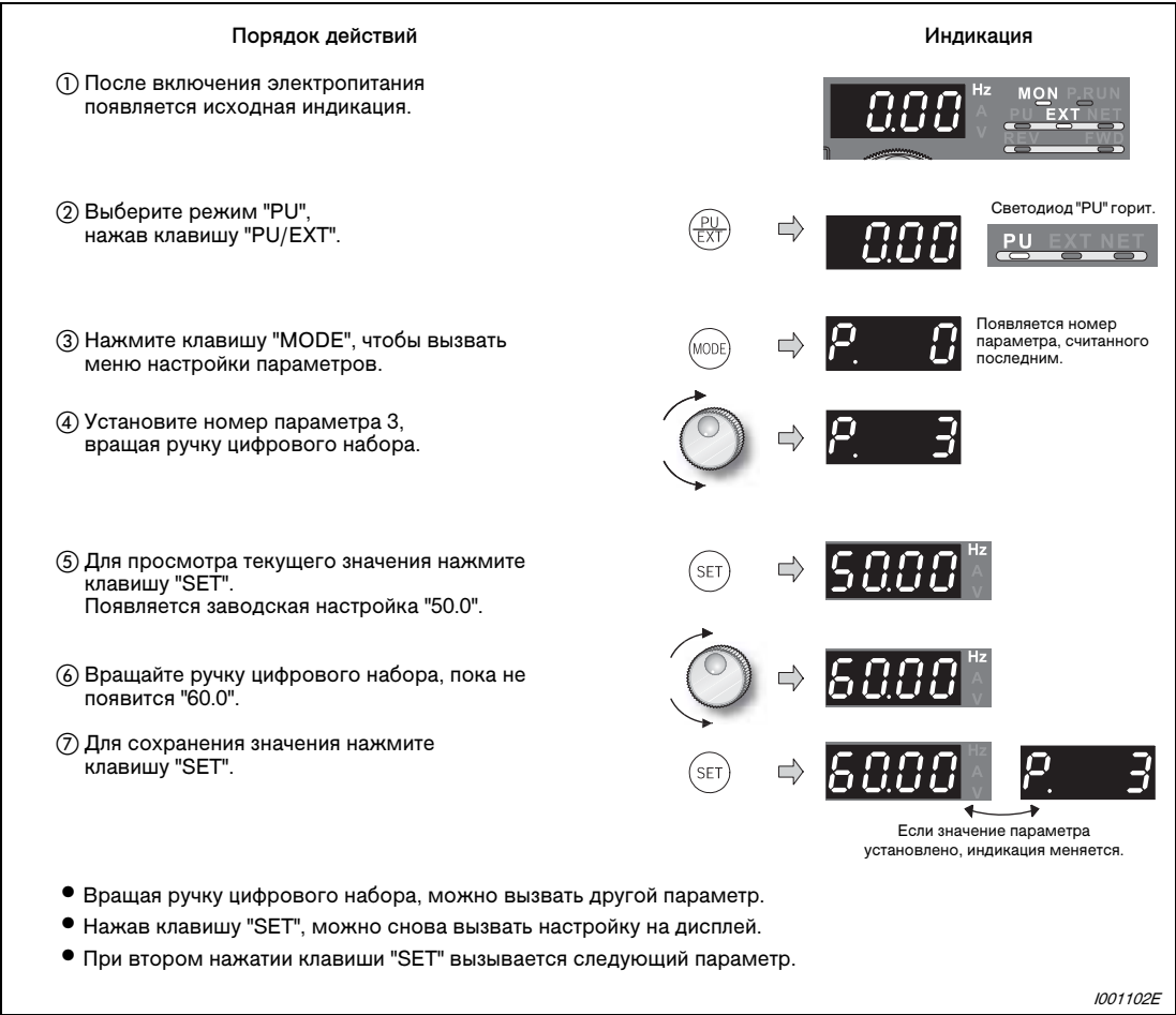
Рис. 5-2: Настройка базовой частоты
