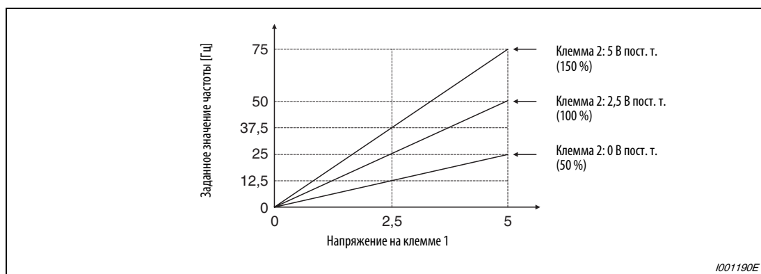
Рис. 6-184: Заданное значение частоты в зависимости от сигнала на клемме 1 и клемме 2
