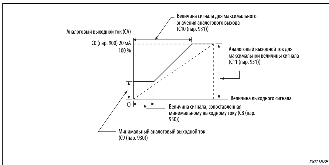
Рис. 6-152: Калибровка выхода СА
