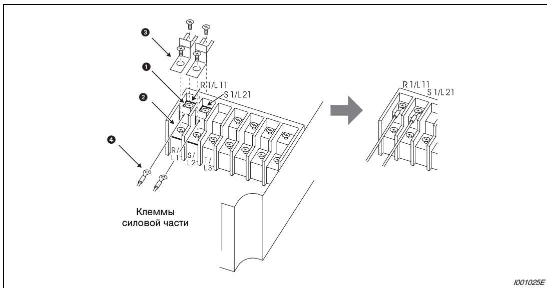
Рис. 3-10: Детализированный вид клемм
