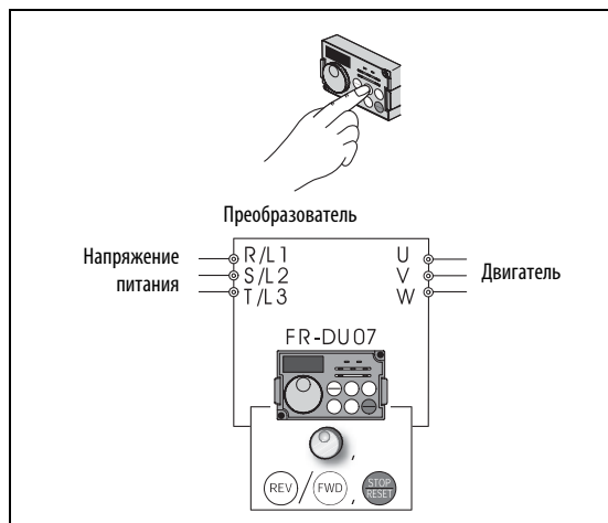
Рис. 6-206: Пульты управления
