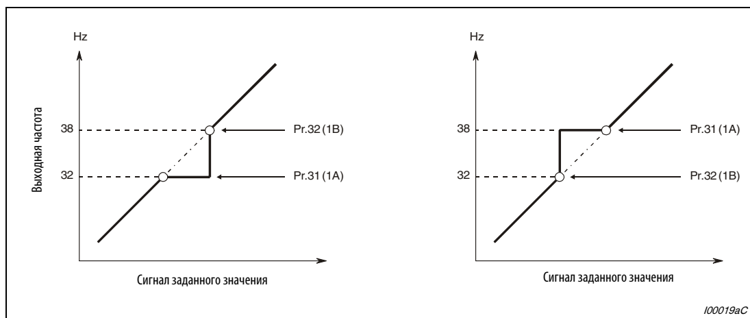
Рис. 6-58: Выбор точки скачка
