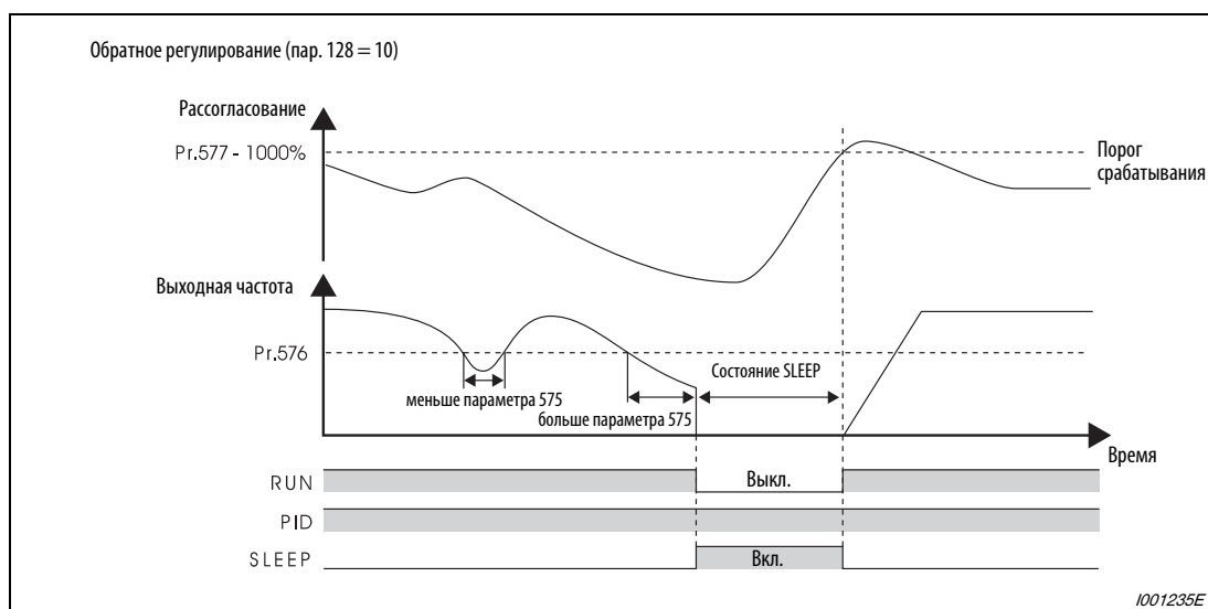
Рис. 6-244: Отключение выхода (функция SLEEP)
