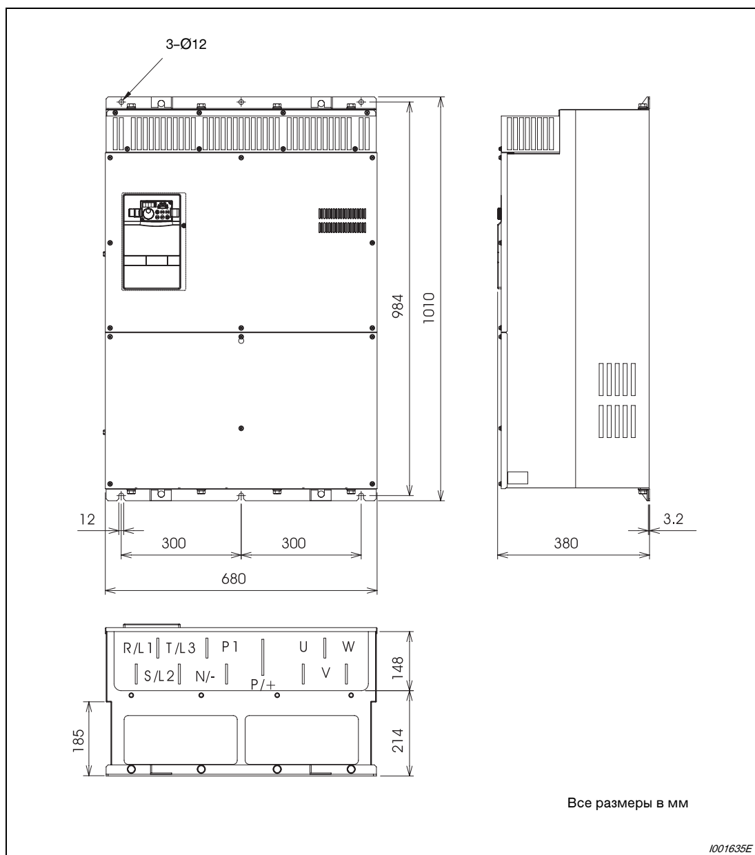
Рис. А-9: Размеры FR-A 740-05470, FR-A 740-006100 и FR-A 740-06830
