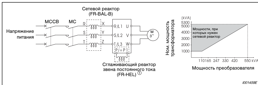
Рис. 3-44: Подключение сетевого реактора
