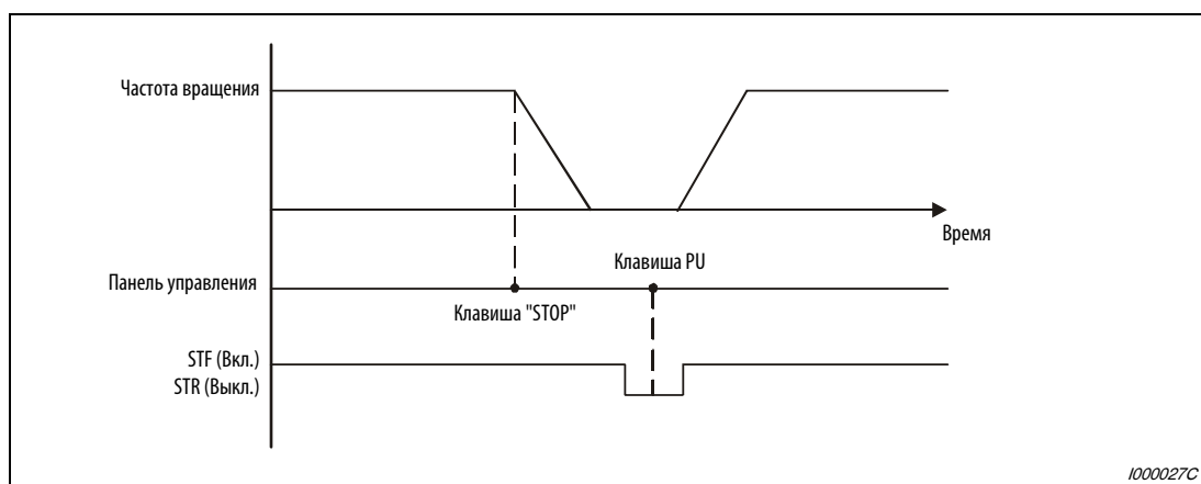
Рис. 6-199: Останов во время внешнего режима управления
