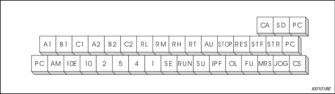
Рис. 3-17: Обзор разводки клемм
