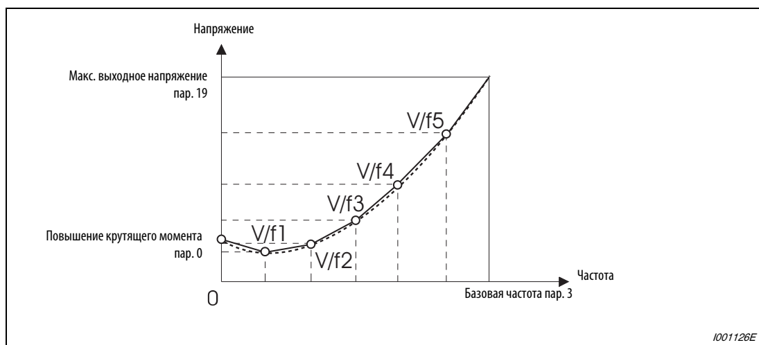
Рис. 6-64: Характеристика U/f
