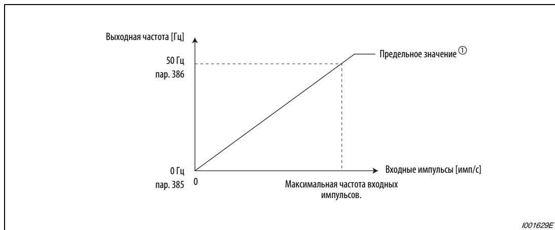
Рис. 6-259: Калибровка импульсного входа
