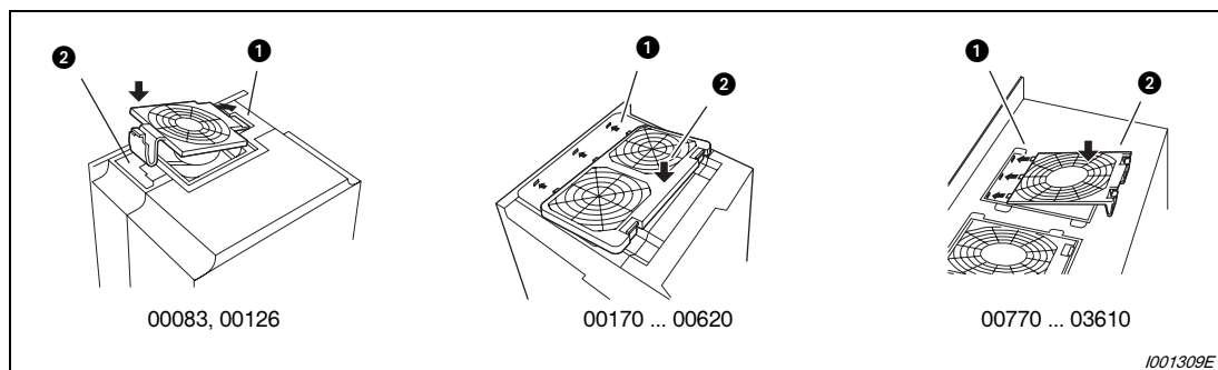
Рис. 8-8: Монтаж кожуха вентилятора
