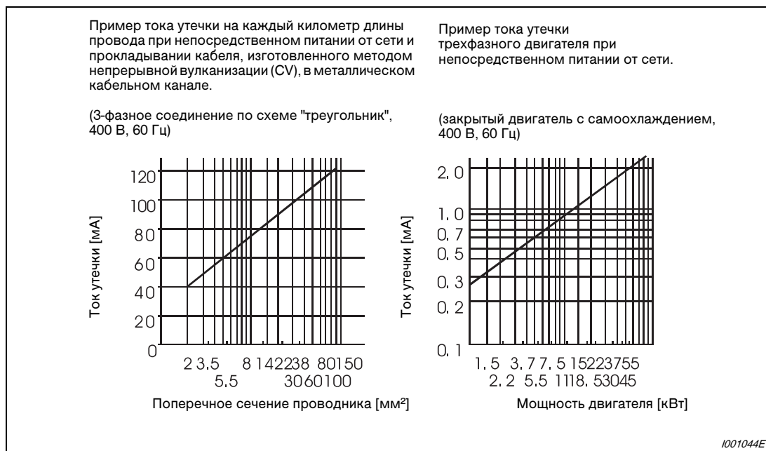
Рис. 3-46: Токи утечки
