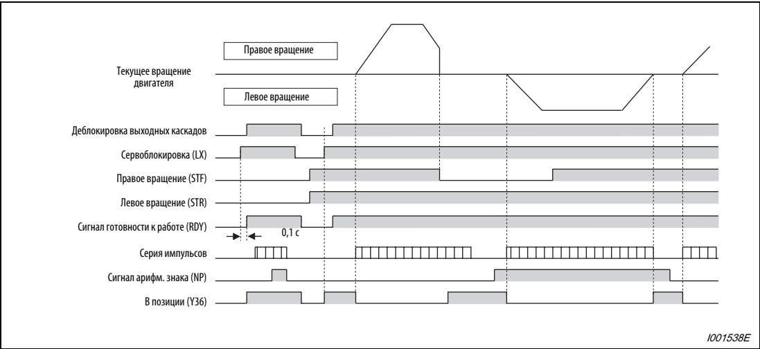
Рис. 6-41: Работа
