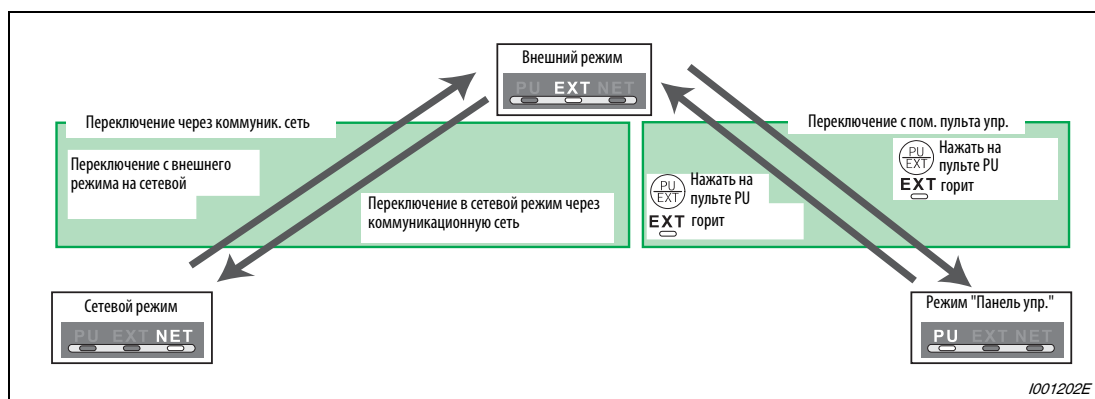
Рис. 6-203: Переключение режима при пар. 340 = 0, 1 или 2
