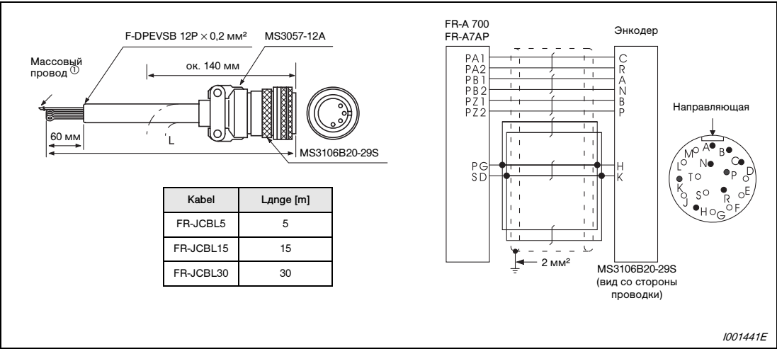
Рис. 3-29: Двигатель SF-JR с энкодером
