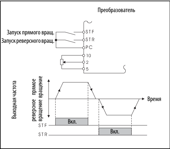
Рис. 6-127: Управление с помощью 2-проводной схемы управления (пар. 250 = 9999)
