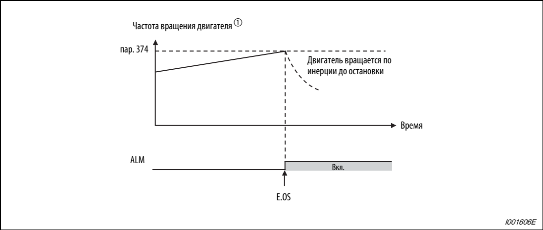
Рис. 6-171: Предел частоты вращения и вывод тревожной сигнализации
