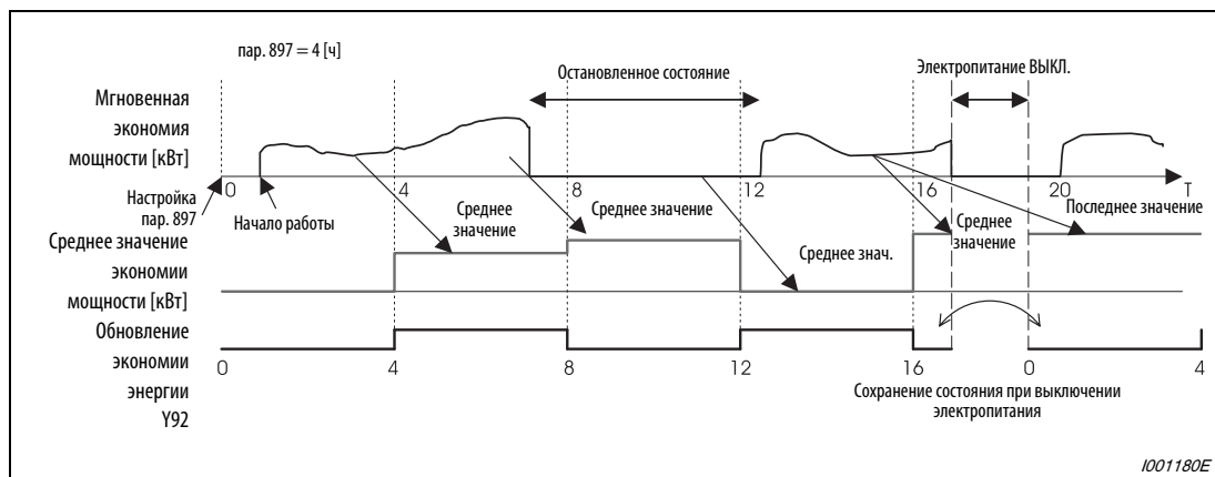
Рис. 6-173: Обновление экономии энергии
