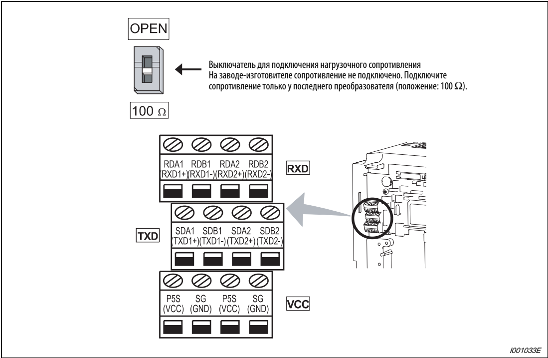
Рис. 6-214: 2-й последовательный интерфейс преобразователя
