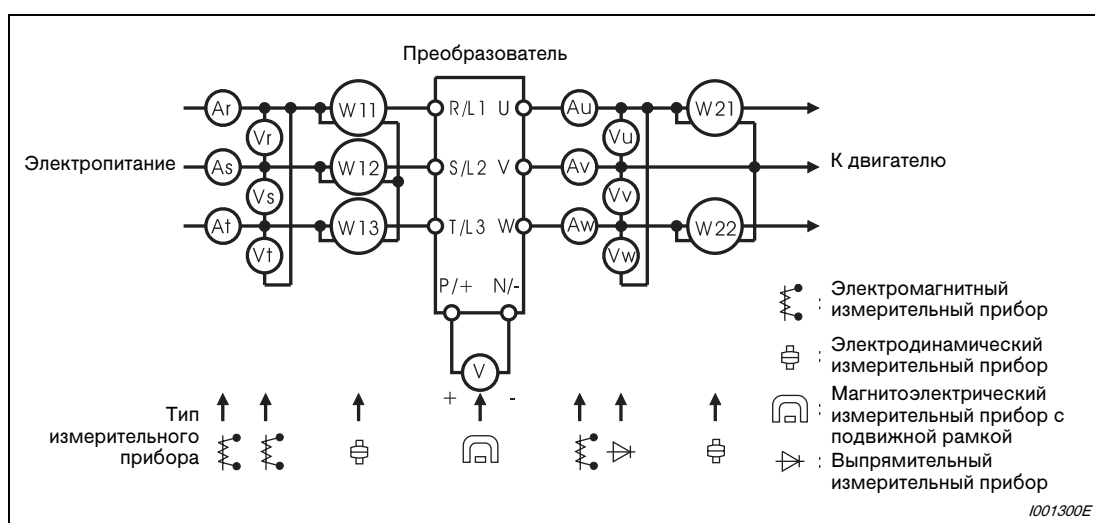
Рис. 7-7: Измерения на силовой части
