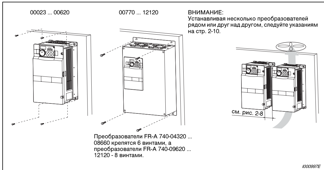
Рис. 2-6: Установка на монтажной панели распределительного шкафа
