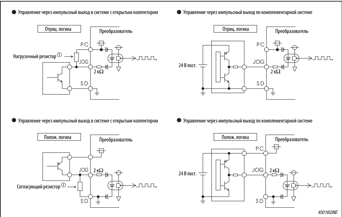
Рис. 6-258: Импульсный вход
