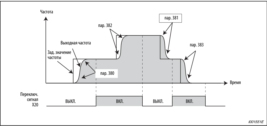
Рис. 6-84: Характеристика, если параметр 29 = "4"
