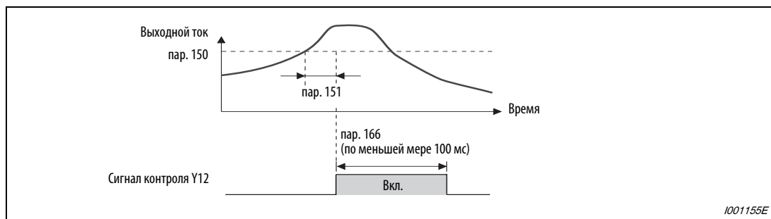
Рис. 6-138: Контроль выходного тока (пар. 166 ≠ 9999, 167 = 0)
