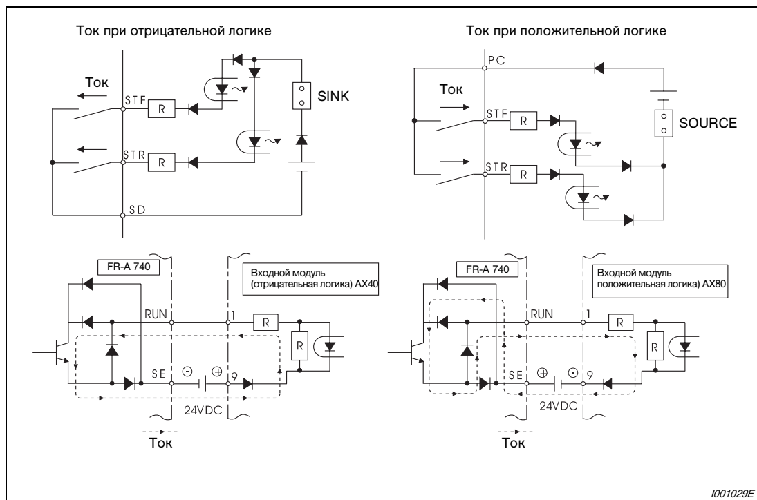
Рис. 3-14: Выбор управляющей логики
