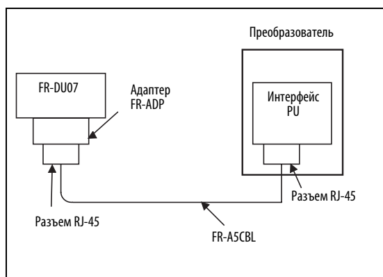
Рис. 6-210: Подключение пульта управления к интерфейсу PU
