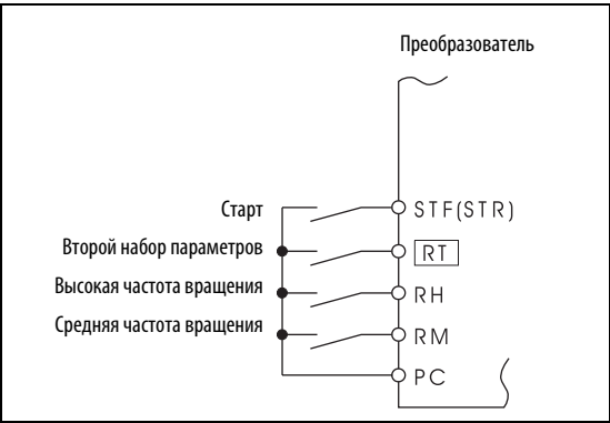
Рис. 6-125: Пример схемы для выбора второго набора параметров
