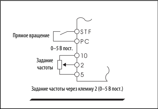
Рис. 6-176: Задание частоты в виде постоянного напряжения 0–5 В
