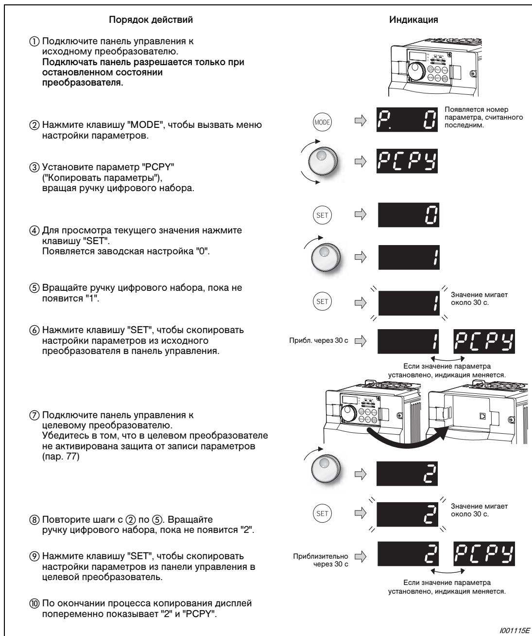
Рис. 4-11: Копирование параметров
