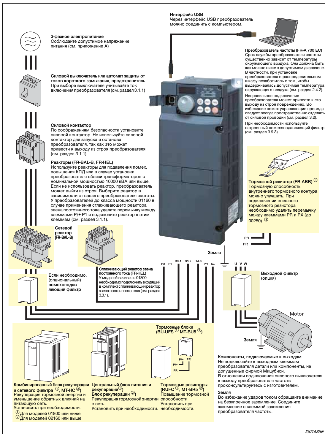
Рис. 3-1: Обзор конфигурации системы
