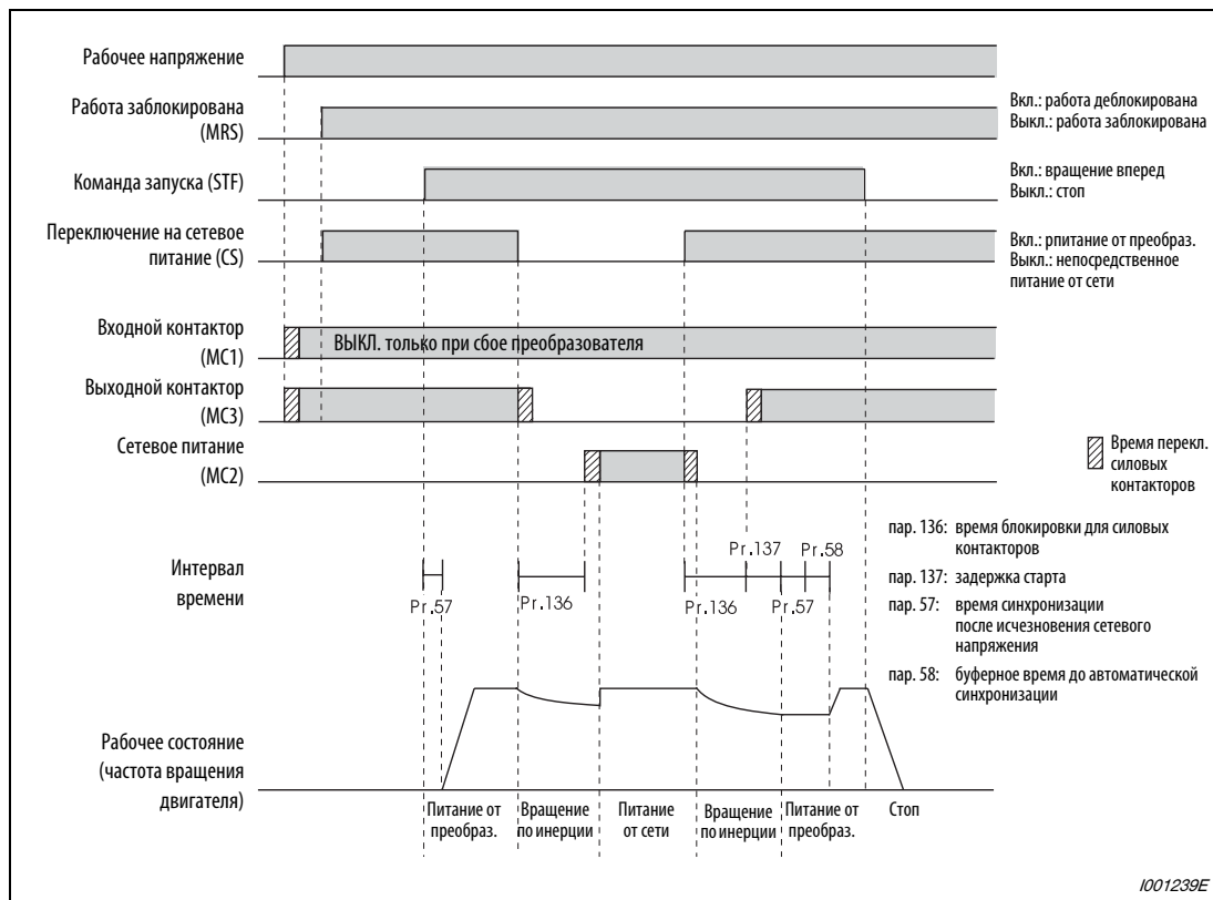
Рис. 6-249: Временная диаграмма сигналов без автоматического переключения на сетевое питание
