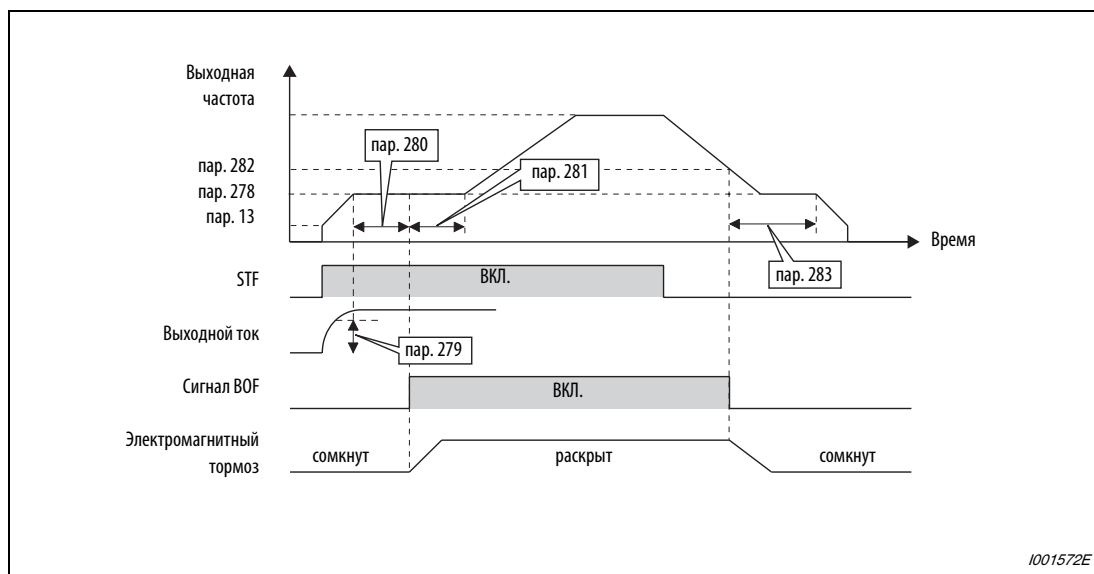
Рис. 6-112: Работа с параметром 292 = 8
