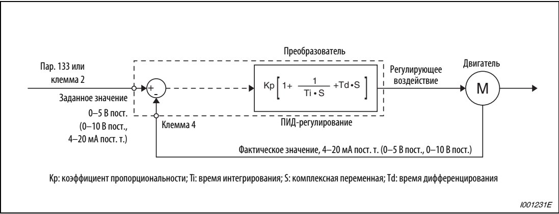
Рис. 6-236: Конфигурация системы для пар. 128 = 20 или 21 (подключение задания/сигнала обратной связи к преобразователю)
