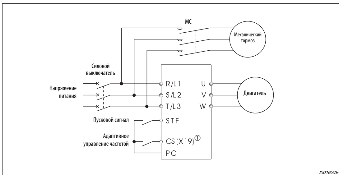
Рис. 6-254: Пример подключения для положительной логики (пар. 186 = 19)
