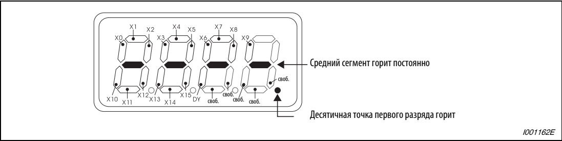
Рис. 6-146: Индикация при установленной опции FR-A7AX
