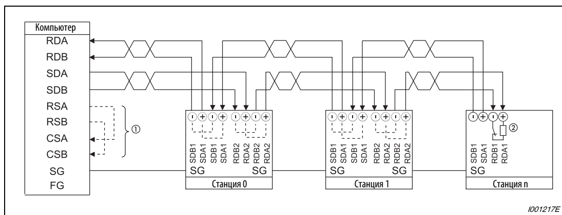
Рис. 6-219: Соединение с несколькими преобразователями частоты
