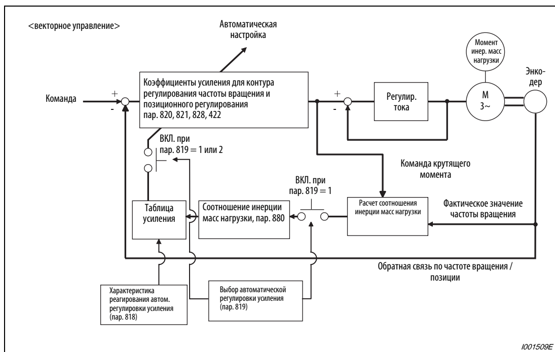
Рис. 6-15: Блок-схема автоматической настройки усиления
