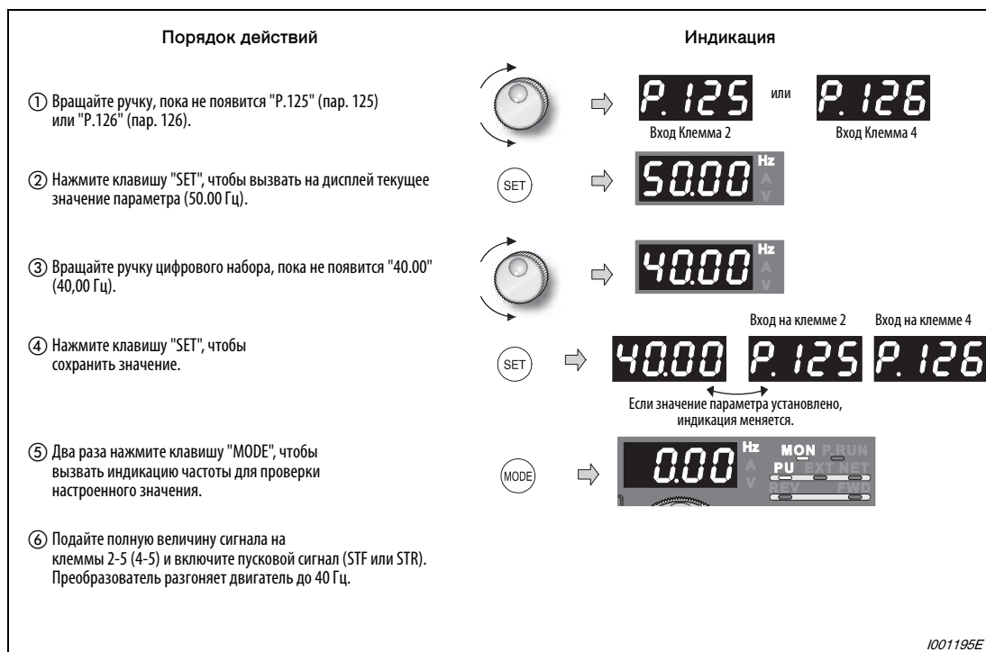
Рис. 6-190: Настройка частоты без изменения настроек входного сигнала напряжения (тока)
