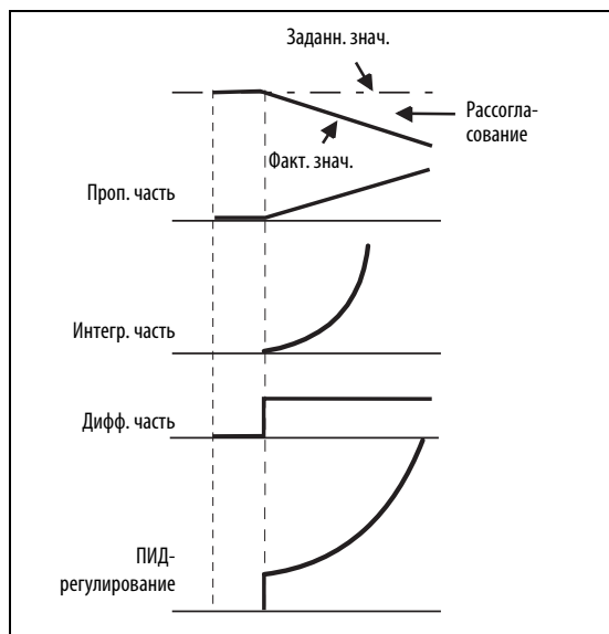
Рис. 6-239: Принцип действия ПИД-регулятора
