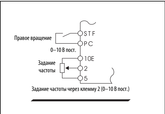
Рис. 6-177: Задание частоты в виде постоянного напряжения 0–10 В
