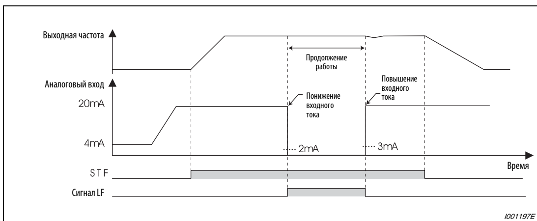
Рис. 6-197: Потеря токового заданного значения во внешнем режиме управления (пар. 573 = 1)
