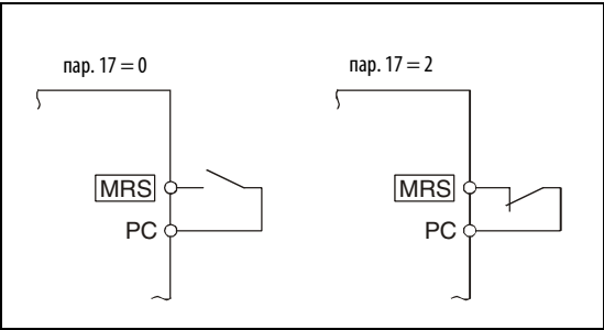
Рис. 6-124: Подключение клеммы MRS при положительной логике
