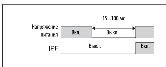
Рис. 6-155: Сигнал IPF
