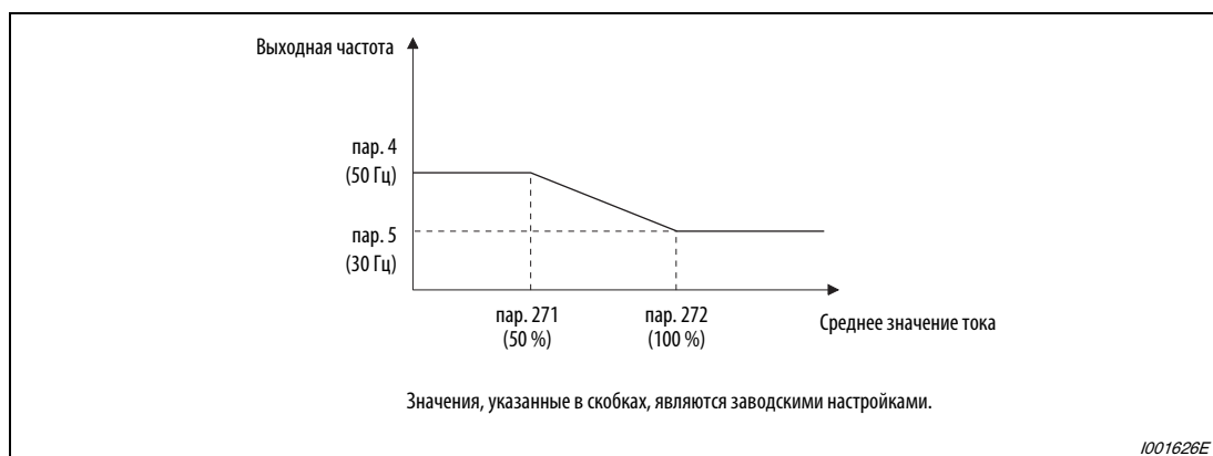
Рис. 6-256: Параметры 271 и 272
