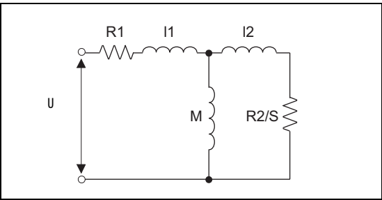
Рис. 6-94: Схема замещения электродвигателя
