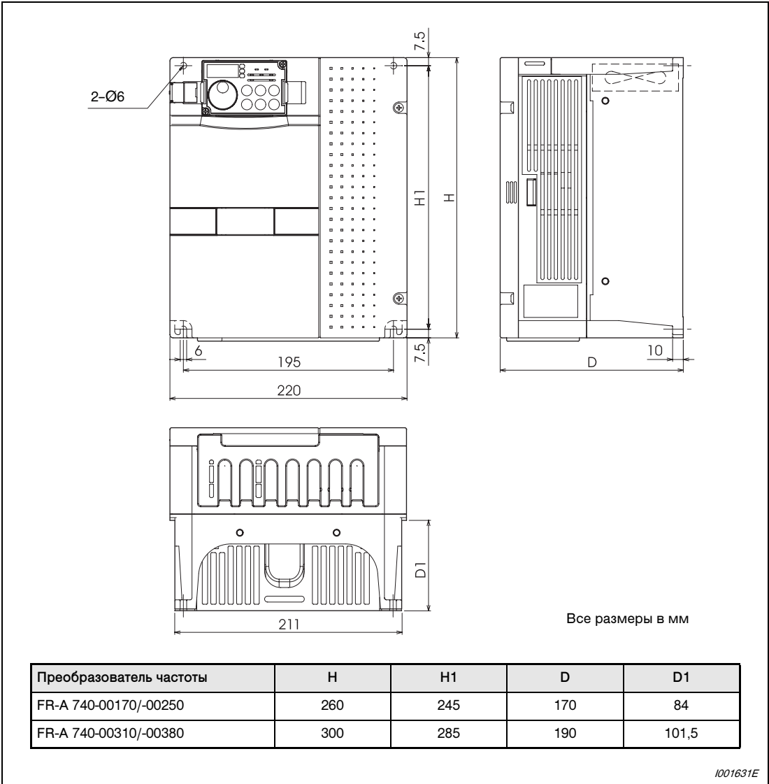
Рис. А-2: Размеры FR-A 740-00170 ... -00380
