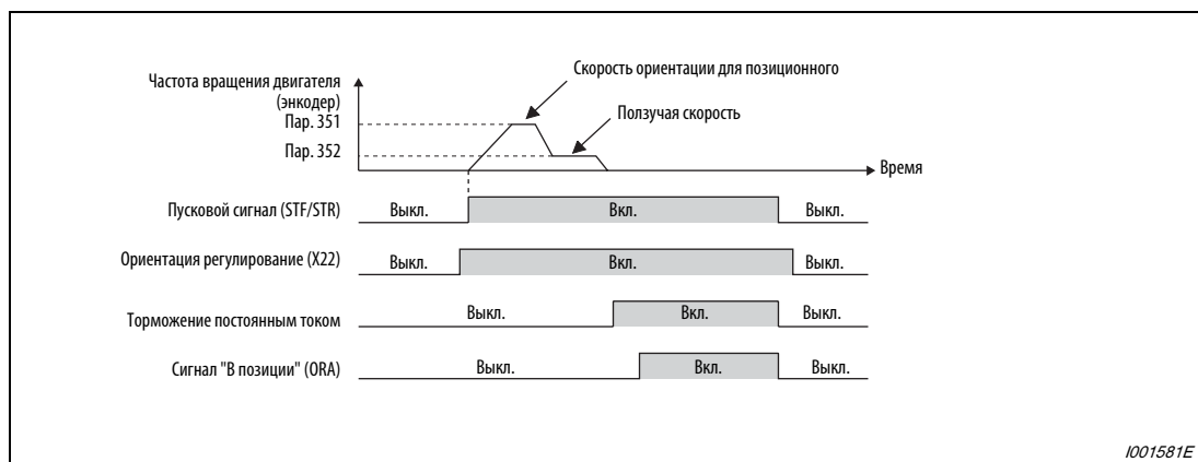
Рис. 6-117: Диаграмма переключения сигналов при запуске ориентирования из неподвижного состояния
