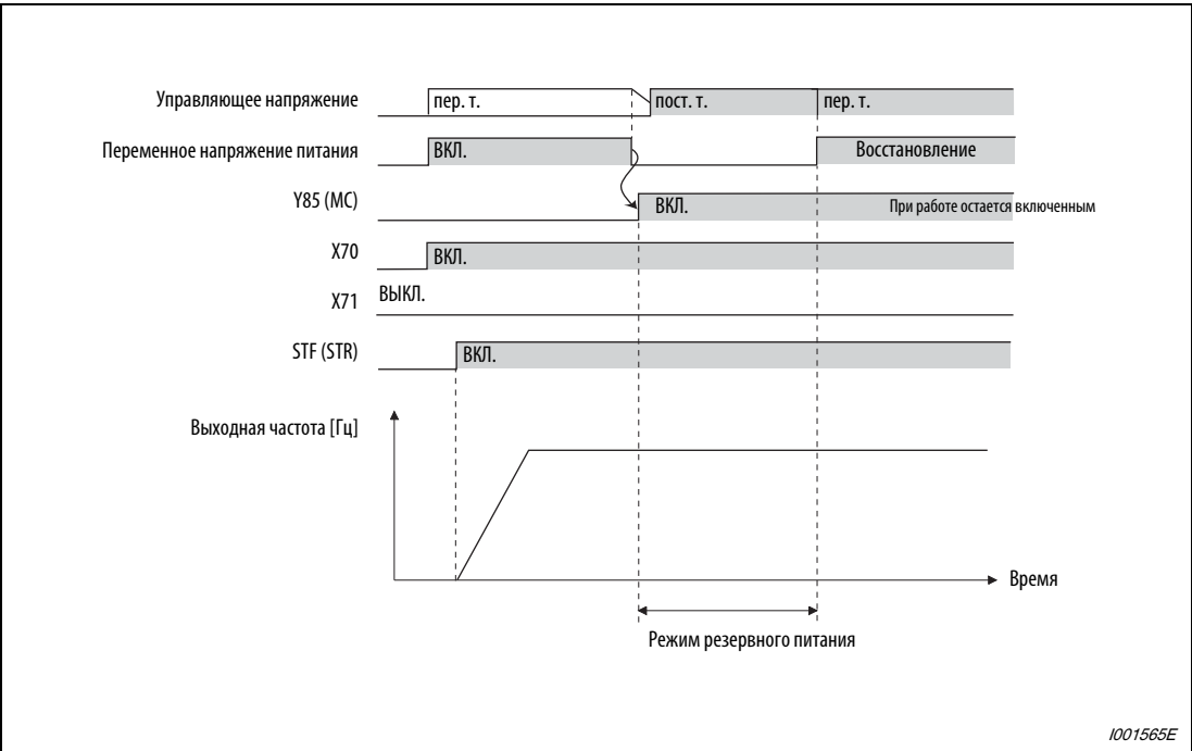
Рис. 6-103: Пример 3 работы при исчезновении сетевого напряжения (при непрерывной работе)
