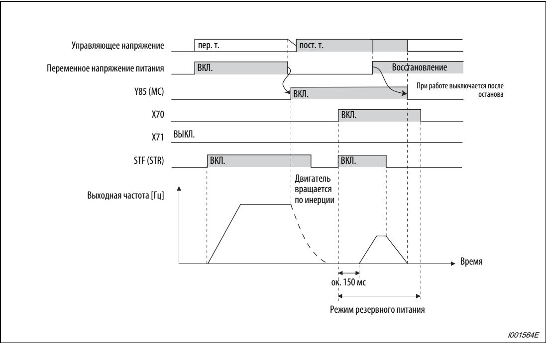
Рис. 6-102: Пример 2 работы при исчезновении сетевого напряжения (после восстановления напряжения питания)
