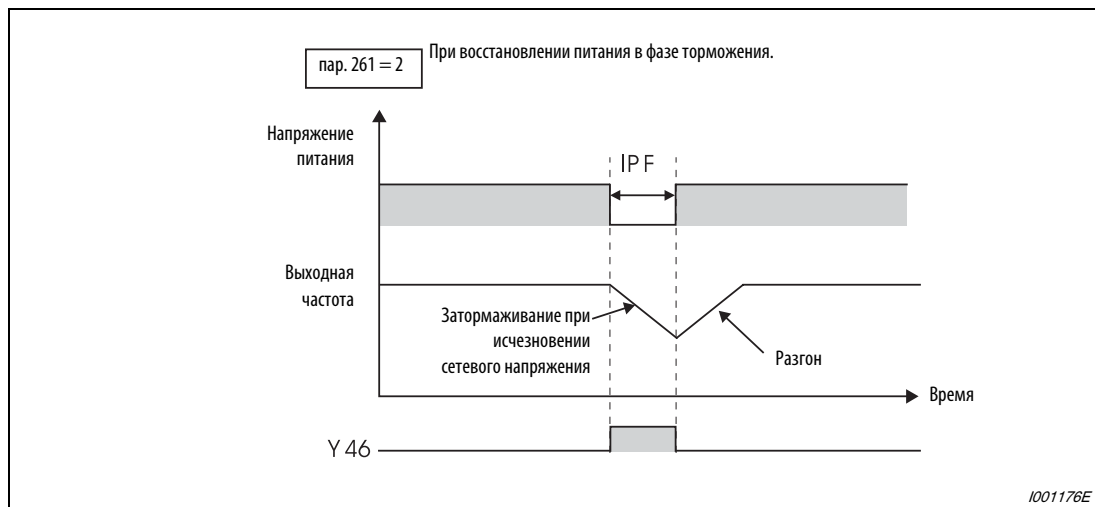
Рис. 6-167: Продолжение работы после исчезновения сетевого напряжения
