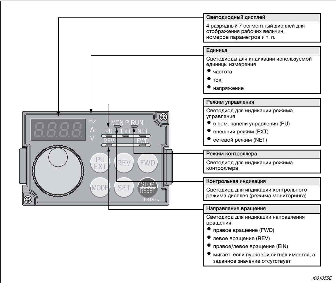
Рис. 4-3: Описание панели управления FR-DU07
