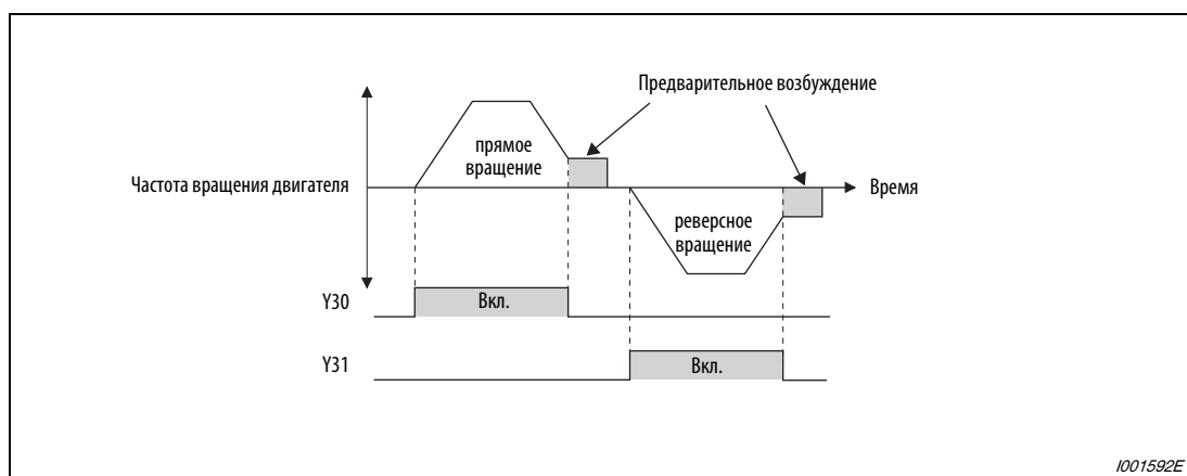
Рис. 6-133: Прямое и реверсное вращение двигателя
