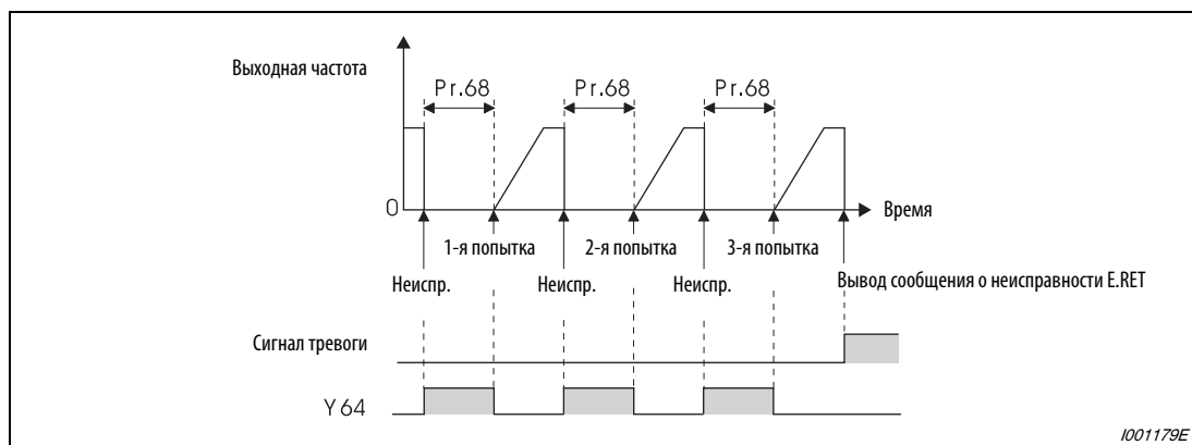
Рис. 6-170: Пример безуспешных попыток перезапуска
