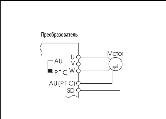
Рис. 6-92: Подключение датчика температуры с положительным температурным коэффициентом
