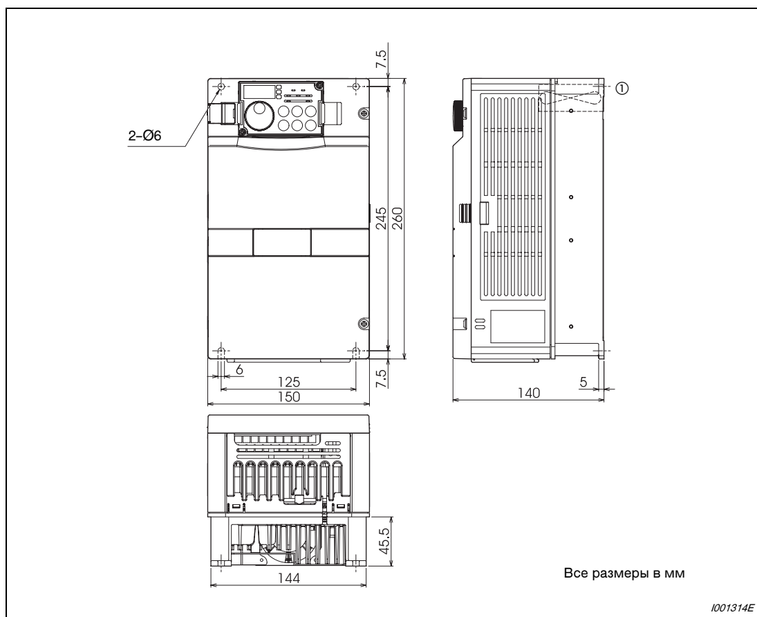
Рис. A-1: Размеры FR-A 740-00023 ... -00126
