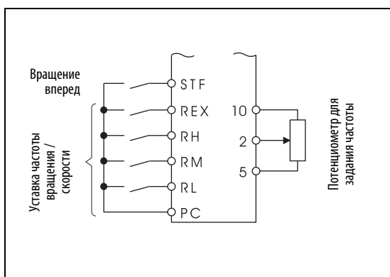
Рис. 6-67: Пример подключения
