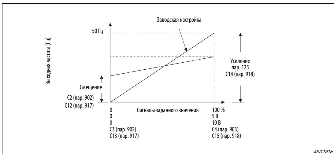
Рис. 6-186: Настройка сигнала на клеммах 1 и 2
