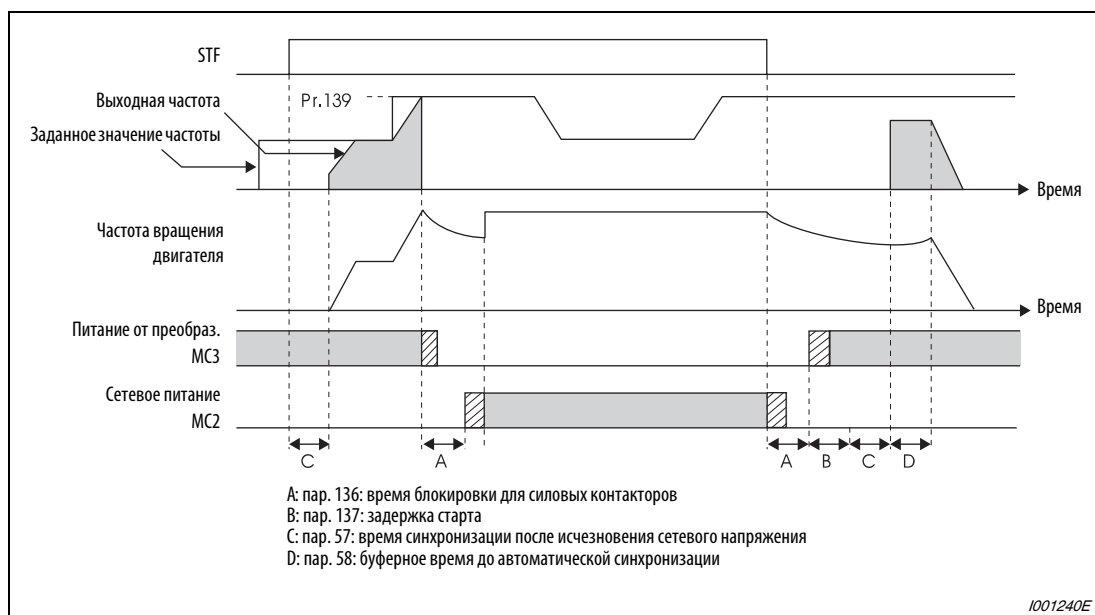
Рис. 6-250: Временная диаграмма сигналов с автоматическим переключением на сетевое питание
