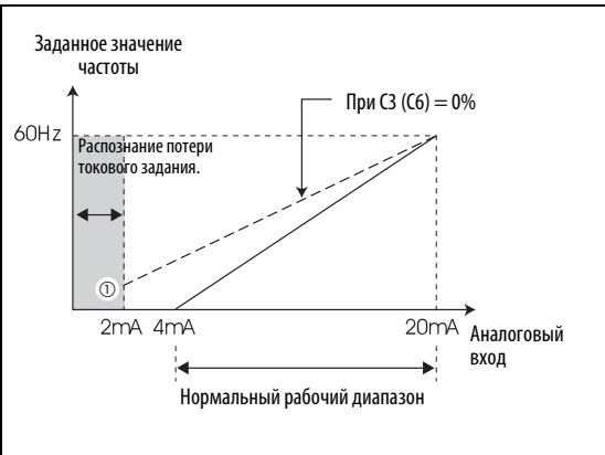
Рис. 6-196: Распознавание потери токового задания.
