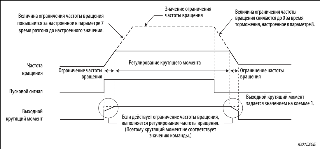
Рис. 6-34: Переходная характеристика
