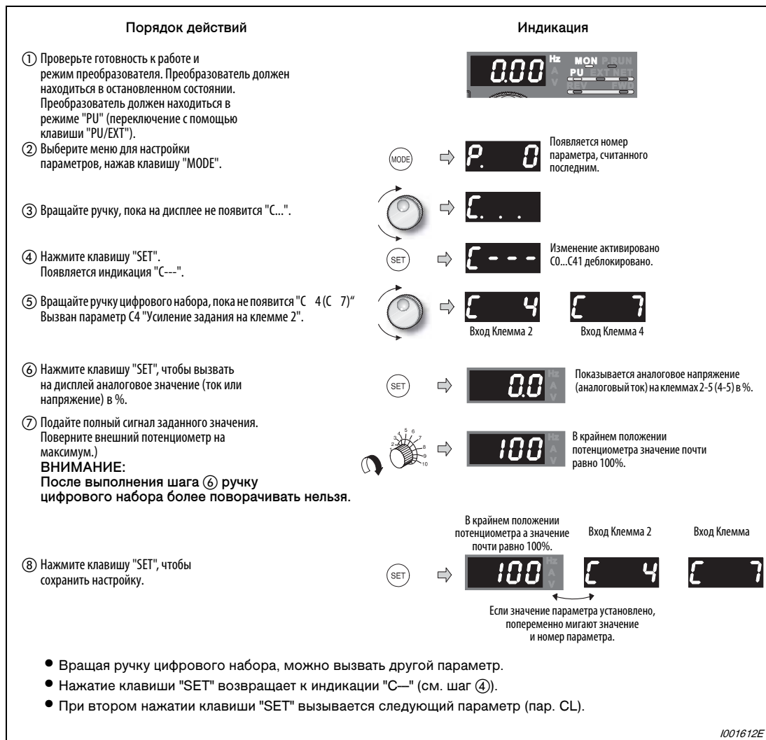
Рис. 6-188: Настройка смещения и усиления с подачей сигнала на клеммы
