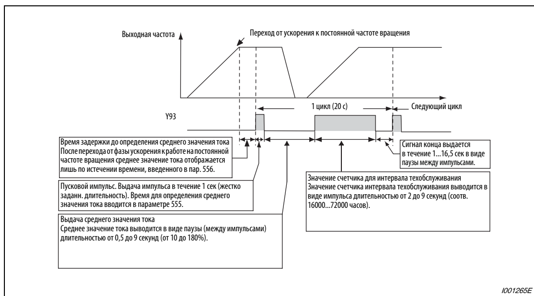
Рис. 6-268: Вывод импульсного сигнала Y93
