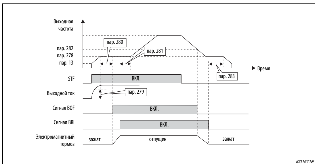
Рис. 6-111: Работа с параметром 292 = 7
