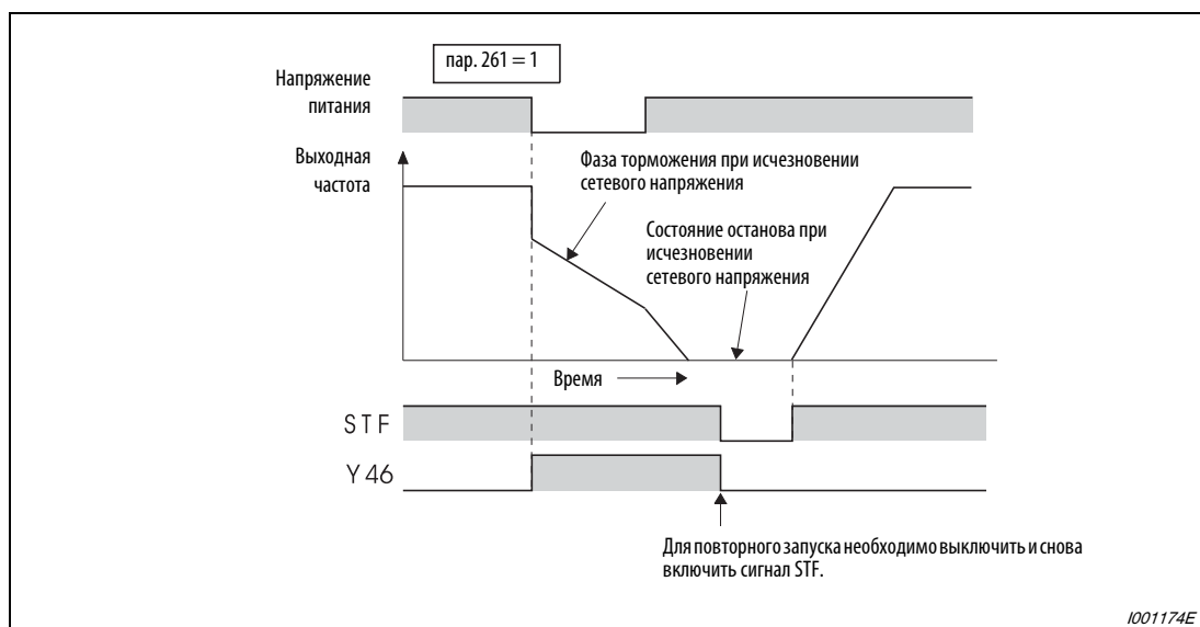
Рис. 6-165: Восстановление электропитания
