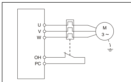
Рис. 6-91: Подключение внешней защиты двигателя
