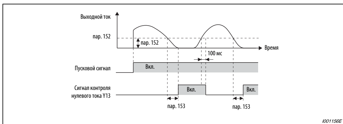
Рис. 6-139: Контроль нулевого тока
