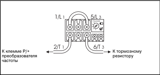
Рис. 3-34: Подключение термовыключателя
