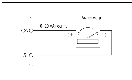
Рис. 6-151: Подключение аналогового измерительного прибора к выходу СА
