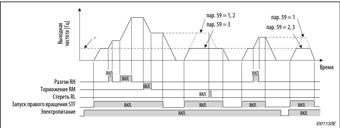
Рис. 6-74: Пример работы цифрового потенциометра
