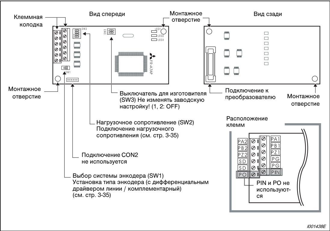
Рис. 3-26: Описание опционального блока FR-A7AP
