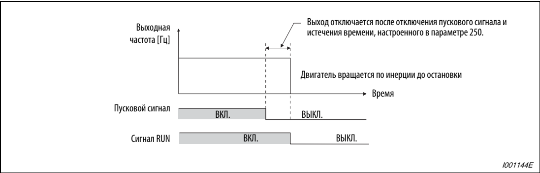
Рис. 6-106: Метод останова, если параметр 250 ≠ 8888 или 9999
