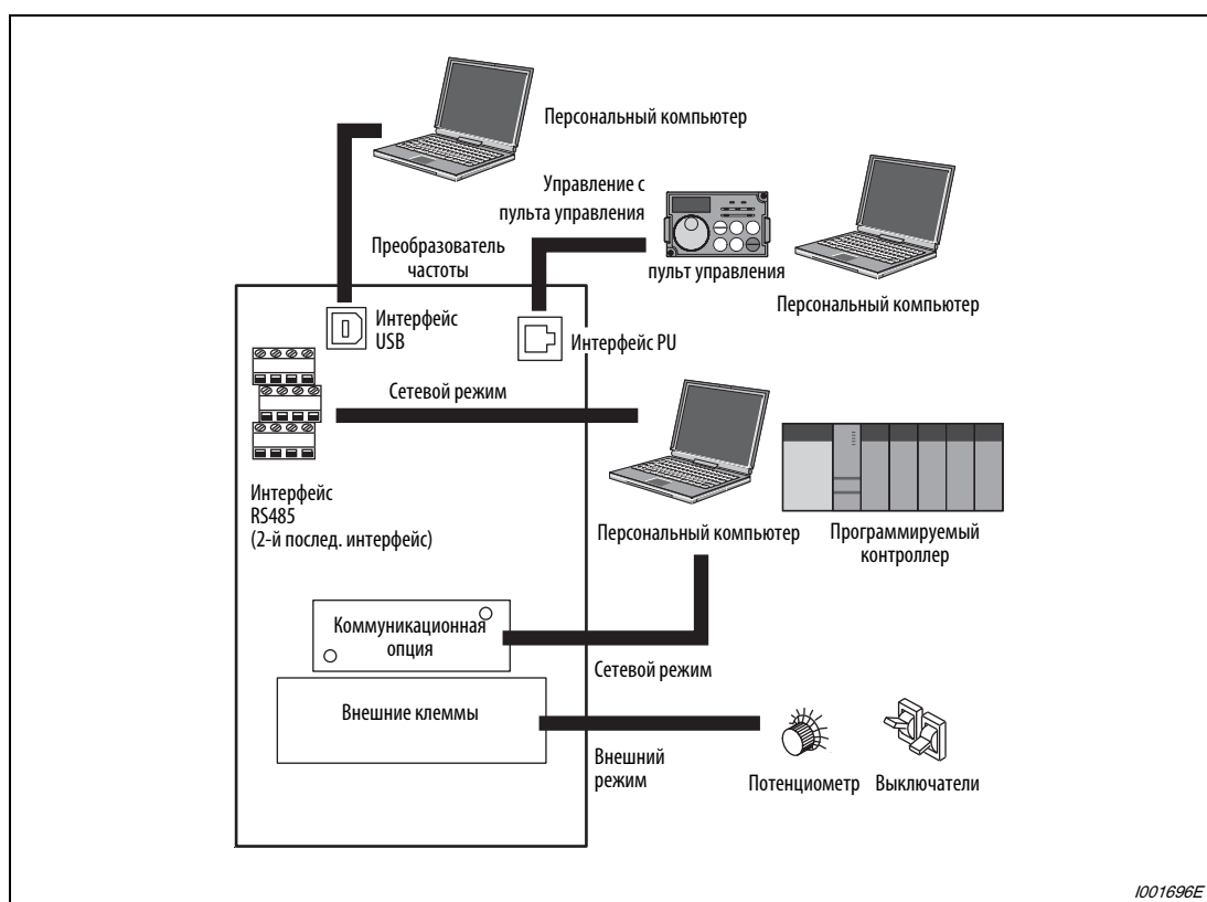
Рис. 6-202: Рабочие режимы преобразователя частоты
