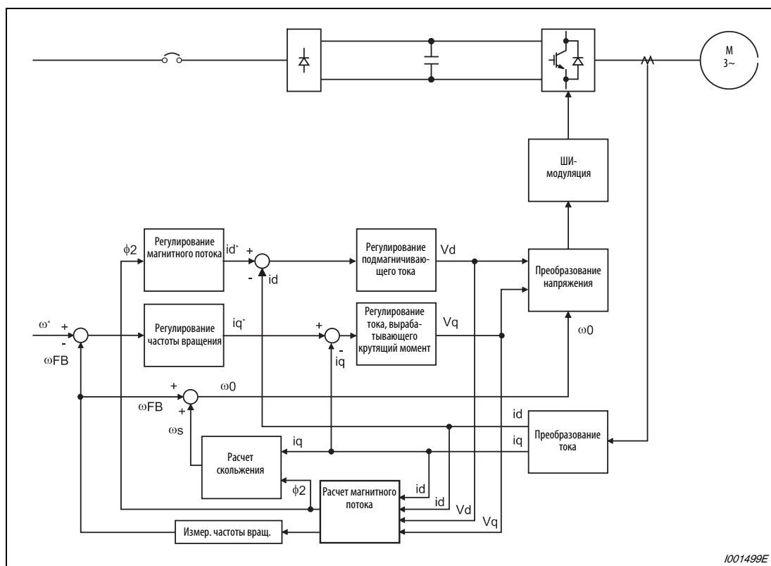
Рис. 6-3: Блок-схема бессенсорного векторного управления
