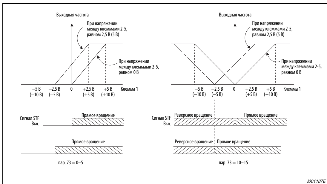
Рис. 6-181: Арифметическое наложение на задающее значение
