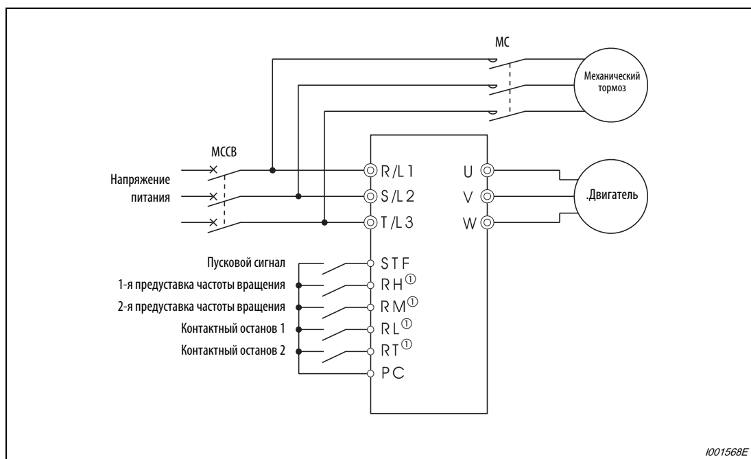
Рис. 6-108: Пример подключения
