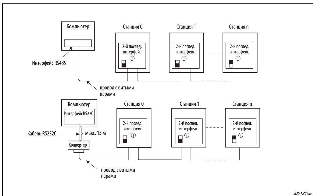
Рис. 6-217: Соединение с несколькими преобразователями частоты
