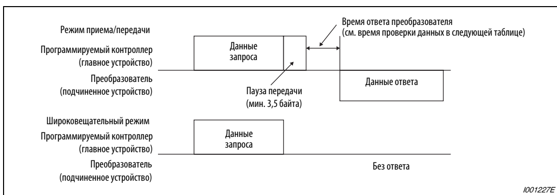
Рис. 6-230: Формат сообщений
