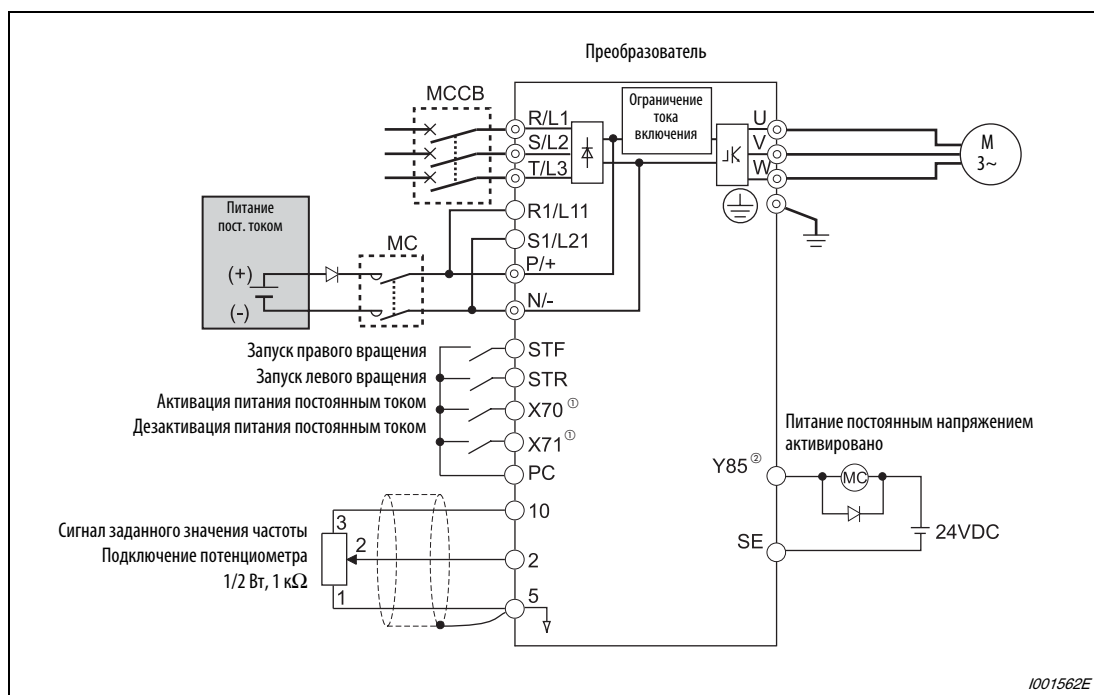
Рис. 6-100: Пример подключения для варианта 2 питания контура постоянного тока
