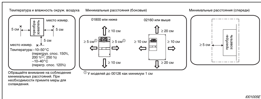
Рис. 2-8: Минимальные расстояния
