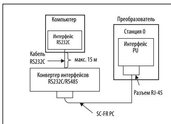
Рис. 6-212: Подключение персонального компьютера с интерфейсом RS232 к интерфейсу PU
