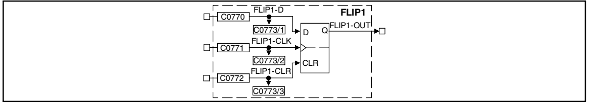
Flipflop (FLIP1)
