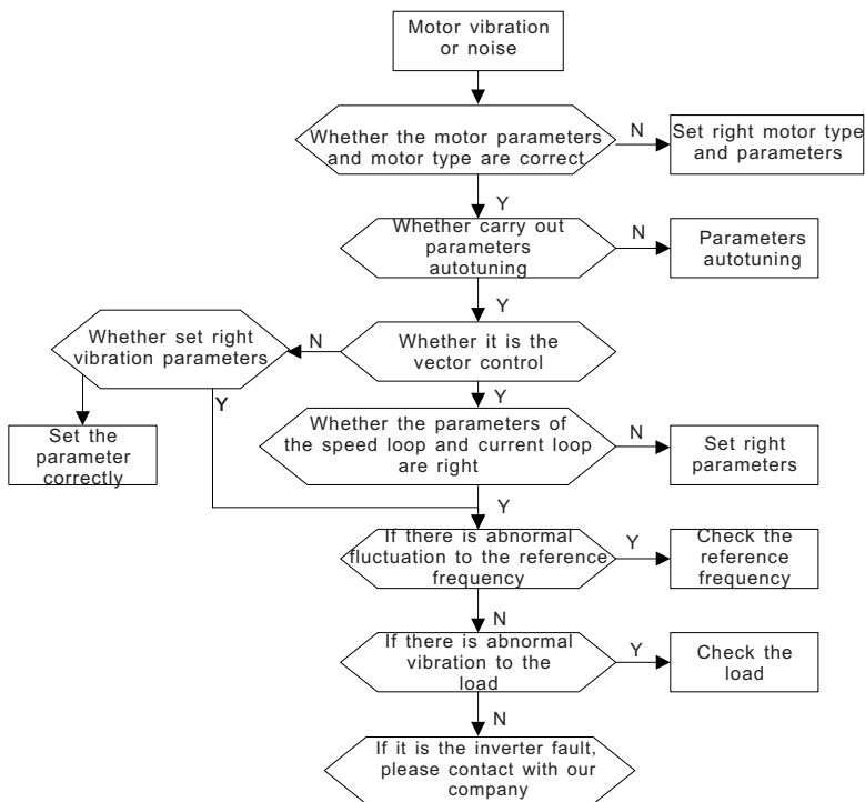
Рис. 8.2. Логика поиска и определения неисправности
