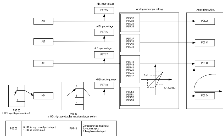
Рис. 7.15. Логика работы аналоговых входов
