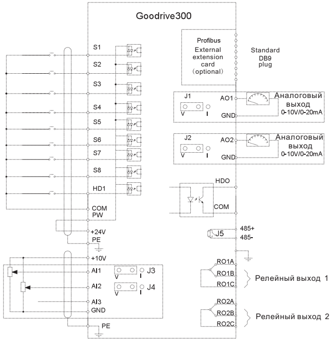
Рис.4-20Клеммы цепей контроля и управления
