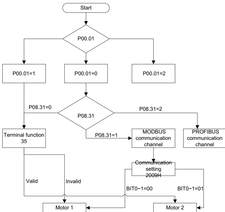
Рис. 7.9. Логика переключения между 2 двигателями
