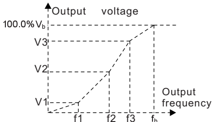
Рис. 7.5. Многоточечная кривая U/F
