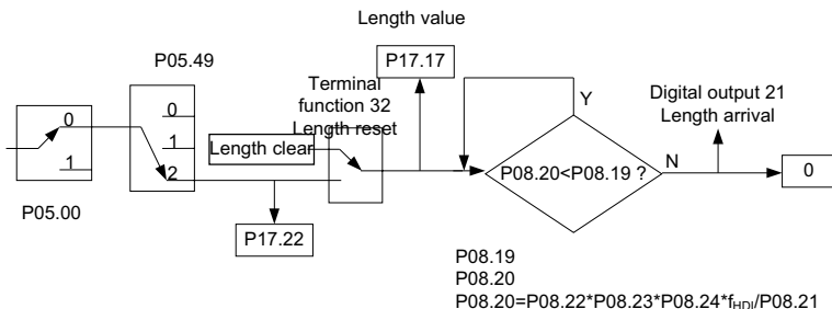
Рис. 7.23. Логика управления фиксированной длиной
