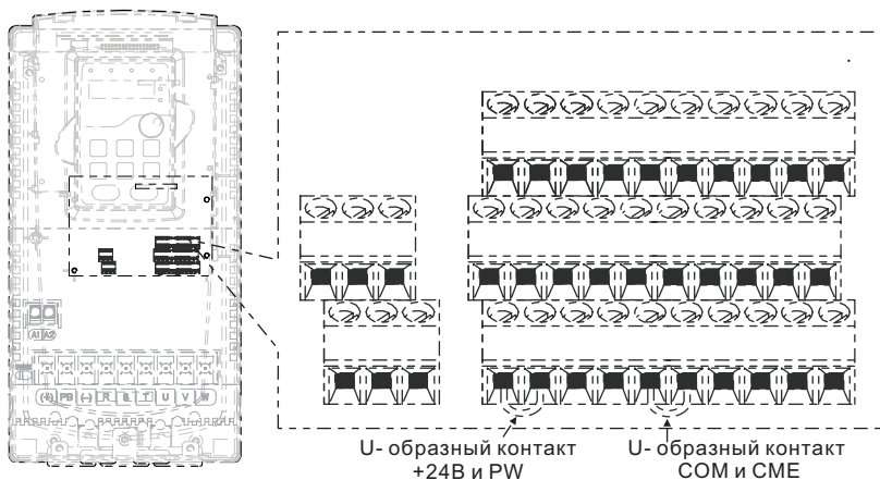
Рис. 4-22 U-образный контакт
