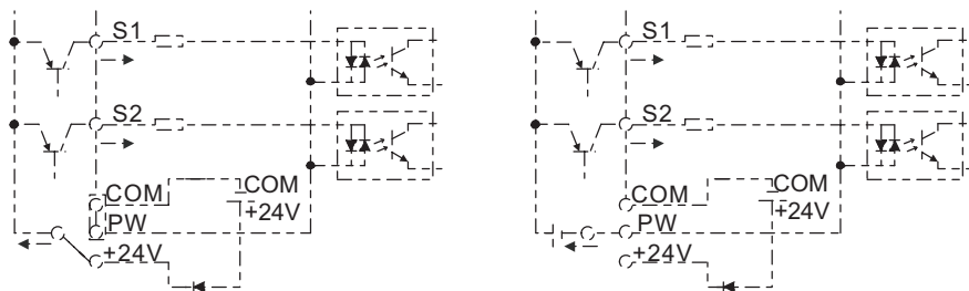
Рис. 4-24 Режим PNP
