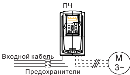
Рис. 4-25 Подключение предохранителей
