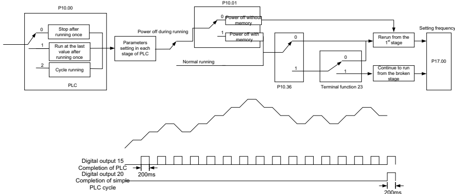
Рис. 7.18. Логика работы PLC
