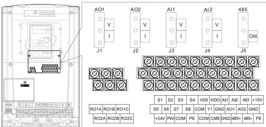
Рис. 4-21Клеммы цепей управления и контроля
