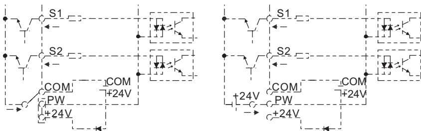
Рис. 4-23 Режим NPN
