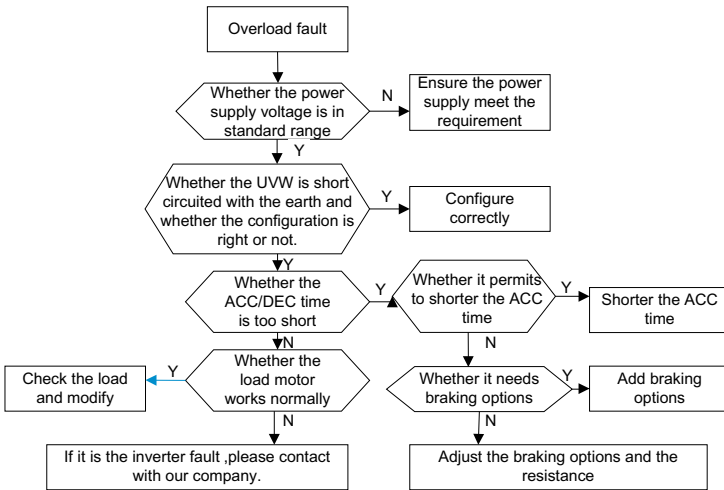
Рис. 8.3. Логика поиска и определения неисправности
