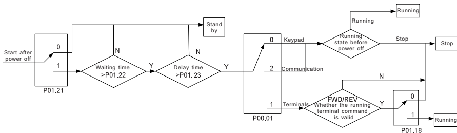
Рис. 7.11. Логика команды управления «Пуск» после перезапуска
