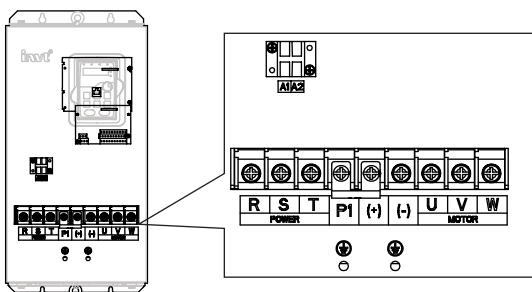
Рис.4-13 37~55 кВ клеммы силовых цепей
