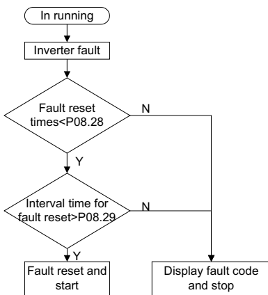
Рис. 7.12. Логика команды управления «Пуск» после сброса ошибки
