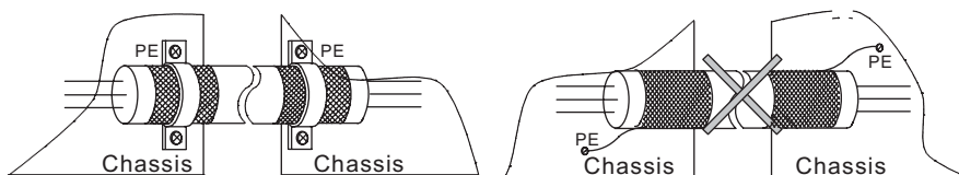
Рис 4-19 Техника заземления 360 градусов
