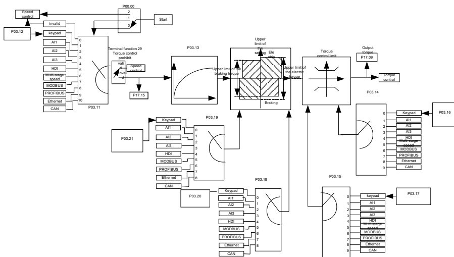
Рис. 7.8. Логика управления крутящим моментом
