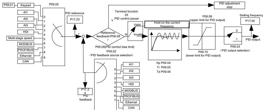
Рис. 7.20. Логика работы PID регулятора
