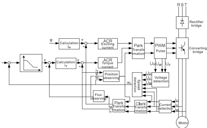
Рис. 7.3. Векторное управление
