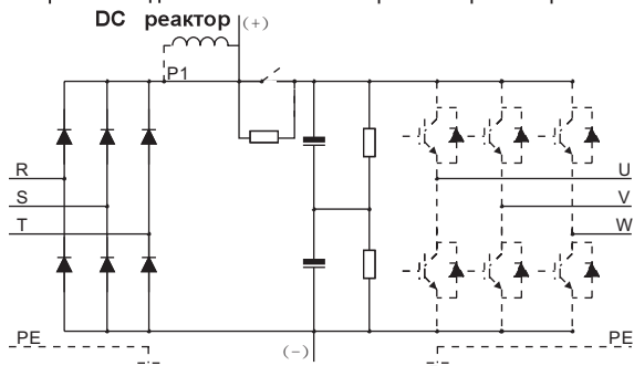
Рис. 3-1 Схема силовой цепи ( \leq 30 кВт (включая 30 кВт))
