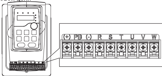
Рис. 4-8 1.5~2.2 кВ клеммы силовых цепей
