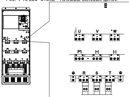
Рис. 4-17 350~500кВ клеммы силовых цепей
