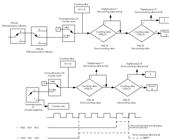
Рис. 7.22. Логика работы счетчика импульсов
