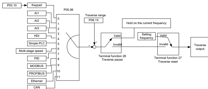
Рис. 7.21. Логика работы перехода
