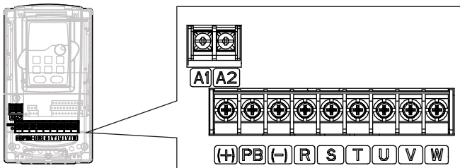
Рис. 4-9 4~9 кВт клеммы силовых цепей
