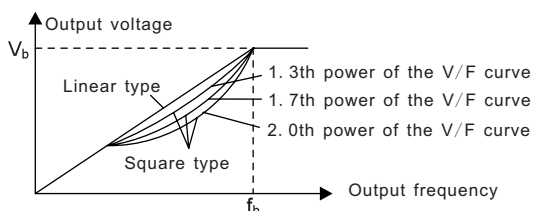
Рис. 7.4. Кривые U/F
