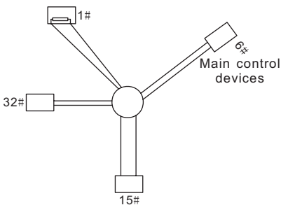
Рис. 10.5 Подключение «Звезда»
