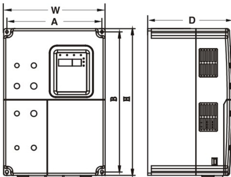
Рисунок А. 1. Габаритные размеры (до 15 кВт)
