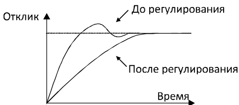
Рисунок 6.25. Подавление переуправления.
