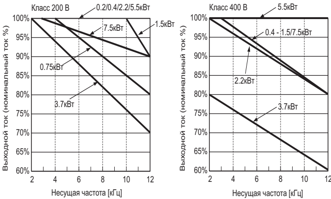
(3) Установка "стенка к стенке" (температура окружающей среды: 40°C)
