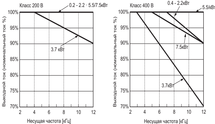
(3) Установка "стенка к стенке" (температура окружающей среды: 40°C)
