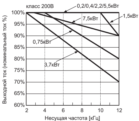
(3) Установка "стенка к стенке" (Температура среды: 40°C)
