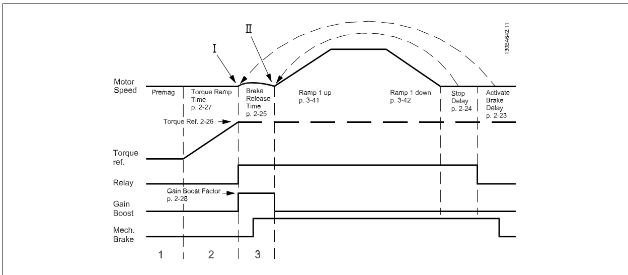
Рисунок 2.4: Последовательность отпущания тормоза при управлении механическим тормозом подъемного механизма
