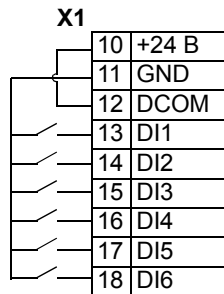
Подключение NPN
