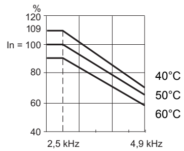
Частота коммутации
