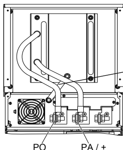
Пример 1: ATV61HD55M3X - D90M3X, ATV61HD90N4 - C16N4
