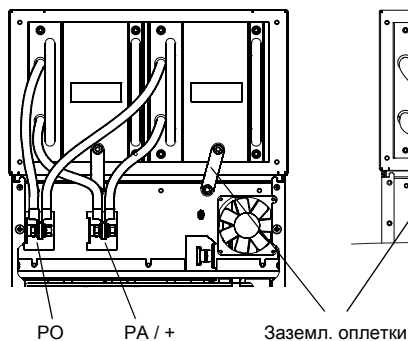
Пример 2: ATV61HC22N4 - C31N4
