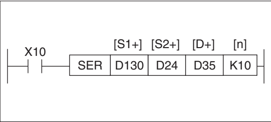
Рис. 6-108: Пример программирования SER-инструкции
