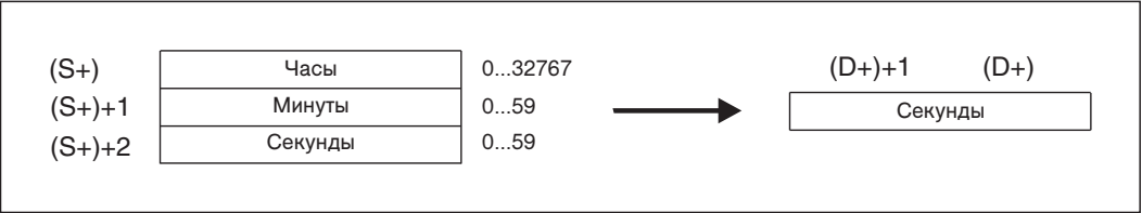
Рис. 7-151: Принцип действия команды DHTOS
