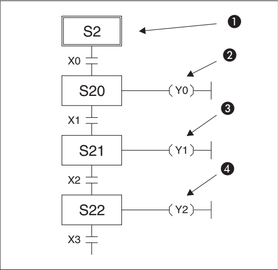
Рис. 3-17: Пример программирования для применения операндов состояния шагов ① Инициализируемое состояние ② Опускание ③ Захват ④ Подъем
