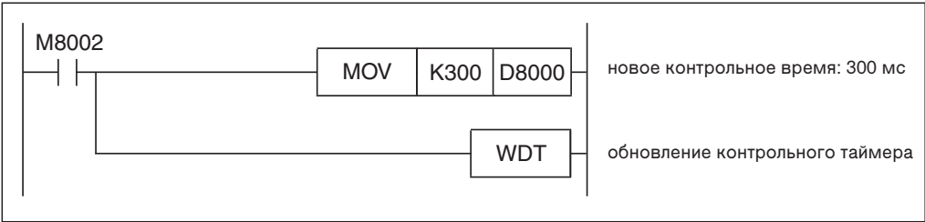
Рис. 7-321: Пример изменения настройки контрольного таймера: в первом цикле программы после запуска контроллера на один цикл устанавливается маркер M8002 и изменяется настройка контрольного таймера.
