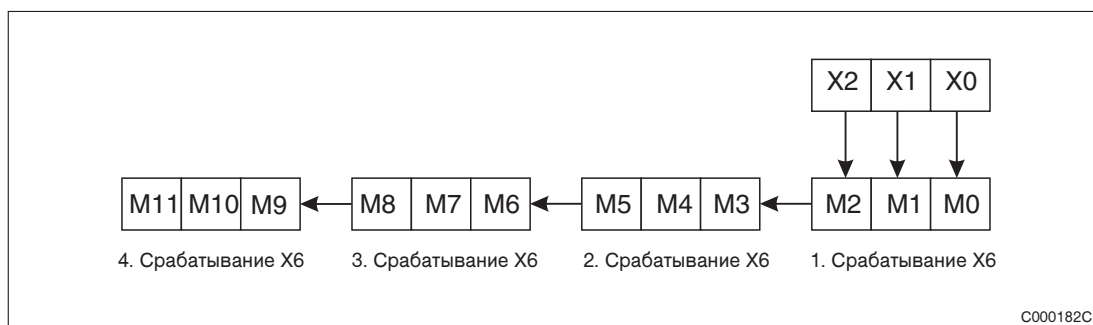
Рис. 6-63: Пример побитного сдвига влево
