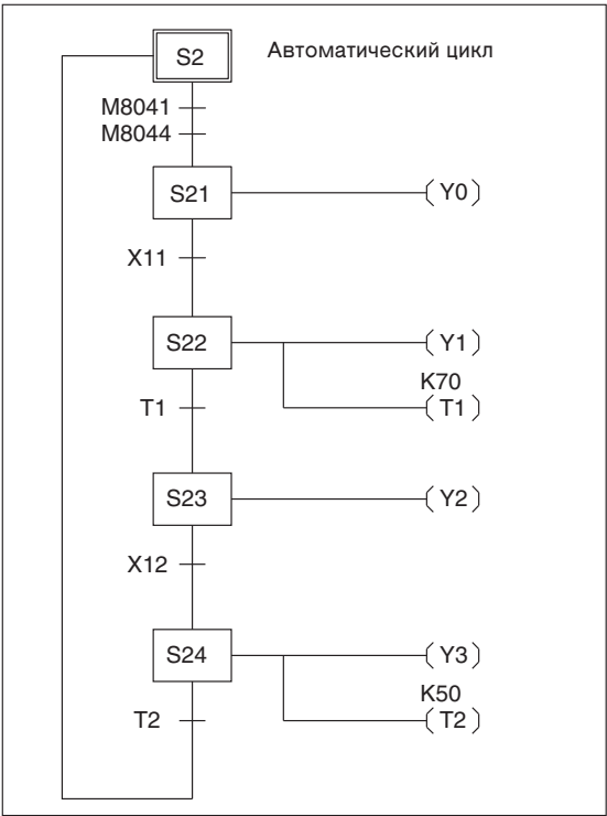
Рис. 6-106: Пример программирования контроля загрузки и разгрузки перемещаемого контейнера по IST-инструкции (автоматика)
