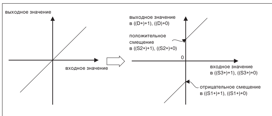
Рис. 7-271: Взаимосвязь между входным и выходным значением без ограничения (слева) и с ограничением (справа) командой DZONE
