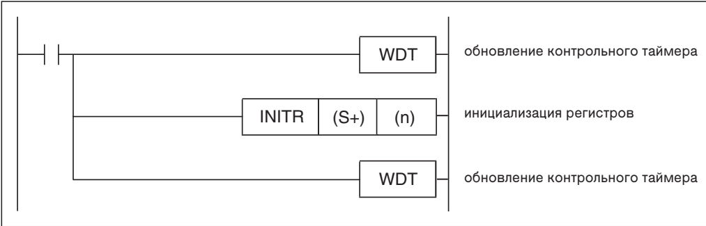
Рис. 7-311: Путем обновления контрольного таймера предотвращается возникновение ошибки при инициализации.
