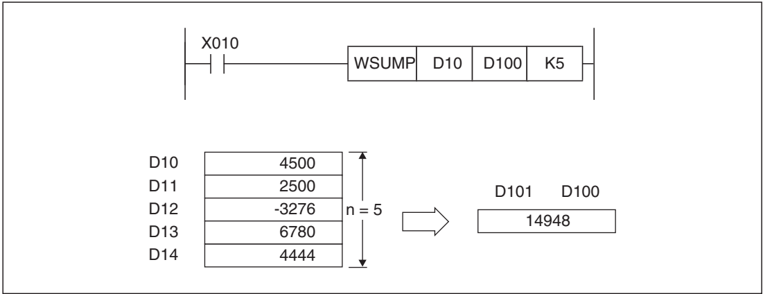
Рис. 7-113: Суммирование с помощью команды WSUMP
