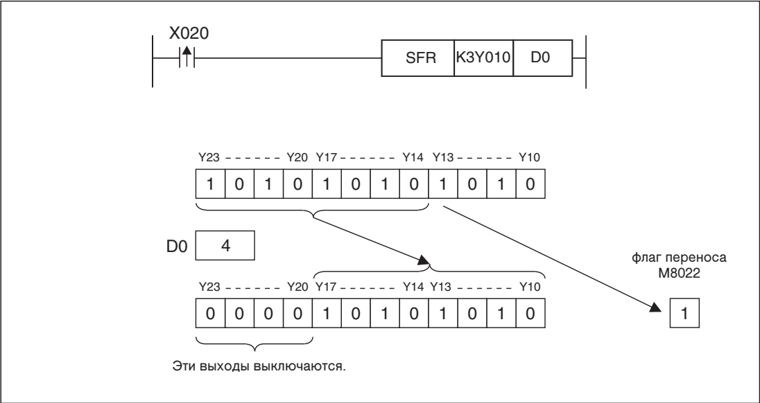
Рис. 7-255: Пример программы для команды SFR; данные сдвигаются вправо на 4 бита.
