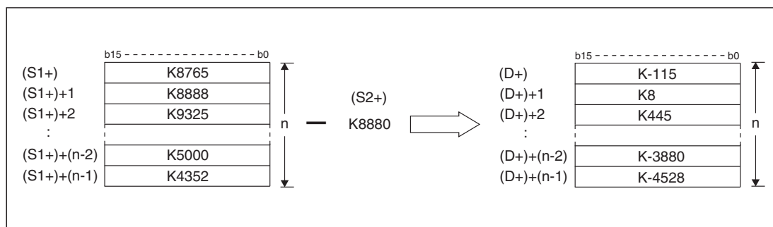
Рис. 7-197: Из содержимого блока данных вычитается константа.
