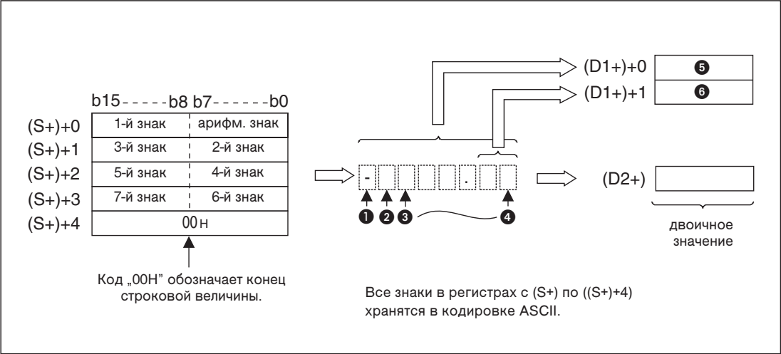
Рис. 7-216: Принцип преобразования строкового числа в 16-битовое двоичное значение с помощью команды VAL или VALP
