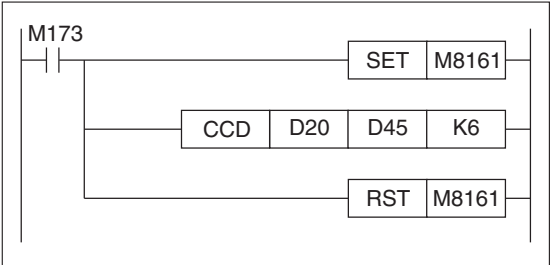
Рис. 7-42: Пример программирования CCD-инструкции
