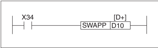
Рис. 7-127: Пример программирования SWAPP-инструкции
