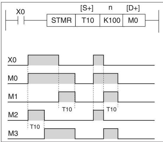
Рис. 6-115: Пример программы для генерации задержки выключения (M0) и импульса (M1) со временем 10 секунд.
