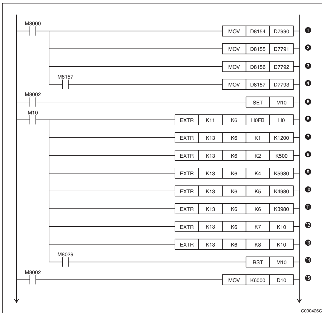
Рис. 7-176: Пример программы с приостановкой функции мониторинга (часть1)
