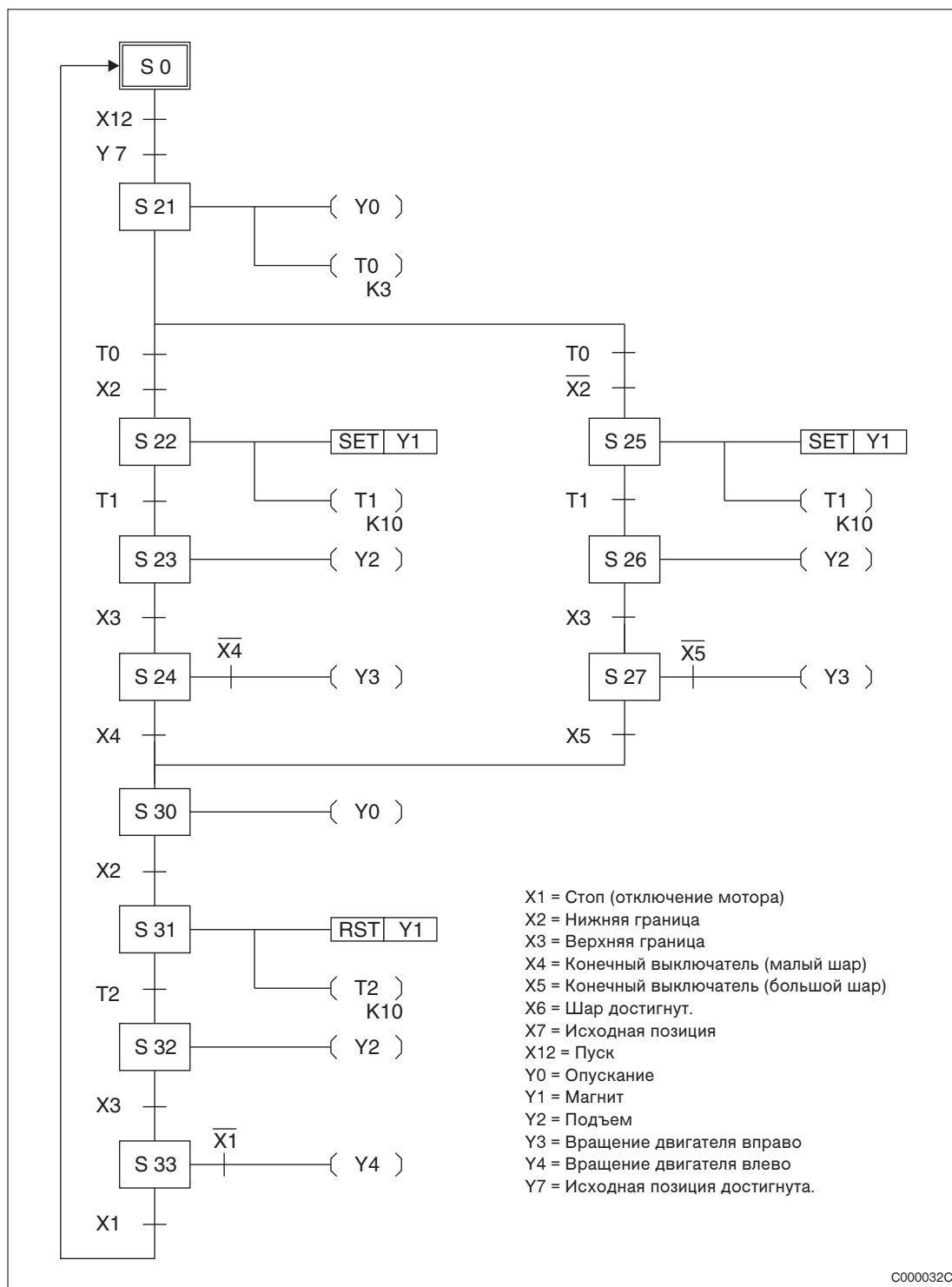
Рис. 5-26: Пример программирования приведенного впереди устройства сортировки
