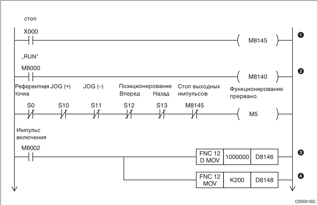
Рис. 7-132: Пример программы движения
