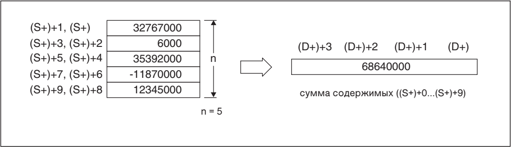
Рис. 7-112: Пример выполнения команды DWSUM для суммирования 32-битных данных
