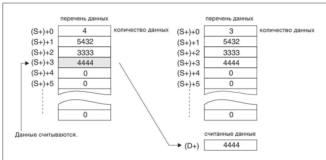
Рис. 7-251: При считывании данных содержимое перечня данных не изменяется.
