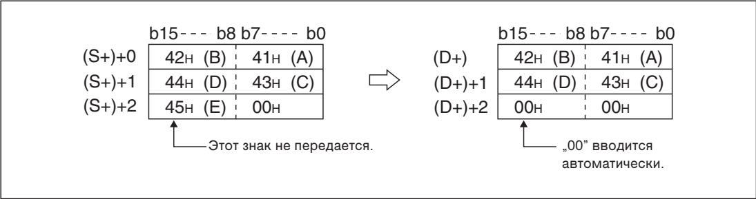
Рис. 7-244: Все знаки после кода „00” игнорируются.
