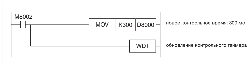
Рис. 7-296: Пример изменения настройки контрольного таймера: в первом программном цикле после запуска контроллера на один цикл устанавливается маркер M8002 и изменяется настройка контрольного таймера.
