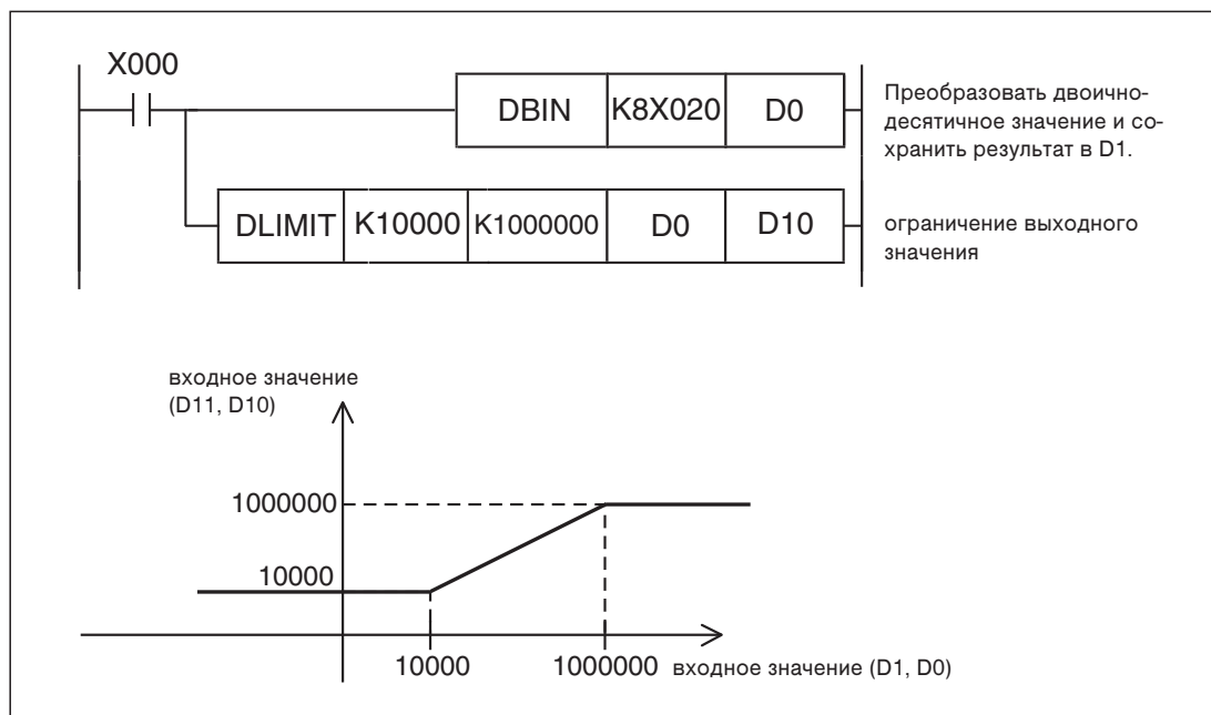
Рис. 7-265: Эта программа ограничивает значение в D11 и D10 пределами 10000 и 1000000.
