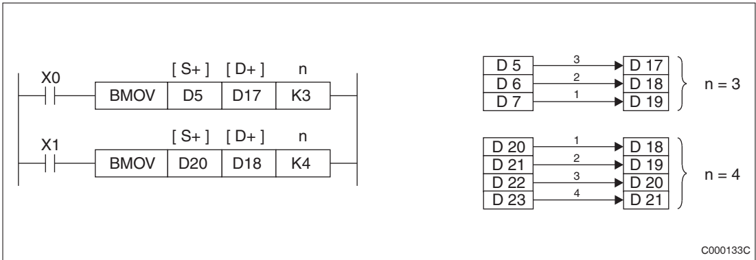
Рис. 6-28: Передача блока
