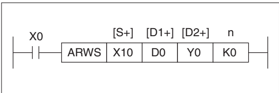
Рис. 7-16: Пример программирования ARWS-инструкции
