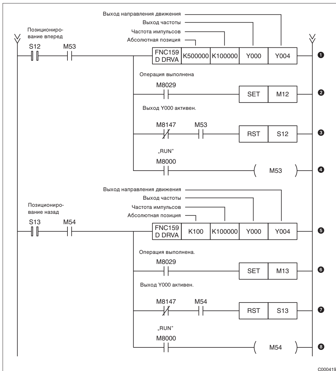
Рис. 7-135: Пример программы
