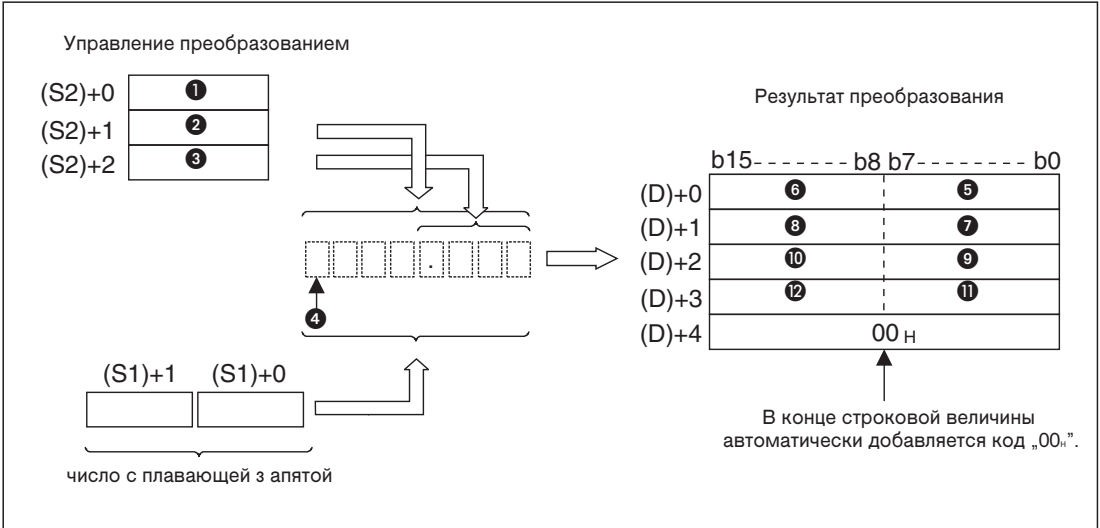
Рис. 7-57: Принцип преобразования числа с плавающей запятой в строковую величину при десятичном представлении результата ❶ Формат отображения; в случае десятичного представления регистр (S2+) + 0) должен содержать значение „0“. ❷ Общее количество разрядов ❸ Количество разрядов дробной части
