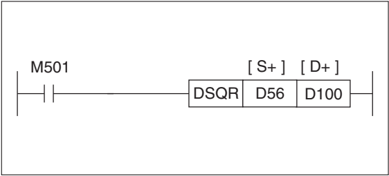
Рис. 6-80: Пример программирования расчета корня квадратного
