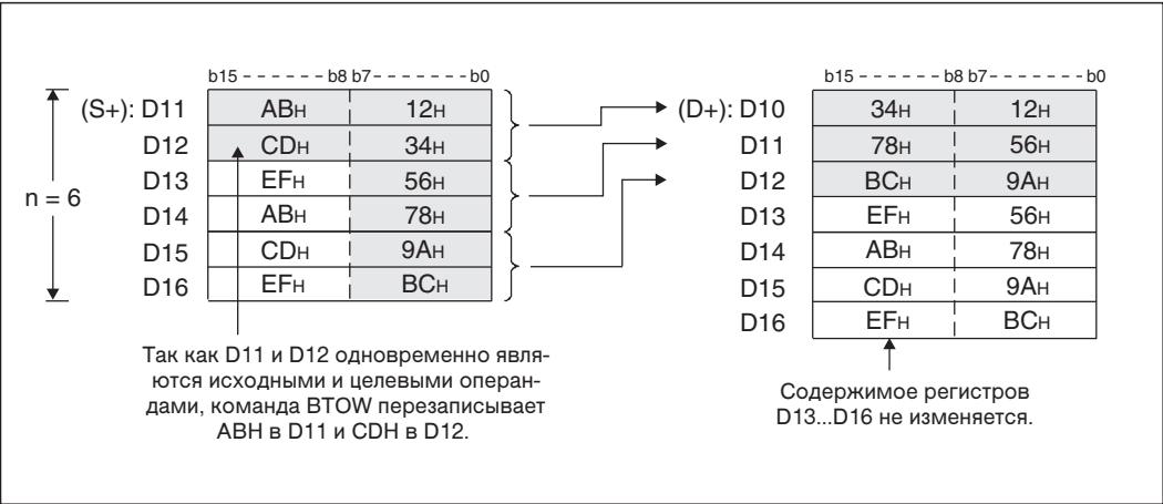
Рис. 7-120: Пример использования одних и тех же операндов в качестве исходной целевой области.
