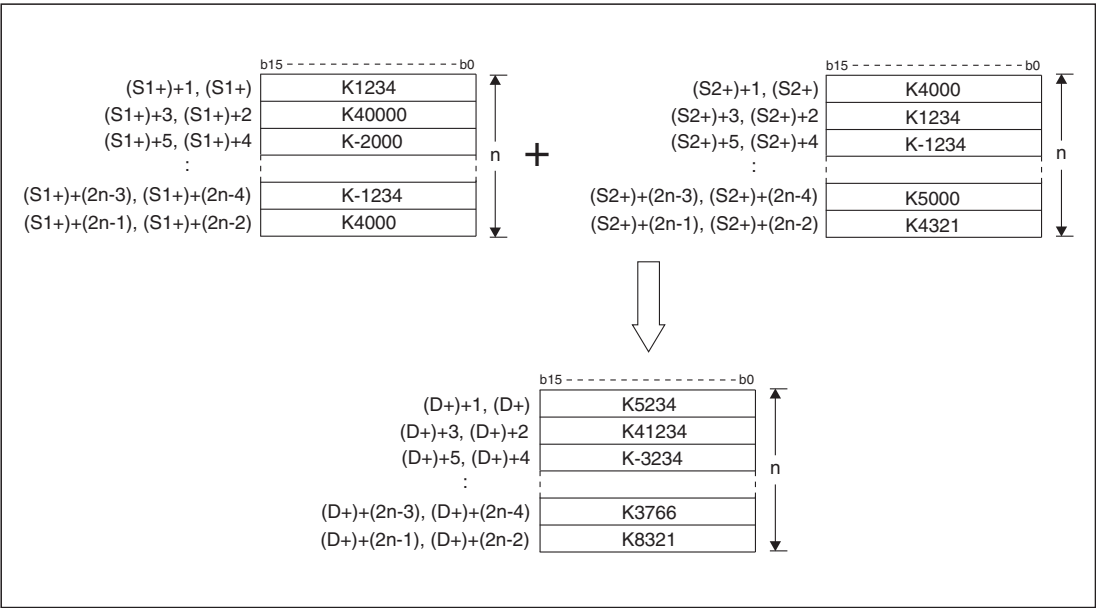
Рис. 7-193: Суммирование содержимых двух блоков данных, состоящих из 32-битных операндов
