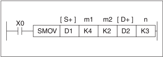
Рис. 6-21 Пример программирования с использованием SMOV-инструкции без специального маркера
