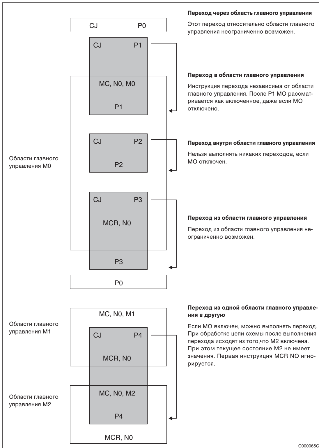
Рис. 6-11: Примеры переходов в области главного управления
