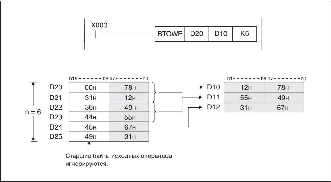
Рис. 7-121: Пример объединения данных с помощью команды BTOWP
