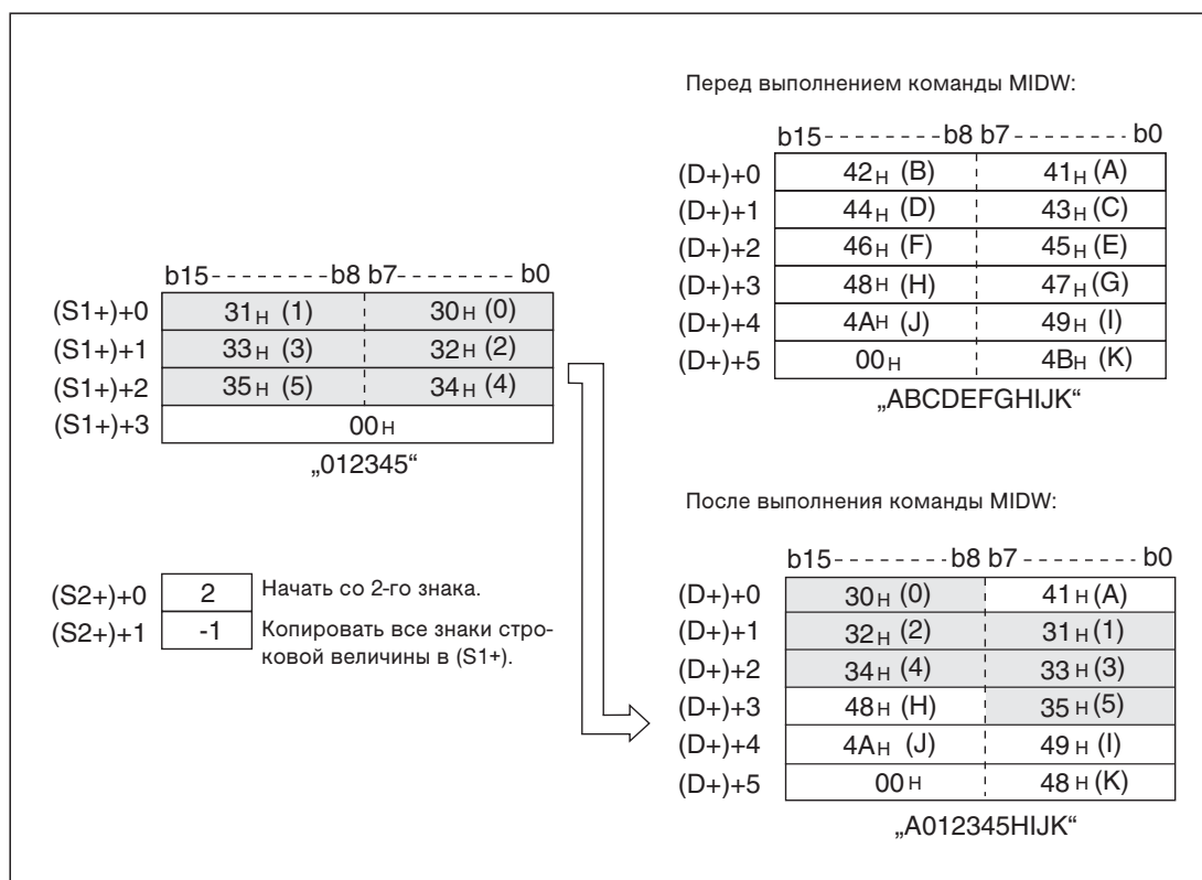
Рис. 7-237: Если ((S2+)+1) имеет значение „-1“, копируются все знаки строковой величины, указанной в (S1+), в строковую величину, указанную в (D+), начиная со знака, указанного в ((S2+)+0).
