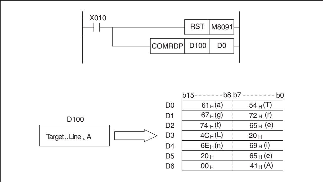
Рис. 7-181: Комментарий к операнду D100 записывается в виде знаков ASCII в регистры с D0 по D6.
