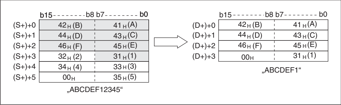
Рис. 7-230: Пример применения команды LEFT: первые 7 знаков строковой величины „ABCDEF12345” считываются и сохраняются по адресу, начиная с (D+).
