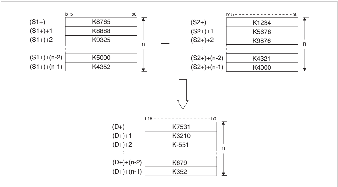
Рис. 7-196: Определение разности содержимых двух блоков данных
