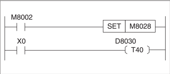
Рис. 8-13: Таймер на 10 мс с переменным временем (FX1S)
