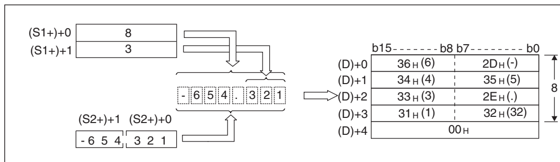
Рис. 7-212: Двоичное значение -654321 преобразуется в строковую величину с общим количеством разрядов 8 (из них 3 в дробной части). Результат сохраняется по адресу, начиная с (D+).
