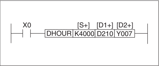
Рис. 7-163: Пример программирования DHOUR-инструкции
