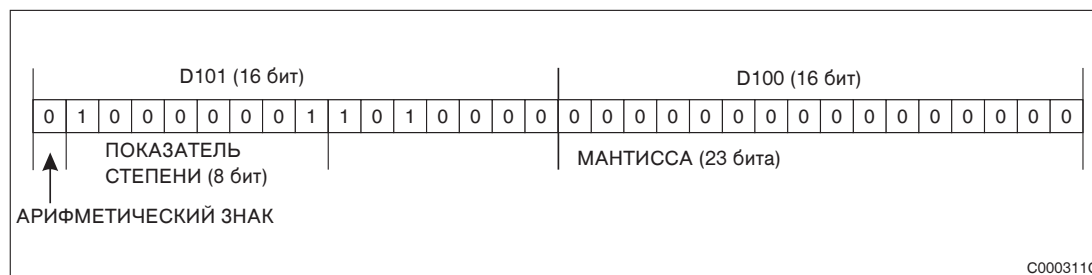
Рис. 3-27: Размещение бит в регистре данных
