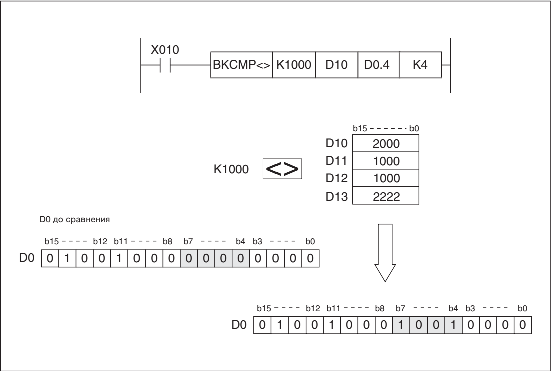
Рис. 7-206: В этом примере результаты сравнения сохраняются в регистре данных. На остальные биты D0 сравнение не влияет.
