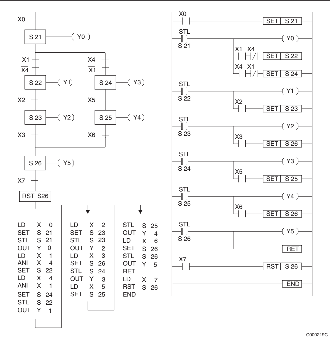
Рис. 5-16: Пример программирования селективного разветвления
