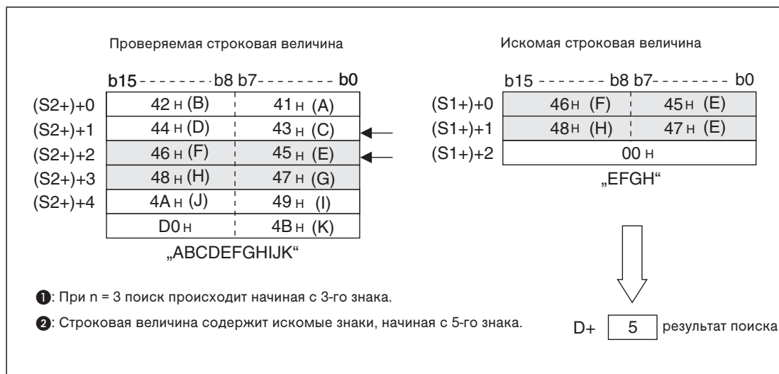
Рис. 7-239: Результат поиска показывает позицию первого знака искомой цепочки символов.
