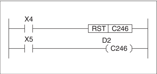
Рис. 3-14: Пример программирования с использованием 2-х фазного счетчика без входов пуска и сброса (C246)
