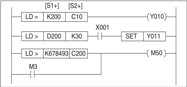
Рис. 7-259: Пример программирования LD□-инструкции
