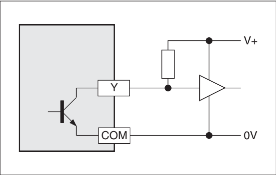
Рис. 7-13: При включенном выходе подключается минус силового напряжения.
