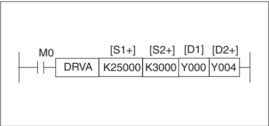
Рис. 7-140 Пример программирования DRVA-инструкции
