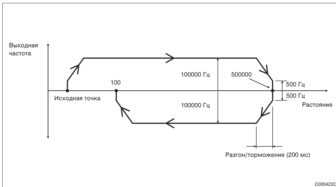
Рис. 7-131: Пример программы
