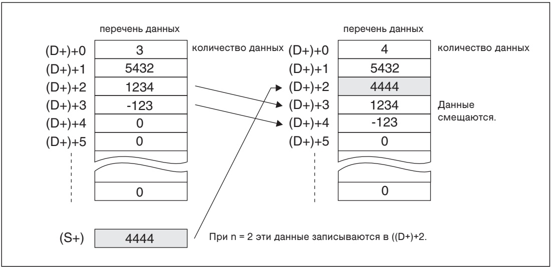
Рис. 7-248: Команда FINS вставляет данные в перечень данных. Имеющиеся данные сдвигаются.
