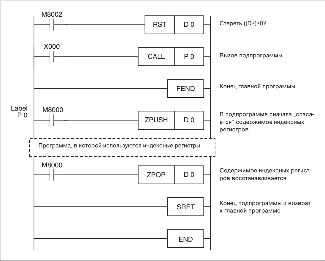
Рис. 7-52: Пример применения команд ZPUSH и ZPOP
