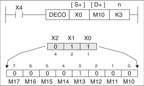
Рис. 6-71: Пример программирования DECO-инструкции с указанием битовых операндов в D+
