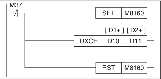
Рис. 6-32: Пример программирования с DXCH-инструкцией со специальным маркером M8160
