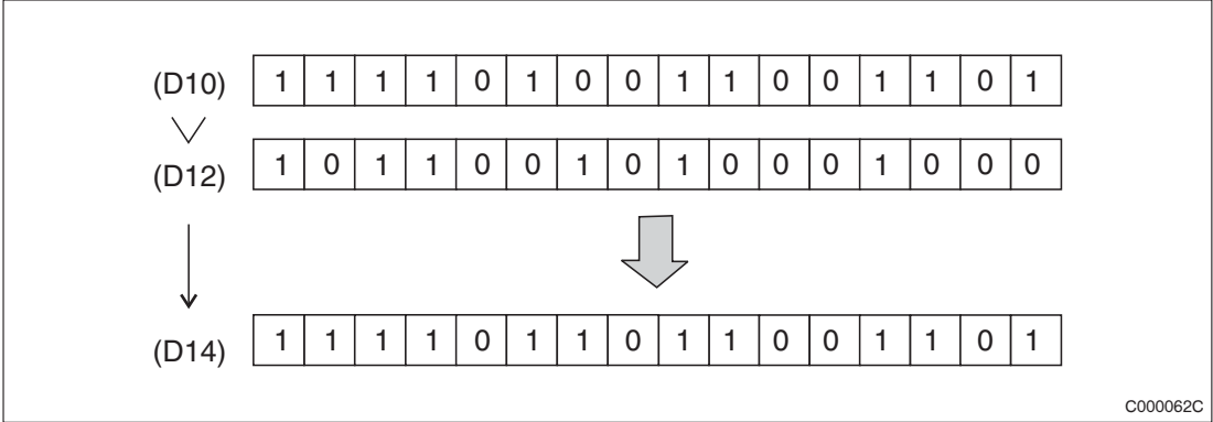
Рис. 6-51: Применение WOR-инструкции
