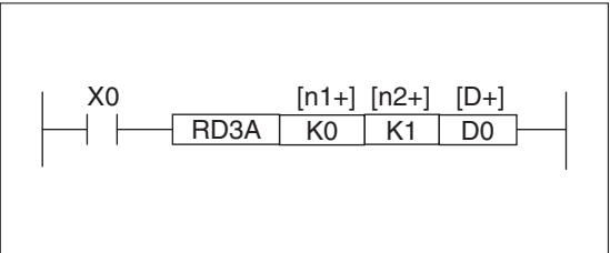
Рис. 7-166: Пример программирования RD3A-инструкции Аналоговое значение аналогового модуля FX0N-3A, установленное в канале 1, передается по адресу 0 в регистр D0.
