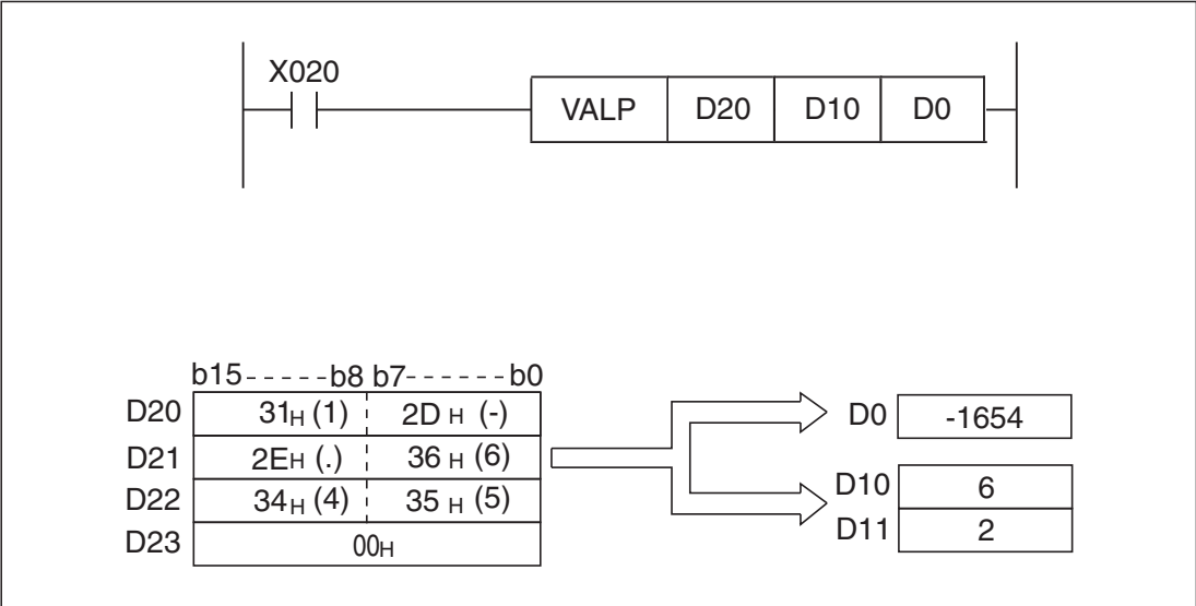
Рис. 7-220: Пример программы для преобразование строкового числа в 16-битовое двоичное число
