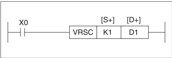
Рис. 7-45: Пример программирования для VRSC-инструкции
