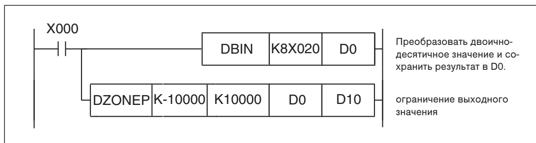
Рис. 7-273: С помощью этой программы не выводятся выходные значения между –10000 и 10000.
