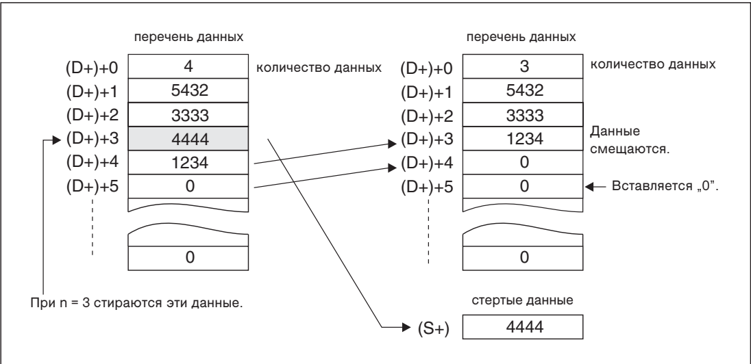
Рис. 7-246: Команда FDEL стирает данные из перечня данных и перемещает их по другому адресу.
