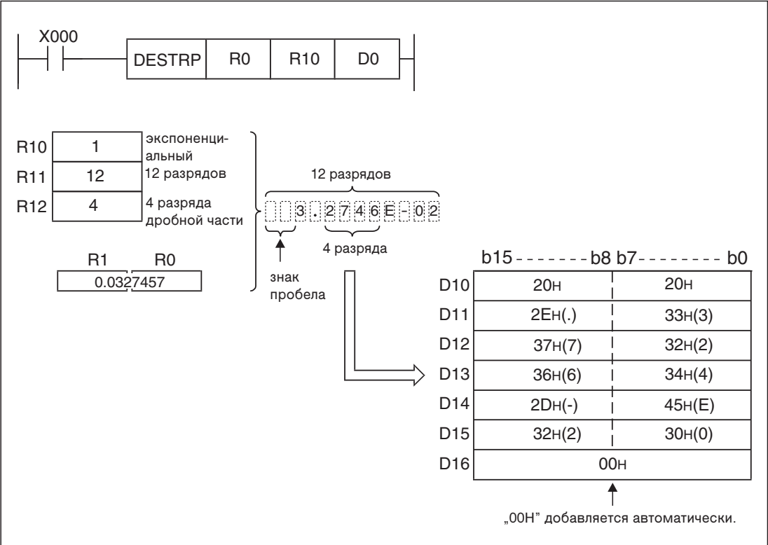
Рис. 7-68: Пример программы для преобразования в экспоненциальное представление
