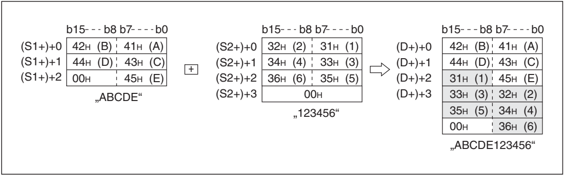
Рис. 7-221: Строковые величины в (S1+) и (S2+) объединяются и записываются в (D+). (Строковая величина из (S2+) здесь изображена на сером фоне.)
