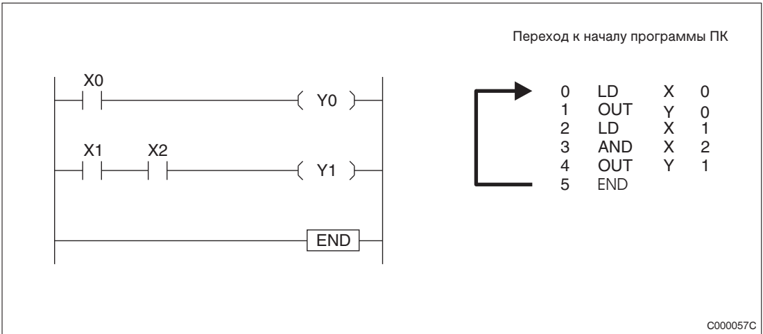
Рис. 4-22: Пример программирования END-инструкции
