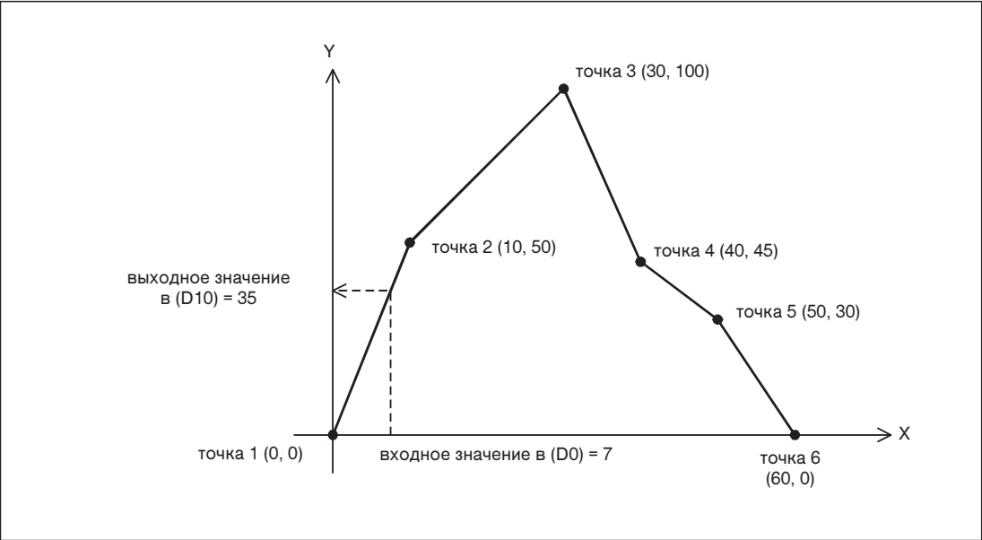
Рис. 7-294: Кривая для масштабирования входного значения в этом примере
