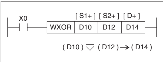
Рис. 6-52: Пример программирования WXOR-инструкции („Исключающего ИЛИ”-связи)
