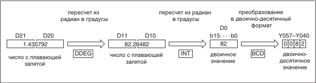
Рис. 7-110: Пример программы, которая при вводе 1.435792 рад преобразует это значение в 82 градуса и выводит результат.
