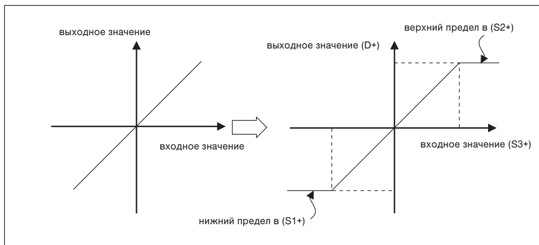
Рис. 7-262: Взаимосвязь между входным и выходным значением без ограничения (слева) и с ограничением (справа) с помощью команды LIMIT
