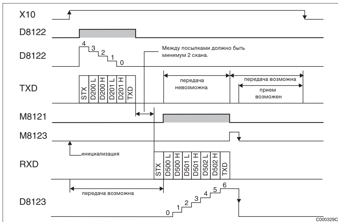
Рис. 7-35: Представление временного процесса
