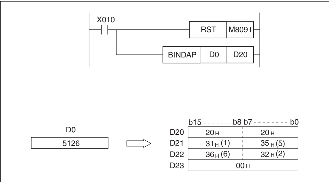
Рис. 7-289: Перед преобразованием сбрасывается маркер M8091, чтобы в D23 было записано значение „00H”.
