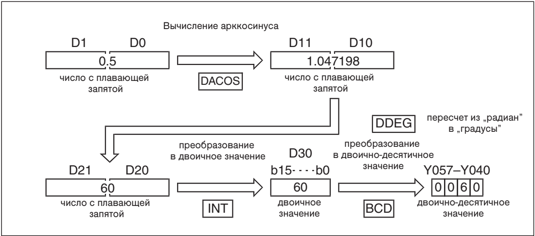
Рис. 7-102: При задании косинуса „0.5” вышеприведенная программа показывает угол „60”.
