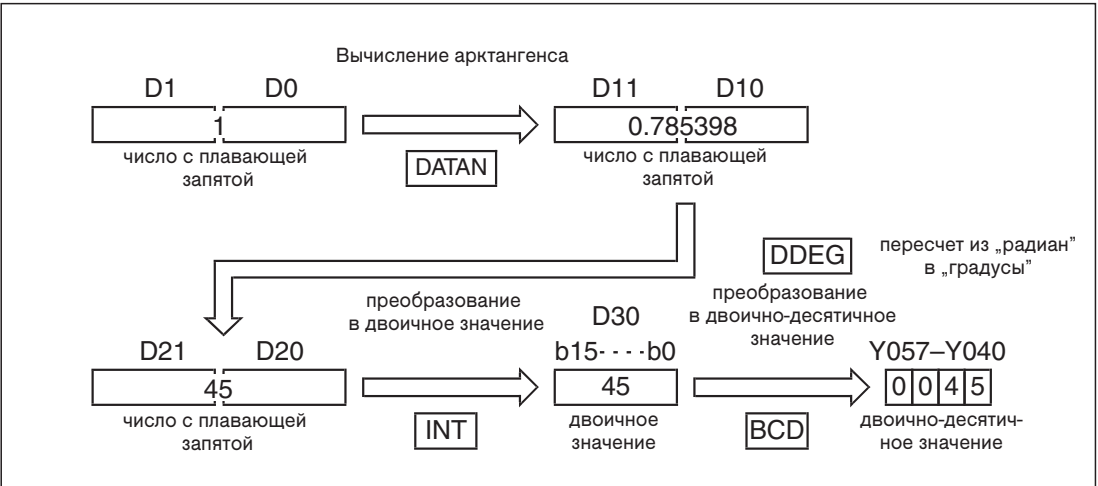
Рис. 7-104: При задании тангенса „1” вышеприведенная программа показывает угол „45”.
