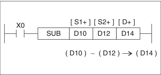
Рис. 6-40: Пример программирования SUB-инструкции
