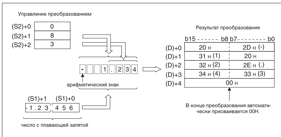
Рис. 7-58: Так как преобразуемое число с плавающей запятой имеет 5 разрядов дробной части, а строковая величина только 3 разряда дробной части, разряды утрачиваются.
