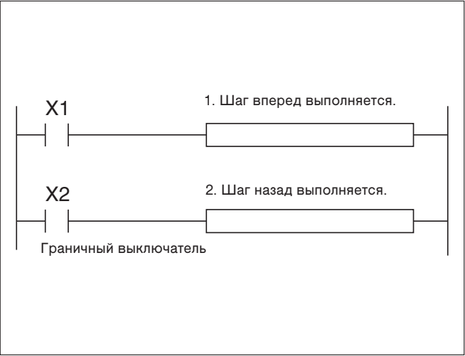
Рис. 5-2: Пример схемы без блокировочных контактов
