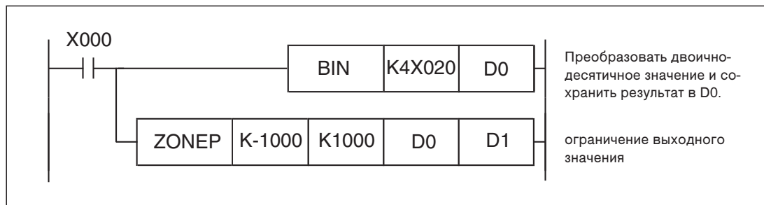
Рис. 7-272: С помощью этой программы не выводятся выходные значения между –1000 и 1000.
