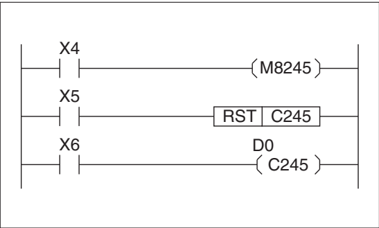
Рис. 3-13: Пример программирования с использо- ванием 1-фазного счетчика с входами пуска и сброса (C245)
