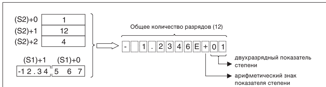
Рис. 7-66: Отображение показателя степени
