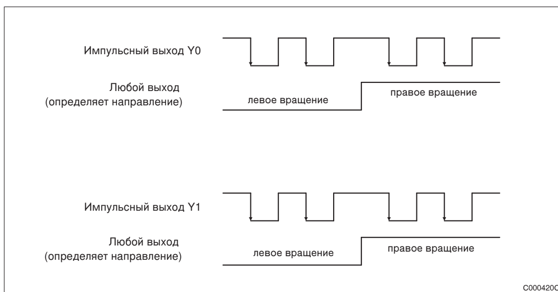
Рис. 7-129: Формат выходных сигналов
