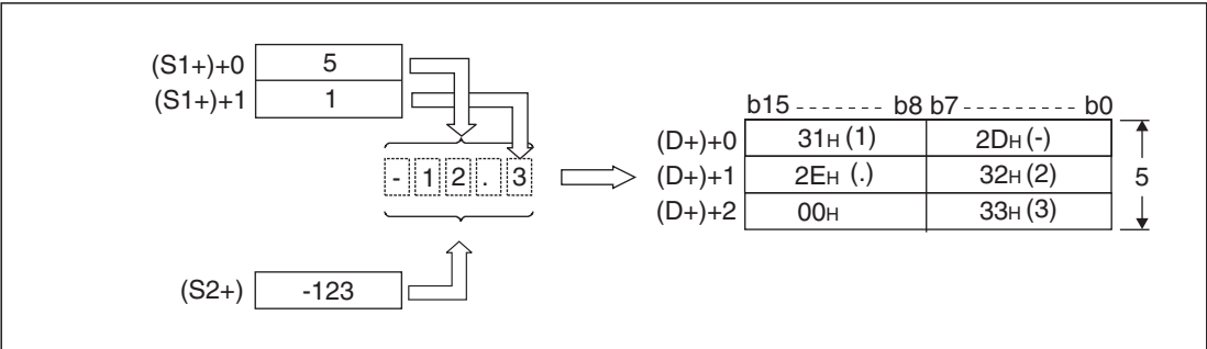
Рис. 7-210: Двоичное значение -123 преобразуется в строковую величину с общим числом разрядов 5 (из них один десятичный разряд после запятой). Результат сохраняется по адресу, начиная с (D+).
