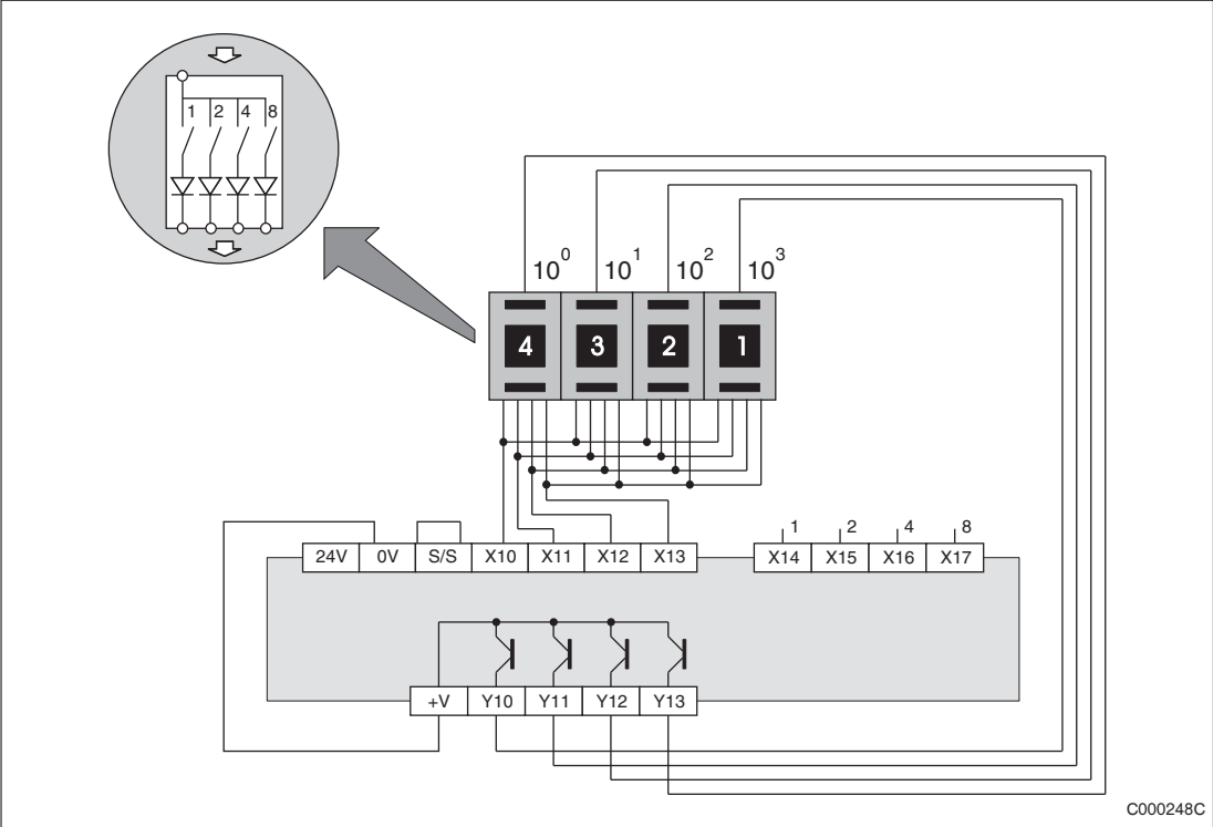
Рис. 7-8: Схема присоединения входов/выходов
