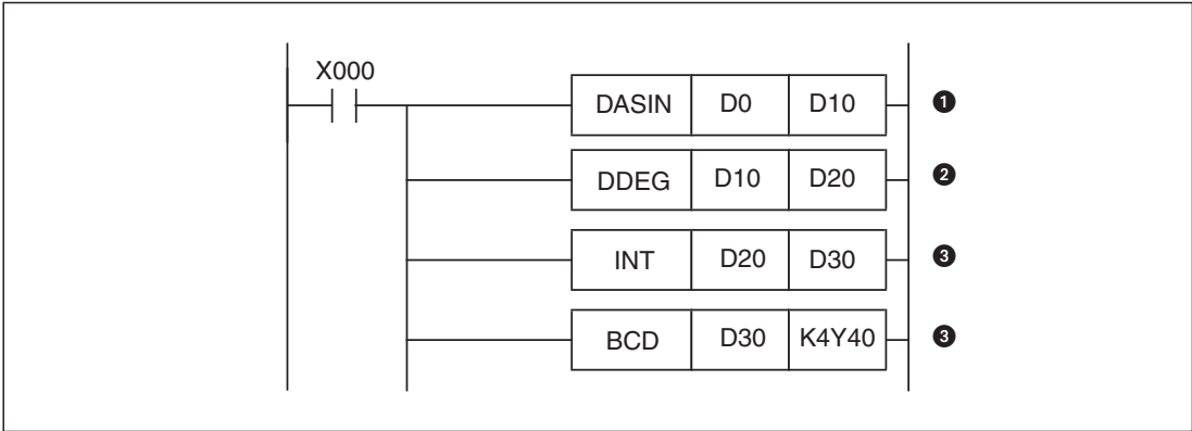
Рис. 7-99: Пример программы для вычисления арксинуса и вывода угла на двоично-десятичный дисплей.
