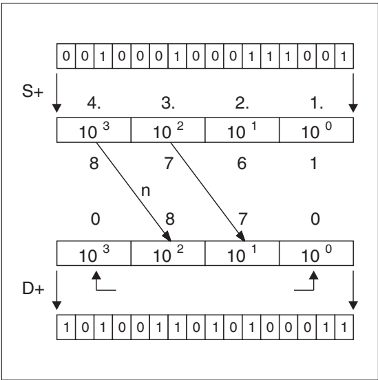
Рис. 6-23: Конвертирование и передача
