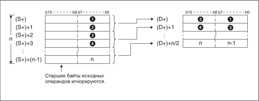
Рис. 7-118: Принцип действия команды BTOW
