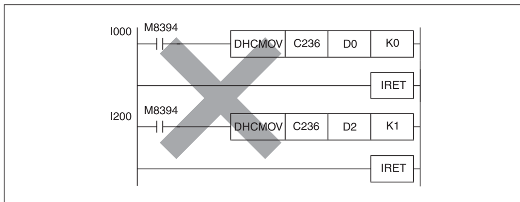
Рис. 7-188: В этом примере команды DHCMOV два раза обращаются к одному и тому же счетчику. Это недопустимо.
