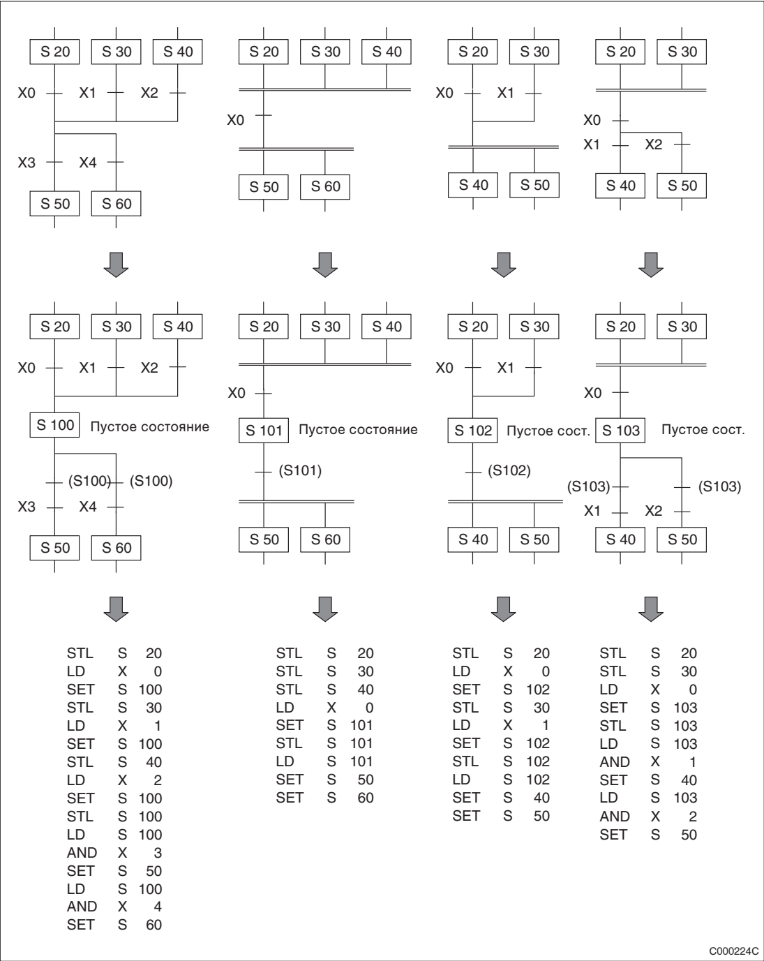
Рис. 5-20: Программирование пустого состояния
