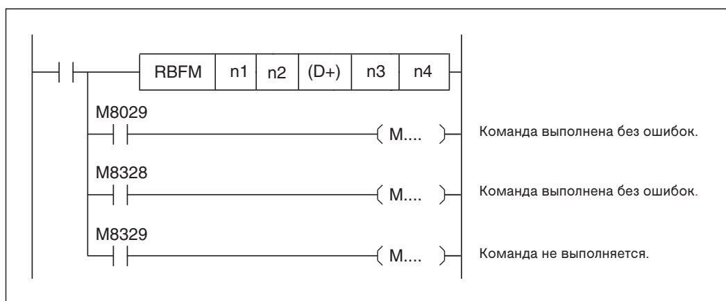
Рис. 7-295: Состояние маркеров M8029, M8328 и M8329 необходимо проверять сразу после команды RBFM.
