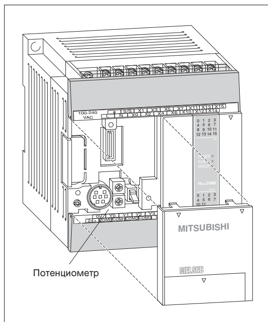
Рис. 3-19: Потенциометры на ПК серии FX1S/FX1N
