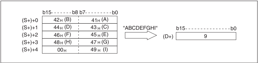
Рис. 7-224: В этом примере подсчитываются знаки в строке „ABCDEFGHI” и в качестве результата в (D+) вводится „9”.
