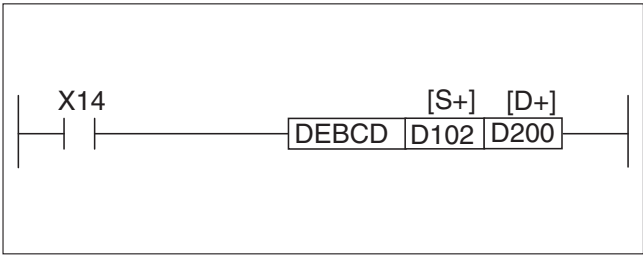
Рис. 7-78: Пример программирования DEBCD-инструкция
