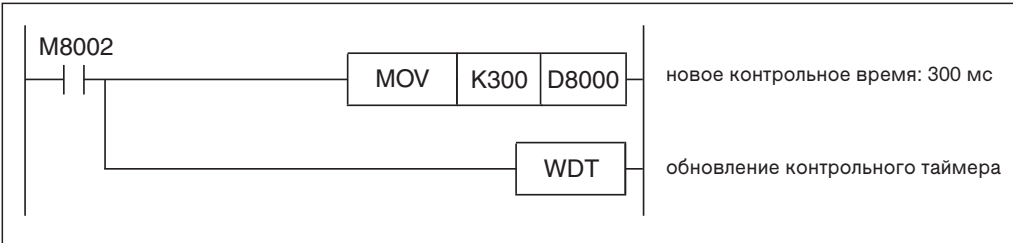
Рис. 7-310: Пример изменения настройки контрольного таймера: в первом цикле программы после запуска контроллера на один цикл устанавливается маркер M8002 и изменяется настройка контрольного таймера.
