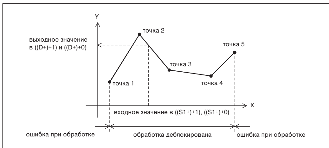
Рис. 7-276: Если входное значение находится вне формы кривой, заданной таблицей, возникает ошибка.
