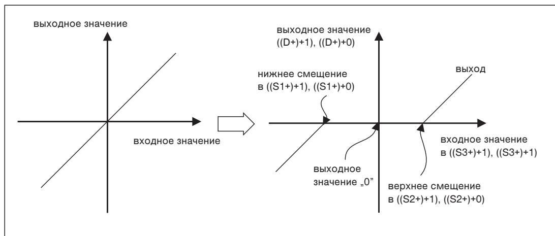
Рис. 7-267: Взаимосвязь между входным и выходным значением без ограничения (слева) и с ограничением (справа) командой DBAND
