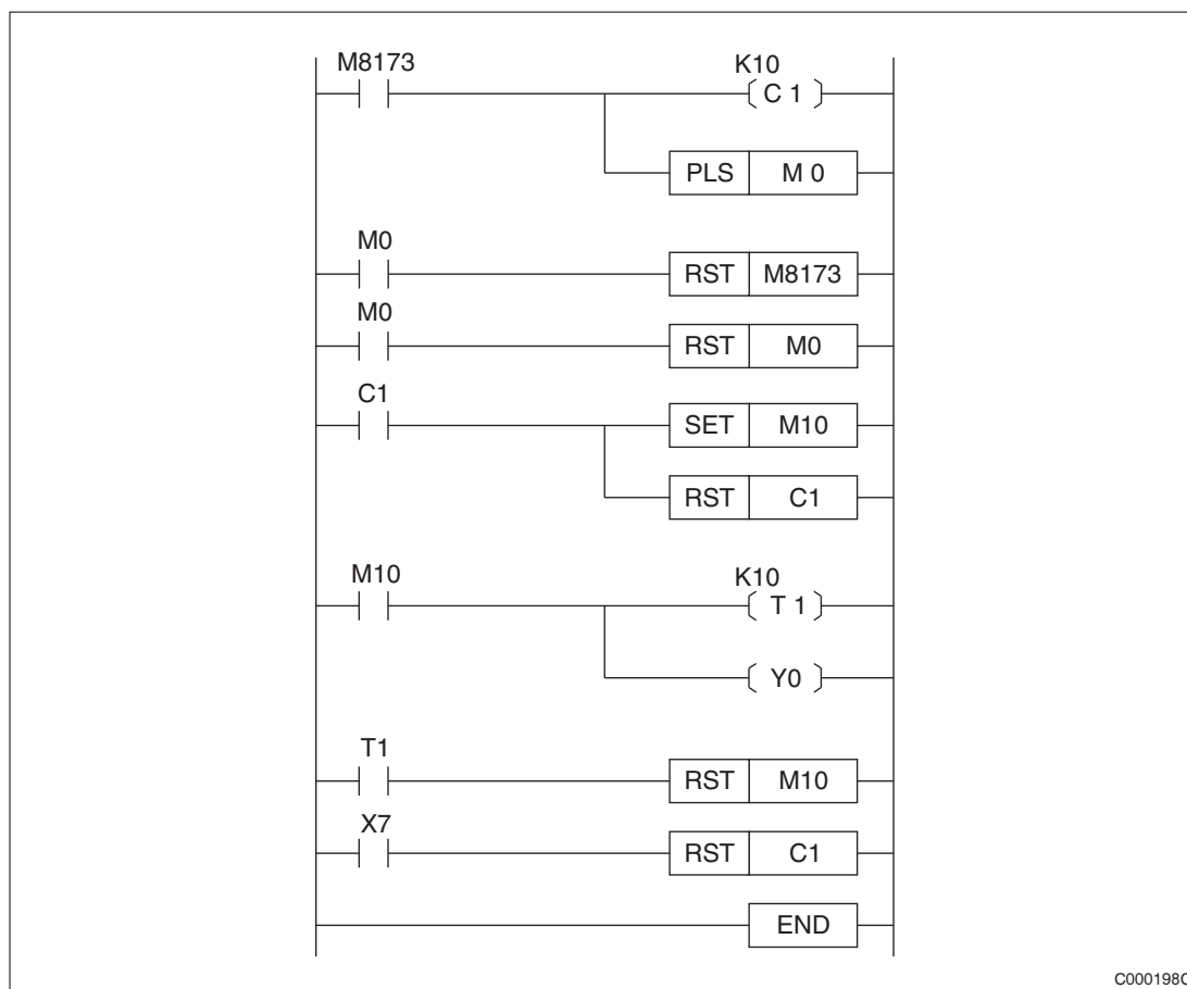
Рис. 8-6: Пример программирования Функции фиксации импульсов и счета импульсов по фотореле и по входу X3
