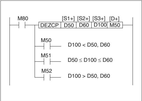
Рис. 7-54: Пример программирования DEZCP-инструкции
