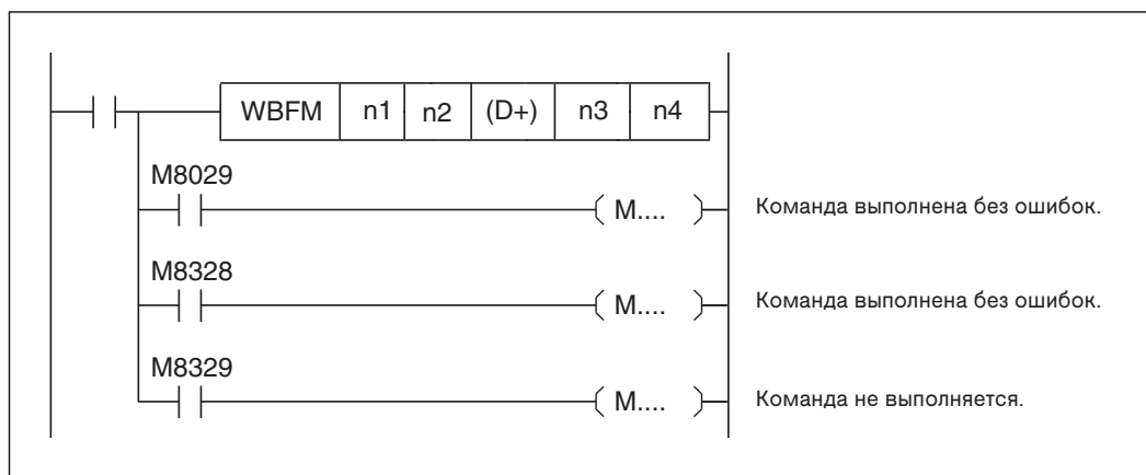
Рис. 7-297: Состояние маркеров M8029, M8328 и M8329 необходимо проверять сразу после команды WBFM.
