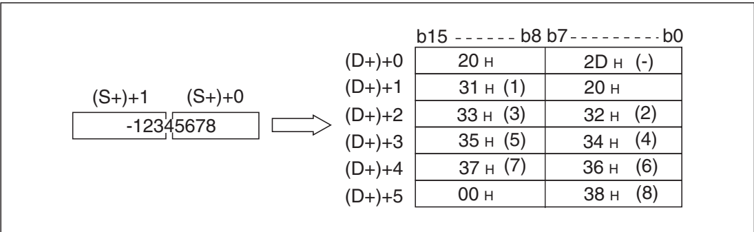
Рис. 7-288: Число „-12345678” преобразуется с помощью команды DBINDA в ASCII-код. Специальный маркер M8091 в этом примере не установлен.
