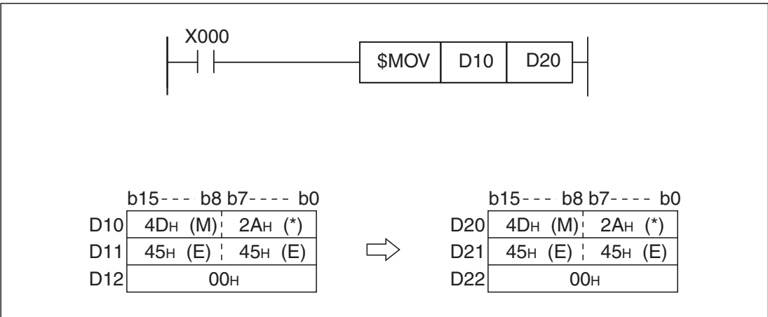
Рис. 7-245: Пример программы для применения команды $MOV
