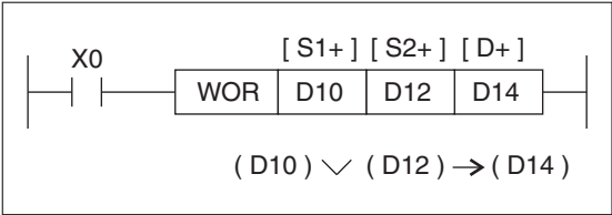
Рис. 6-50: Пример программирования WOR-инструкции („ИЛИ”-связи)
