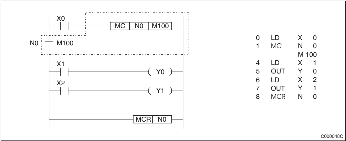
Рис. 4-14: Пример программирования инструкций МС и MCR
