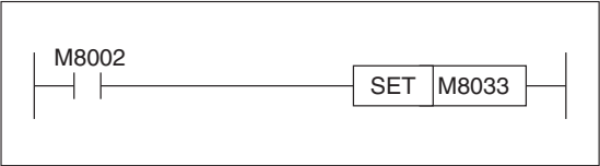
Рис. 8-2: Пример программирования
