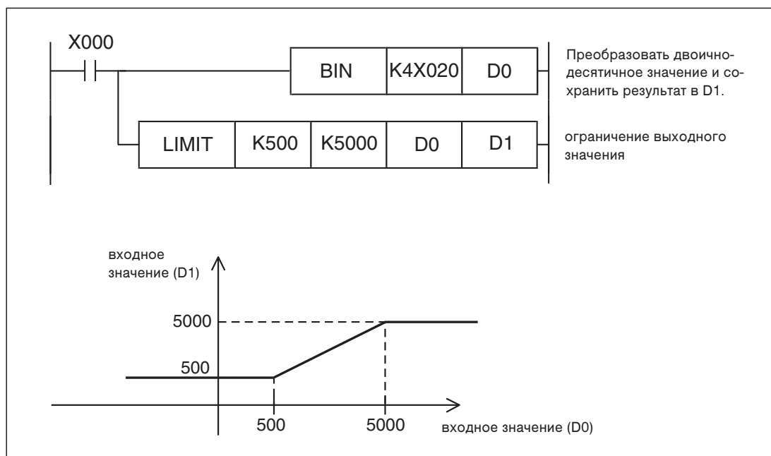
Рис. 7-264: Эта программа ограничивает значение в D1 пределами 500 и 5000.
