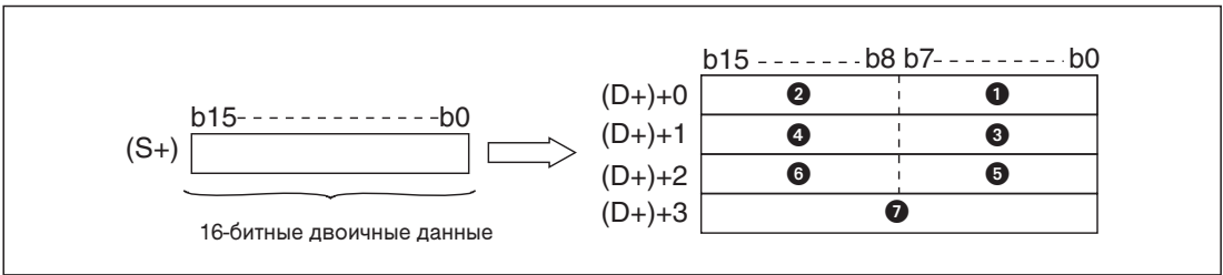
Рис. 7-285: Команда BINDA преобразует двоичные данные в число с количеством разрядов до 5.
