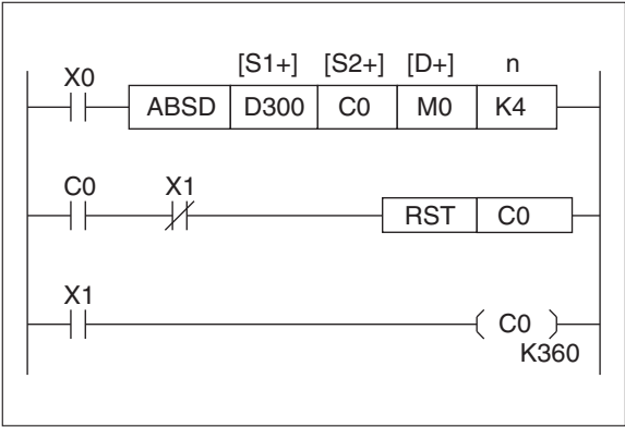
Рис. 6-110: Пример программирования ABSD-инструкции
