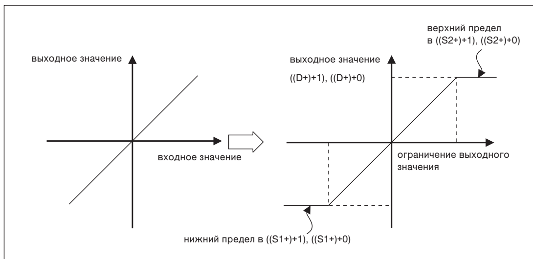
Рис. 7-263: Взаимосвязь между входным и выходным значением без ограничения (слева) и с ограничением (справа) с помощью команды LIMIT
