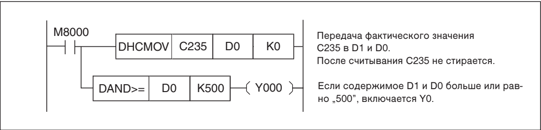
Рис. 7-189: Пример выполнения команды DHCMOV в циклической программе
