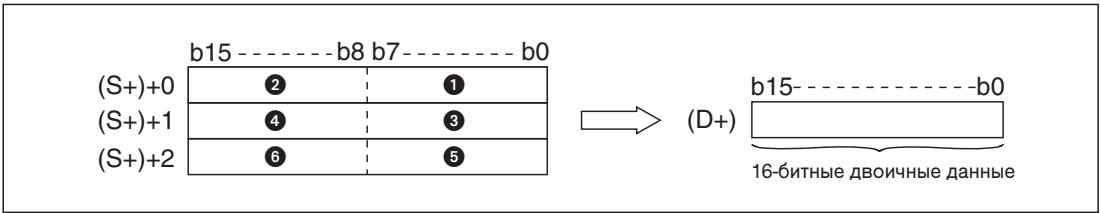
Рис. 7-280: Команда DABIN преобразует число, имеющее до 5 разрядов, в двоичные данные.
