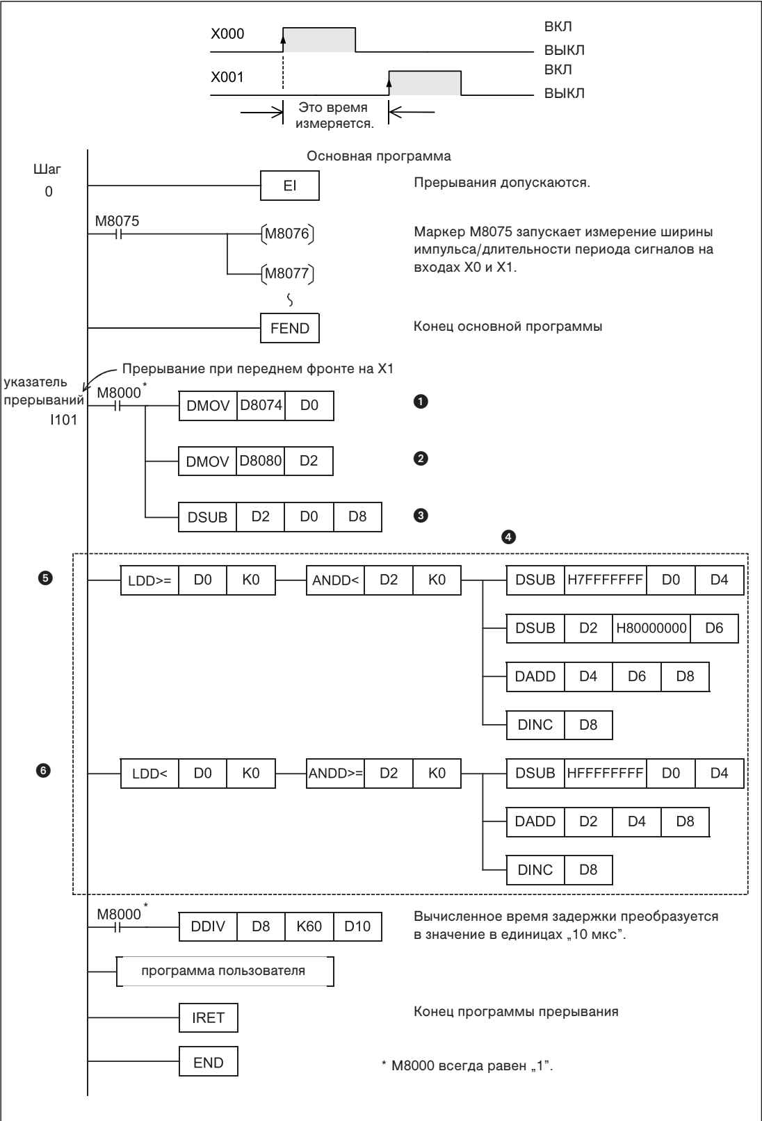
Рис. 8-10: Пример измерения задержки при включении двух входов
