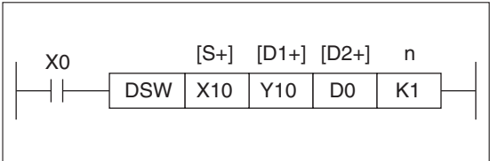
Рис. 7-7: Пример программирования DSW-инструкции
