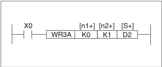
Рис. 7-167: Пример программирования WR3A-инструкции
