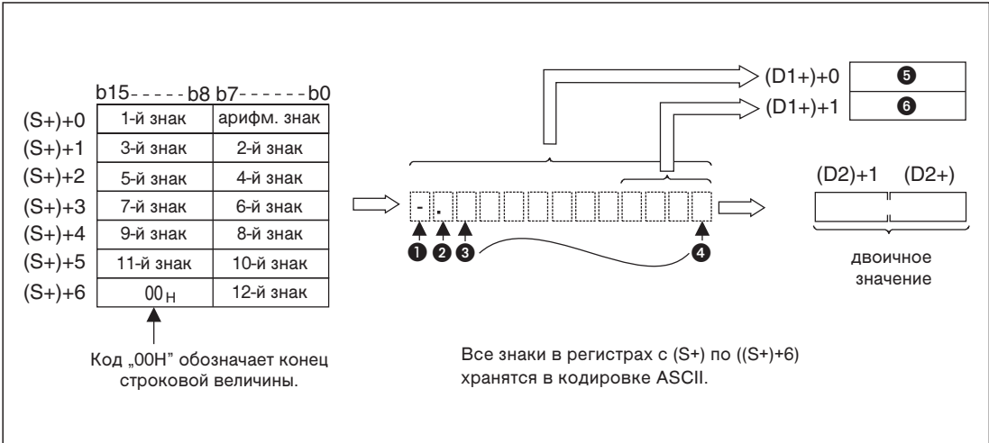
Рис. 7-218: Принцип преобразования строкового числа в 32-битовое двоичное значение с помощью команды DVAL или DVALP
