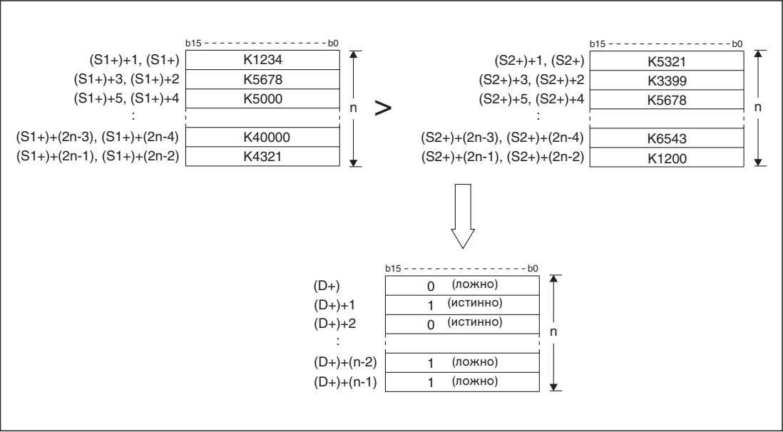
Рис. 7-203: Сравнение содержимых двух блоков данных на „больше” (DBKCMR>)
