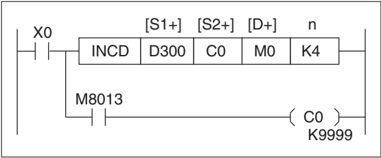
Рис. 6-112: Пример программирования INCD-инструкции
