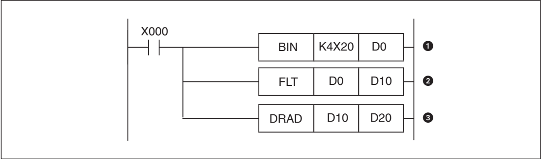
Рис. 7-106: Пример программы для применения команды DRAD
