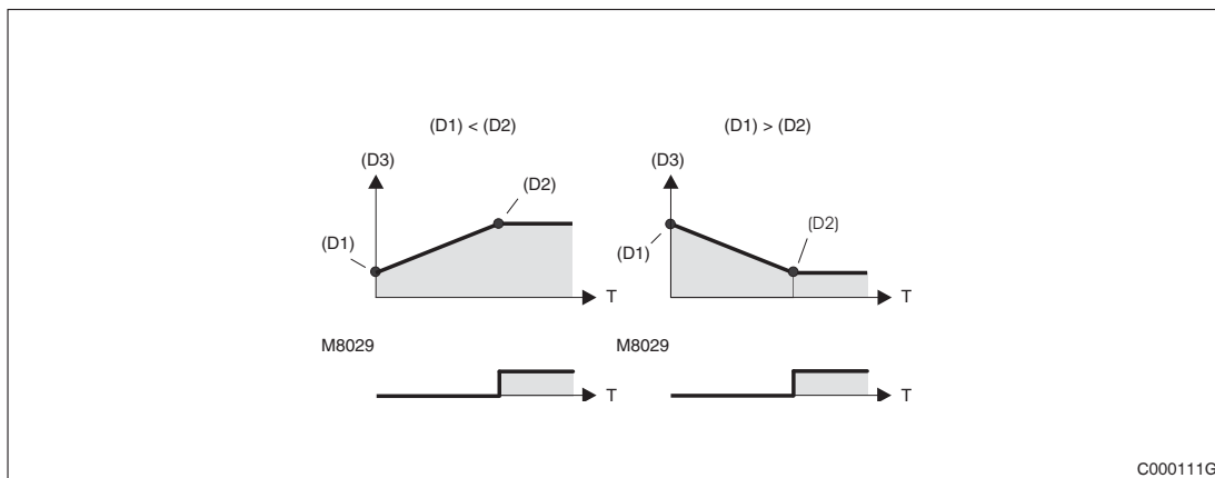
Рис. 6-121: Временные процессы этой схемы
