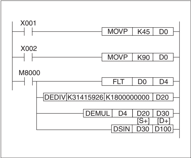
Рис. 7-96: Пример программирования DSIN-инструкции с преобразованием в радианы
