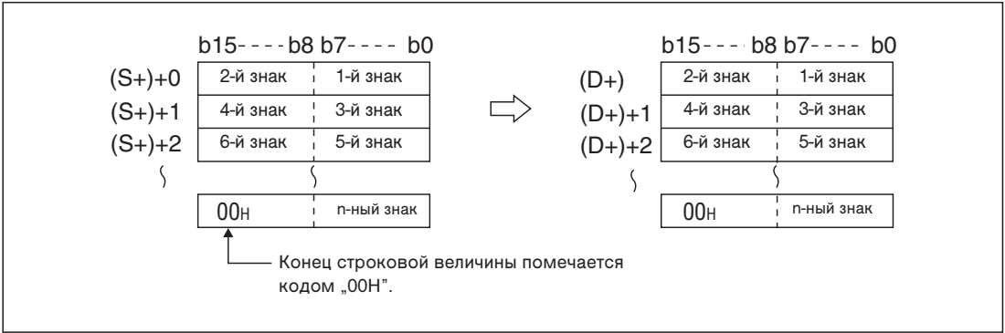
Рис. 7-242: Принцип передачи данных с помощью команды $MOV
