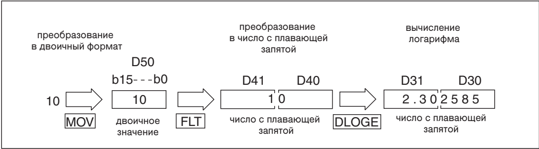
Рис. 7-89: Обработка данных в этом примере программы
