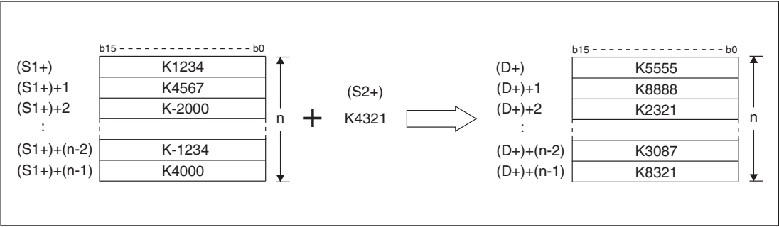
Рис. 7-192: Прибавление константы к содержимому блока данных
