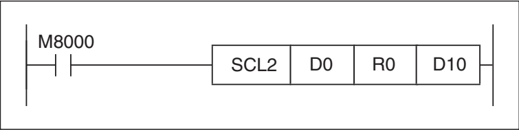
Рис. 7-293: Пример программы для команды SCL
