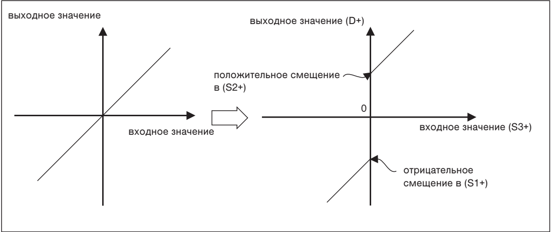
Рис. 7-270: Взаимосвязь между входным и выходным значением без ограничения (слева) и с ограничением (справа) командой ZONE
