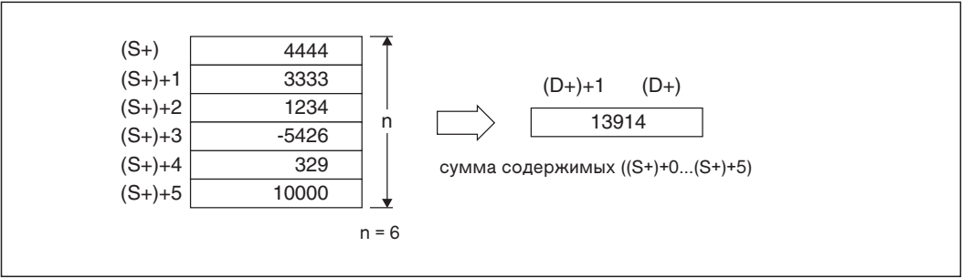
Рис. 7-111: Пример выполнения команды WSUM для суммирования 16-битных данных
