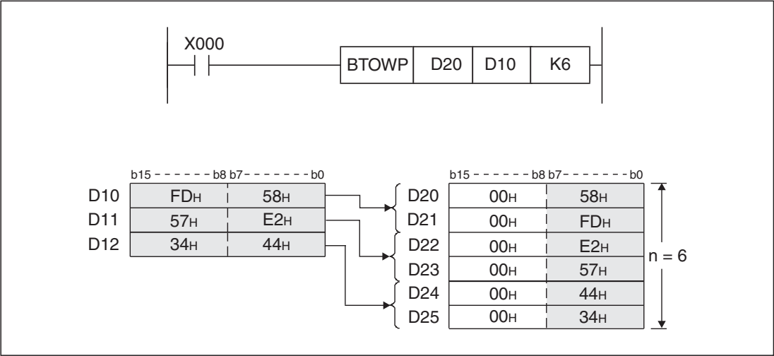
Рис. 7-117: Пример разделения данных с помощью команды WTOBP
