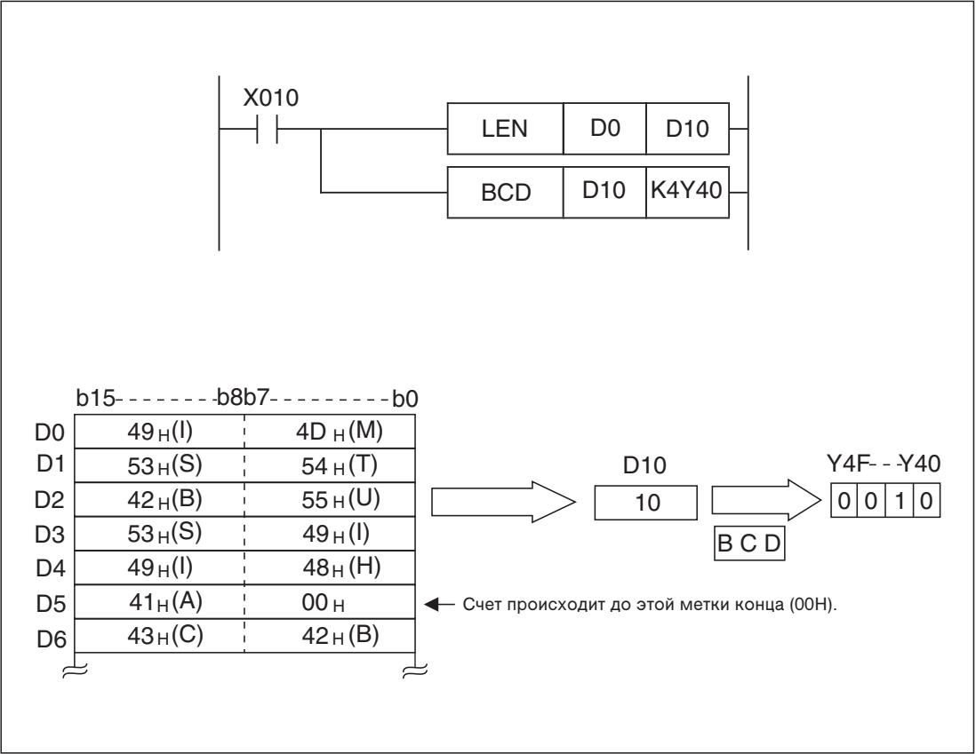
Рис. 7-225: В этом примере подсчитывается число знаков в слове „MITSUBISHI”.
