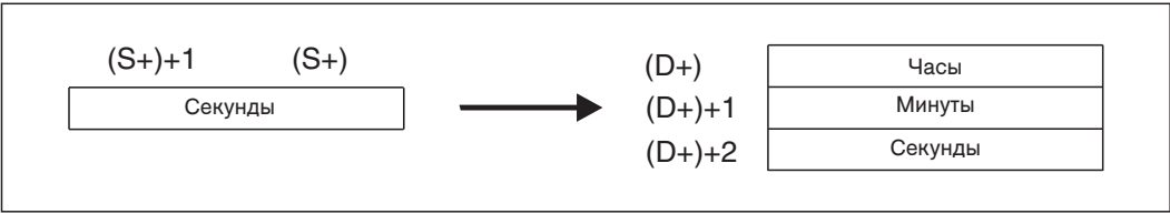
Рис. 7-156: Принцип действия команды DSTOH
