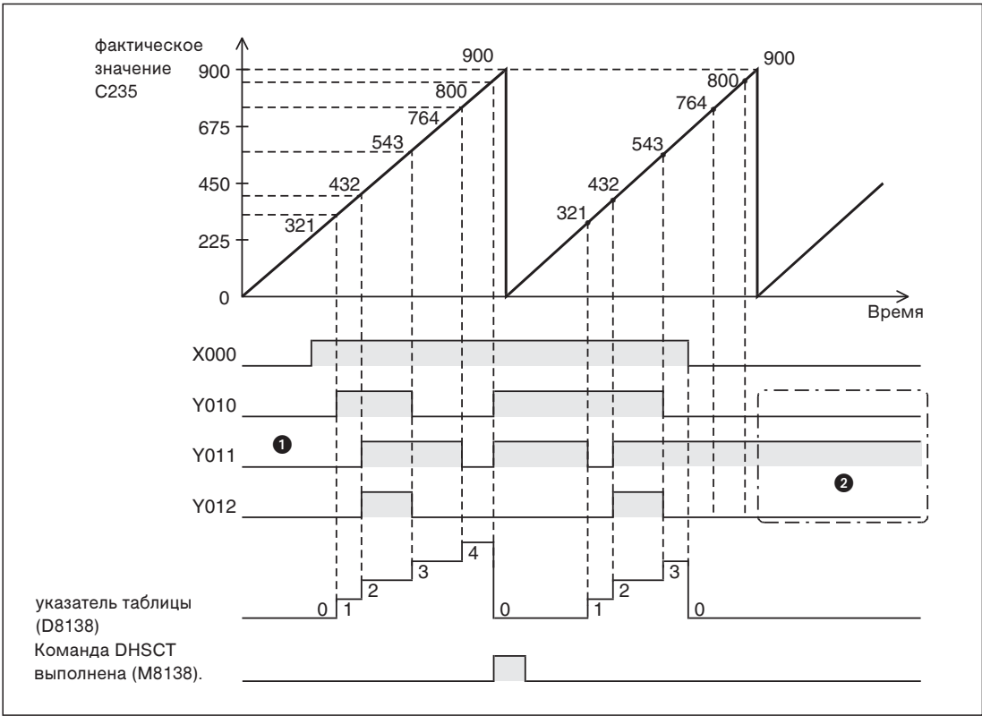
Рис. 7-302: Изменения сигналов для этого примера программы
