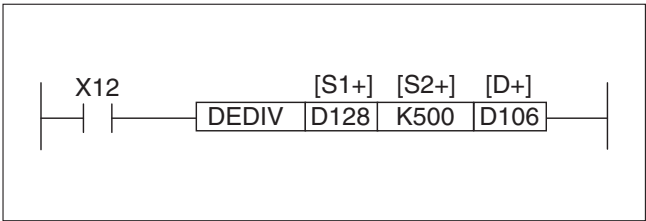
Рис. 7-83: Пример программирования DEDIV-инструкции
