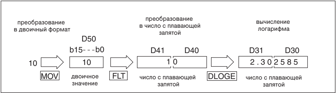
Рис. 7-92: Обработка данных в этом примере программы
