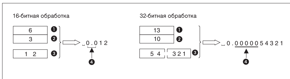
Рис. 7-208: Автоматическое вставление нулей
