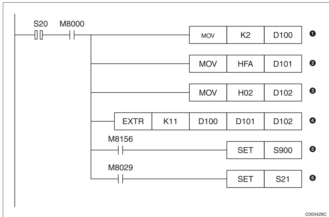
Рис. 7-178: Пример с вызовом функции EXTR в пошаговой программе
