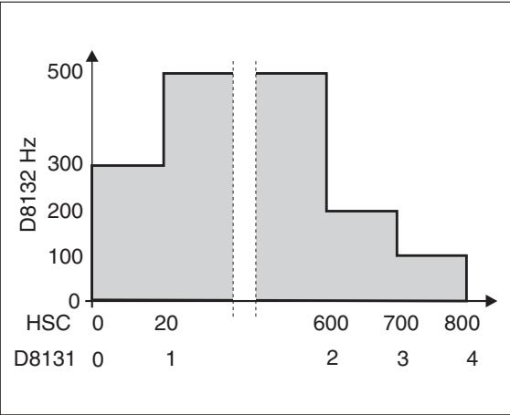
Рис. 6-95. Изменение частоты при применении DHSZ-инструкции со специальным маркером M8132
