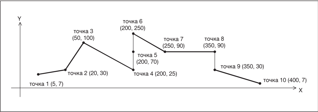
Рис. 7-292: Пример конфигурации кривой
