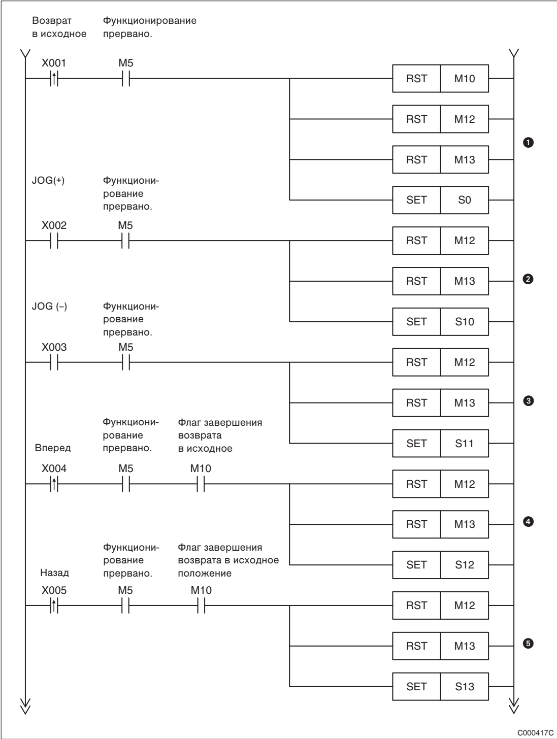
Рис. 7-133: Пример программы
