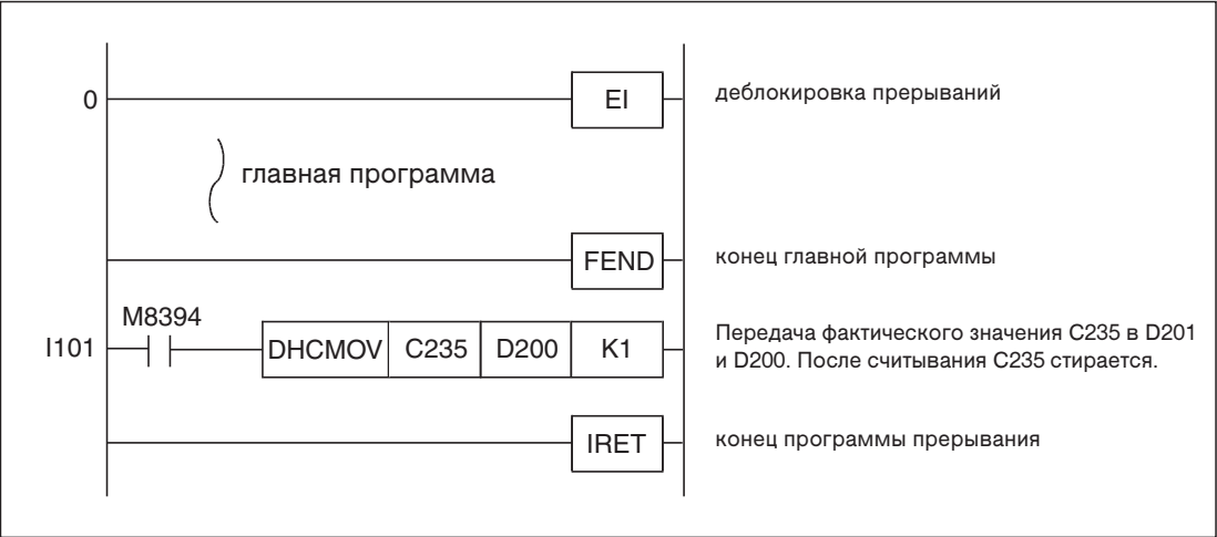
Рис. 7-190: Пример выполнения команды DHCMOV в программе прерывания
