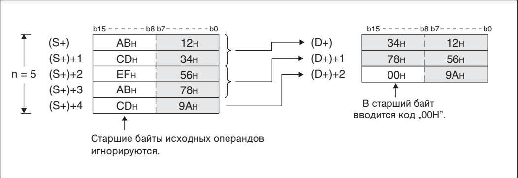
Рис. 7-119: Например, если в (n) указано „5”, данные вводятся от (D+) до младшего байта ((D+)+2), а старший байт ((D+)+2) стирается.
