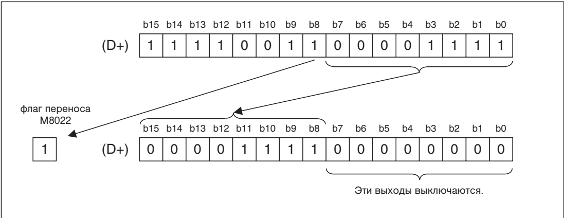
Рис. 7-256: При n = 8 данные смещаются влево на 8 позиций
