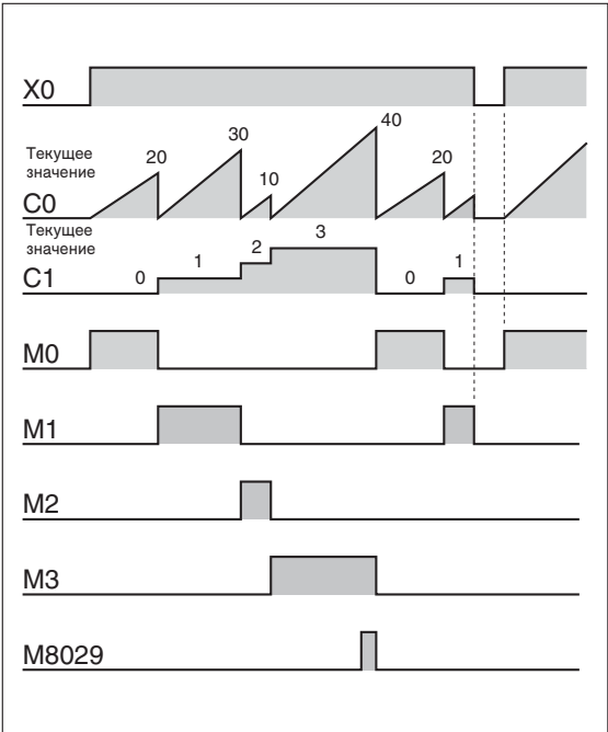
Рис. 6-113: Временная характеристика соответствует рассмотренному выше примеру включения и отключения маркеров.
