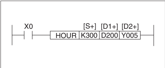
Рис. 7-162: Пример программирования HOUR-инструкции
