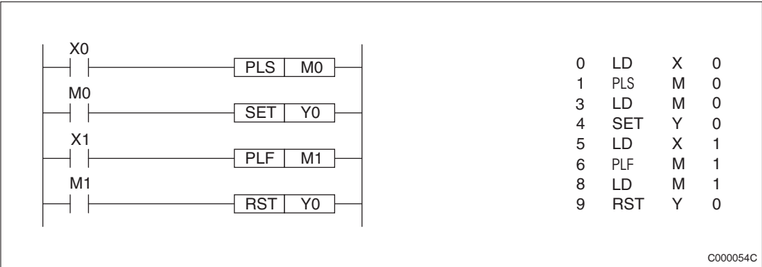
Рис. 4-18: Пример программирования инструкций PLS и PLF
