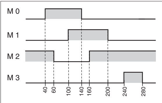
Рис. 6-111: Временная характеристика включения/отключения маркеров
