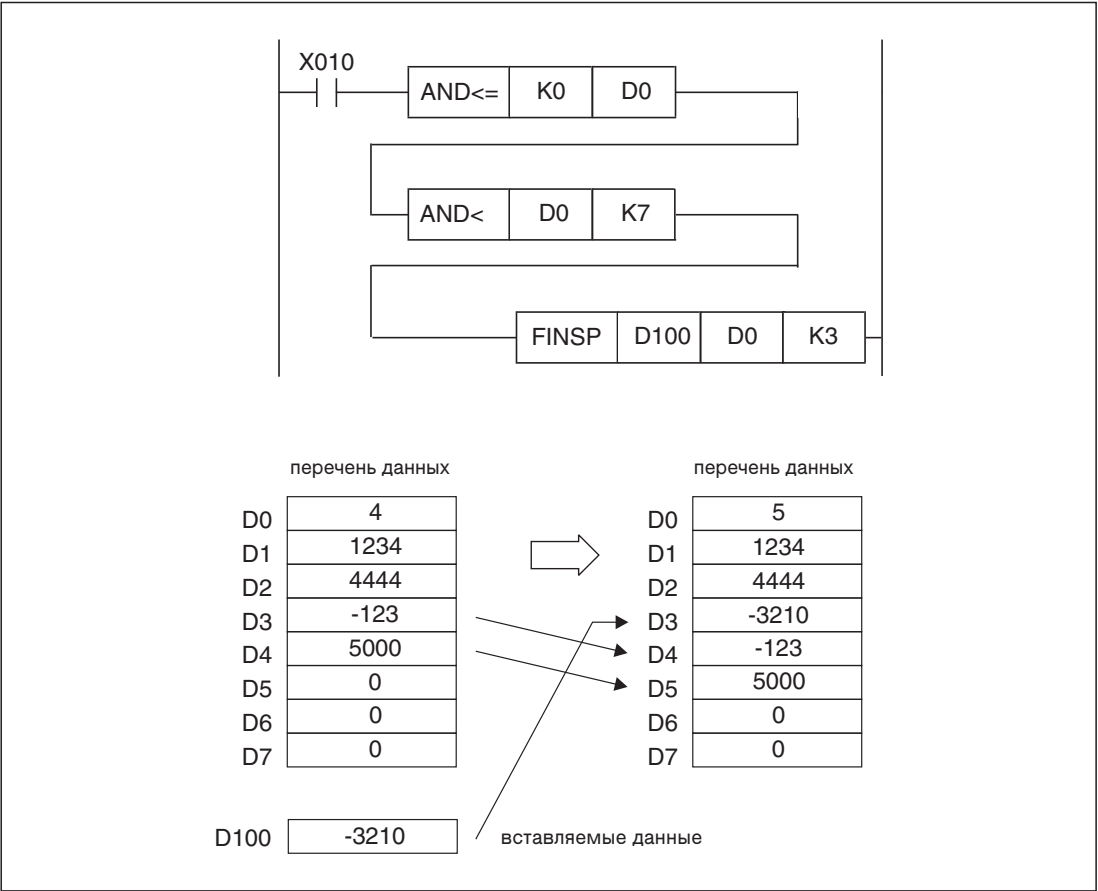
Рис. 7-249: Пример программы для команды FINS
