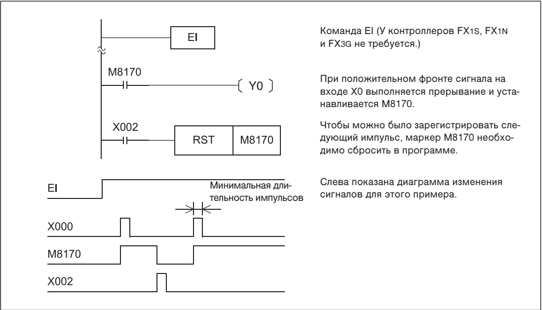
Рис. 8-5: Пример программы и диаграмма изменения сигналов для функции перехвата
