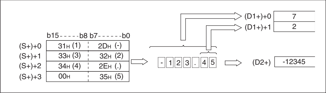
Рис. 7-217: Строковое число „-123.45“ преобразуется в двоичный вид. Результат записывается в (D2+).
