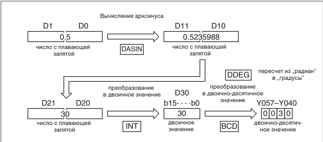
Рис. 7-100: При задании синуса „0.5” вышеприведенная программа выводит угол „30”.
