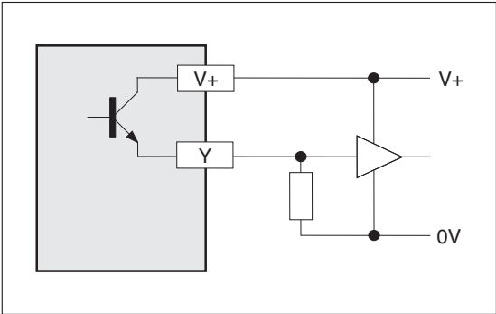
Рис. 7-12: При включенном выходе подключается плюс силового напряжения.
