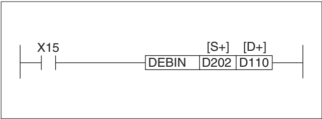
Рис. 7-79: Пример программирования DEBIN-инструкции
