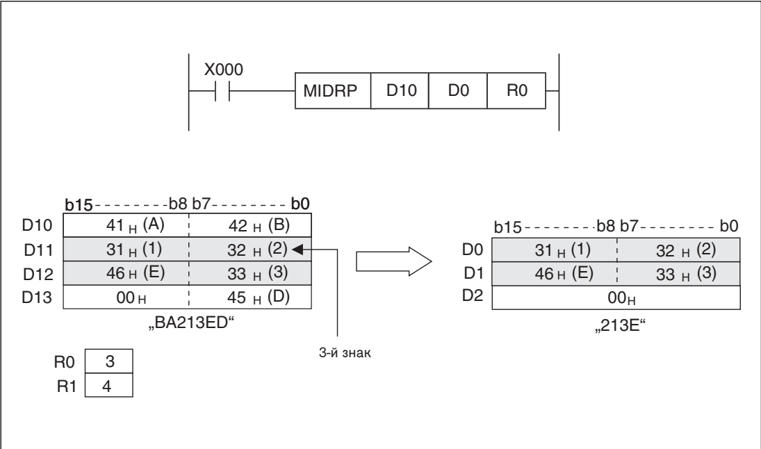
Рис. 7-234: Из строковой величины „BA213ED” копируются знаки „213E”.
