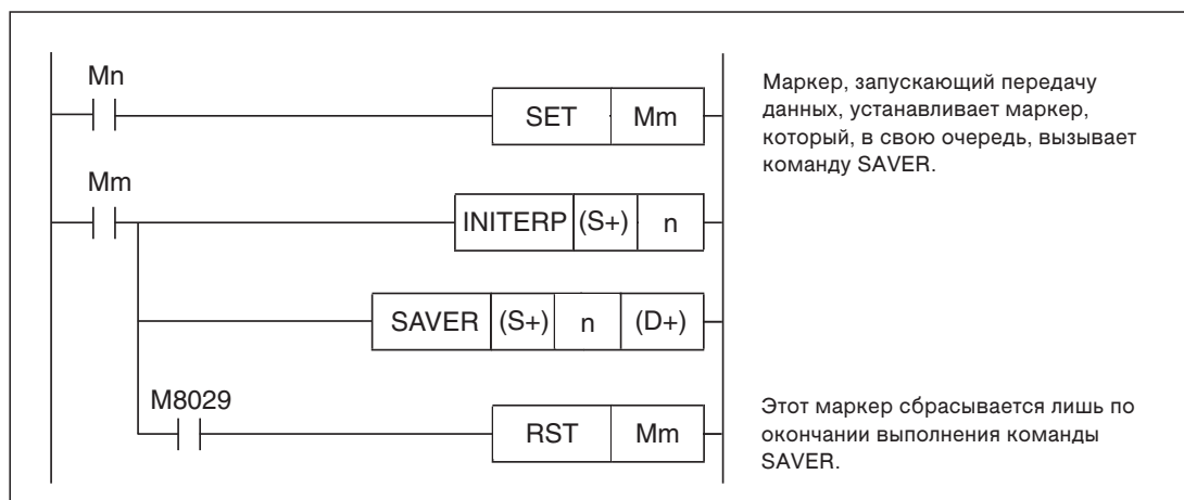
Рис. 7-306: В этом примере программы второй маркер (Mm) предотвращает неполное выполнение команды SAVER после сброса пусковой команды (Mn).
