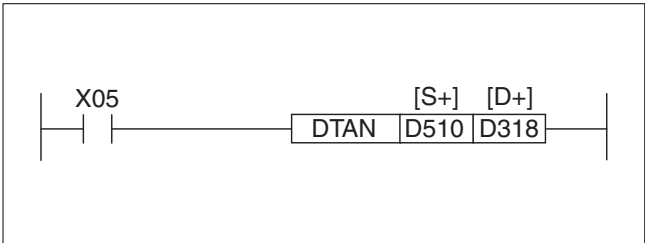
Рис. 7-98: Пример программирования DTAN-инструкции
