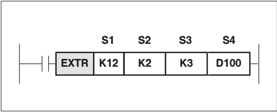
Рис. 7-171: Пример команды EXTR K12
