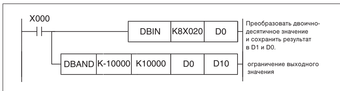
Рис. 7-269: С помощью этой программы все входные значения между -10000 и 10000 не сохраняются в D11 и D10.
