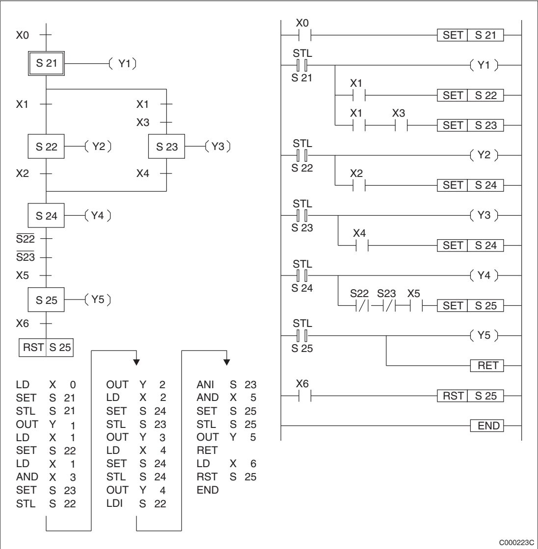
Рис. 5-19: Комбинация из селективного и параллельного разветвления
