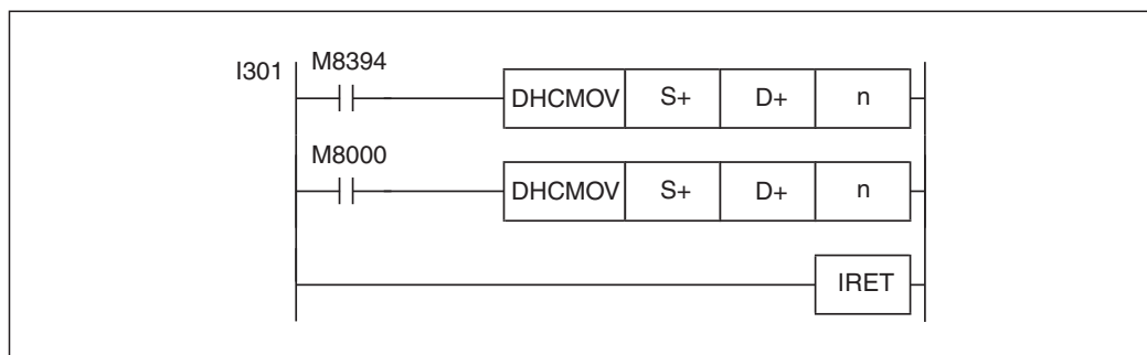
Рис. 7-187: В этом примере из-за указателя прерывания I301 при включении входа X3 сначала выполняется первая команда DHCMOV. Затем обрабатывается вторая команда DHCMOV.
