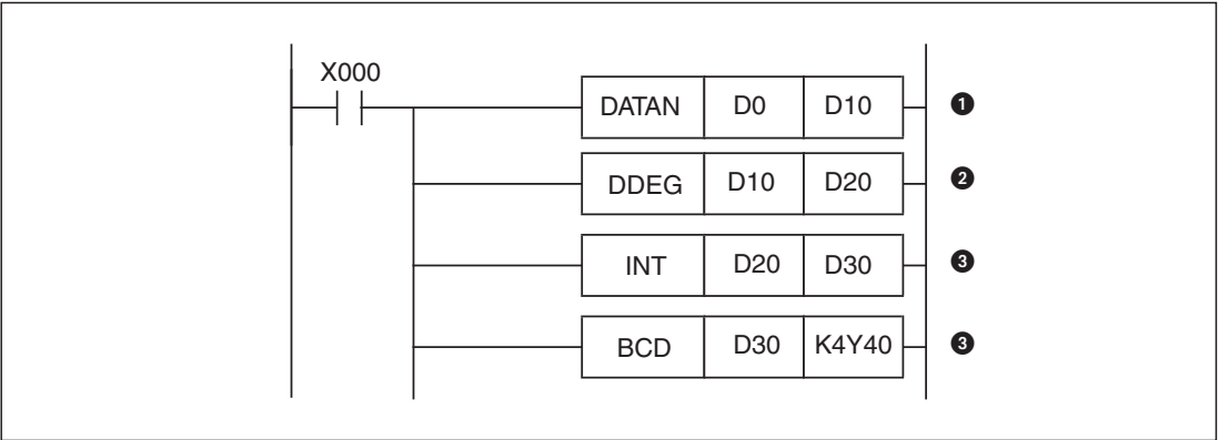
Рис. 7-103: Пример программы для вычисления арктангенса и вывода угла на двоично-десятичный дисплей.
