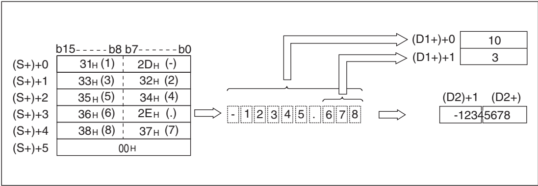
Рис. 7-219: Строковое число „-12345.78” преобразуется в двоичный вид. Результат записывается в ((D2+) + 1) и (D2+).
