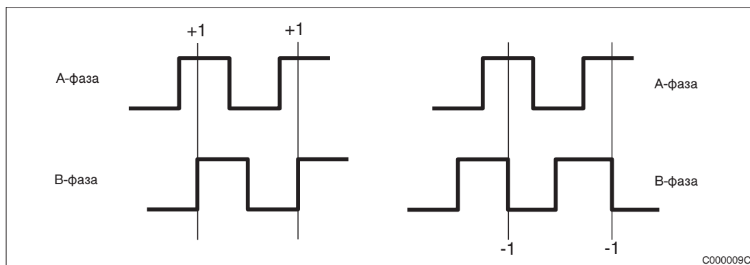
Рис. 3-15: АВ-фазный счетчик
