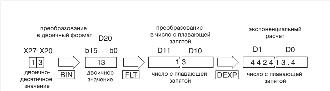
Рис. 7-86: Вышеприведенном примере с помощью двоично-десятичных выключателей введено значение „13”.
