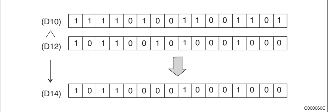
Рис. 6-49: Применение WAND-инструкции
