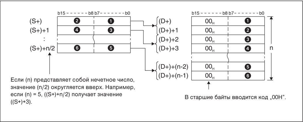
Рис. 7-114: Принцип действия команды WTOB
