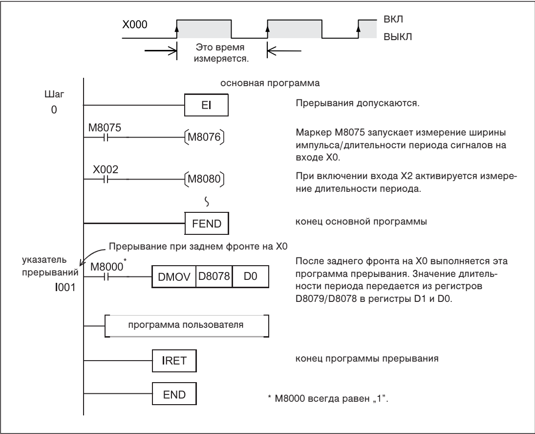
Рис. 8-8: Пример программы для измерения длительности периода сигнала на входе X0
