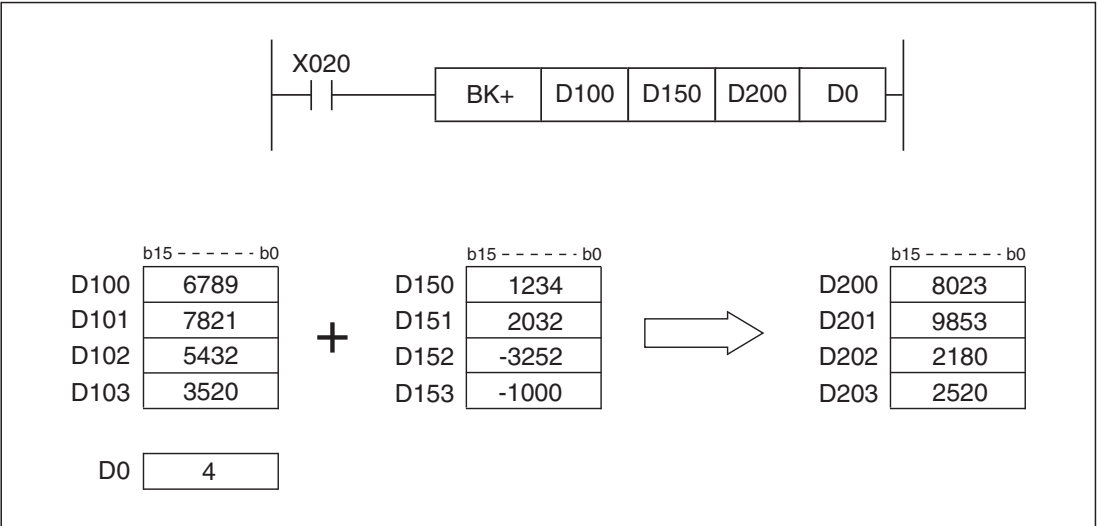
Рис. 7-195: Прибавление константы к содержимому блока данных
