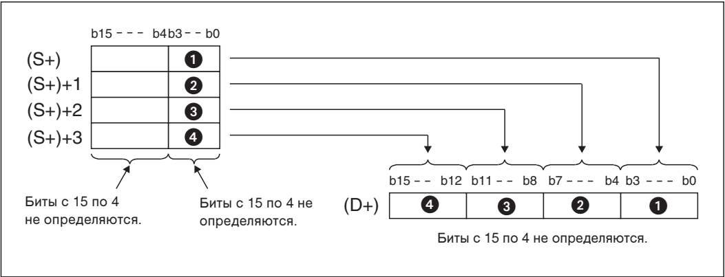
Рис. 7-122: Принцип действия команды UNI
