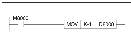
Рис. 8-15: Пример программирования
