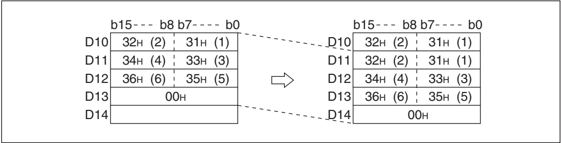
Рис. 7-243: В этом примере содержимое D10 не изменяется.
