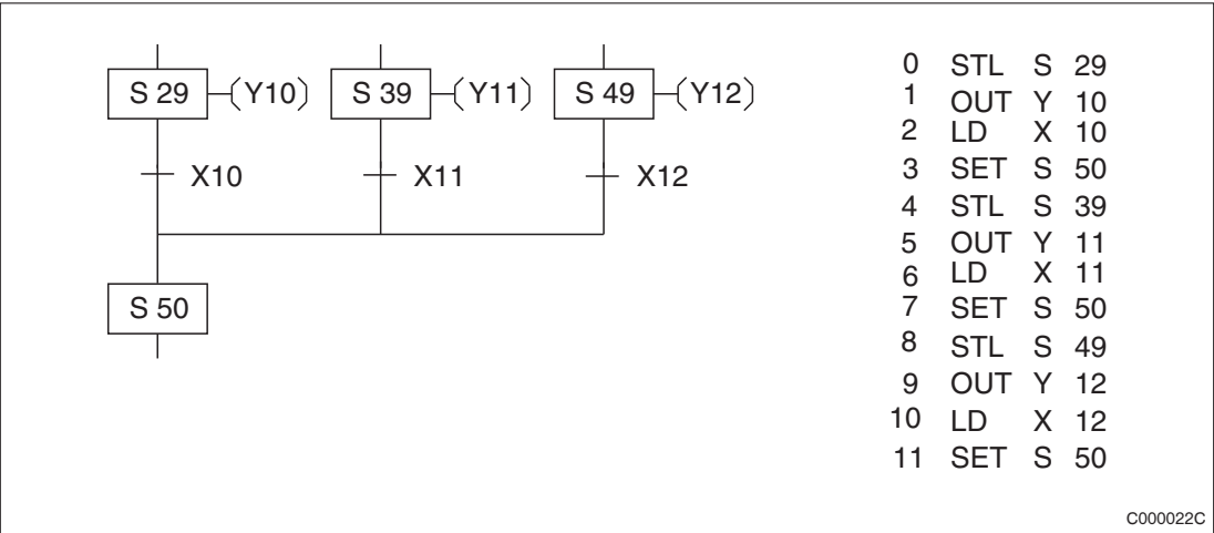
Рис. 5-15: Сборка (окончание) селективного разветвления
