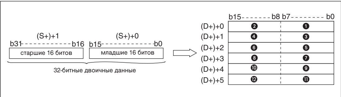
Рис. 7-287: Команда DBINDA преобразует двоичные данные в число с количеством разрядов до 10.
