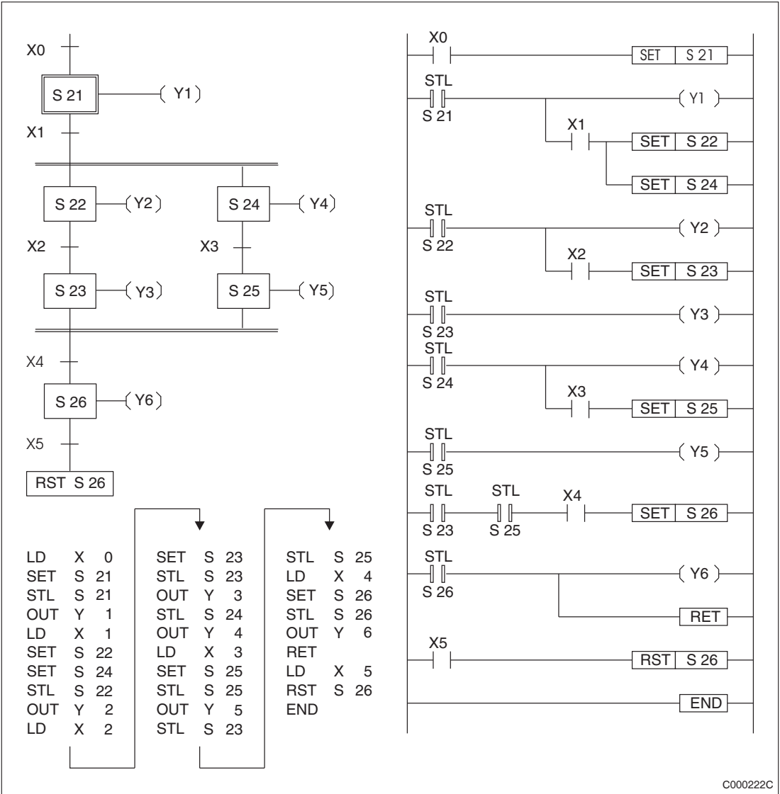
Рис. 5-18: Параллельное разветвление
