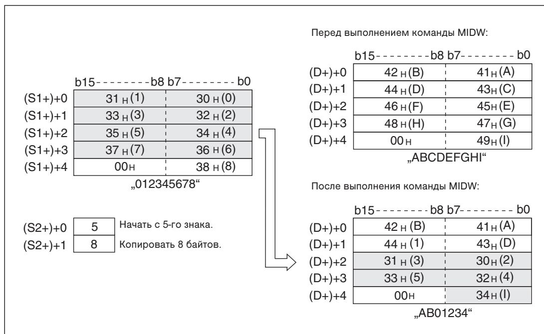
Рис. 7-236: В строковую величину в (D+) вставляются только знаки до кода „00H“. В этом примере требуется, начиная с 5-го знака строковой величины, в (D+) записать 8 знаков. Однако, начиная с 5-го знака, в ((D+)+2) можно заменить только 5 знаков. Остальные знаки строковой величины в (S1+) отрезаются.
