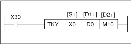
Рис. 7-1: Программирование TKY-инструкции
