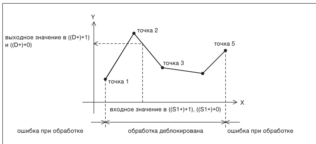
Рис. 7-291: Если входное значение находится вне формы кривой, заданной таблицей, возникает ошибка.
