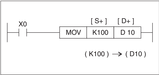
Рис. 6-20: Пример программирования с использованием MOV-инструкции
