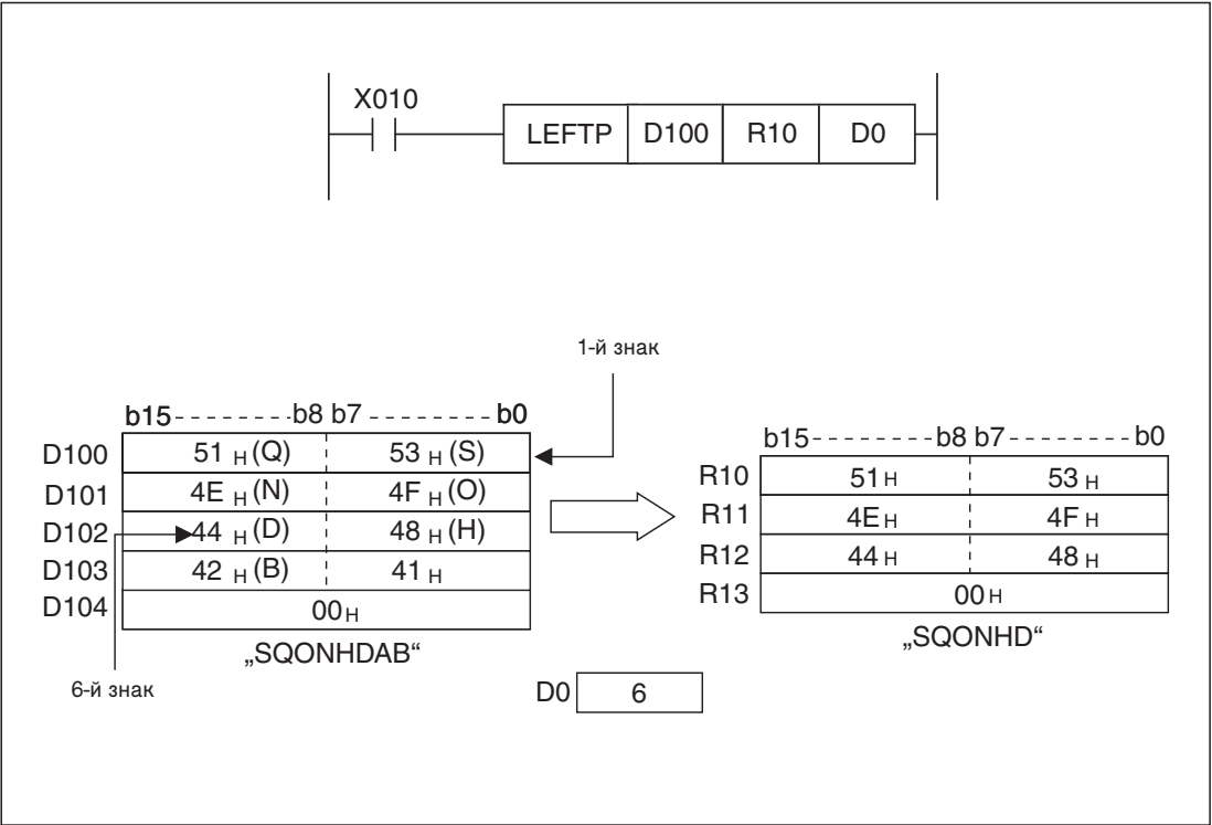
Рис. 7-231: Пример программы применения команды LEFT(P)
