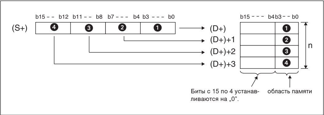
Рис. 7-125: Принцип действия команды DIS
