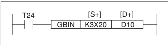
Рис. 7-165: Пример программирования GBIN-инструкции
