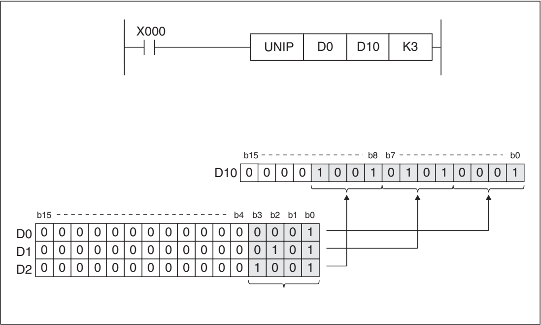
Рис. 7-124: Пример группирования 4-битных данных с помощью команды UNIP
