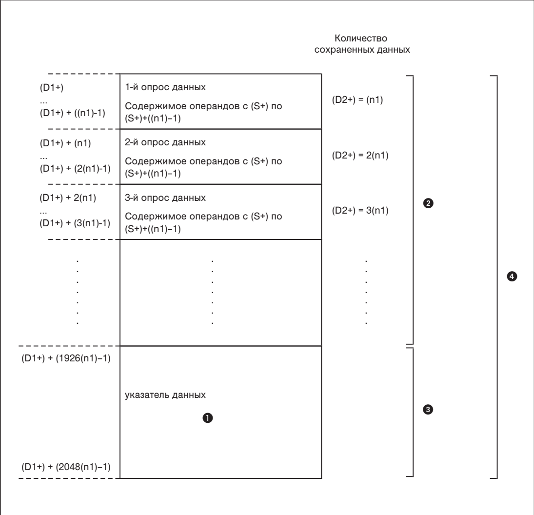
Рис. 7-313: Использование расширенных регистров и расширенных файловых регистров командой LOGR.
