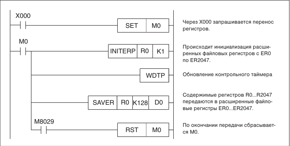
Рис. 7-307: Перед выполнением команды SAVER необходимо с помощью команды INITER инициализировать расширенные файловые регистры.
