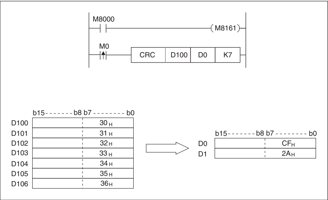
Рис. 7-185: Обработка данных в 8-битном режиме (M8161 установлен)
