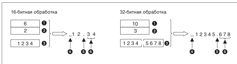
Рис. 7-207: Автоматическое вставление десятичной запятой (в виде точки) и знака пробела
