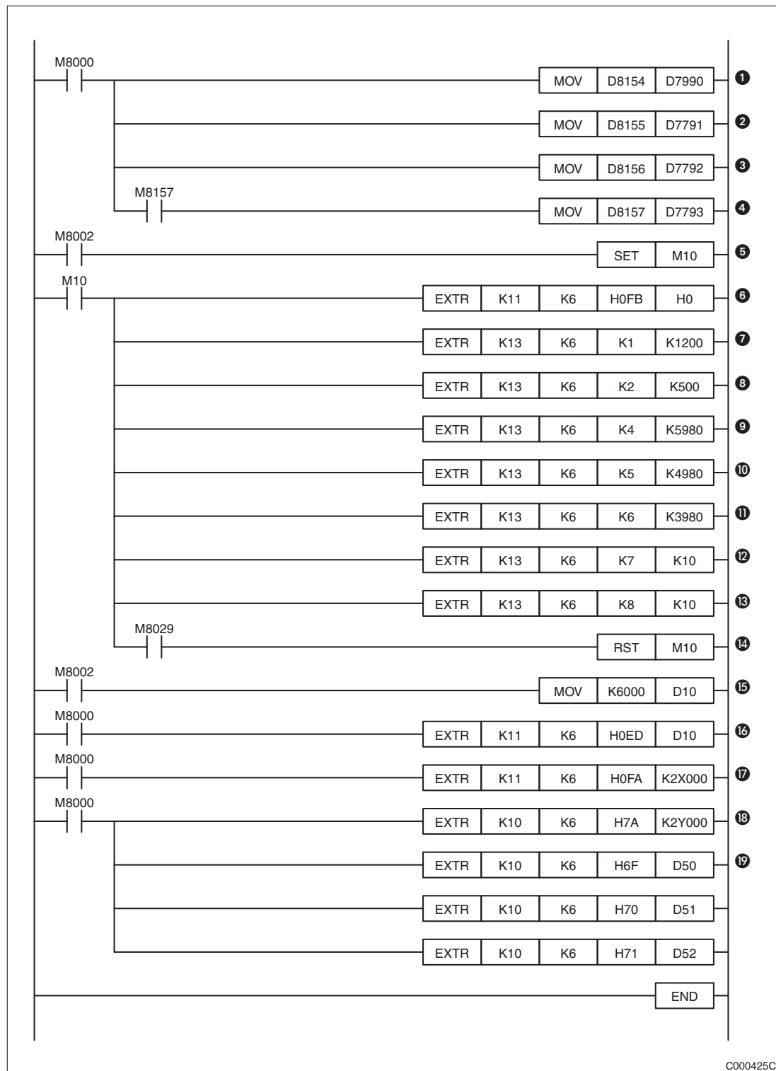
Рис. 7-175: Пример программы по управлению и диагностике преобразователя частоты
