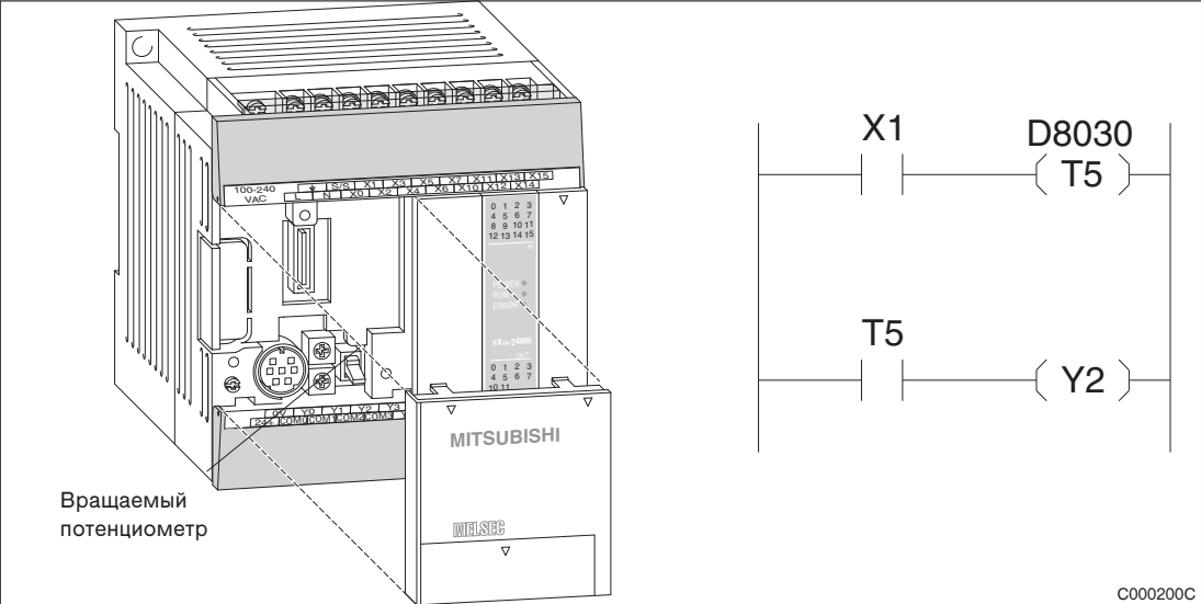
Рис. 3-7: Пример настройки задания уставки времени в базовом блоке FX1N в регистр данных D8030 с помощью потенциометра
