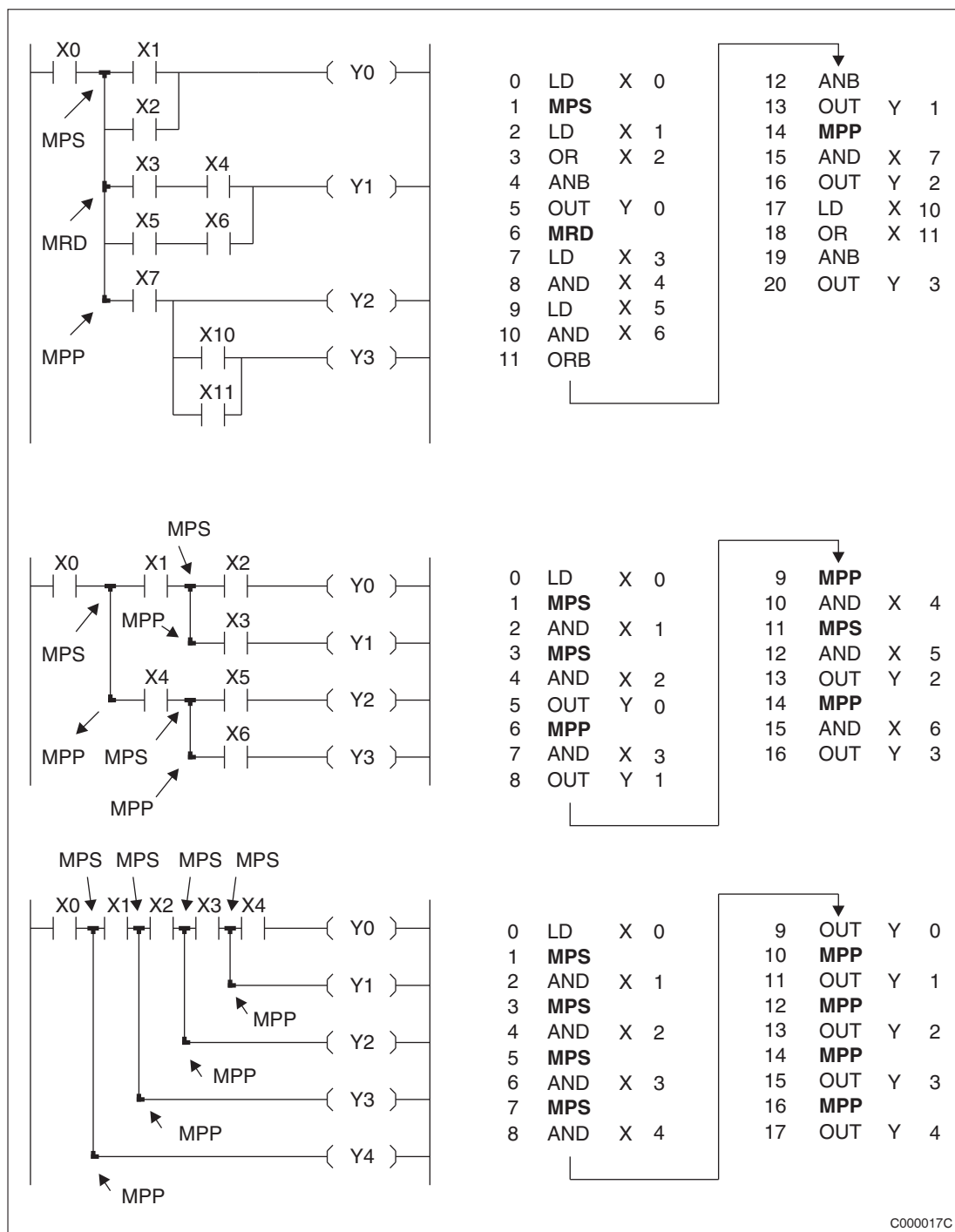
Рис. 4-13: Примеры программирования инструкций MPS, MRD и MPP
