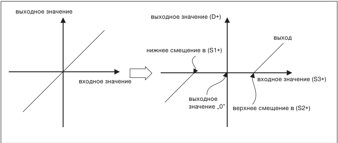
Рис. 7-266: Взаимосвязь между входным и выходным значением без ограничения (слева) и с ограничением (справа) командой BAND
