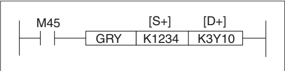
Рис. 7-164: Пример программирования GRY-инструкции
