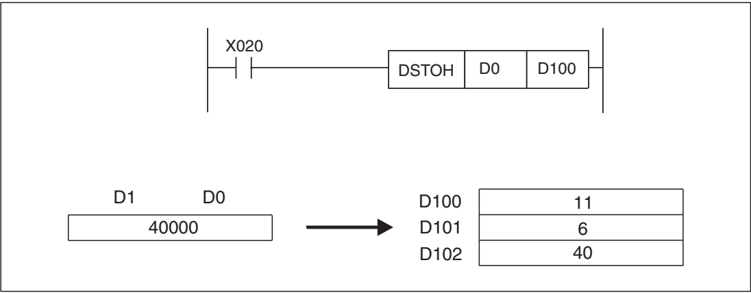
Рис. 7-158: В этом примере регистры D1и D0 содержат значение „40000” [секунд], которое соответствует 11 часам, 6 минутам и 40 секундам.
