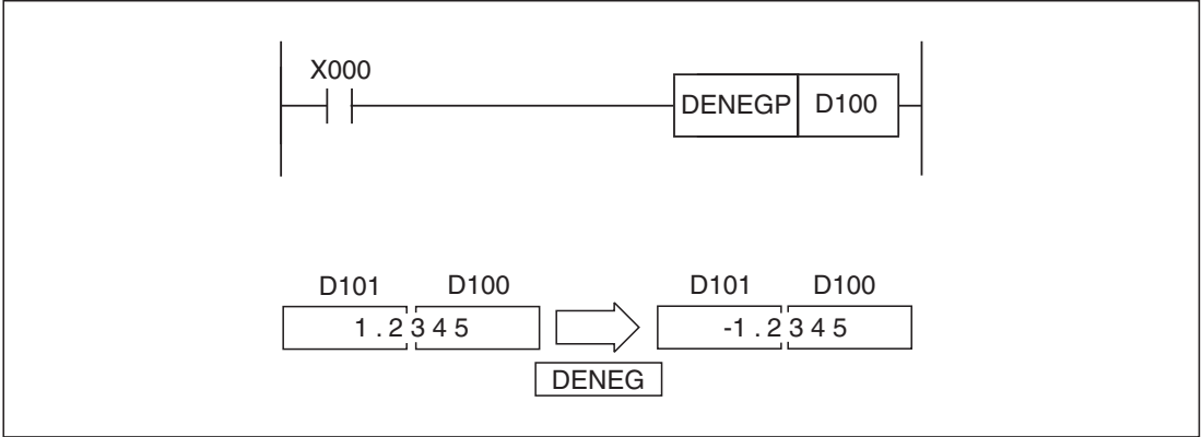
Рис. 7-94: Пример программы для инвертирования арифметического знака с помощью команды DENEG
