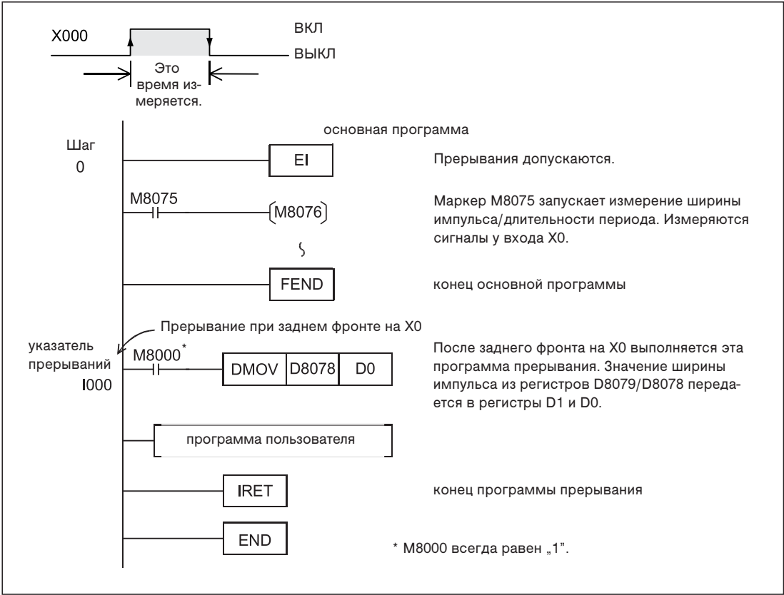
Рис. 8-7: Пример программы для измерения ширины импульса сигнала на входе X0
