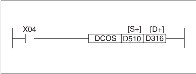
Рис. 7-97: Пример программирования DCOS-инструкции
