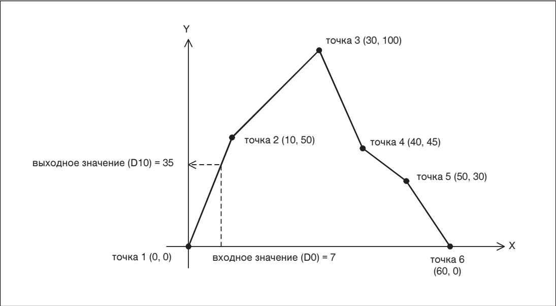
Рис. 7-279: Кривая для масштабирования входного значения в этом примере
