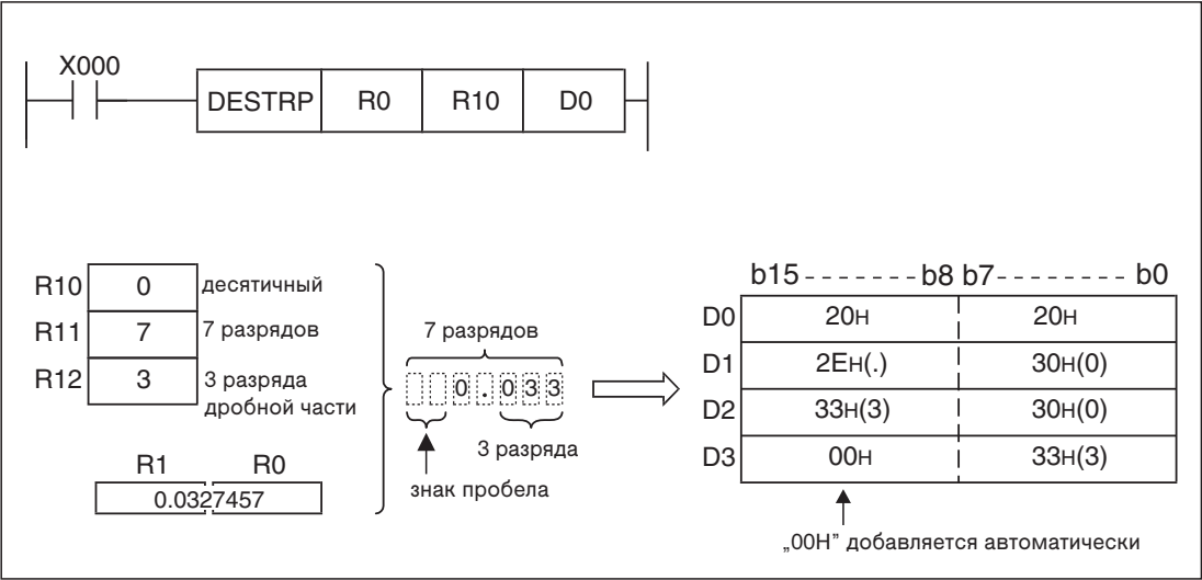
Рис. 7-67: Пример программы для преобразования в десятичное представление
