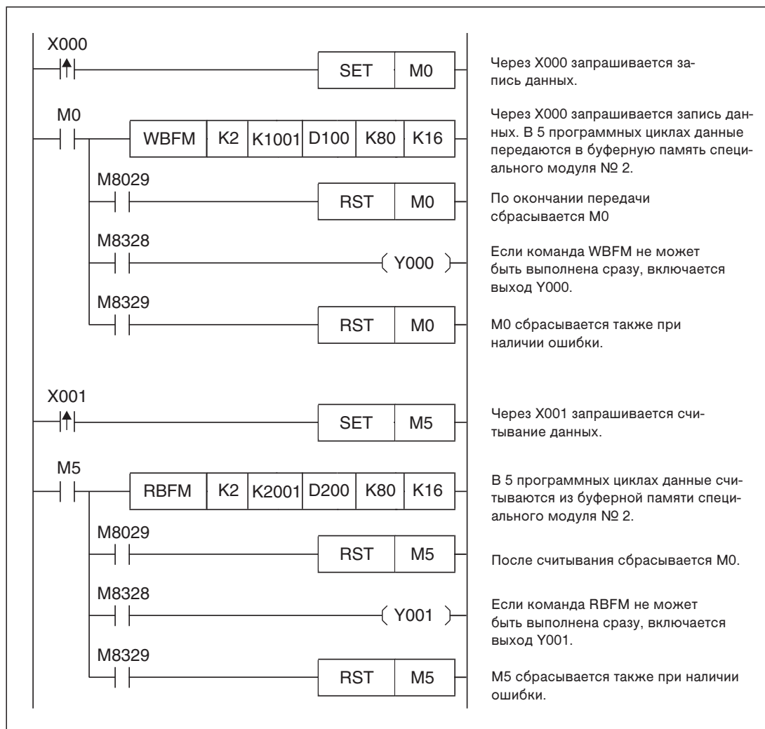
Рис. 7-299: Пример программы для записи 80 слов данных в буферную память специального модуля с адресом 2 и их считывания из этой буферной памяти.
