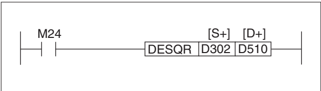
Рис. 7-93: Пример программирования DESQR-инструкции
