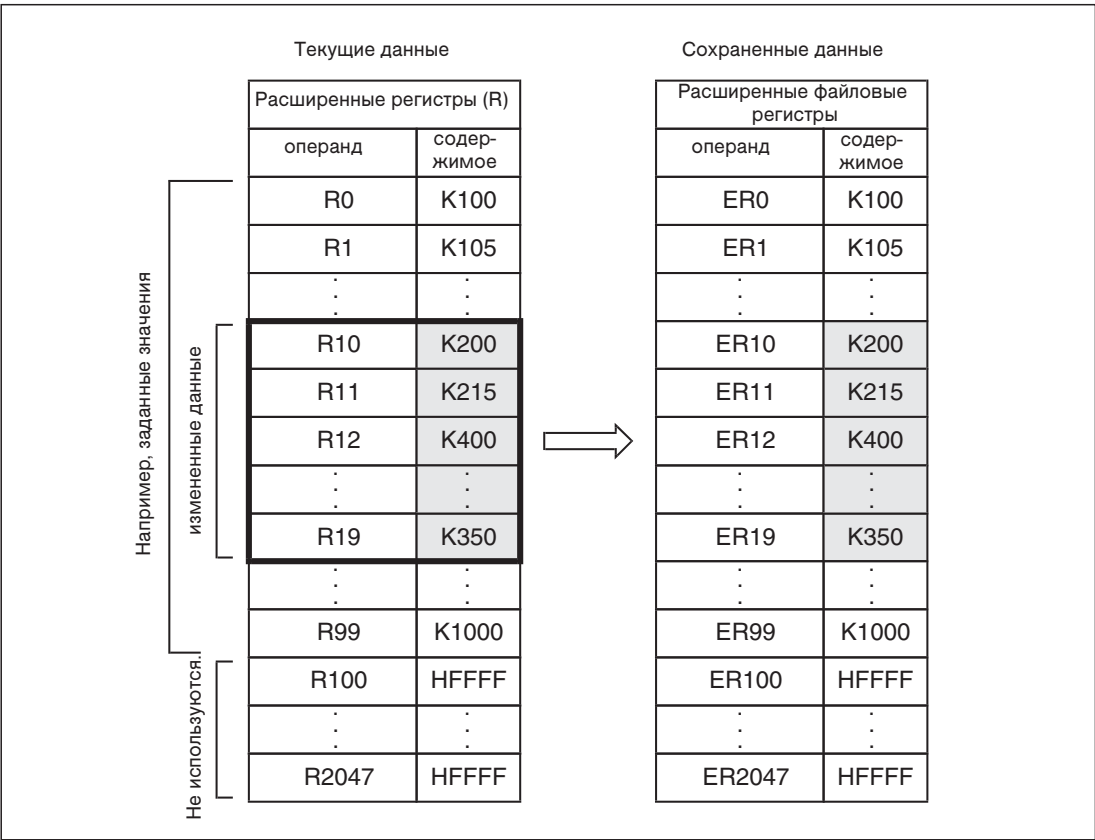
Рис. 7-320: Данные передаются при включении X001.
