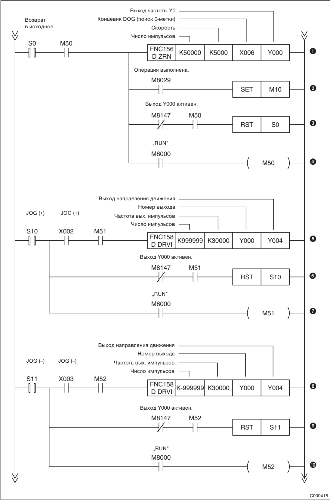
Рис. 7-134: Пример программы
