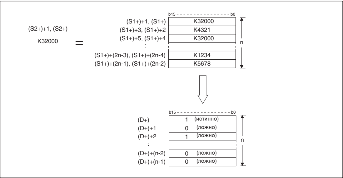
Рис. 7-204: Константа сравнивается с содержимым блока данных на „равно” (DBKCMR=)
