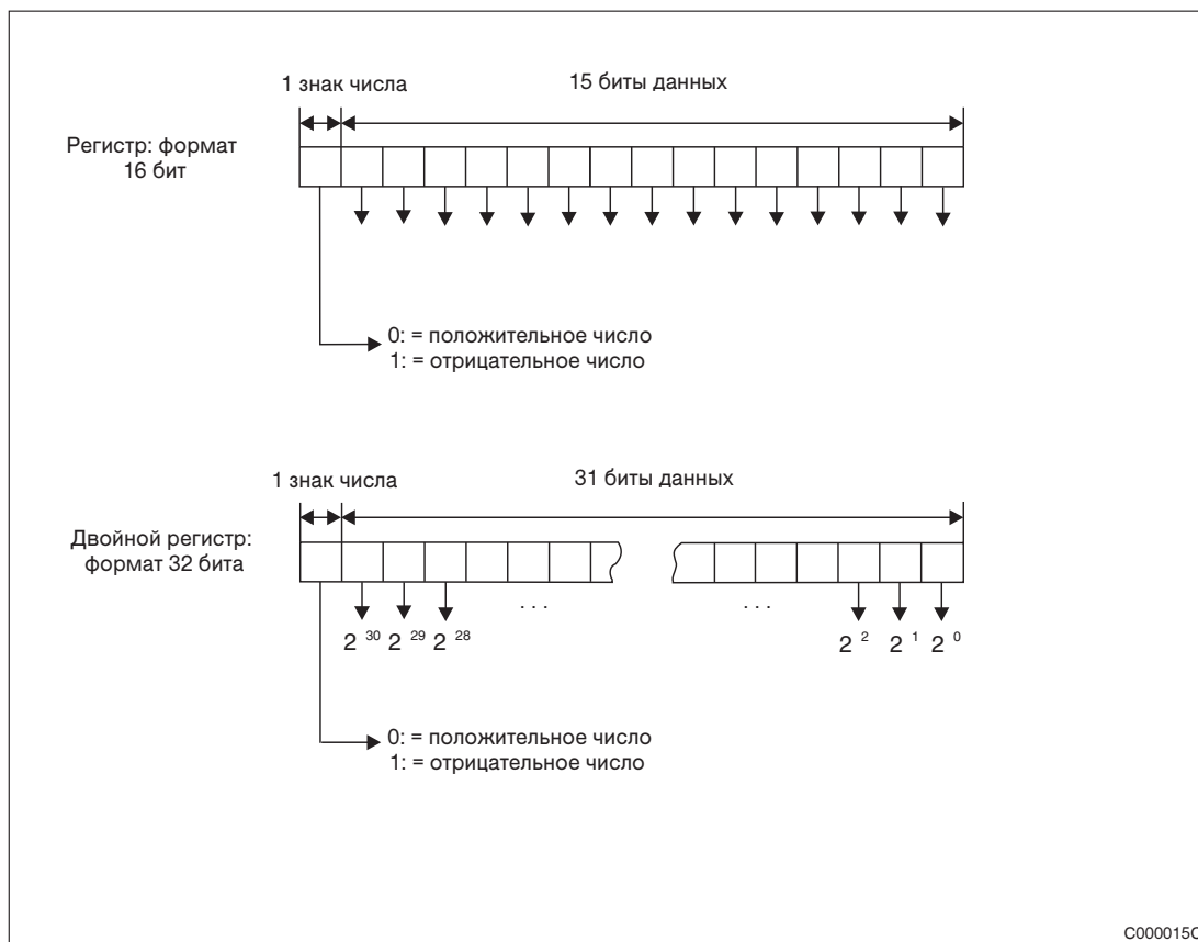
Рис. 3-18: Структура регистра (16 бит) и двойного регистра (32 бита)
