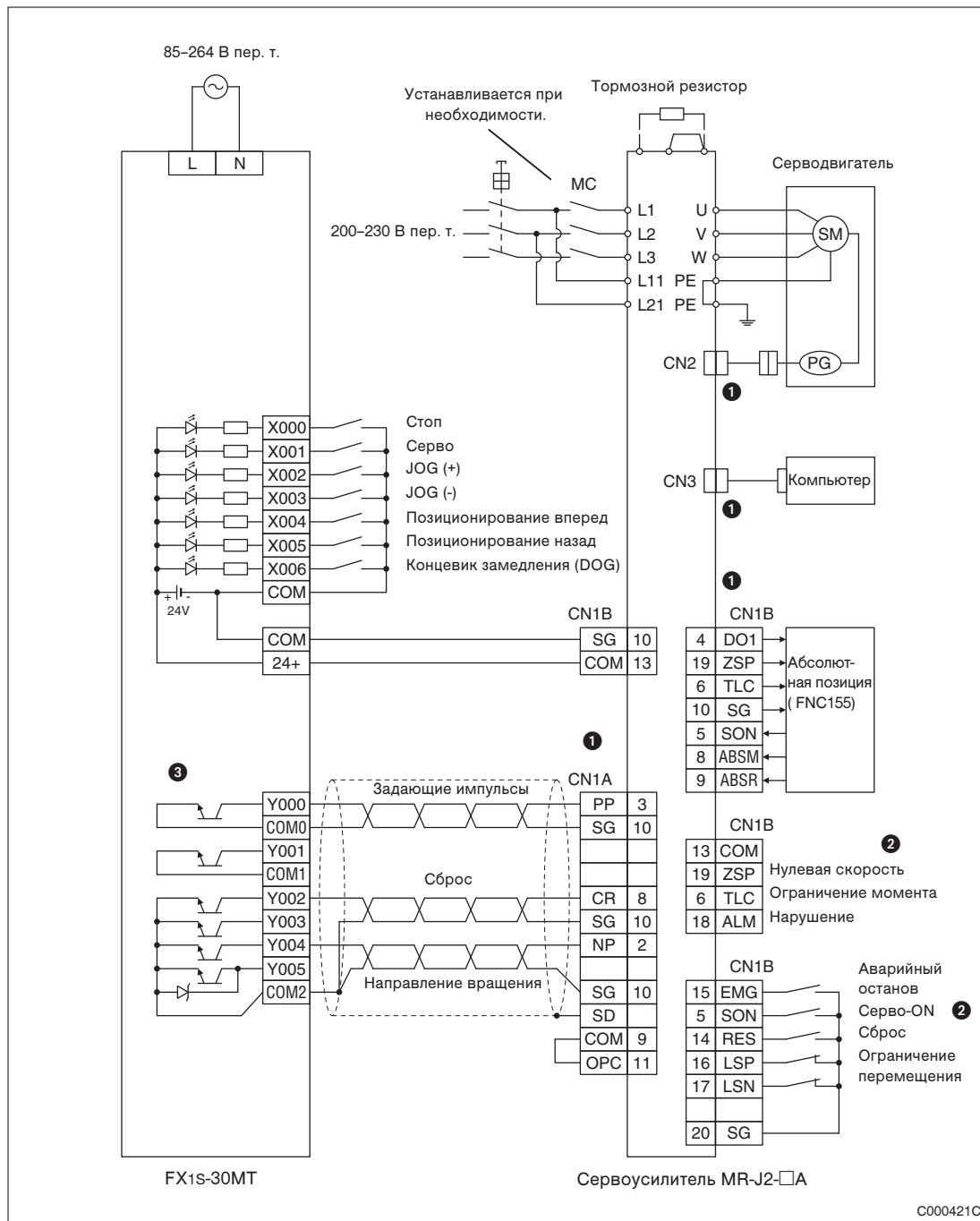
Рис. 7-130: Принципиальная схема
