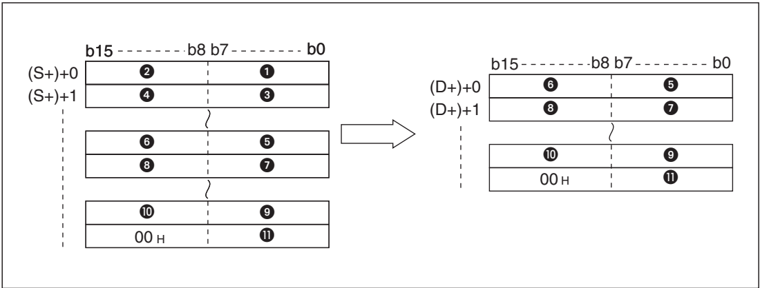
Рис. 7-226: С помощью команды RIGHT считываются знаки, начиная с конца строковой величины.
