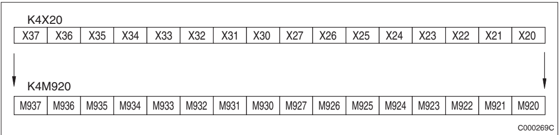
Рис. 7-37: Распределение маркеров
