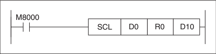
Рис. 7-278: Пример программы для команды SCL
