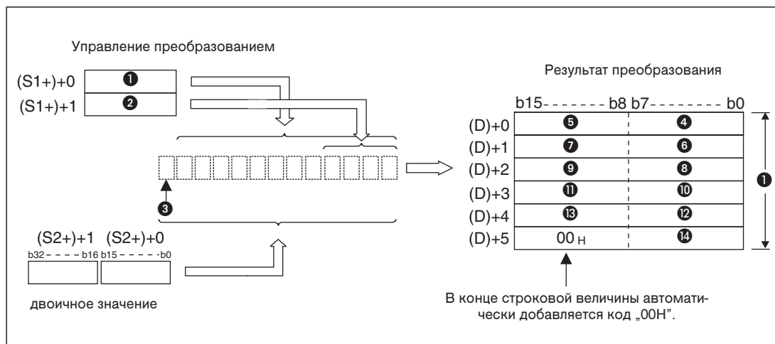
Рис. 7-211: Принцип преобразования 32-битного двоичного значения в строковую величину
