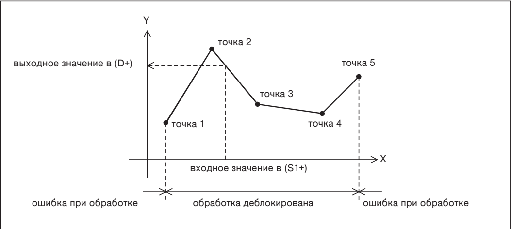
Рис. 7-274: Если входное значение находится вне кривой, заданной таблицей, возникает ошибка.
