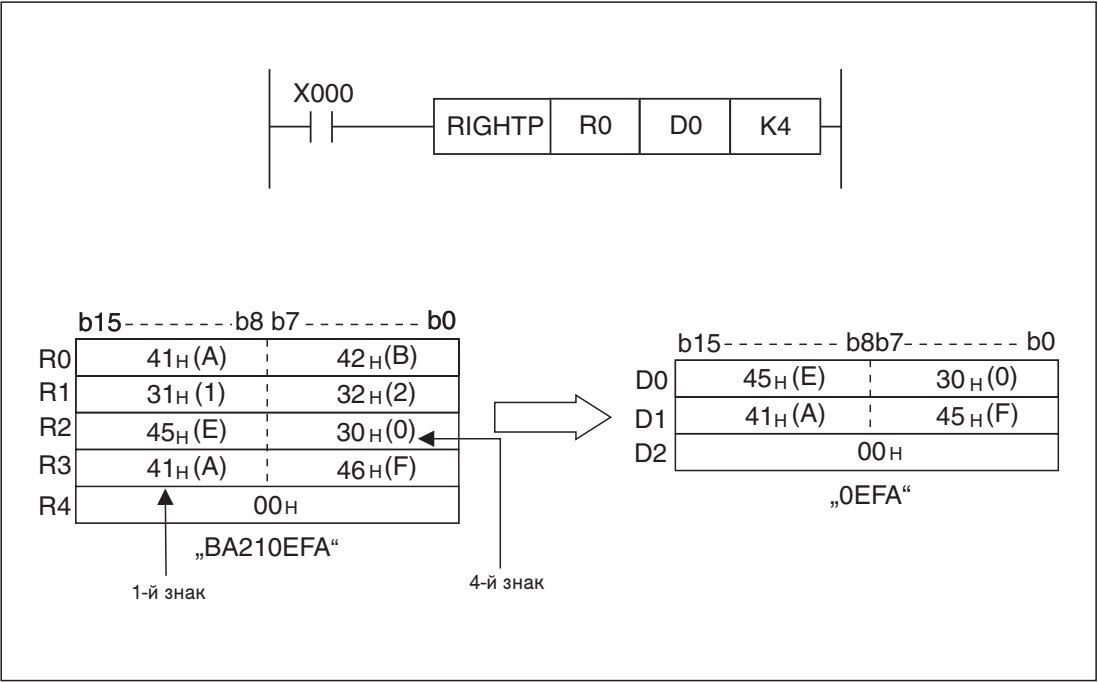
Рис. 7-228: Пример программы применения команды RIGHT(P)
