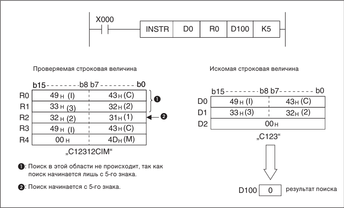
Рис. 7-241: В этом примере искомая цепочка символов не найдена, поэтому результатом поиска является „0”.
