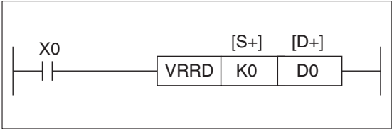
Рис. 7-44: Пример программирования для VRRD-инструкции
