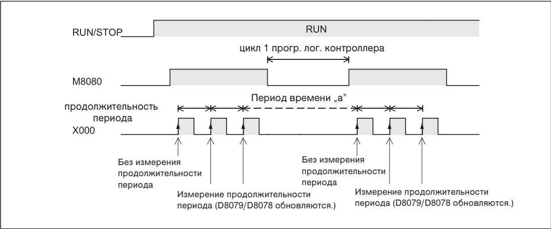
Рис. 8-9: Диаграмма изменения сигналов для вышеприведенного примера
