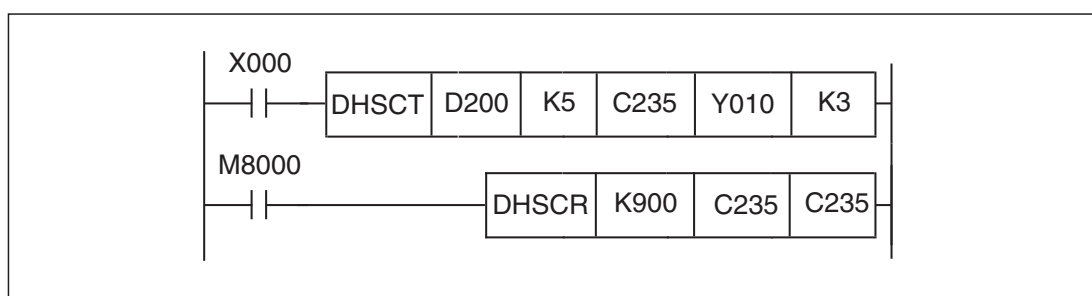
Рис. 7-301: Если счетчик C235 достиг значения „900”, этот счетчик сбрасывается.
