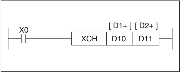
Рис. 6-31: Пример программирования XCH-инструкции без специального маркера
