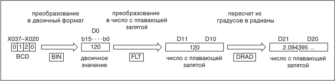
Рис. 7-107: Пример программы, которая при вводе 120° выводит результат преобразования 2.094395 рад.
