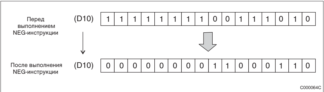
Рис. 6-55: Функция NEG-инструкции
