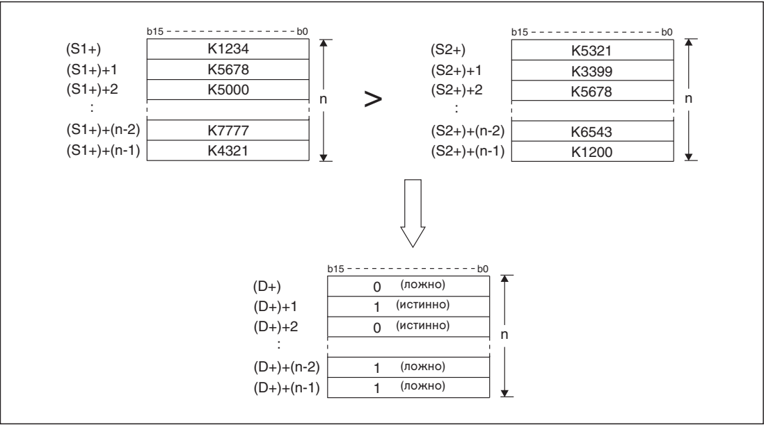
Рис. 7-201: В этом примере содержимые двух блоков данных с помощью команды BKCMР> сравниваются на „больше”.
