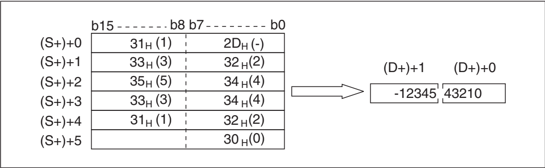
Рис. 7-283: Число „-1234543210” в кодировке ASCII преобразуется с помощью команды DDABIN.
