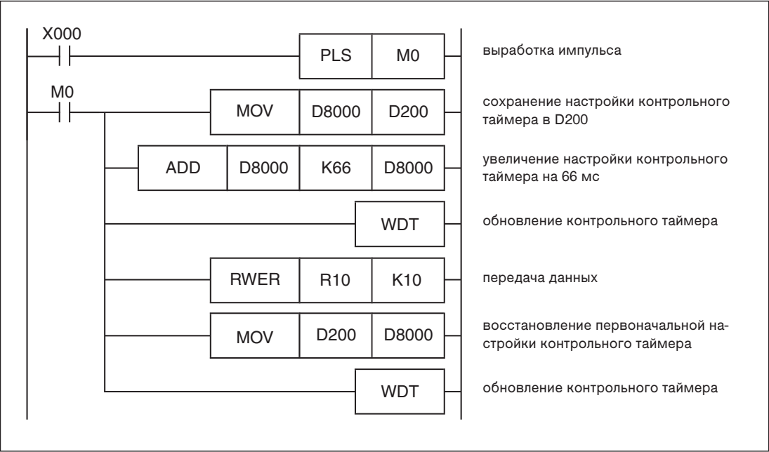
Рис. 7-319: В этом примере программы содержимые 10 расширенных регистров с R10 по R19 сохраняются в кассете памяти. На время передачи данных повышается настройка контрольного таймера.
