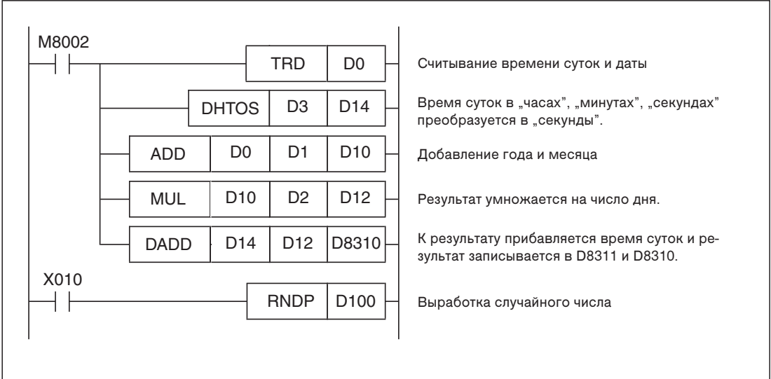
Рис. 7-182: В этом примере из времени суток и даты образуется основа для генерирования случайного числа.
