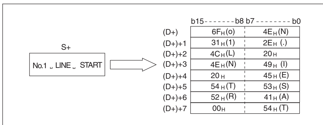
Рис. 7-180: В этом примере в байте после последнего знака вводится „00H”.
