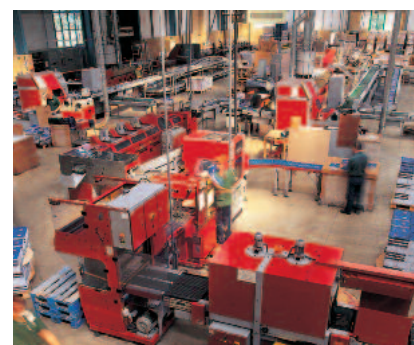
Пример управления конвейерами
