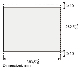
Dimensioni: mm
