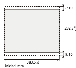
Unidad: mm
