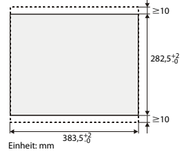
Einheit: mm
