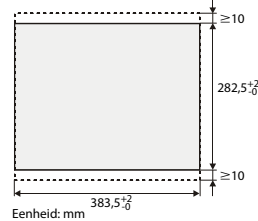
Eenheid: mm
