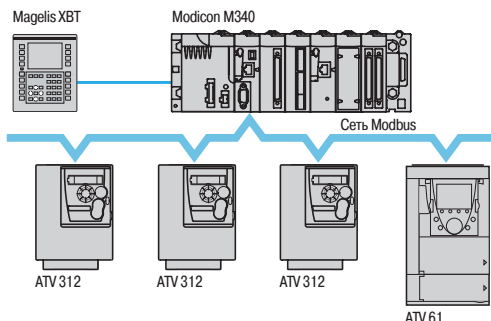
Пример конфигурации на шине Modbus
