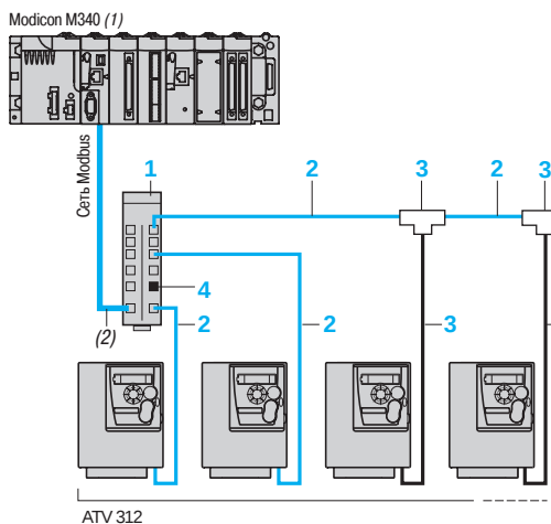
Пример архитектуры сети Modbus с подключением через разветвительный блок и разъемы RJ45
