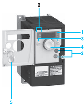
ATV 312H075M2 с открытой крышкой
