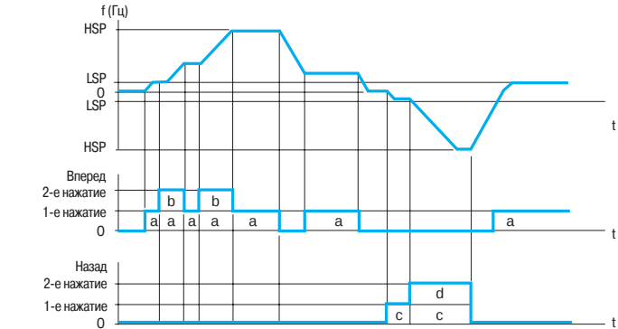
Пример с кнопками двойного действия и одним дискретным входом
