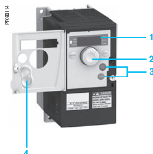
ATV 312H075M2 с открытой крышкой
