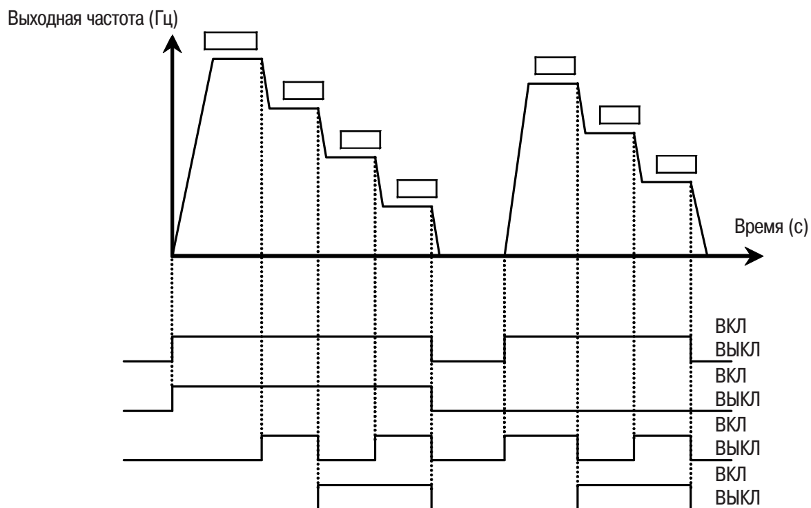
Пример предварительно заданных скоростей (7 скоростей)
