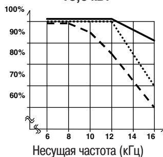
Выходной ток 18,5 кВт
