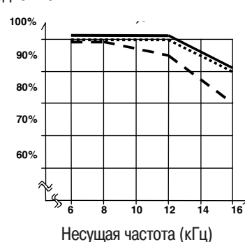
Выходной ток 7,5 кВт
