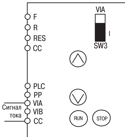
(5) Настройка внешним токовым сигналом (4 - 20 мА пост. тока)
