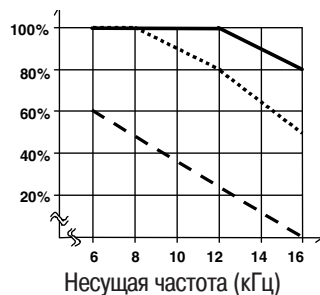
Выходной ток 37 кВт
