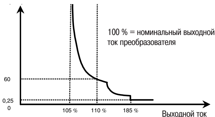
Характеристики защиты преобразователя от перегрузок
