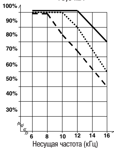
Выходной ток 18,5 кВт
