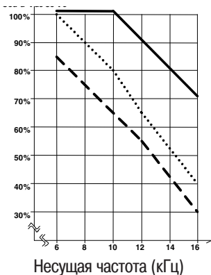
Выходной ток 30 кВт
