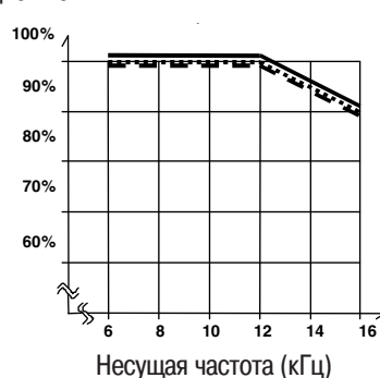
Выходной ток 5,5 кВт
