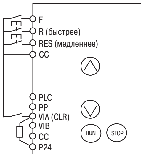
(6) Настройка внешним сигналом Быстрее/Медленнее
