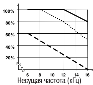
Выходной ток 55 кВт
