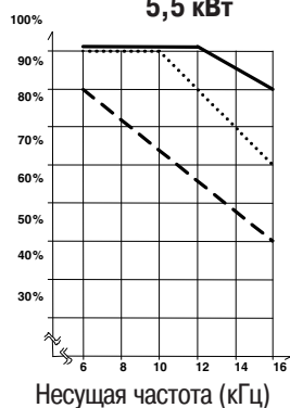
Выходной ток 5,5 кВт
