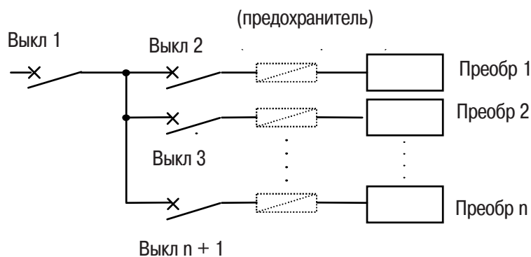
Отключение выбранного преобразователя
