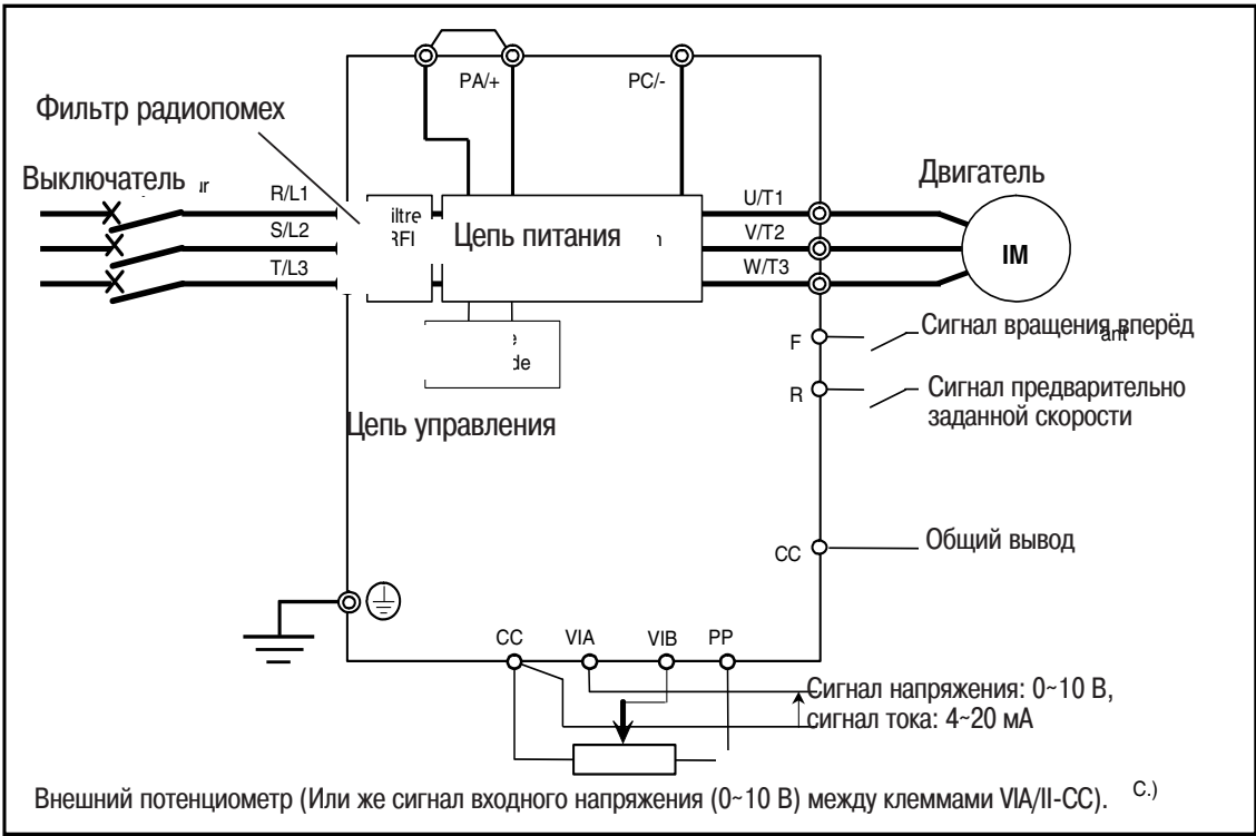
(1) Схема соединений
