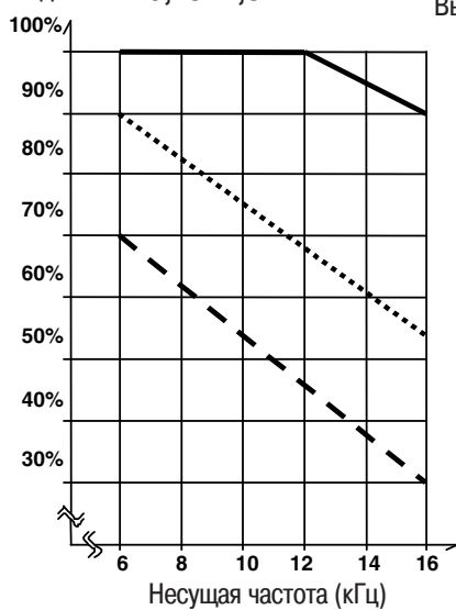
Выходной ток 0,75–7,5 кВт
