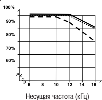
Выходной ток 15 кВт
