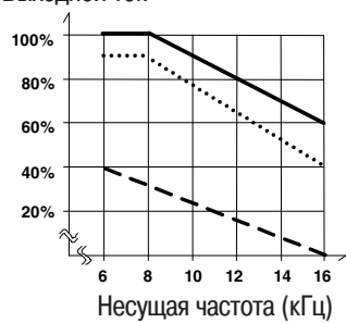
Выходной ток 45 кВт
