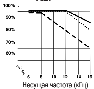
Выходной ток 4 кВт
