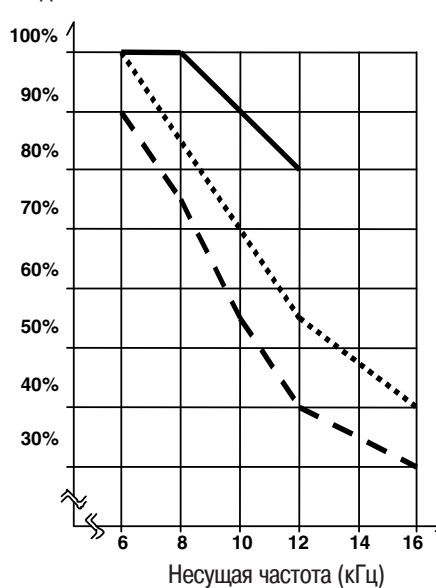
Выходной ток 30 кВт
