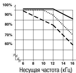
Выходной ток 11 кВт
