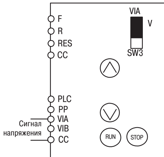
(3) Настройка внешним сигналом напряжения 1 (0 - 10 В пост. тока)
