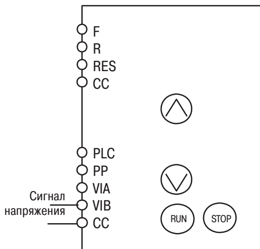
(4) Настройка внешним сигналом напряжения 2 (0 - 10 В пост. тока)
