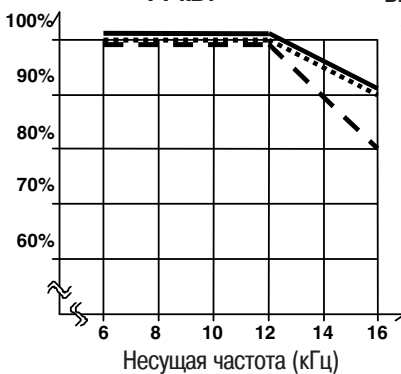
Выходной ток 11 кВт
