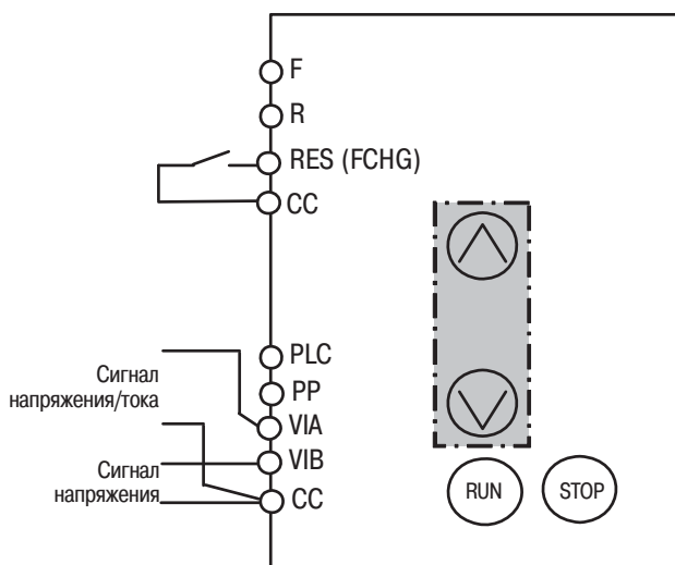
(11) Переключение между аналоговой настройкой и настройкой через клеммник со встроенного терминала
