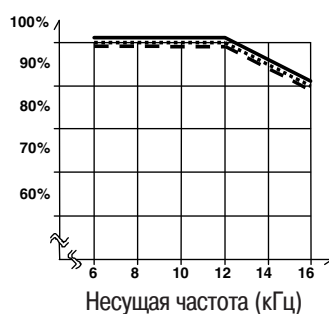
Выходной ток 7,5 кВт
