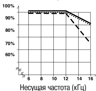
Выходной ток 15 кВт
