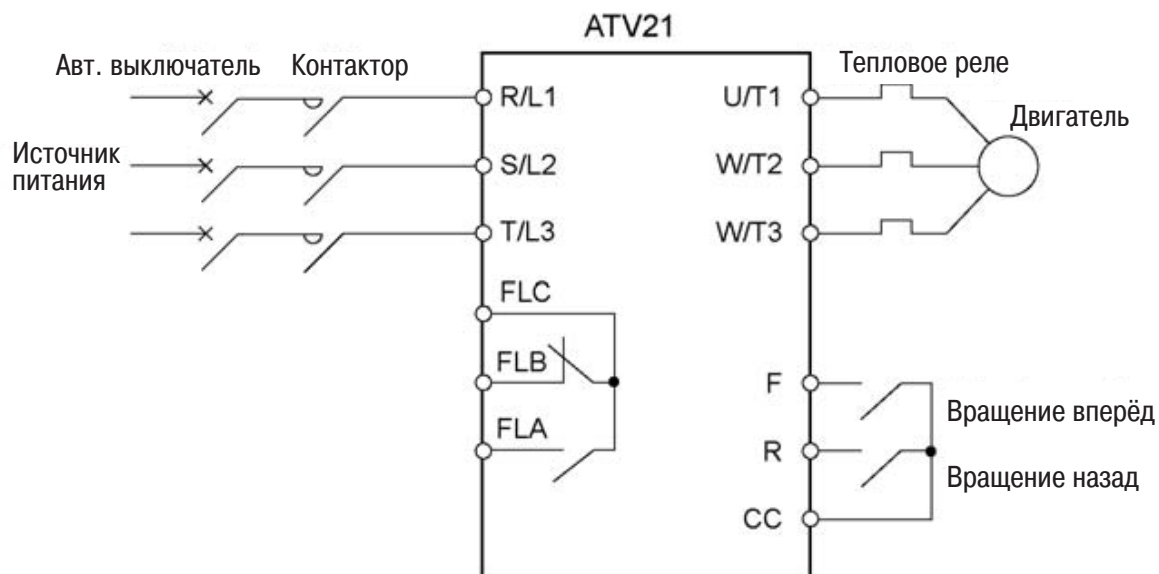
Пример подключения магнитного контактора к первичной цепи
