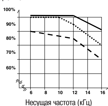
Выходной ток 4 кВт
