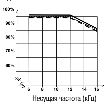
Выходной ток 11 кВт
