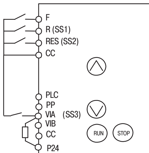
(7) Предварительно заданная скорость
