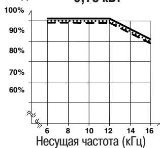
Выходной ток 0,75 кВт
