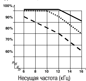
Выходной ток 2,2 кВт
