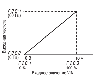
Пример настройки клеммы VIA (вход напряжения)
