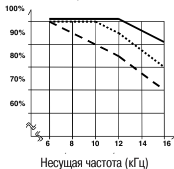
Выходной ток 1,5 кВт
