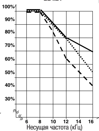
Выходной ток 22 кВт
