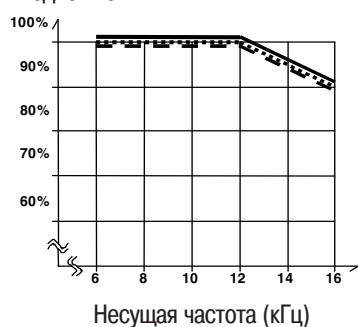
Выходной ток 0,75 кВт
