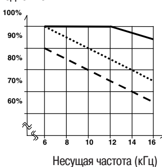
Выходной ток 18,5 кВт
