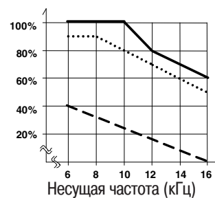
Выходной ток 75 кВт
