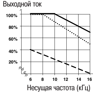
Выходной ток 55 кВт
