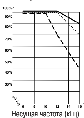
Выходной ток 2,2 кВт
