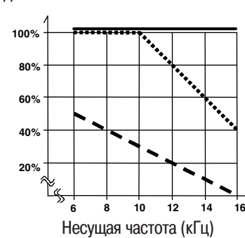
Выходной ток 30 кВт
