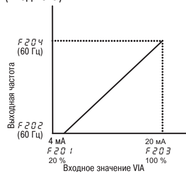
Пример настройки клеммы VIA (вход тока)
