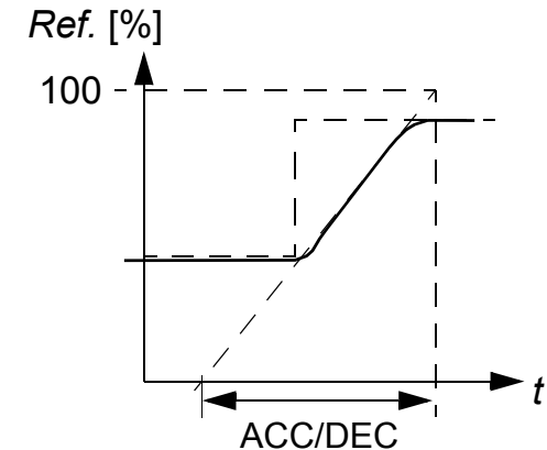
ACC/DEC 시간
