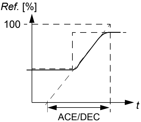
Tiempo ACE/DEC
