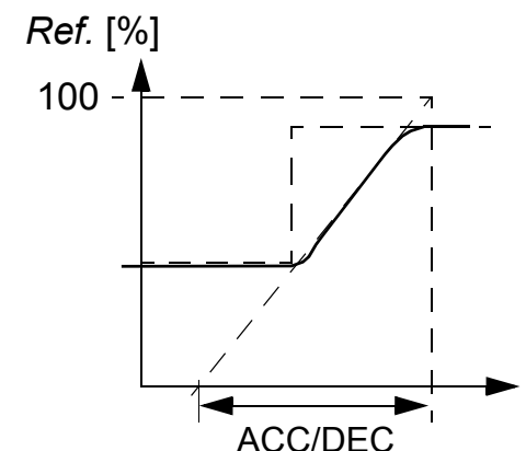
Tempo ACC/DEC
